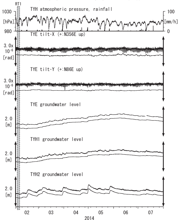
第7図 Tilt and groundwater level at TYE and TYH (時間値) (2014/02/01 00:00 - 2014/08/01 00:00 (JST))
