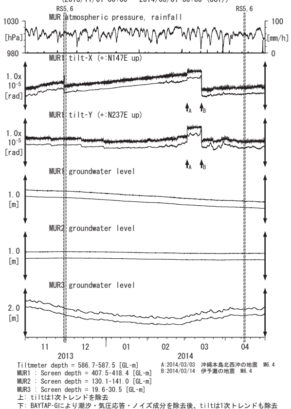
第26図 Tilt and groundwater level at MUR (時間値) (2013/11/01 00:00 - 2014/05/01 00:00 (JST))
