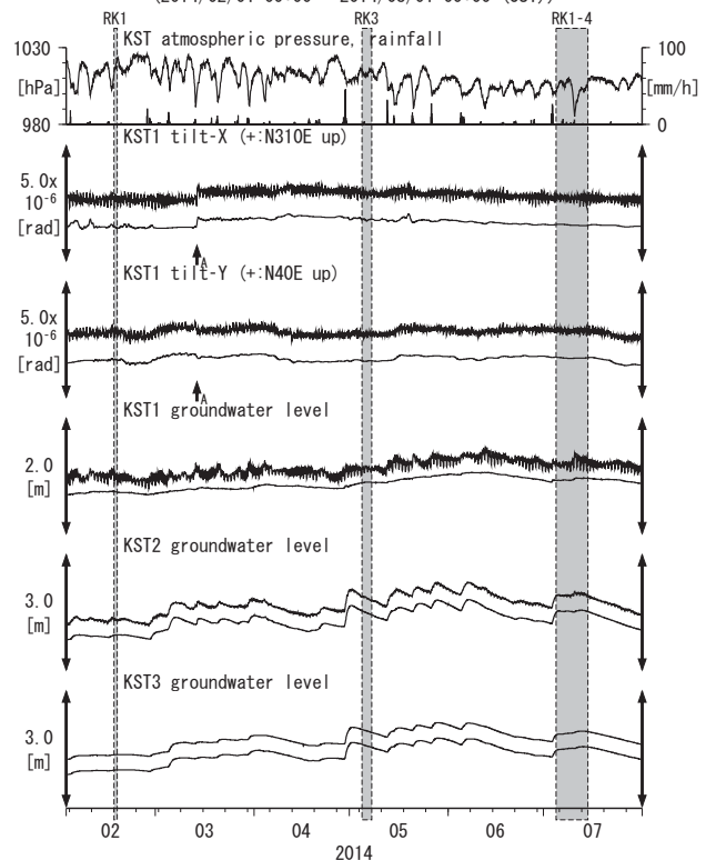
第20図 Tilt and groundwater level at KST (時間値) (2014/02/01 00:00 - 2014/08/01 00:00 (JST))
