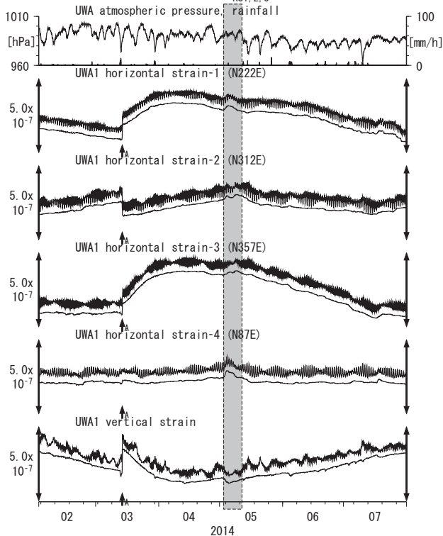
第33図 Crustal strains at UWA (時間値) (2014/02/01 00:00 - 2014/08/01 00:00 (JST))
