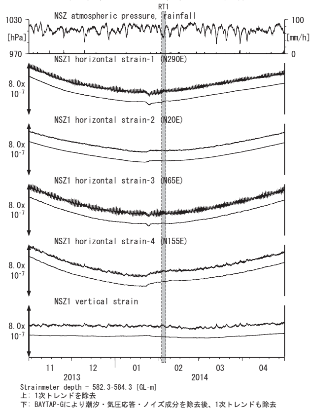
図4: Crustal strains changes at NSZ 西尾善明 (時間値) (2013/11/01 00:00 - 2014/05/01 00:00 (JST))
