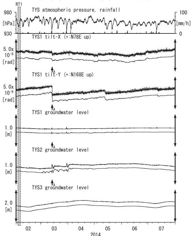
Tiltmeter depth = 585.9-586.7 [GL-m] A: 2014/03/14 伊予灘の地震 M6.2 TYS1 : Screen depth = 404.8-426.7 [GL-m] TYS2 : Screen depth = 148.8-154.3 [GL-m] TYS3 : Screen depth = 26.8-32.3 [GL-m] 上: tiltは1次トレンド除去 下: BAYTAP-Gにより潮汐・気圧応答・ノイズ成分除去、tiltは1次トレンドも除去
