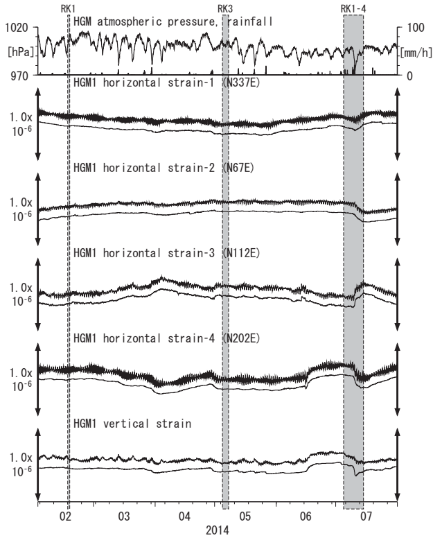
第17図 Crustal strains at HGM (時間値) (2014/02/01 00:00 - 2014/08/01 00:00 (JST))
