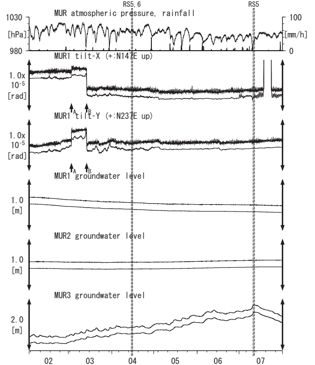
第26図 Tilt and groundwater level at MUR (時間値) (2014/02/01 00:00 - 2014/08/01 00:00 (JST))
