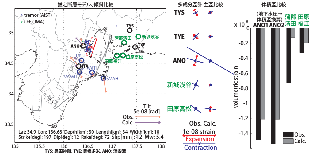
第58図: (上段)プレート境界面上のバッチ(断層面)をすべらせた際の、歪・傾斜の観測値と計算値の残差分布図。断層面サイズは固定(20x20km)。赤色矩形は最小残差の断層面を表す。このバッチのすべり量、Mwを下部に示している。
