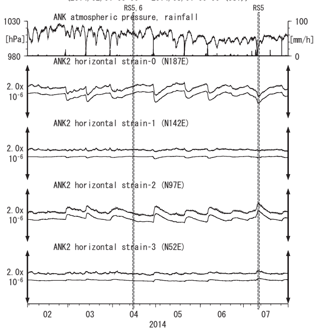
第23図 Crustal strains at ANK (時間値) (2014/02/01 00:00 - 2014/08/01 00:00 (JST))
