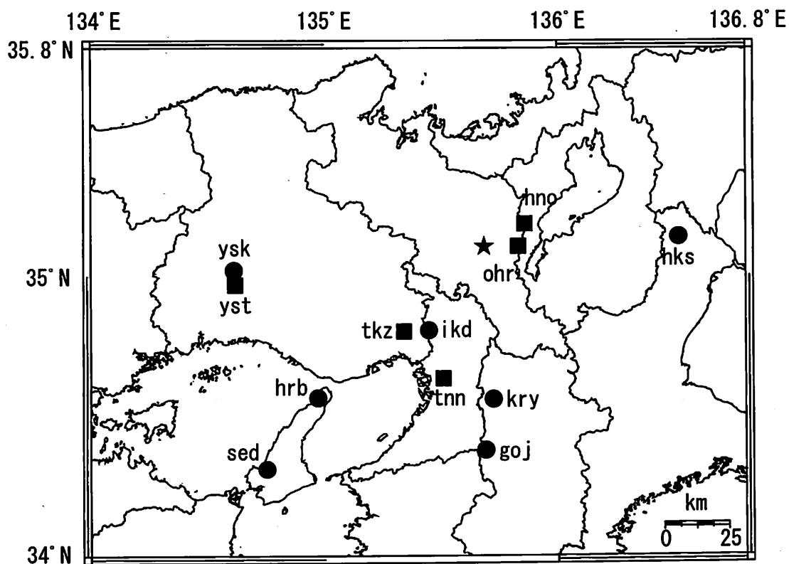
Fig.1 観測点分布図（●・■）。●は地下水のみの観測点で、■はボアホール型歪計を併設している観測点。★は、2014年6月11日の京都府南部の地震の震央。
