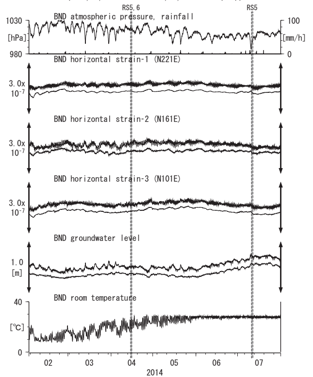
第22図 Crustal strains and groundwater level at BND (時間値) (2014/02/01 00:00 - 2014/08/01 00:00 (JST))
