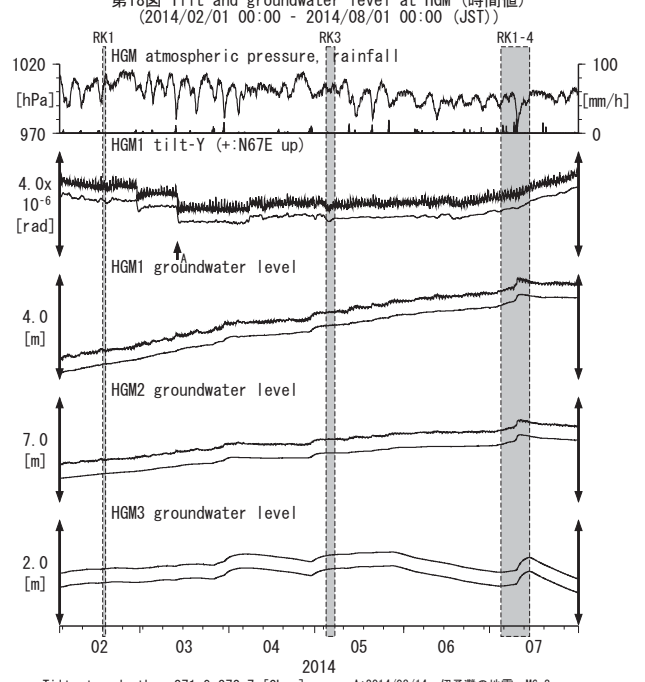
第18図 Tilt and groundwater level at HGM (時間値) (2014/02/01 00:00 - 2014/08/01 00:00 (JST))
