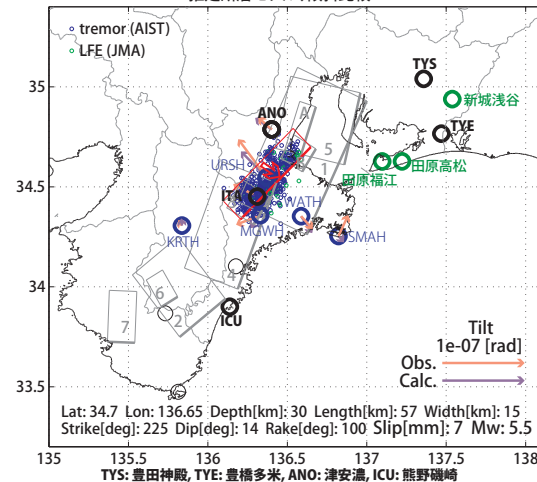
推定断層モデル、傾斜比較
