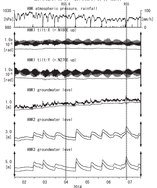
第24図 Tilt and groundwater level at ANK (時間値) (2014/02/01 00:00 - 2014/08/01 00:00 (JST))
