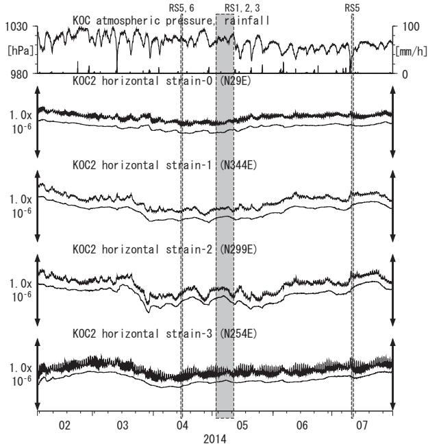
第27図 Crustal strains at KOC (時間値) (2014/02/01 00:00 - 2014/08/01 00:00 (JST))
