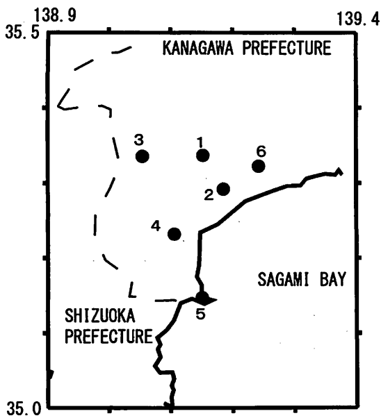
1図 地下水観測点の分布 (●) 10km
