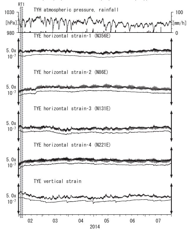
第6図 Crustal strain at TYE (時間値) (2014/02/01 00:00 - 2014/08/01 00:00 (JST))
