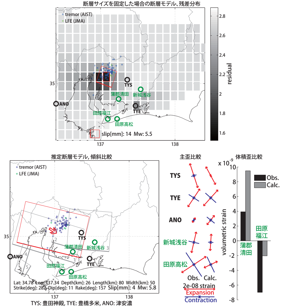
第66図: (上段)プレート境界面上のバッチ(断層面)をすべらせた際の、歪の観測値と計算値の残差分布図。断層面サイズは固定(20x20km)。赤色矩形は最小残差の断層面を表す。このバッチのすべり量、Mwを下部に示している。
