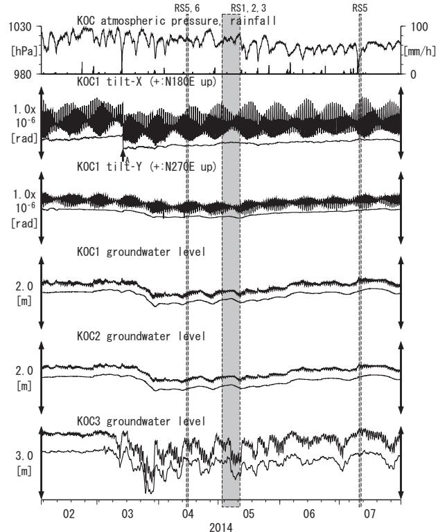
第28図 Tilt and groundwater level at KOC (時間値) (2014/02/01 00:00 - 2014/08/01 00:00 (JST))
