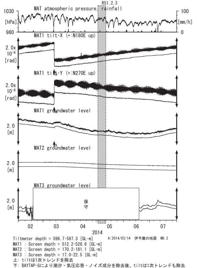
第36図 Tilt and groundwater level at MAT (時間値) (2014/02/01 00:00 - 2014/08/01 00:00 (JST))
