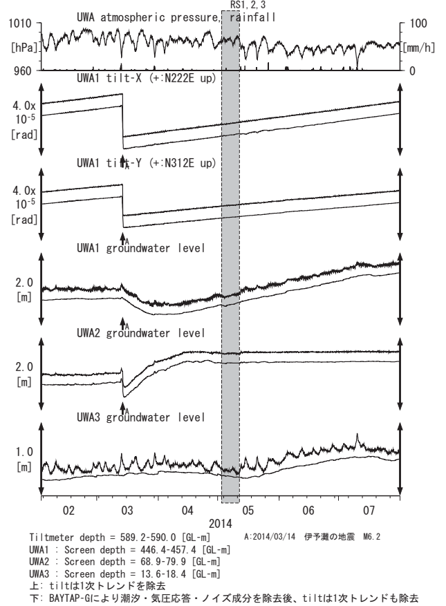
第34図 Tilt and groundwater level at UWA (時間値) (2014/02/01 00:00 - 2014/08/01 00:00 (JST))
