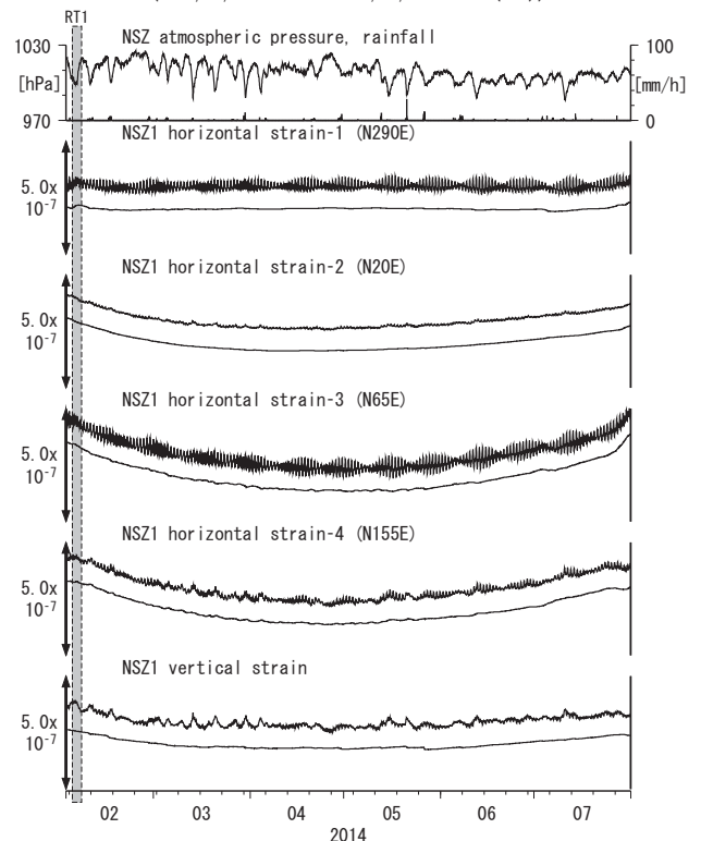
Strainmeter depth = 582.3-584.3 [GL-m] 上: 1次トレンドを除去 下: BAYTAP-Gにより潮汐・気圧応答・ノイズ成分を除去後、1次トレンドも除去
