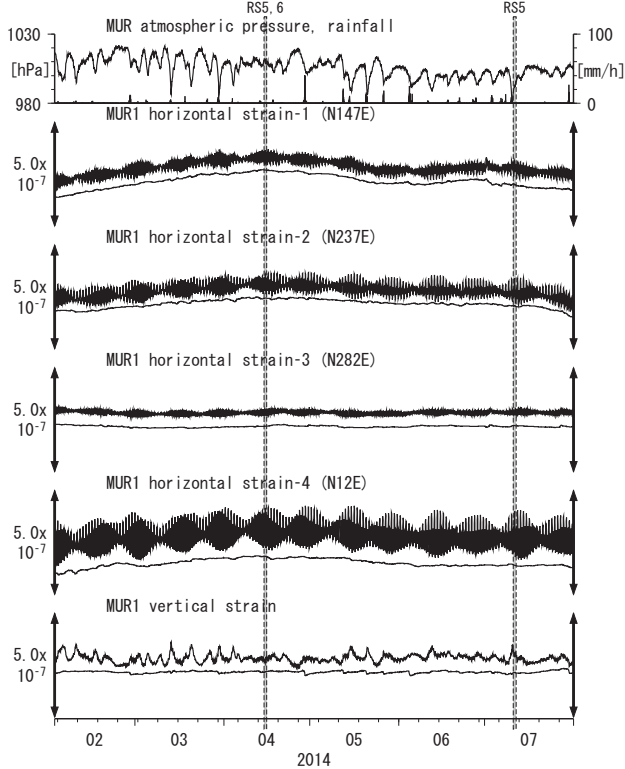
第25図 Crustal strains at MUR (時間値) (2014/02/01 00:00 - 2014/08/01 00:00 (JST))
