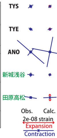
多成分歪計主歪比較
