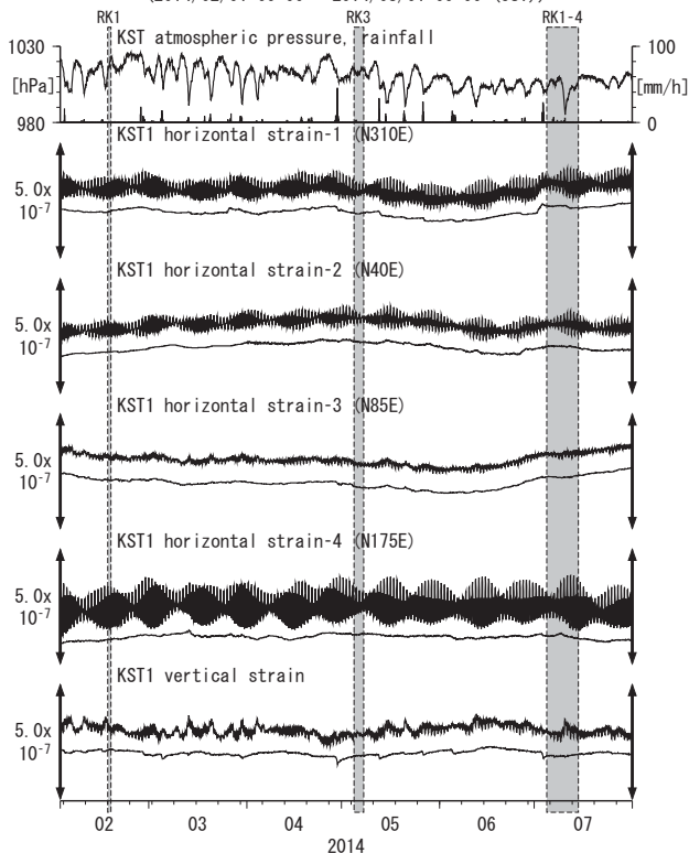
第19図 Crustal strains at KST (時間値) (2014/02/01 00:00 - 2014/08/01 00:00 (JST))
