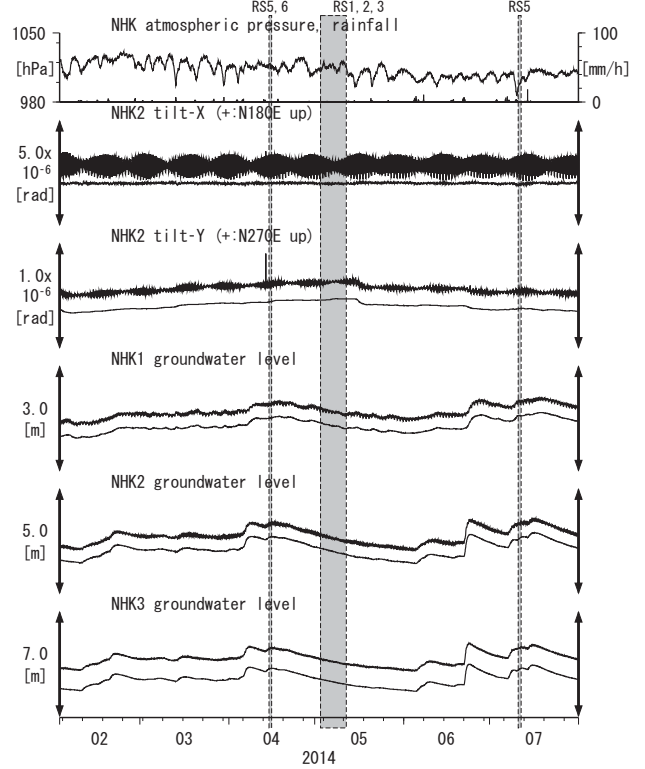
第38図 Tilt and groundwater level at NHK (時間値) (2014/02/01 00:00 - 2014/08/01 00:00 (JST))
