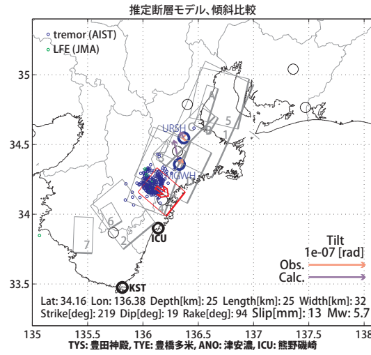
第62図: (上段)プレート境界面上のパッチ(断層面)をすべらせた際の、歪・傾斜の観測値と計算値の残差分布図。断層面サイズは固定(20x20km)。赤色矩形は最小残差の断層面を表す。このパッチのすべり量、Mwを下部に示している。 (下段)断層面推定結果(赤色矩形)。灰色の矩形は、最近周辺で発生した短期的SSEの推定断層面を示す。1: 2013年9月8-10日(Mw5.8), 2: 同年10月26-27日(Mw5.5), 3: 2014年1月9-11日午前(Mw5.6), 4: 同月11日午後-13日(Mw5.6), 5: 同月23-25日(Mw5.8), 6: 同年2月15日午後-18日(Mw5.3), 7: 同年6月26-28日午前(Mw5.5), A: 同年7月3-4日(Mw5.4), B: 同月5-6日(Mw5.6), C: 同月7-8日(Mw5.5), D: 同月9-10日(Mw5.8) 傾斜の観測値・モデルからの計算値との比較を地図内に、主歪の歪観測値・モデルからの計算値との比較を右側に示す。 (共通)小さい青色丸印は産総研による深部低周波微動、緑色丸印は気象庁一元化カタログによる低周波イベントの震央位置を示す。黒色は産総研の、青色は防災科研Hi-netの観測点名を示す。
