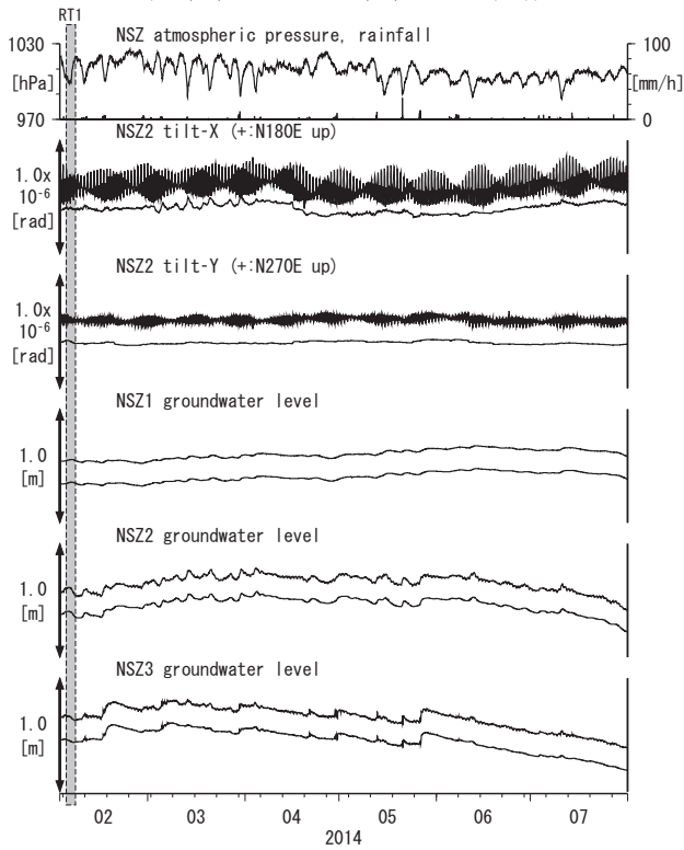
図5: Tilt and groundwater level changes at NSZ 西尾善明 (時間値) (2014/02/01 00:00 - 2014/08/01 00:00 (JST))
