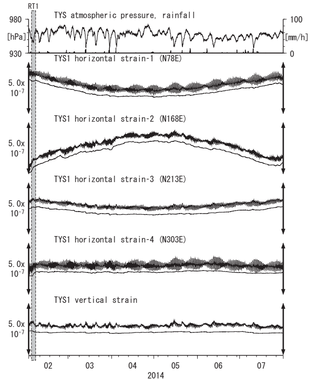
Strainmeter depth = 586.7-588.1 [GL-m] 上: 1次トレンドを除去 下: BAYTAP-Gにより潮汐・気圧応答・ノイズ成分を除去後、1次トレンドも除去
