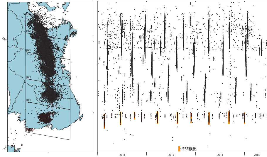
第55図: 2011年1月~2014年6月の紀伊半島における深部低周波微動の時空間分布図。橙色網掛けは、RK0領域において微動に伴う短期的SSEの発生が検出されたイベントを示す。RK0領域では、小規模な微動活動が年間8回前後発生している。
