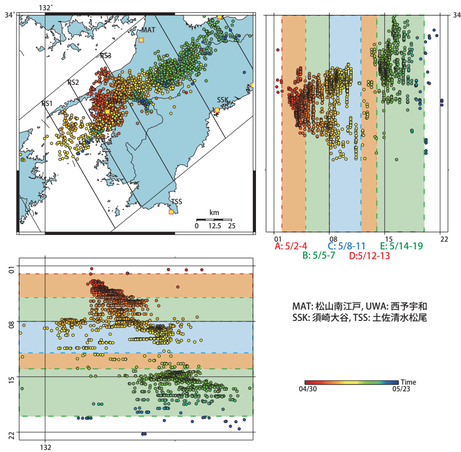
第45図: 2014/04/30 0:00 - 05/23 0:00 における四国西部～豊後水道周辺の深部低周波微動の時空間分布図。エンベロープ相関法により決定。
