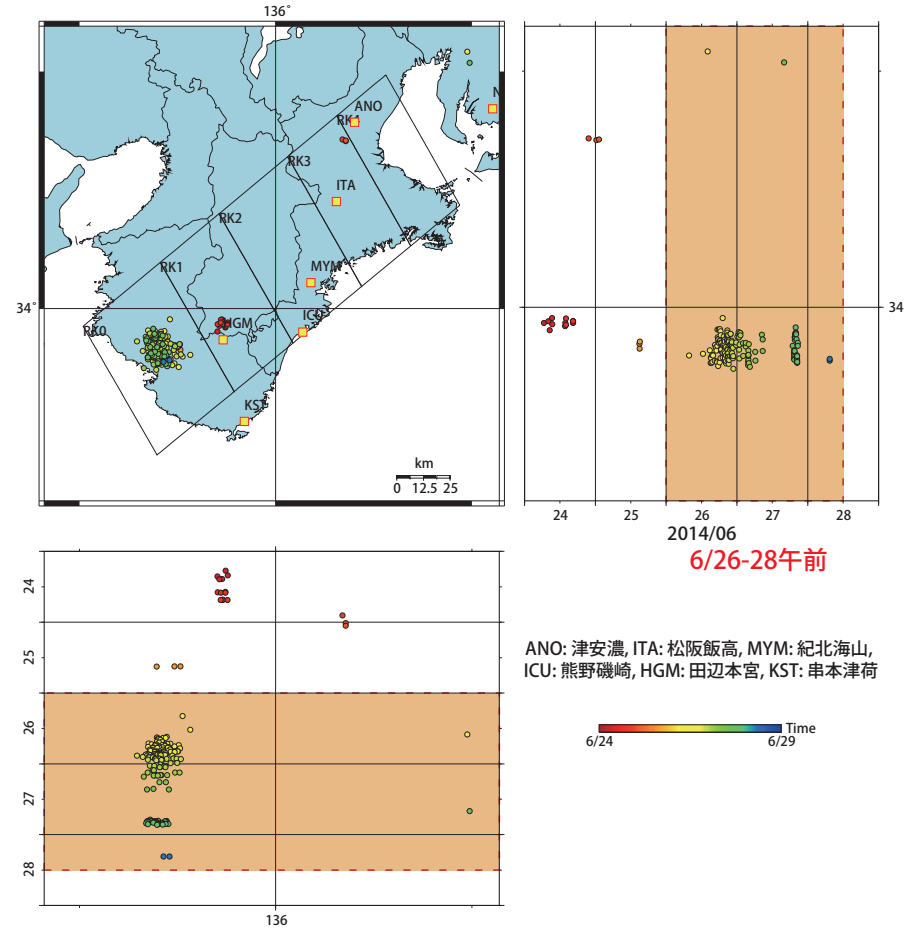
第52図: 2014/6/24 0:00 - 6/29 0:00 における紀伊半島周辺の深部低周波微動の時空間分布図。エンベロープ相関法により決定。
