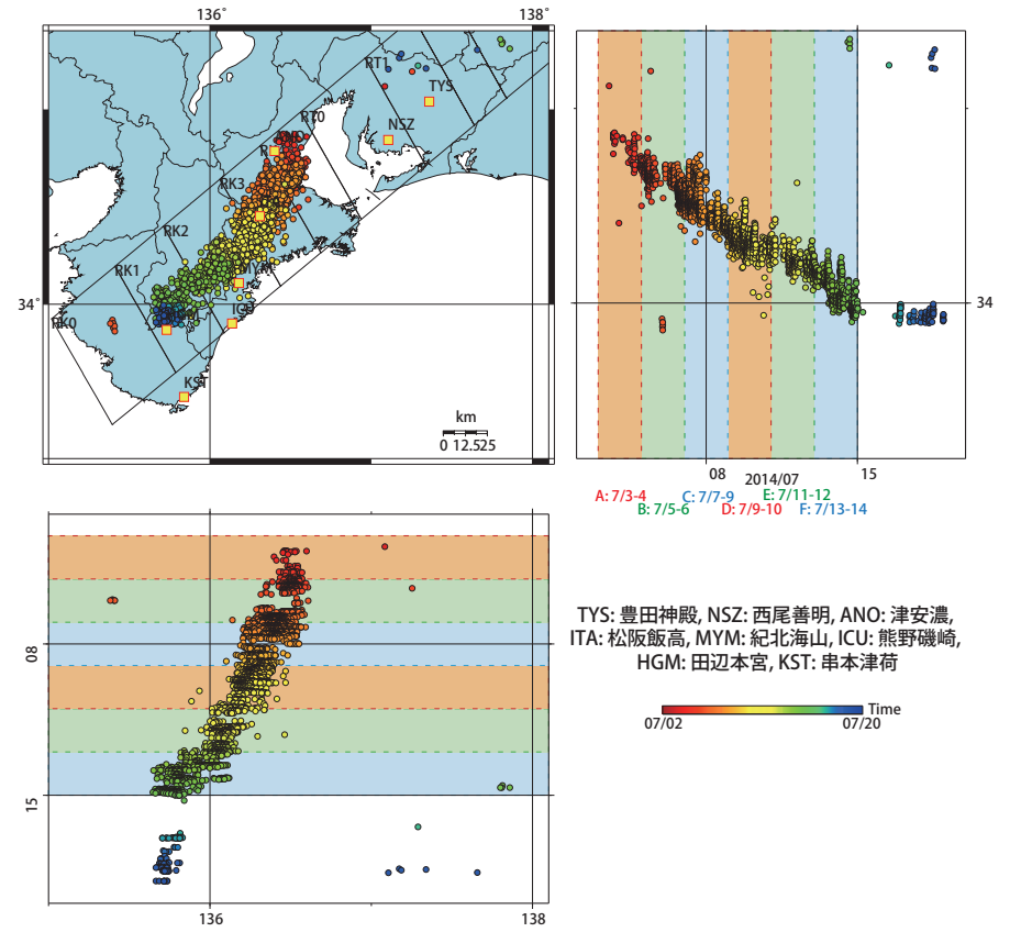
第56図: 2014/7/2 0:00 - 7/20 0:00 における紀伊半島および愛知県周辺の深部低周波微動の時空間分布図。エンベロップ相関法により決定。
