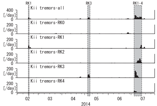
第42図 Deep low-frequency tremors in Kii Peninsula (日値) (2014/02/01 00:00 - 2014/08/01 00:00 (JST))
