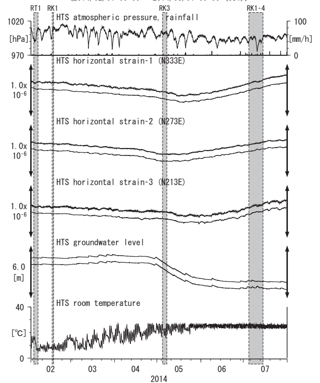
第8図 Crustal strains and groundwater level at HTS (時間値) (2014/02/01 00:00 - 2014/08/01 00:00 (JST))
