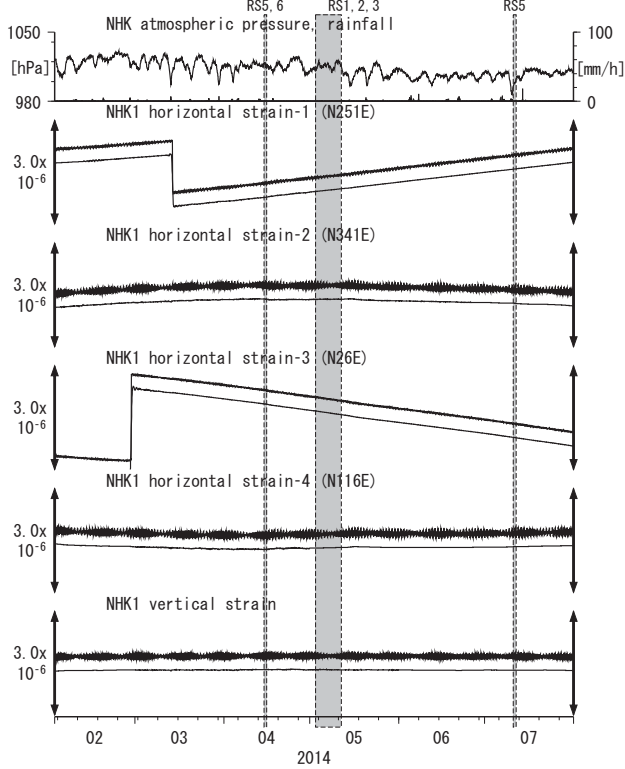
第37図 Crustal strains at NHK (時間値) (2014/02/01 00:00 - 2014/08/01 00:00 (JST))
