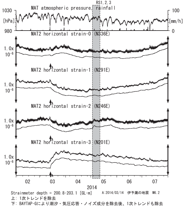
第35図 Crustal strains at MAT (時間値) (2014/02/01 00:00 - 2014/08/01 00:00 (JST))
