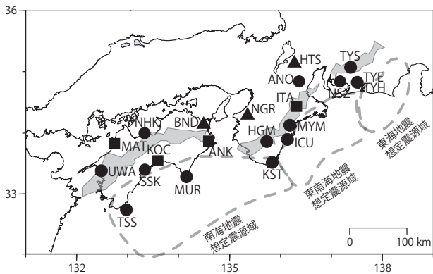
第1図: 地下水位観測点の分布図 (●・■・▲)。●はデジタル方式の石井式歪計・傾斜計を用いている新規観測点、■はGladwin式歪計・ミットヨ式傾斜計を併設している新規観測点、▲はアナログ方式の石井式歪計を併設している既存の観測点。灰色の領域は短期的SSE及び深部低周波変動が定常的に発生していると考えられる地域。
