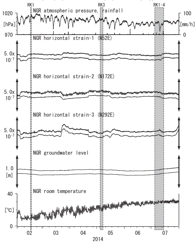
第21図 Crustal strains and groundwater level at NGR (時間値) (2014/02/01 00:00 - 2014/08/01 00:00 (JST))
