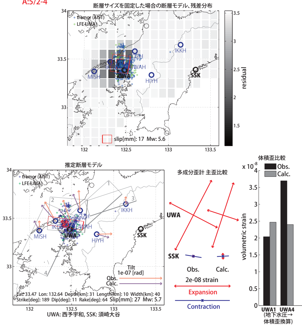
第47図: (上段)プレート境界面上のパッチ(断層面)をすべらせた際の、歪・傾斜の観測値と計算値の残差分布図。断層面サイズは固定(20x20km)。赤色矩形は最小残差の断層面を表す。このパッチのすべり量、Mwを下部に示している。
