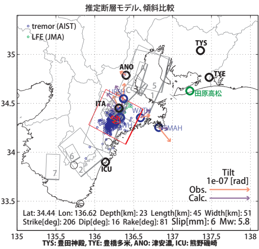
第61図: (上段)プレート境界面上のパッチ(断層面)をすべらせた際の、歪・傾斜の観測値と計算値の残差分布図。断層面サイズは固定(20x20km)。赤色矩形は最小残差の断層面を表す。このパッチのすべり量、Mwを下部に示している。 (下段)断層面推定結果(赤色矩形)。灰色の矩形は、最近周辺で発生した短期的SSEの推定断層面を示す。1: 2013年9月8-10日(Mw5.8), 2: 同年10月26-27日(Mw5.5), 3: 2014年1月9-11日午前(Mw5.6), 4: 同月11日午後-13日(Mw5.6), 5: 同月23-25日(Mw5.8), 6: 同年2月15日午後-18日(Mw5.3), 7: 同年6月26-28日午前(Mw5.5), A: 同年7月3-4日(Mw5.4), B: 同月5-6日(Mw5.6), C: 同月7-8日(Mw5.5) 傾斜の観測値・モデルからの計算値との比較を地図内に、主歪の歪観測値・モデルからの計算値との比較を右側に示す。 (共通)小さい青色丸印は産総研による深部低周波微動、緑色丸印は気象庁一元化カタログによる低周波イベントの震央位置を示す。黒色は産総研の、青色は防災科研Hi-netの観測点を、緑色は気象庁の観測点名を示す。
