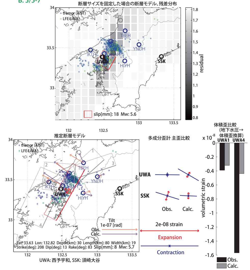
第48図: (上段)プレート境界面上のパッチ(断層面)をすべらせた際の、歪・傾斜の観測値と計算値の残差分布図。断層面サイズは固定(20x20km)。赤色矩形は最小残差の断層面を表す。このパッチのすべり量、Mwを下部に示している。
