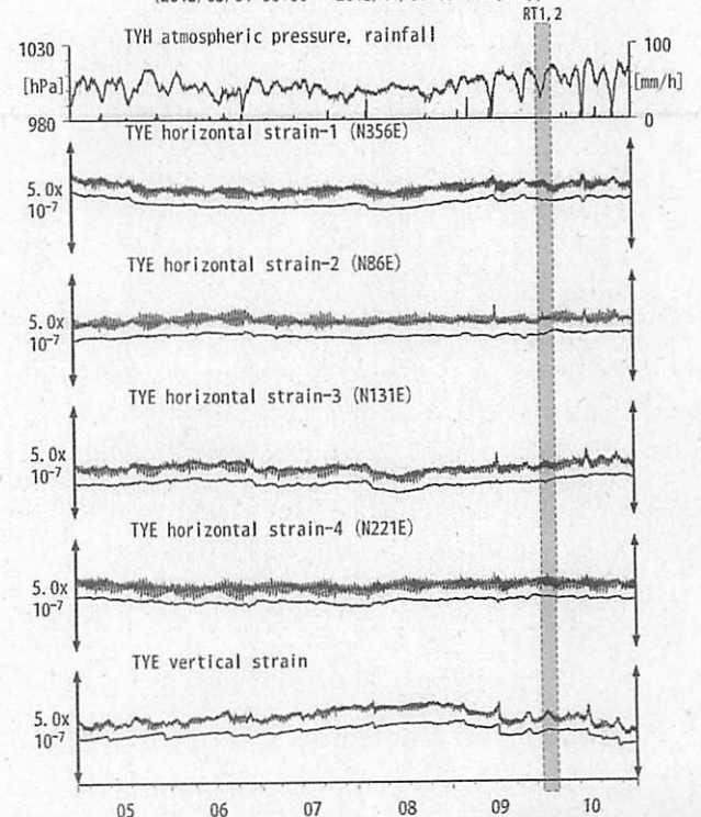
第4図 Crustal strain at TYE (時間値) (2013/05/01 00:00 - 2013/11/01 00:00 (JST))
