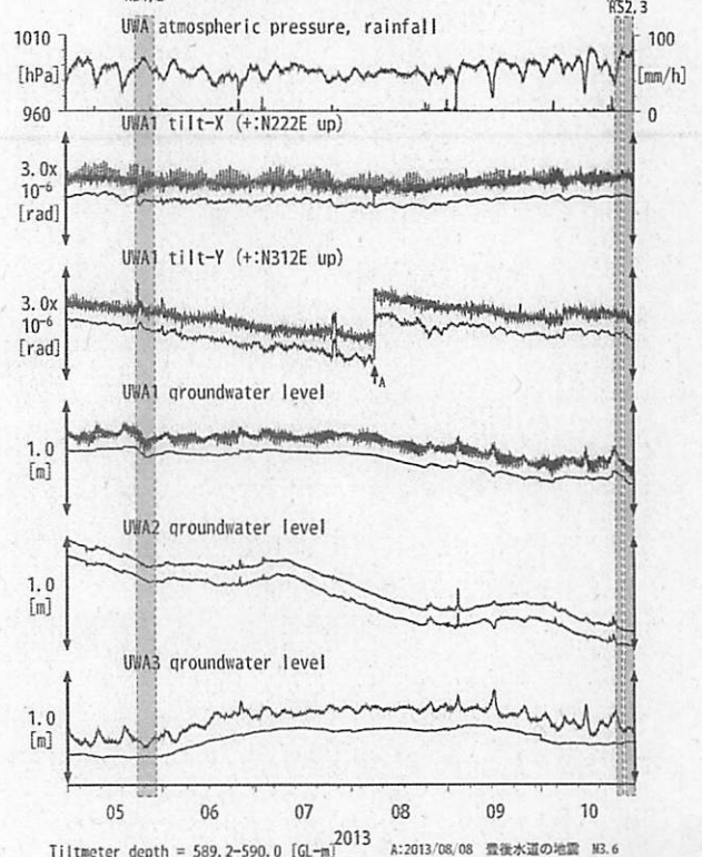
第32図 Tilt and groundwater level at UWA (時間値) (2013/05/01 00:00 - 2013/11/01 00:00 (JST))
