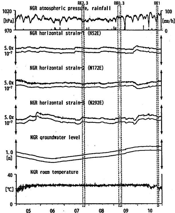
第19図 Crustal strains and groundwater level at NGR (時間値) (2013/05/01 00:00 - 2013/11/01 00:00 (JST))
