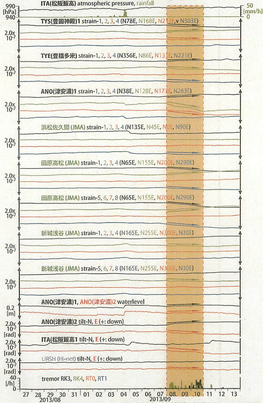
第45図: 愛知県~三重県における歪観測結果(時間値) (2013/08/27 00:00 - 2013/09/14 00:00 (JST))
