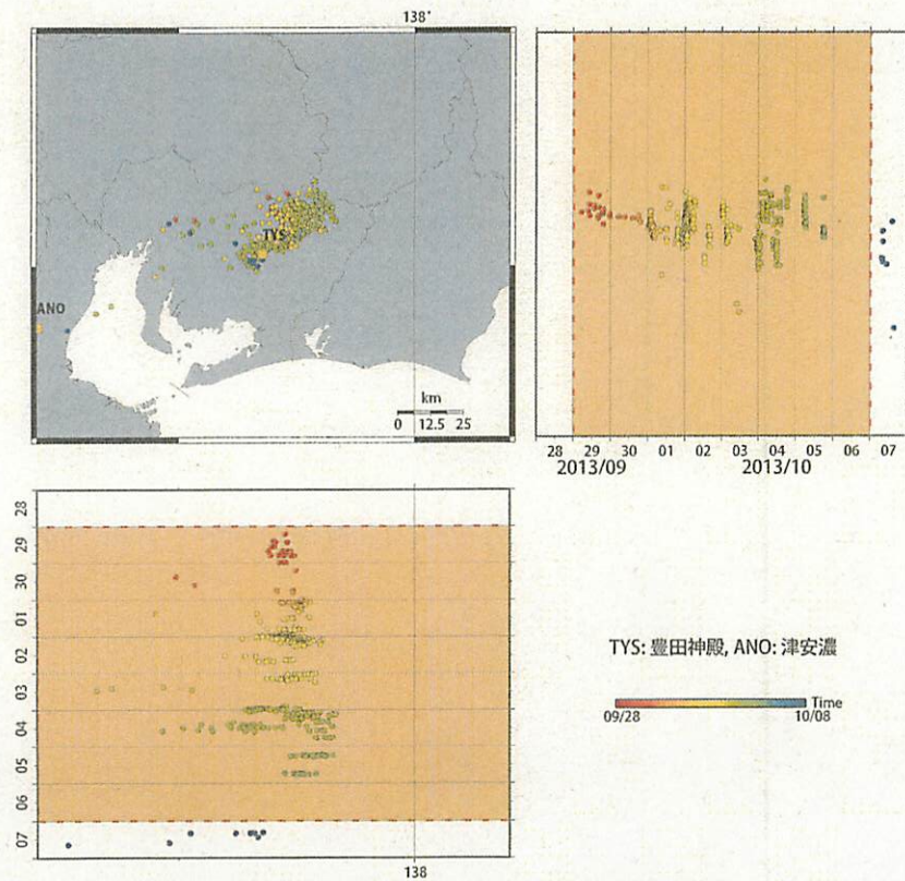
第47図: 2013/9/28 0:00 - 10/8 0:00 における愛知県周辺の深部低周波微動の時空間分布図。エンペローブ相関法により決定。
