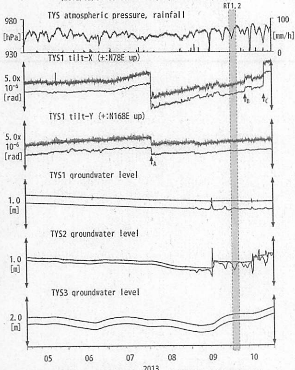
第3図 Tilt and groundwater level at TYS (時間値) (2013/05/01 00:00 - 2013/11/01 00:00 (JST))
