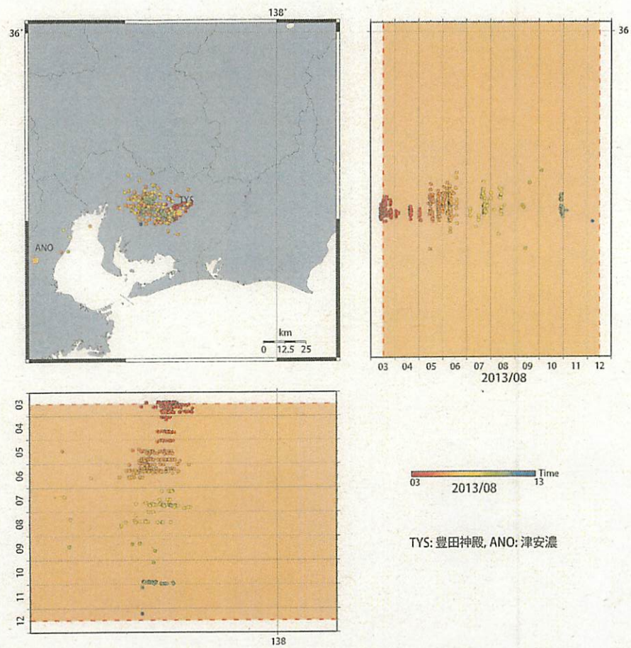
第41図: 2013/8/3 0:00 - 8/13 0:00 における愛知県周辺の深部低周波微動の時空間分布図。エンベロープ相関法により決定。
