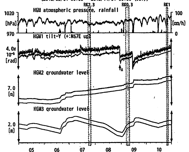
第16図 Tilt and groundwater level at HGM (時間値) (2013/05/01 00:00 - 2013/11/01 00:00 (JST))
