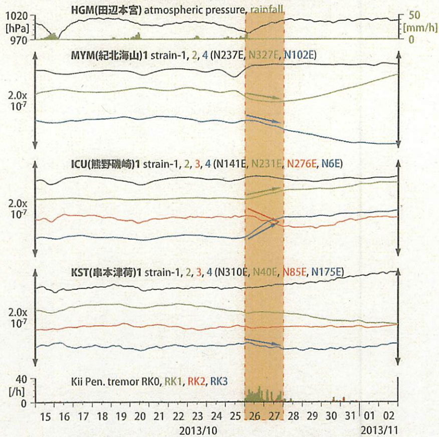
第51図: 紀伊半島における歪観測結果 (2013/10/15 00:00 - 2013/11/03 00:00 (JST))
