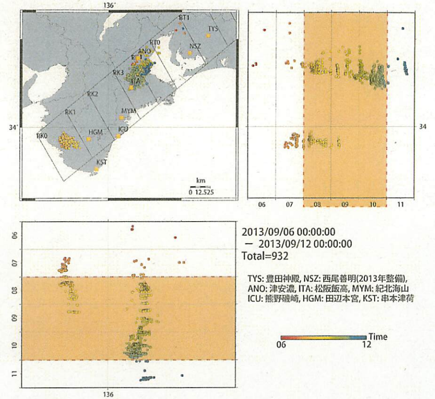
第44図: 2013/9/6 0:00 - 9/12 0:00 の紀伊半島および愛知県における深部低周波微動の時空間分布図。エンベロープ相関法により決定。
