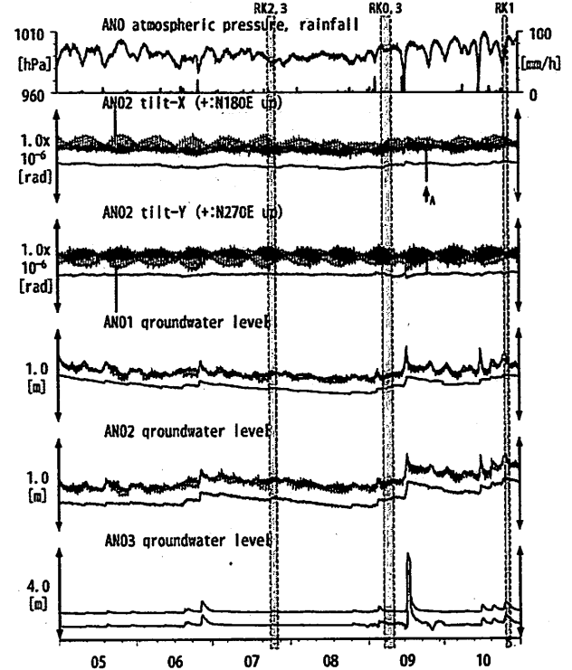
第8図 Tilt and groundwater level at ANO (時間値) (2013/05/01 00:00 - 2013/11/01 00:00 (JST))
