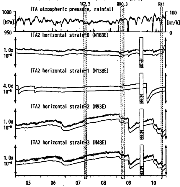
第9図 Crustal strains at ITA (時間値) (2013/05/01 00:00 - 2013/11/01 00:00 (JST))
