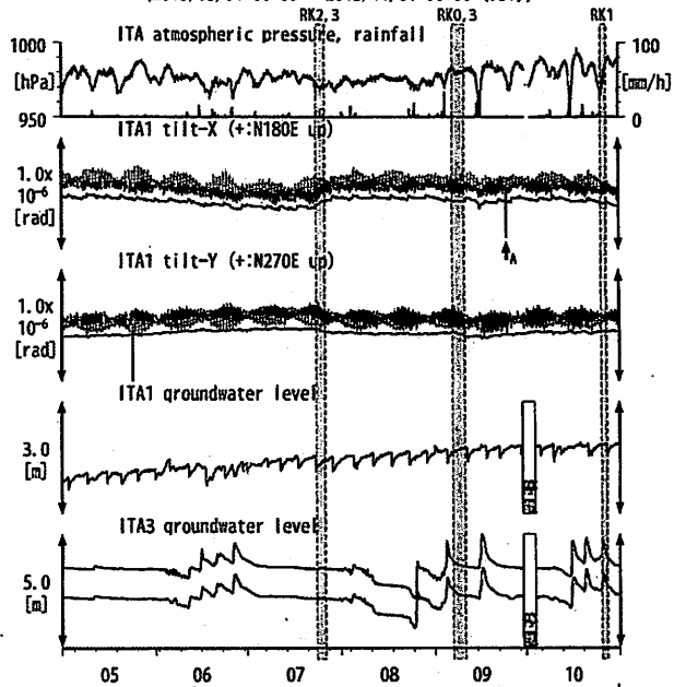
第10図 Tilt and groundwater level at ITA (時間値) (2013/05/01 00:00 - 2013/11/01 00:00 (JST))
