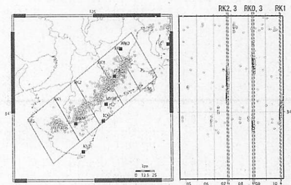
第37図 紀伊半島における深部低周波微動の時空間分布図(産総研による決定)
