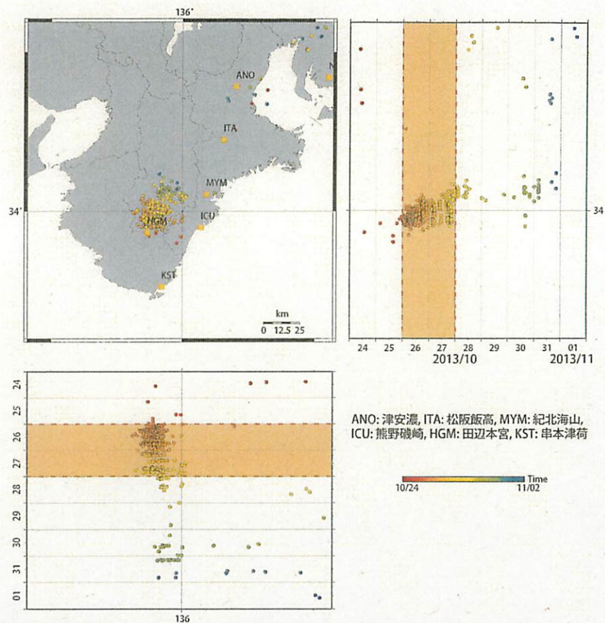
第50図: 2013/10/24 0:00 - 11/02 0:00 における紀伊半島の深部低周波微動の時空間分布図。エンベロープ相関法により決定。
