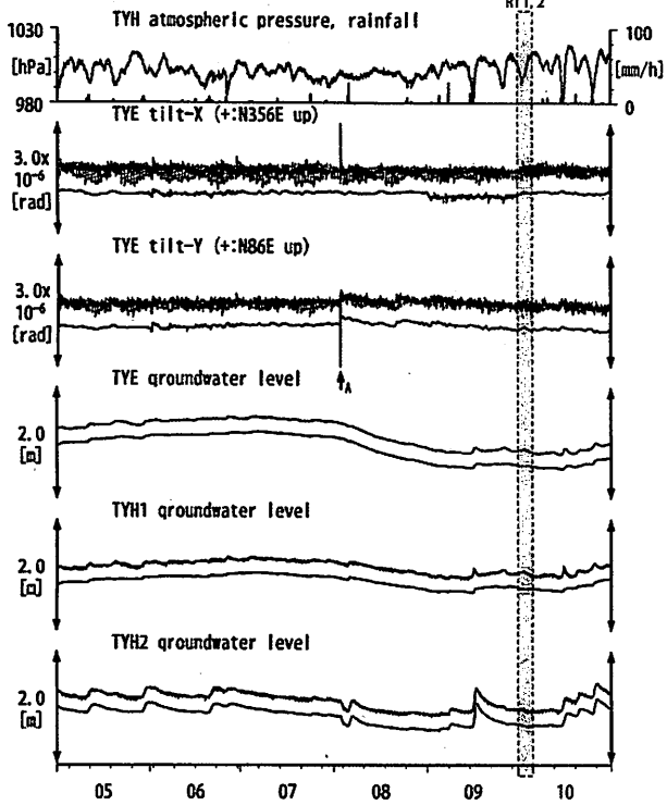
第5図 Tilt and groundwater level at TYE and TYH (時間値) (2013/05/01 00:00 - 2013/11/01 00:00 (JST))
