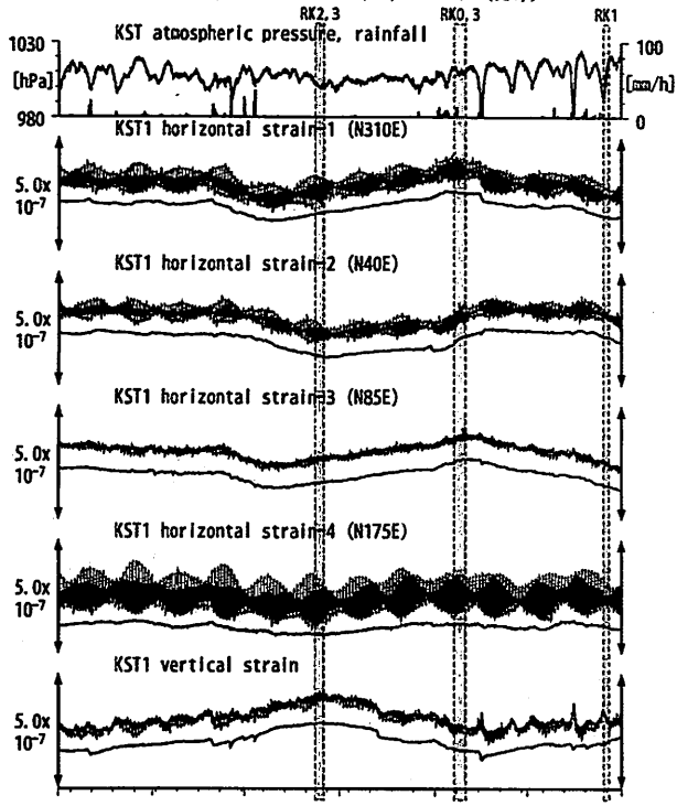
第17図 Crustal strains at KST (時間値) (2013/05/01 00:00 - 2013/11/01 00:00 (JST))
