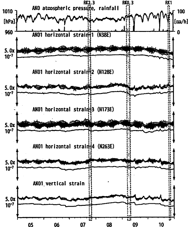
第7図 Crustal strains at ANO (時間値) (2013/05/01 00:00 - 2013/11/01 00:00 (JST))
