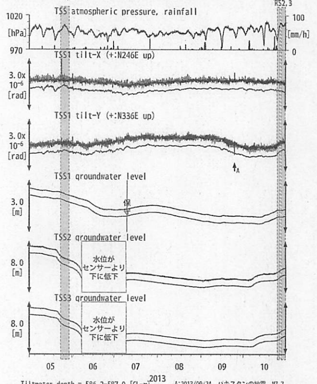
第30図 Tilt and groundwater level at TSS (時間値) (2013/05/01 00:00 - 2013/11/01 00:00 (JST))
