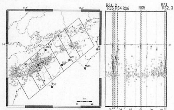
第39図 四国地方における深部低周波微動の時空間分布図(産総研による決定)
