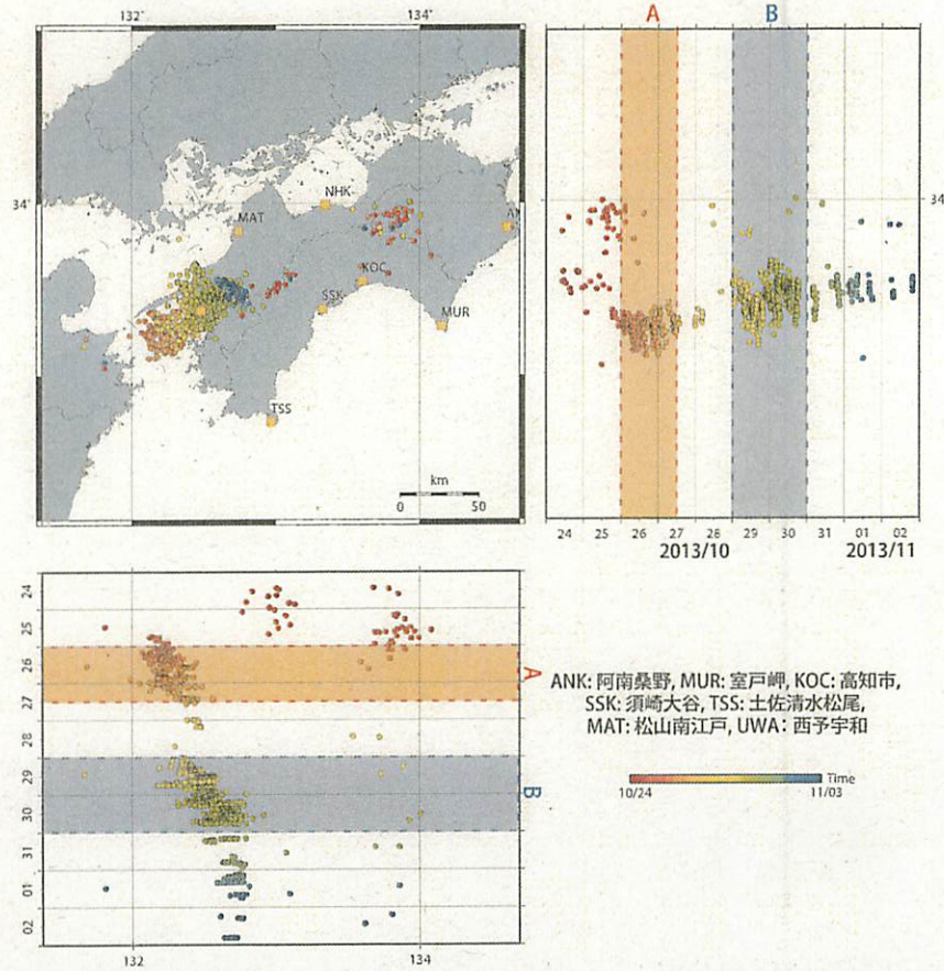
第53図: 2013/10/24 0:00 - 11/02 0:00 における四国地方の深部低周波微動の時空間分布図。エンベロープ相関法により決定。
