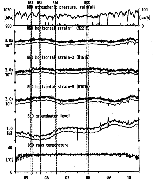
第20図 Crustal strains and groundwater level at BND (時間値) (2013/05/01 00:00 - 2013/11/01 00:00 (JST))
