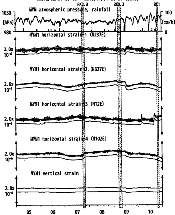
第11図 Crustal strains at MYM (時間値) (2013/05/01 00:00 - 2013/11/01 00:00 (JST))
