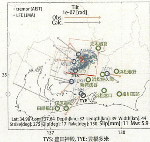
推定断層モデル、傾斜比較
