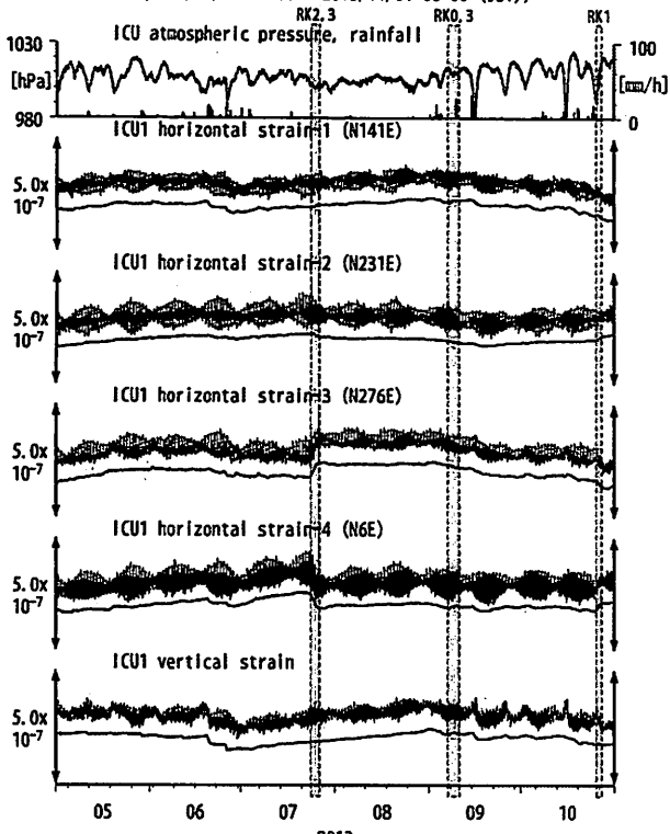
第13図 Crustal strains at ICU (時間値) (2013/05/01 00:00 - 2013/11/01 00:00 (JST))
