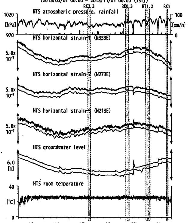
第6図 Crustal strains and groundwater level at HTS (時間値) (2013/05/01 00:00 - 2013/11/01 00:00 (JST))
