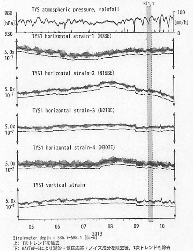
第2図 Crustal strains at TYS (時間値) (2013/05/01 00:00 - 2013/11/01 00:00 (JST))
