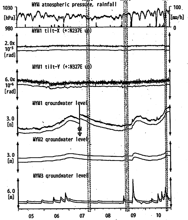
第12図 Tilt and groundwater level at MYM (時間値) (2013/05/01 00:00 - 2013/11/01 00:00 (JST))
