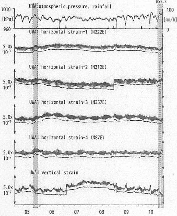
第31図 Crustal strains at UWA (時間値) (2013/05/01 00:00 - 2013/11/01 00:00 (JST))
