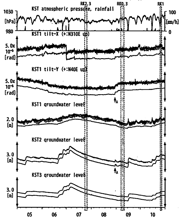
第18図 Tilt and groundwater level at KST (時間値) (2013/05/01 00:00 - 2013/11/01 00:00 (JST))
