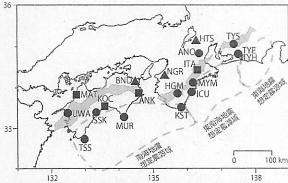
第1図: 地下水観測点の分布図 (●・■・▲)。●はデジタル方式の石井式歪計・傾斜計を用いている新規観測点、■はGladwin式歪計・ミットヨコ式傾斜計を併設している新規観測点、▲はアナログ方式の石井式歪計を併設している既存の観測点。灰色の領域は短期的SSE及び深部低周波微動が定期的に発生していると考えられる地域。
