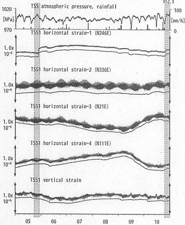
第29図 Crustal strains at TSS (時間値) (2013/05/01 00:00 - 2013/11/01 00:00 (JST))
