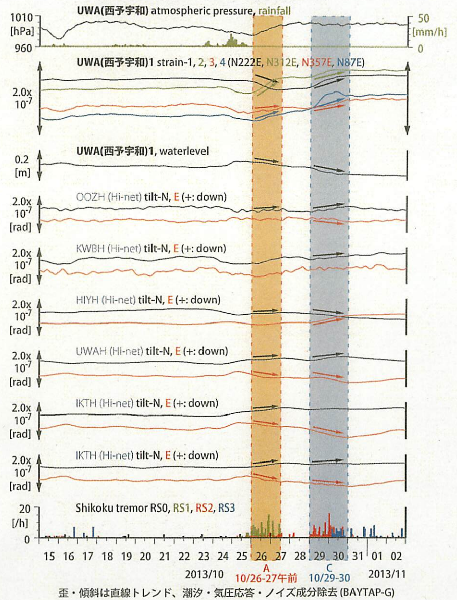
第54図: 四国における歪・傾斜観測結果 (2013/10/15 00:00 - 2013/11/03 00:00 (JST))
