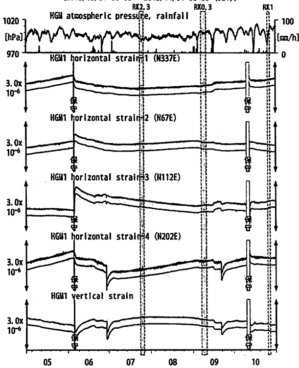
第15図 Crustal strains at HGM (時間値) (2013/05/01 00:00 - 2013/11/01 00:00 (JST))
