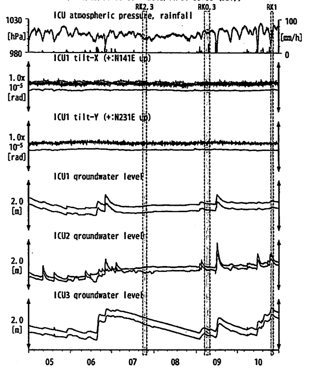
第14図 Tilt and groundwater level at ICU (時間値) (2013/05/01 00:00 - 2013/11/01 00:00 (JST))
