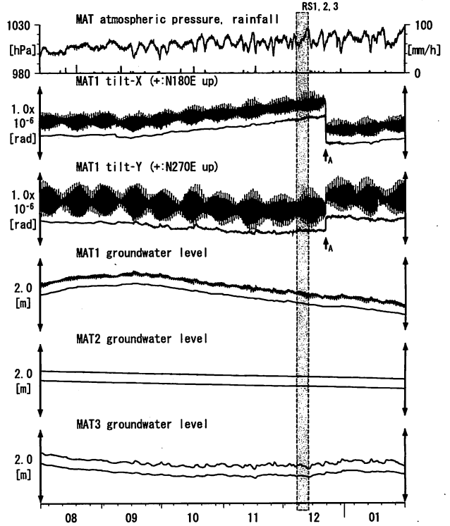
第34図 Tilt and groundwater level at MAT (時間値) (2012/08/01 00:00 - 2013/02/01 00:00)
