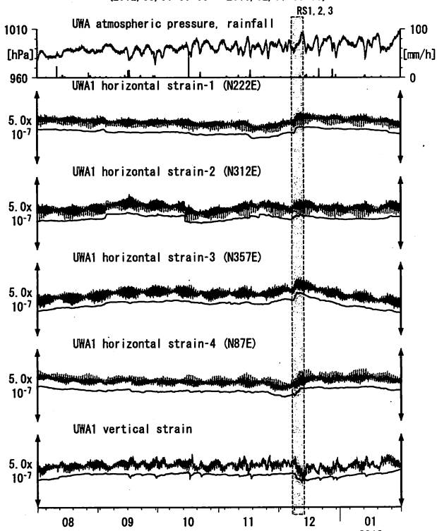
第31図 Crustal strains at UWA (時間値) (2012/08/01 00:00 - 2013/02/01 00:00)
