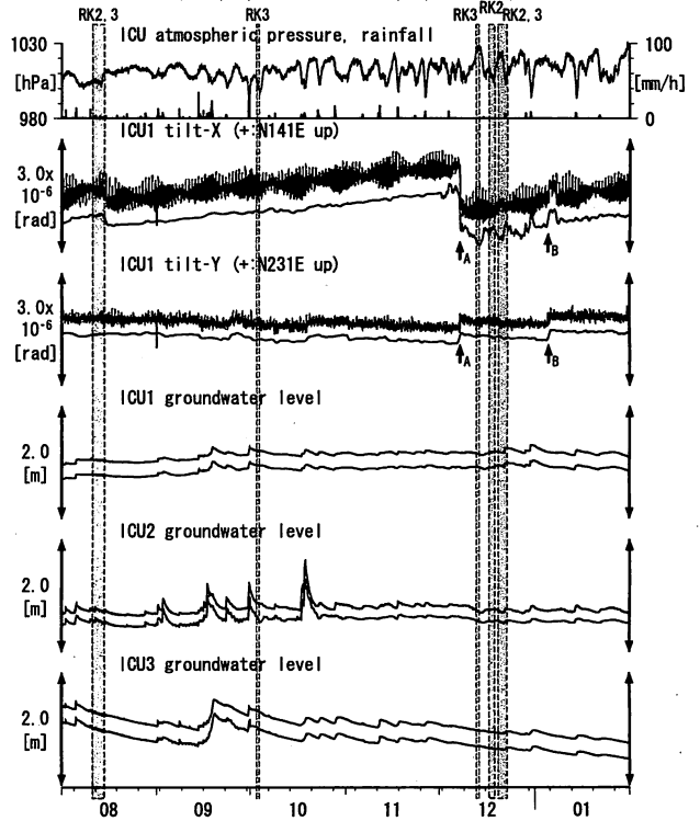
第14図 Tilt and groundwater level at ICU (時間値)
