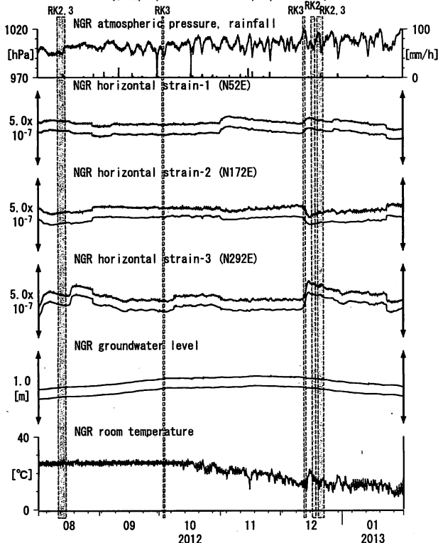
第19図 Crustal strains and groundwater level at NGR (時間値) (2012/08/01 00:00 - 2013/02/01 00:00)
