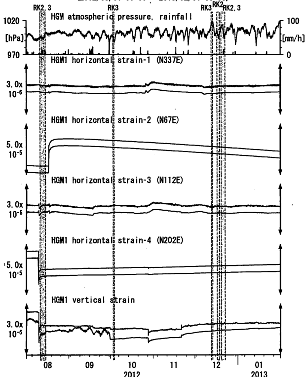
第15図 Crustal strains at HGM (時間値)
