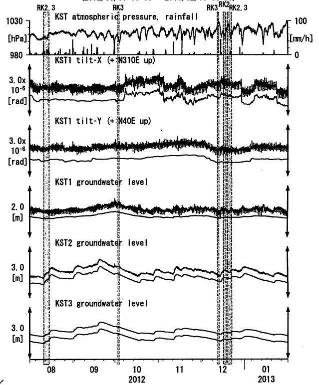
第18図 Tilt and groundwater level at KST (時間値) (2012/08/01 00:00 - 2013/02/01 00:00)
