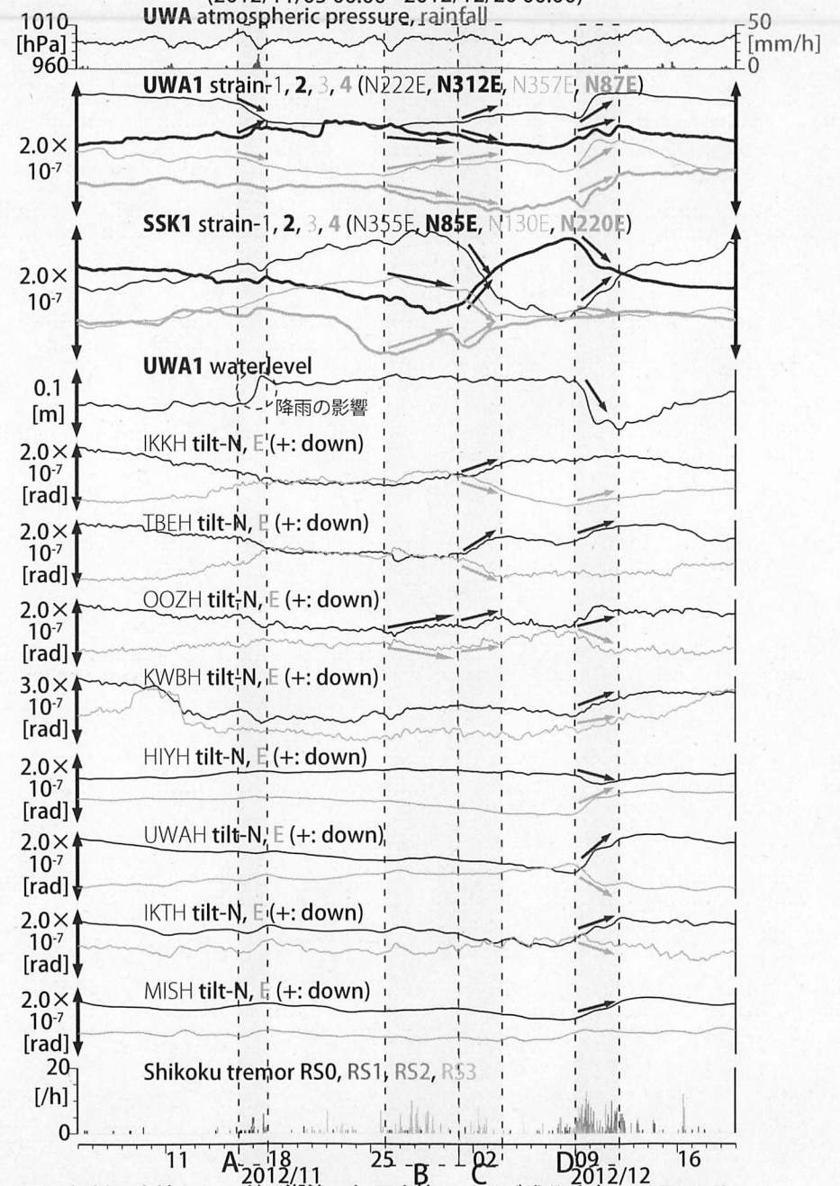
図42: 四国における歪・傾斜観測結果 (2012/11/05 00:00 - 2012/12/20 00:00)
