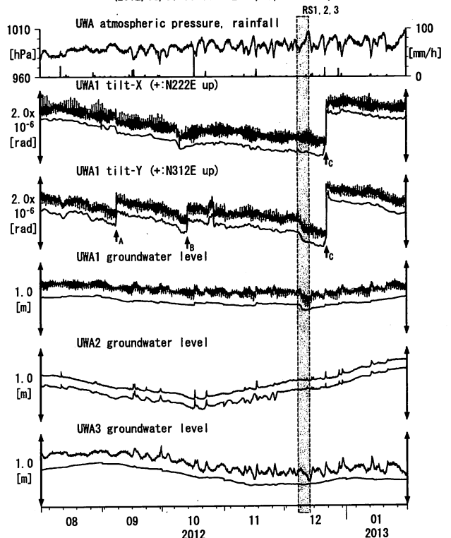
第32図 Tilt and groundwater level at UWA (時間値) (2012/08/01 00:00 - 2013/02/01 00:00)
