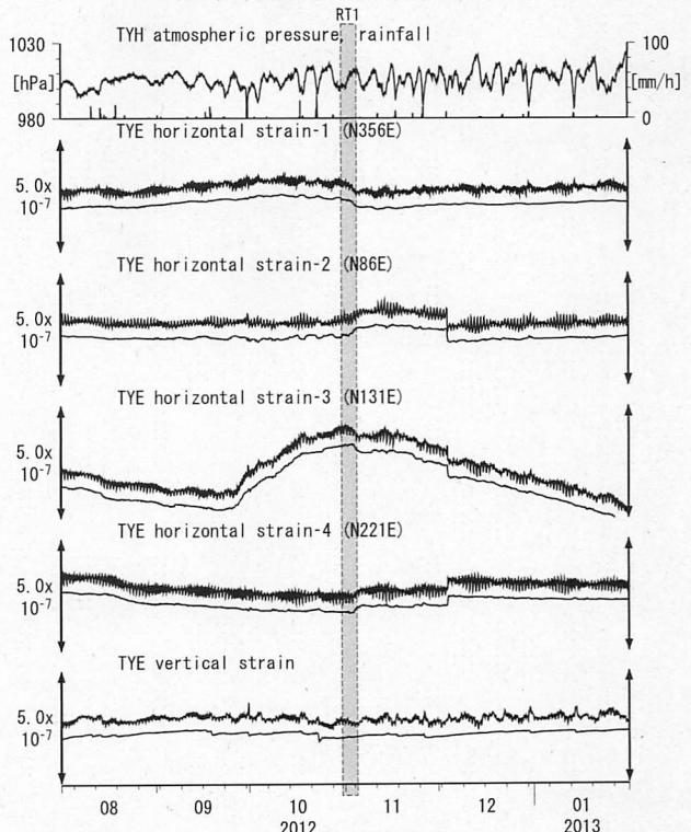
第4図 Crustal strain at TYE (時間値) (2012/08/01 00:00 - 2013/02/01 00:00)
