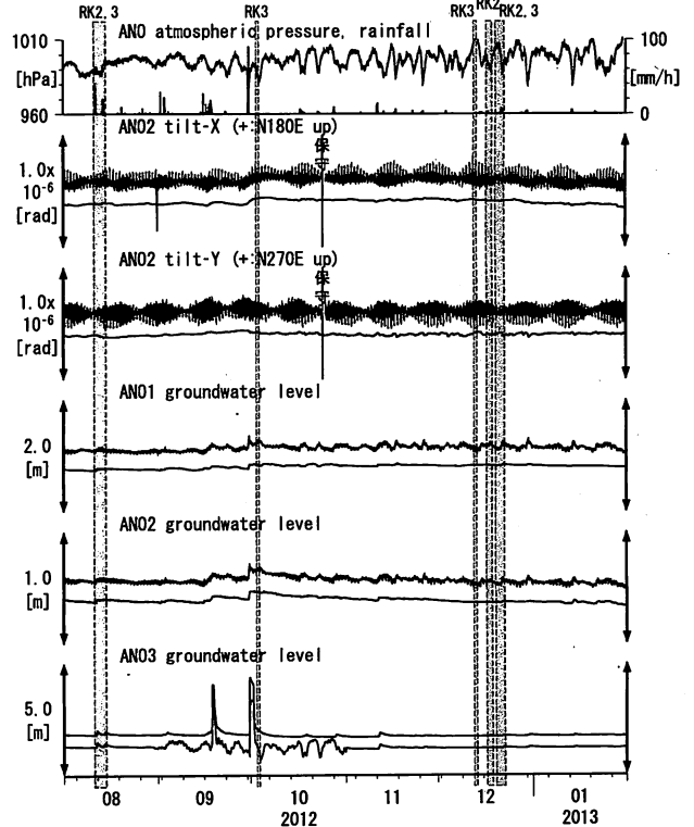
第8図 Tilt and groundwater level at ANO (時間値) (2012/08/01 00:00 - 2013/02/01 00:00)
