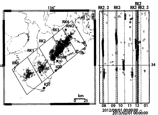
第37図 紀伊半島における深部低周波微動の時空間分布図(産総研による決定)
