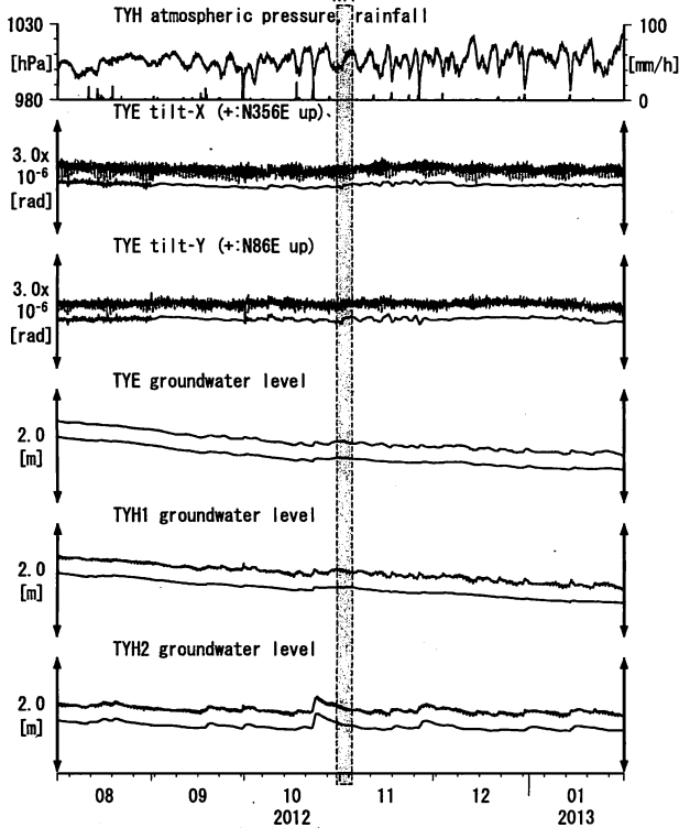
第5図 Tilt and groundwater level at TYE and TYH (時間値) (2012/08/01 00:00 - 2013/02/01 00:00)
