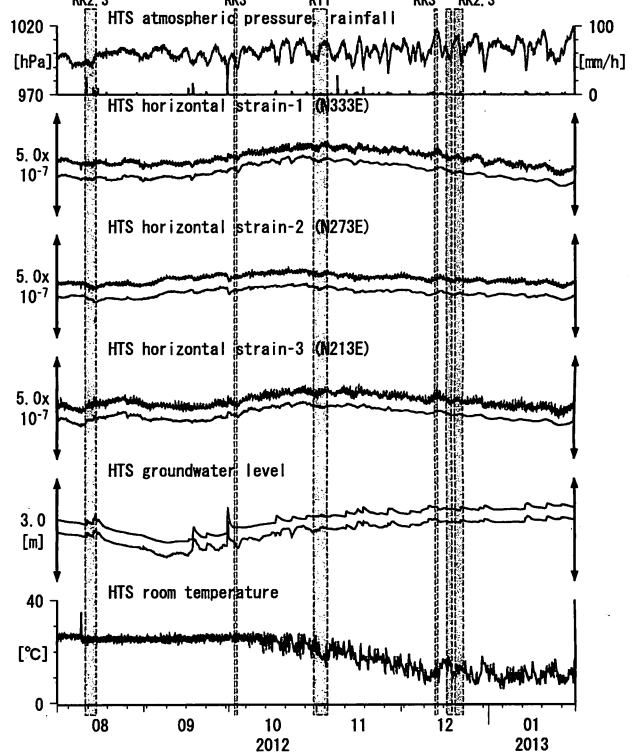
第6図 Crustal strains and groundwater level at HTS (時間値) (2012/08/01 00:00 - 2013/02/01 00:00)
