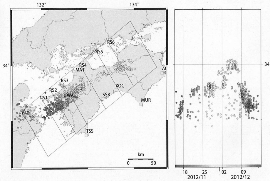
第41図: 2012/11/15 0:00 - 12/10 0:00 における四国地方の深部低周波微動の時空間分布図。 エンベロープ相関法により決定。
