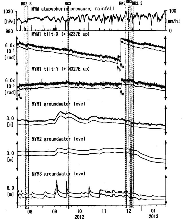
第12図 Tilt and groundwater level at MYM (時間値) (2012/08/01 00:00 - 2013/02/01 00:00)
