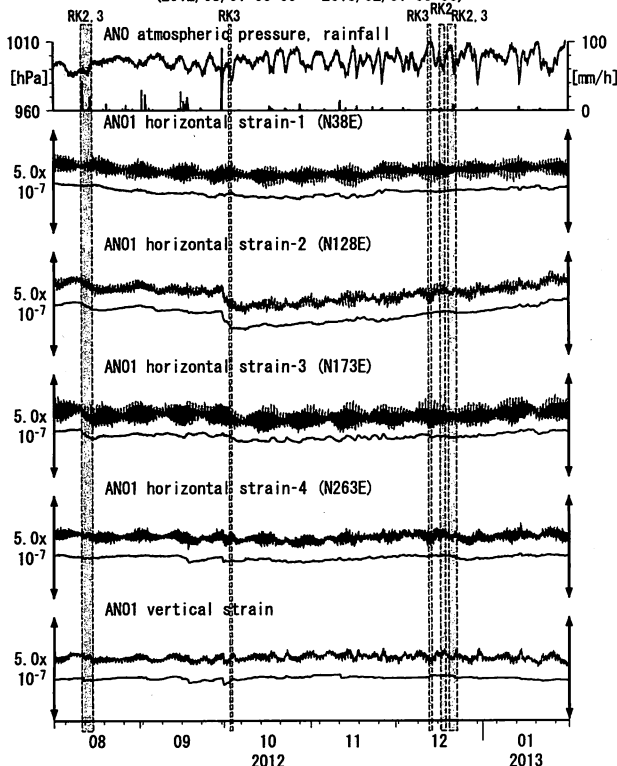
第7図 Crustal strains at ANO (時間値) (2012/08/01 00:00 - 2013/02/01 00:00)
