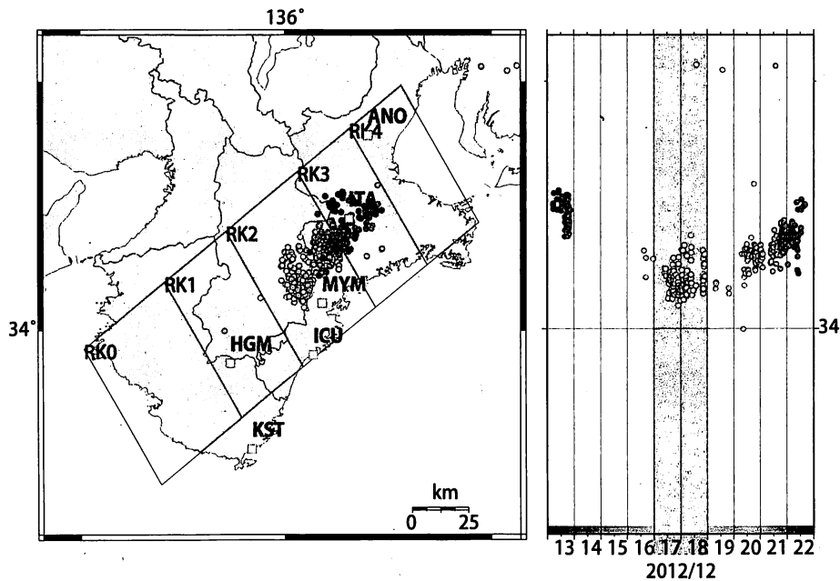
第51図: 2012/12/13 0:00 - 12/23 0:00 における紀伊半島の深部低周波微動の時空間分布図。 エンベロープ相関法により決定。
