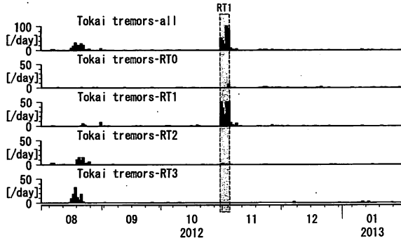
第36図 Deep low-frequency tremors in Tokai (日値) (2012/08/01 00:00 - 2013/02/01 00:00)
