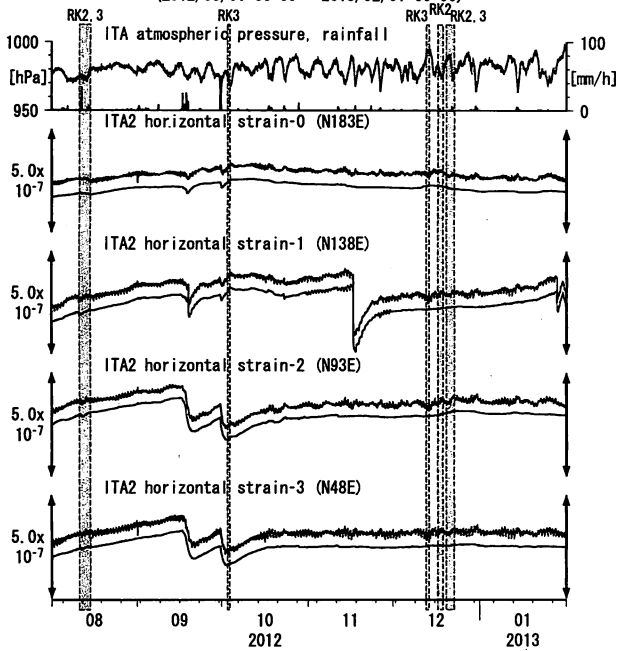
第9図 Crustal strains at ITA (時間値) (2012/08/01 00:00 - 2013/02/01 00:00)
