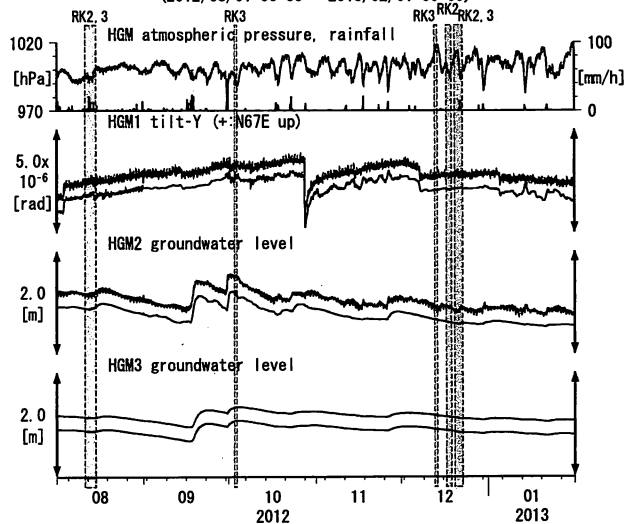
第16図 Tilt and groundwater level at HGM (時間値)
