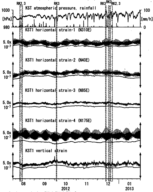
第17図 Crustal strains at KST (時間値) (2012/08/01 00:00 - 2013/02/01 00:00)
