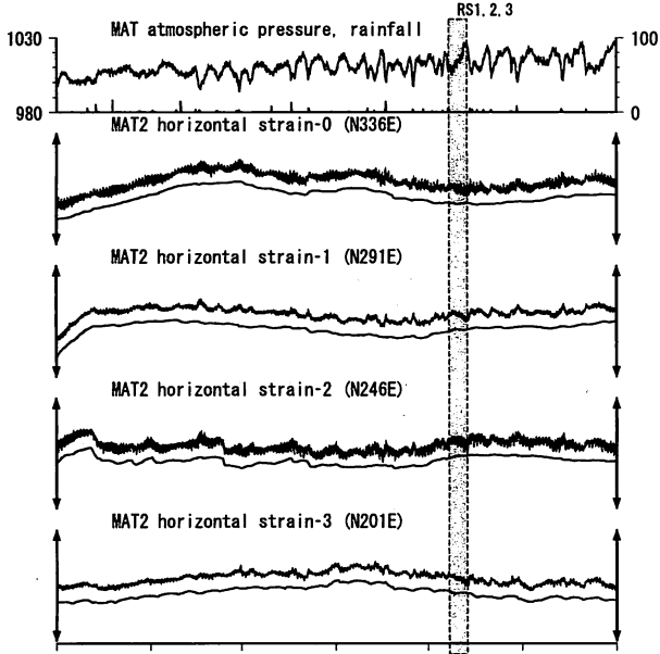
第33図 Crustal strains at MAT (時間値) (2012/08/01 00:00 - 2013/02/01 00:00)
