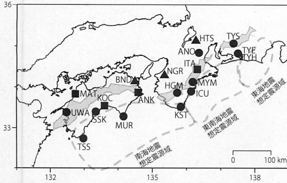
第1図: 地下水観測点の分布図 (●・■・▲)。●はデジタル方式の石井式歪計・傾斜計を用いている新規観測点、■はGladwin式歪計・ミットヨ式傾斜計を併設している新規観測点、▲はアナログ方式の石井式歪計を併設している既存の観測点。灰色の領域は短期的SSE及び深部低周波地震が定期的に発生していると考えられる地域。
