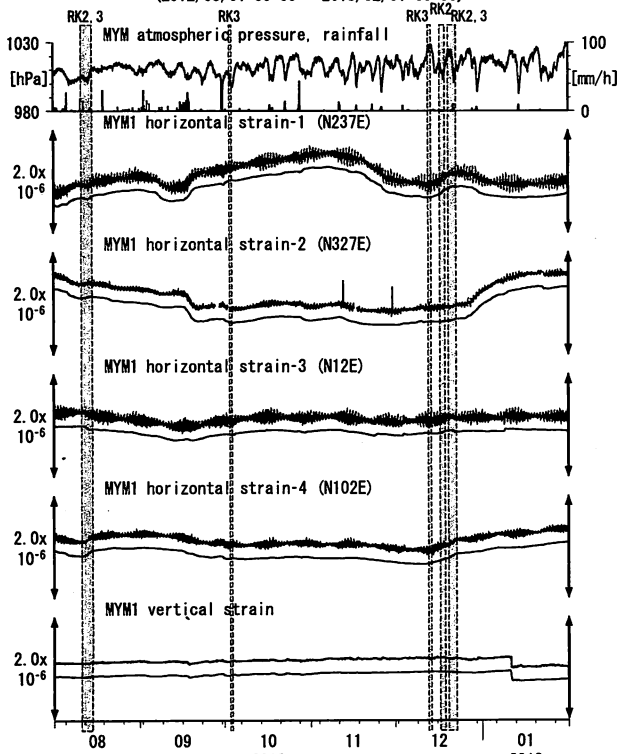
第11図 Crustal strains at MYM (時間値) (2012/08/01 00:00 - 2013/02/01 00:00)
