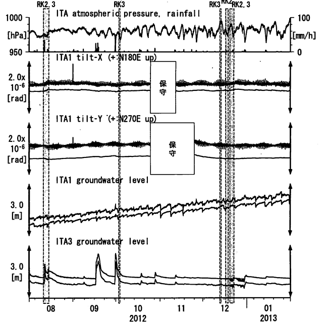
第10図 Tilt and groundwater level at ITA (時間値) (2012/08/01 00:00 - 2013/02/01 00:00)
