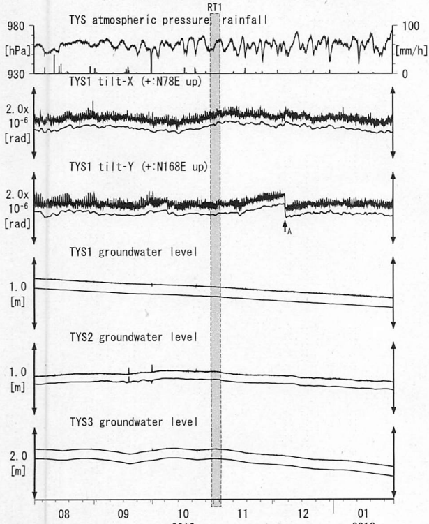
第3図 Tilt and groundwater level at TYS (時間値) (2012/08/01 00:00 - 2013/02/01 00:00)
