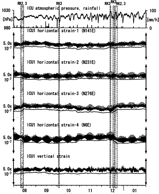
第13図 Crustal strains at ICU (時間値)
