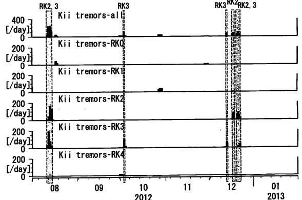
第38図 Deep low-frequency tremors in Kii Peninsula (日値) (2012/08/01 00:00 - 2013/02/01 00:00)
