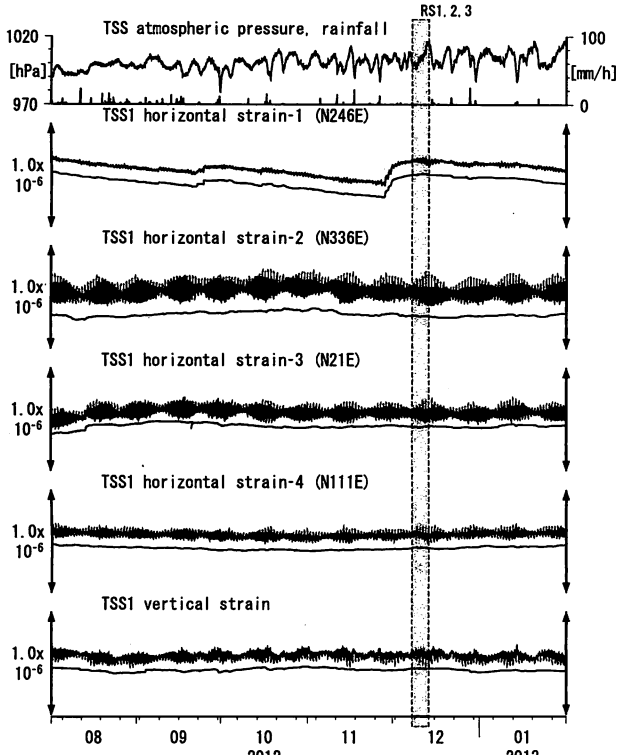
第29図 Crustal strains at TSS (時間値) (2012/08/01 00:00 - 2013/02/01 00:00)
