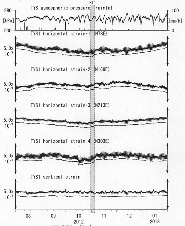
第2図 Crustal strains at TYS (時間値) (2012/08/01 00:00 - 2013/02/01 00:00)
