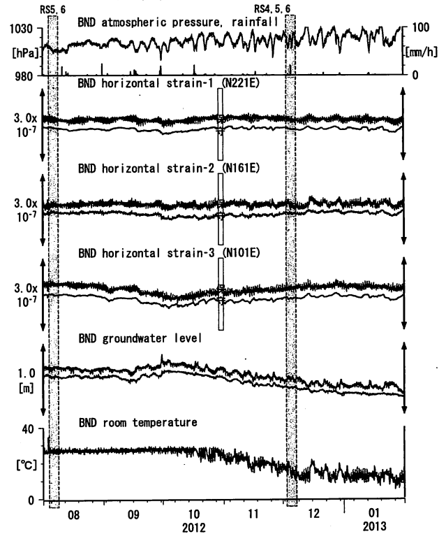
第20図 Crustal strains and groundwater level at BND (時間値) (2012/08/01 00:00 - 2013/02/01 00:00)
