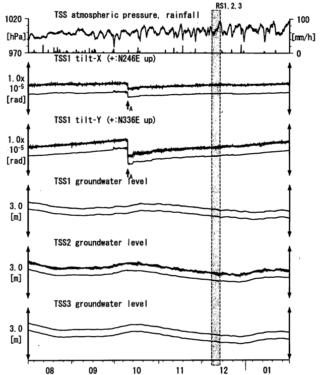
第30図 Tilt and groundwater level at TSS (時間値) (2012/08/01 00:00 - 2013/02/01 00:00)
