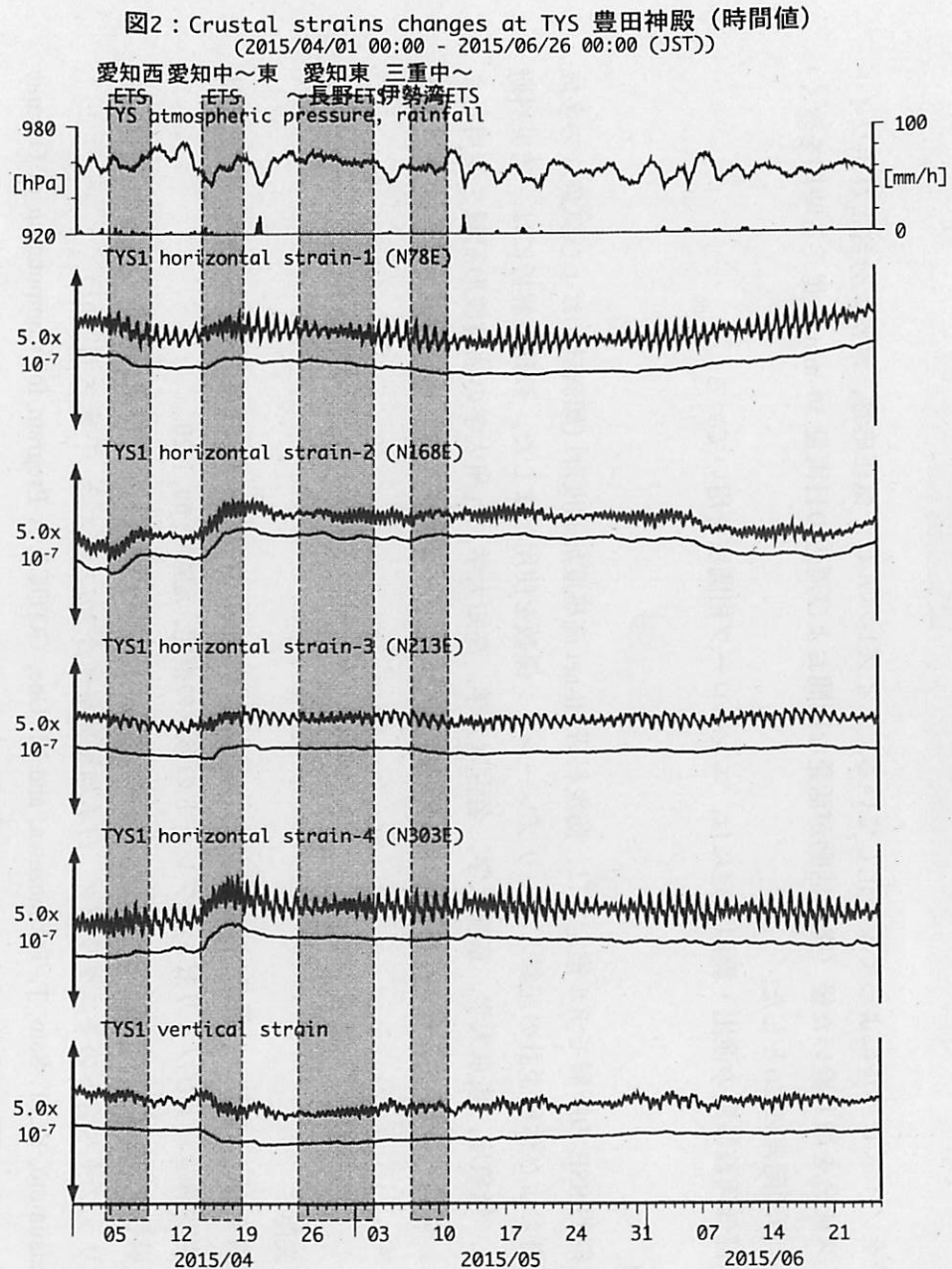
Strainmeter depth = 586.7-588.1 [GL-m] 上: 1次トレンドを除去 下: BAYTAP-Gにより潮汐・気圧応答・ノイズ成分を除去後、1次トレンドも除去
