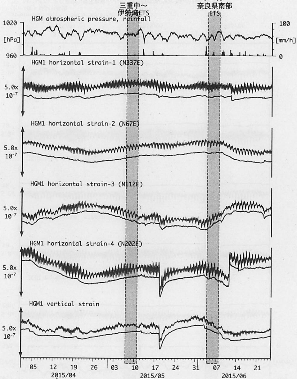
図17: Crustal strains changes at HGM 田辺本宮 (時間値) (2015/04/01 00:00 - 2015/06/26 00:00 (JST))
