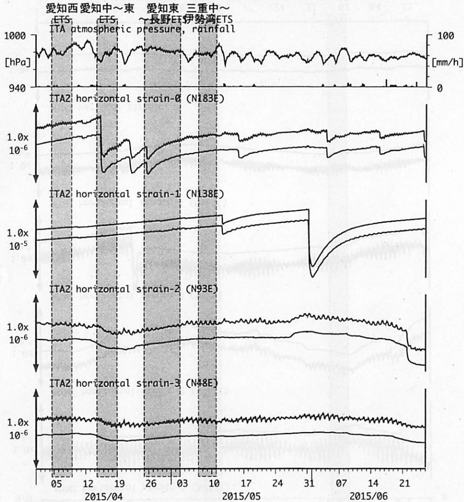
図11: Crustal strain changes at ITA 松阪飯高 (時間値) (2015/04/01 00:00 - 2015/06/26 00:00 (JST))
