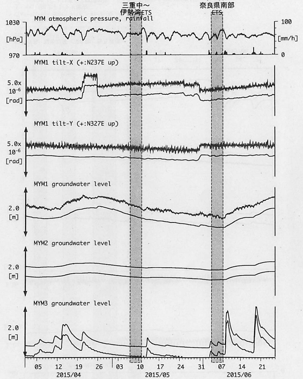
図14 : Tilt and groundwater level changes at MYM 紀北海山 (時間値) (2015/04/01 00:00 - 2015/06/26 00:00 (JST))
