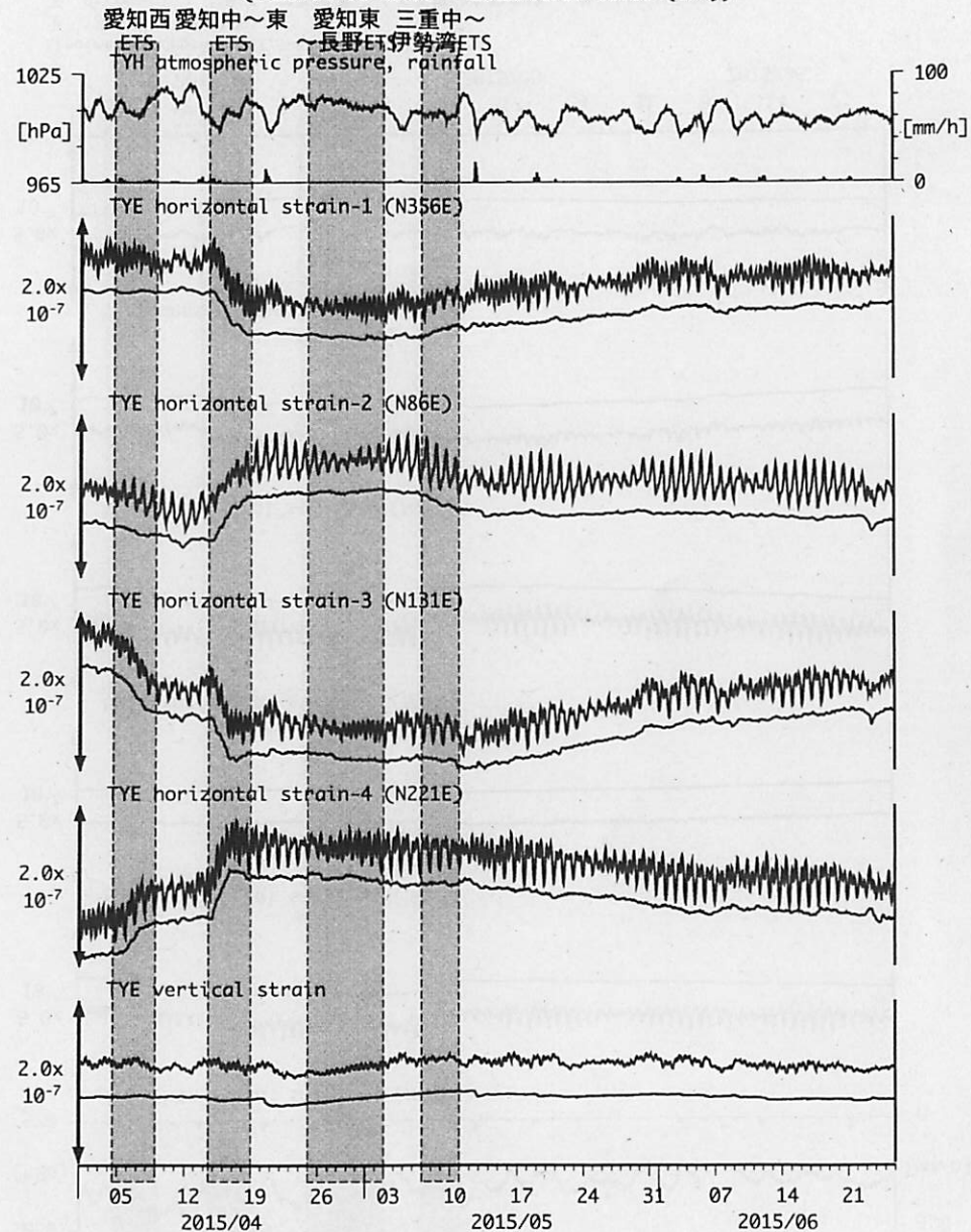
図6: Crustal strain changes at TYE 豊橋多米 (時間値) (2015/04/01 00:00 - 2015/06/26 00:00 (JST))
