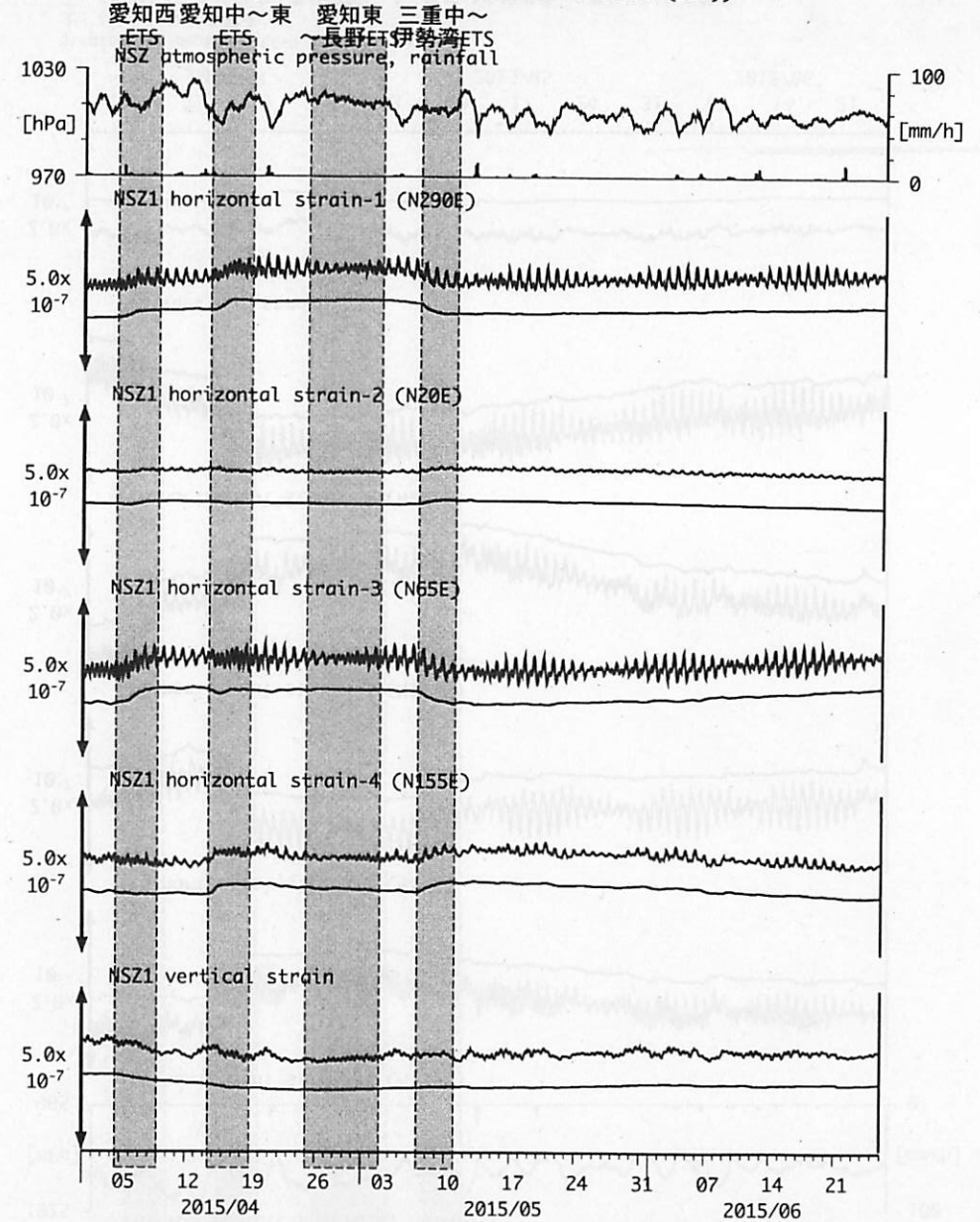
図4: Crustal strains changes at NSZ 西尾善明 (時間値) (2015/04/01 00:00 - 2015/06/26 00:00 (JST))
