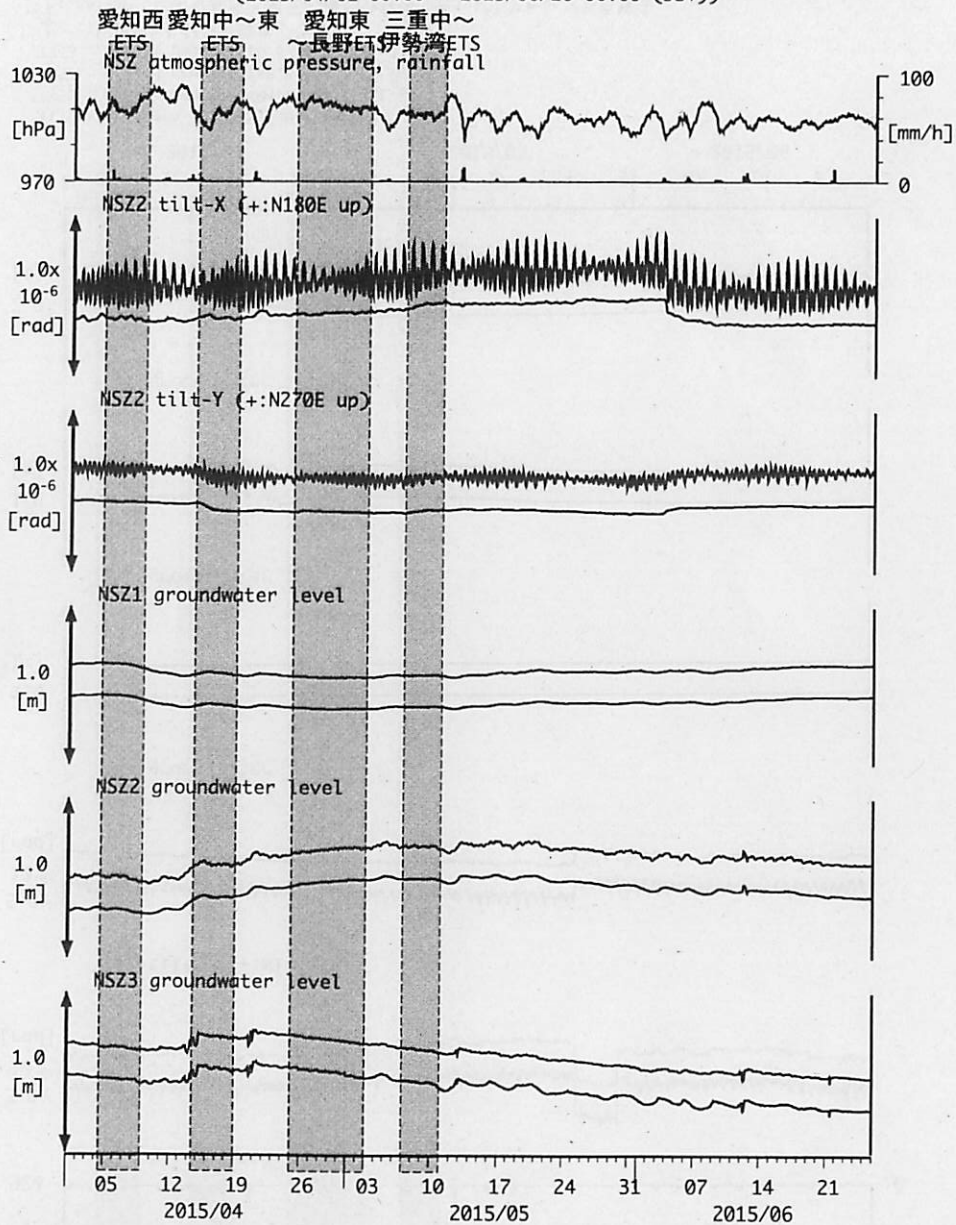
図5: Tilt and groundwater level changes at NSZ 西尾善明 (時間値) (2015/04/01 00:00 - 2015/06/26 00:00 (JST))
