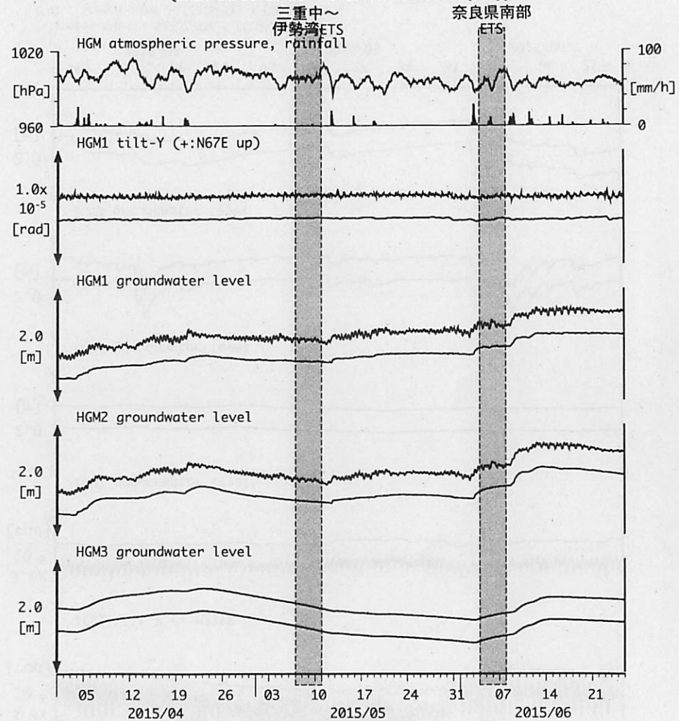
図18: Tilt and groundwater level changes at HGM 田辺本宮 (時間値) (2015/04/01 00:00 - 2015/06/26 00:00 (JST))
