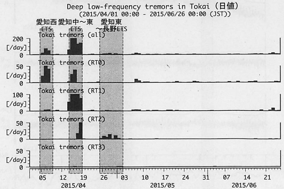
図22 (上段) 愛知県およびその周辺における深部低周波微動の時空間分布、(下段) 各領域における発生頻度(日値)。
