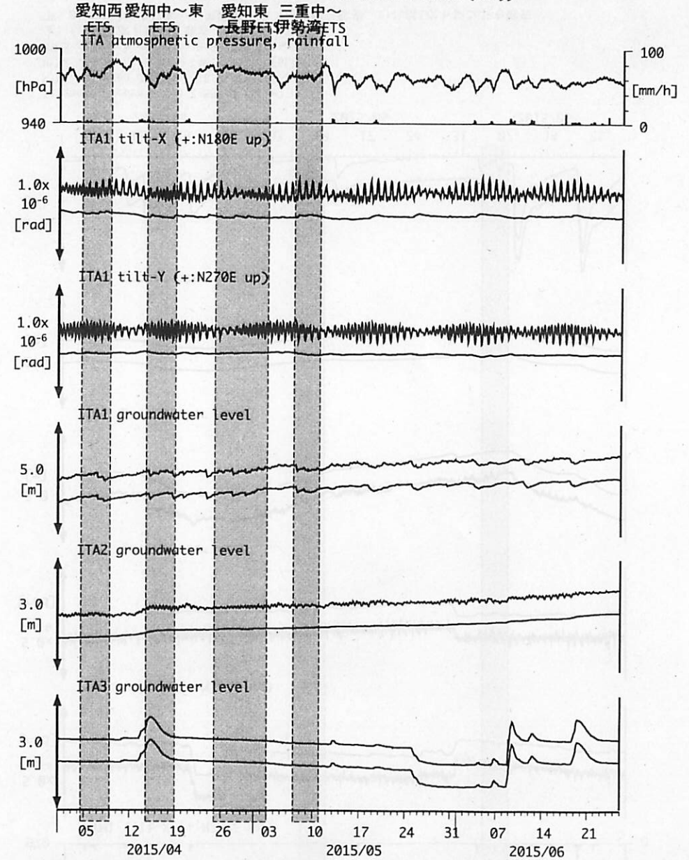
図12: Tilt and groundwater level changes at ITA 松阪飯高 (時間値) (2015/04/01 00:00 - 2015/06/26 00:00 (JST))
