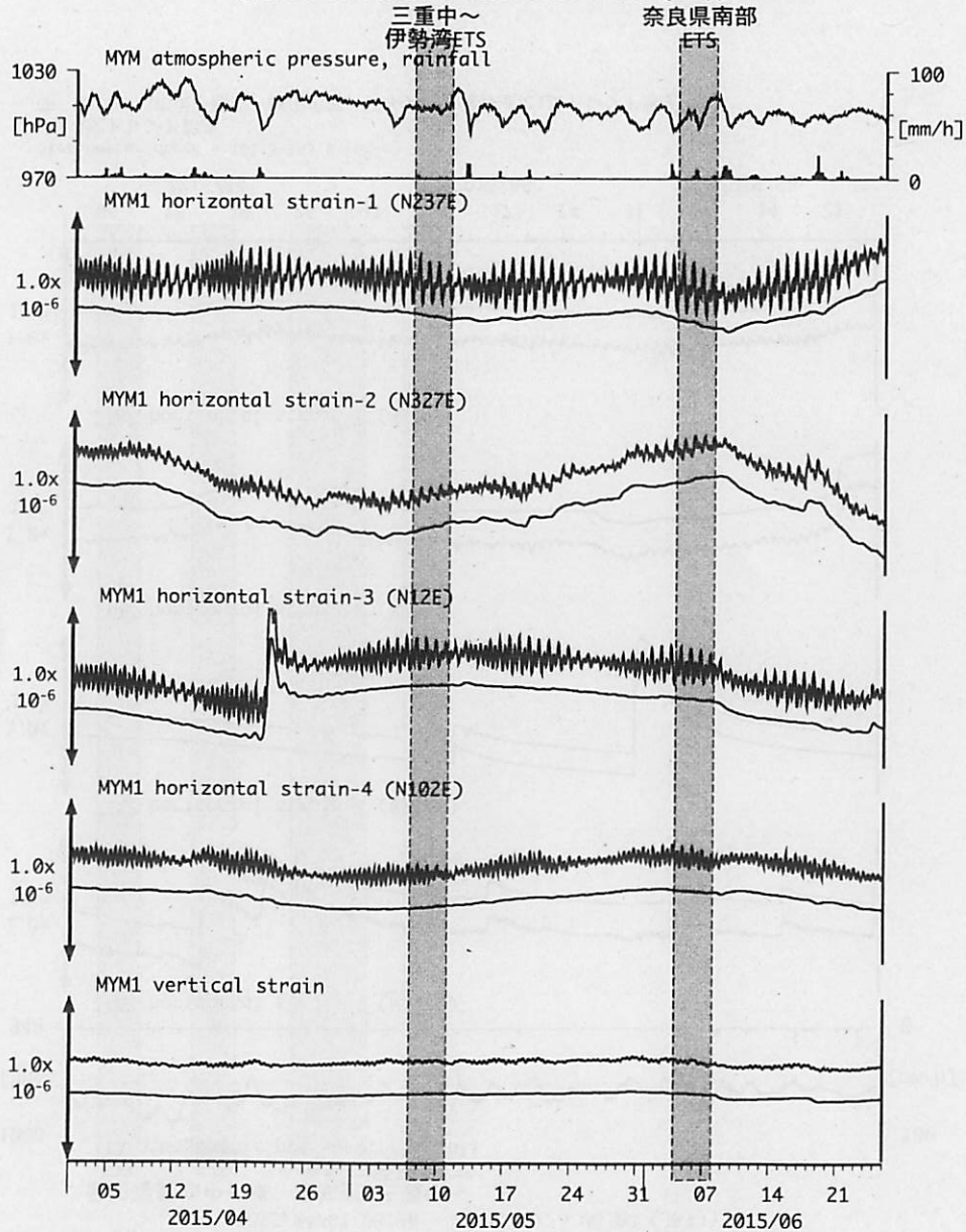
図13 : Crustal strain changes at MYM 紀北海山 (時間値) (2015/04/01 00:00 - 2015/06/26 00:00 (JST))
