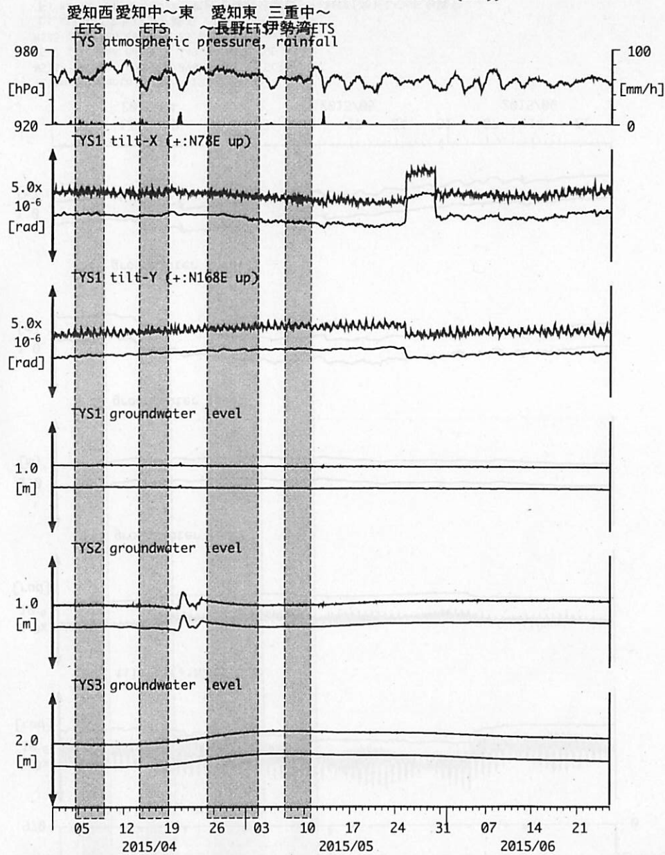
図3: Tilt and groundwater level changes at TYS 豊田神殿 (時間値) (2015/04/01 00:00 - 2015/06/26 00:00 (JST))
