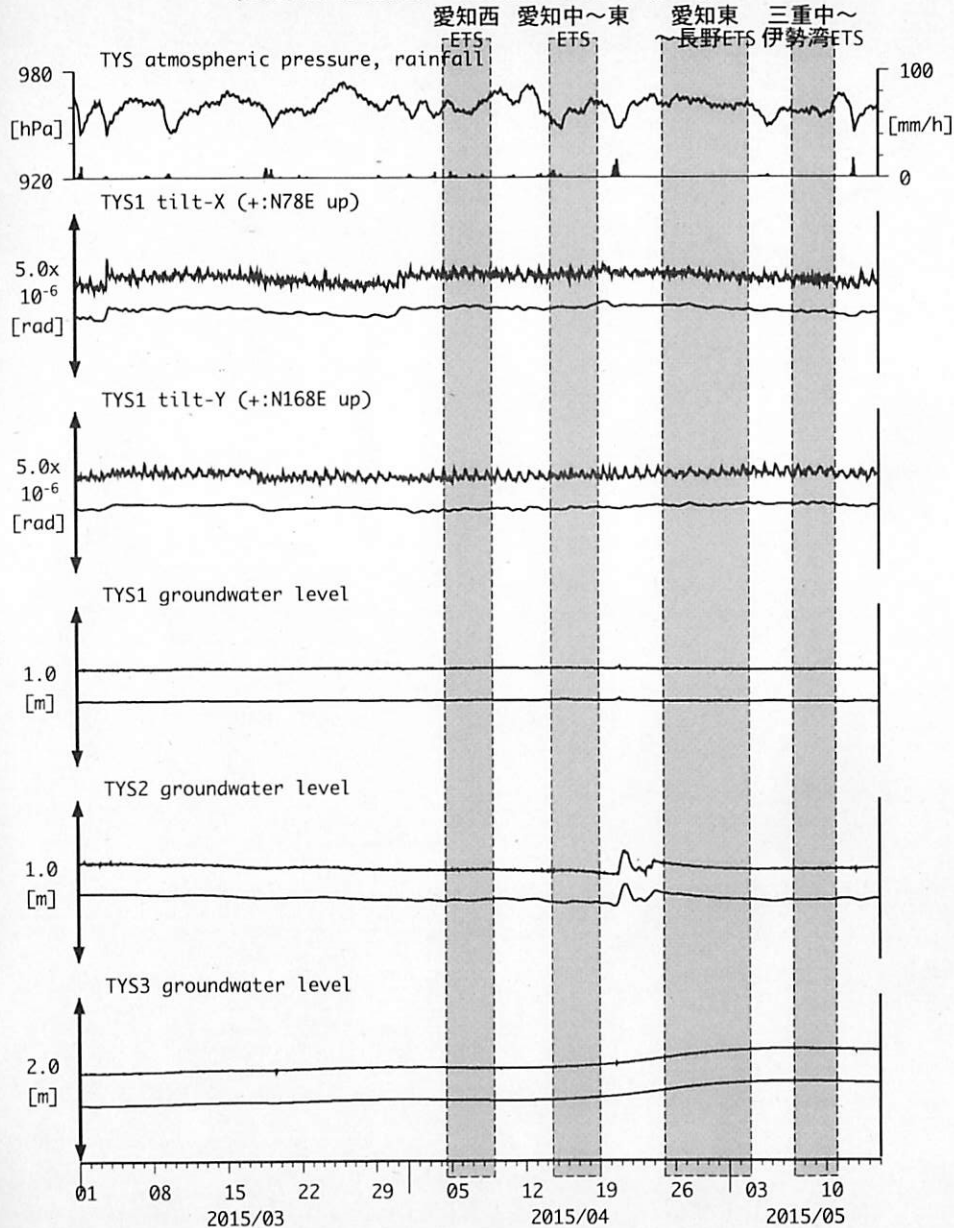
図3: Tilt and groundwater level changes at TYS 豊田神殿 (時間値) (2015/03/01 00:00 - 2015/05/15 00:00 (JST))
