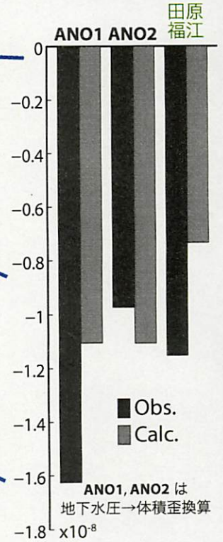
図 26 : 2015/05/07-10 の多成分歪計・傾斜計の変化 (図 25 網掛) を説明する断層モデル。
