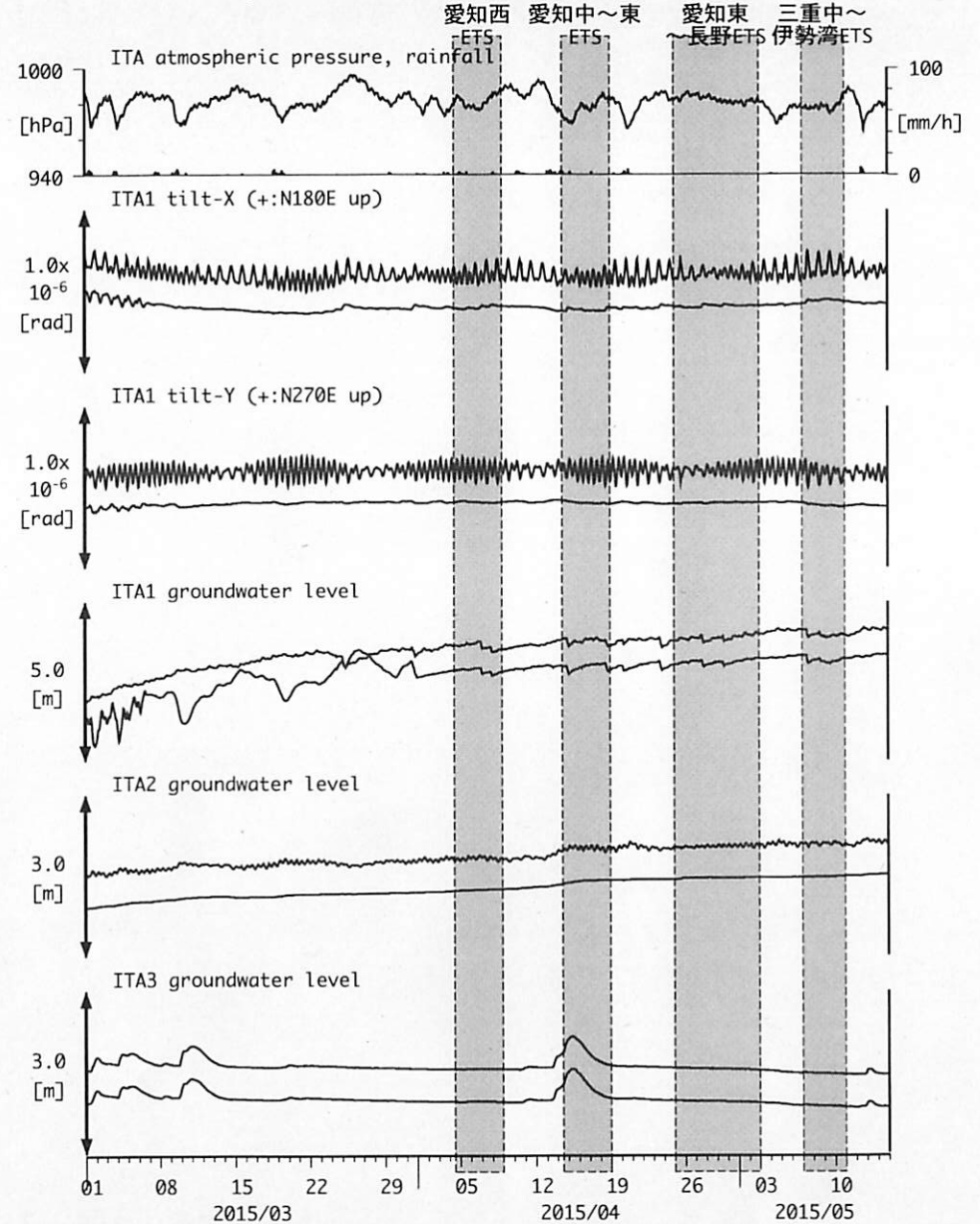
図12: Tilt and groundwater level changes at ITA 松阪飯高 (時間値) (2015/03/01 00:00 - 2015/05/15 00:00 (JST))
