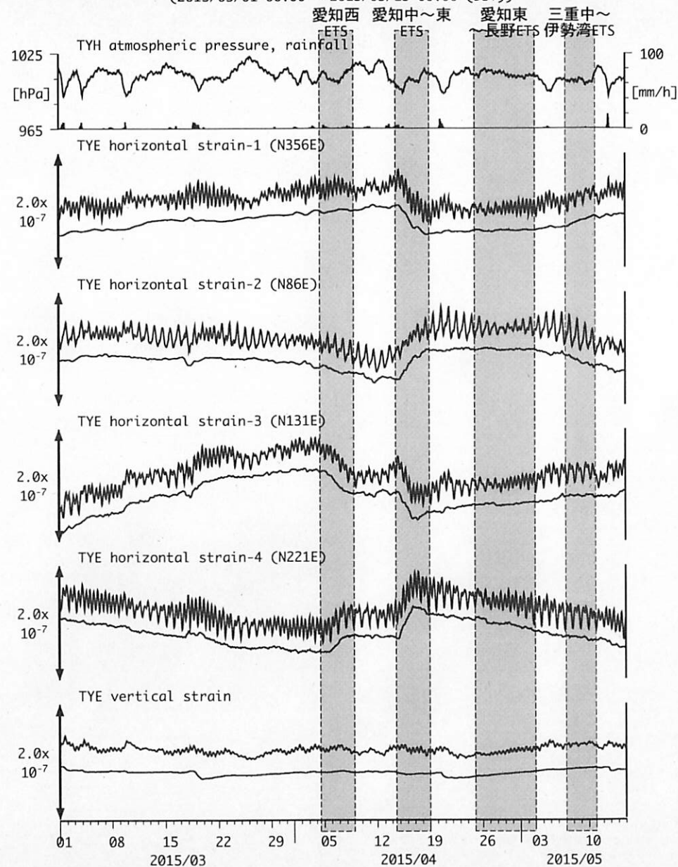
図6: Crustal strain changes at TYE 豊橋多米 (時間値) (2015/03/01 00:00 - 2015/05/15 00:00 (JST))
