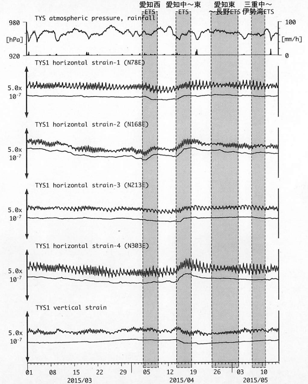
図2: Crustal strains changes at TYS 豊田神殿 (時間値) (2015/03/01 00:00 - 2015/05/15 00:00 (JST))
