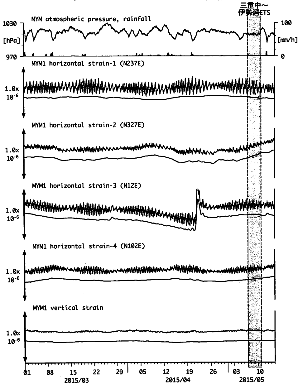
図13: Crustal strain changes at MYM 紀北海山 (時間値) (2015/03/01 00:00 - 2015/05/15 00:00 (JST))
