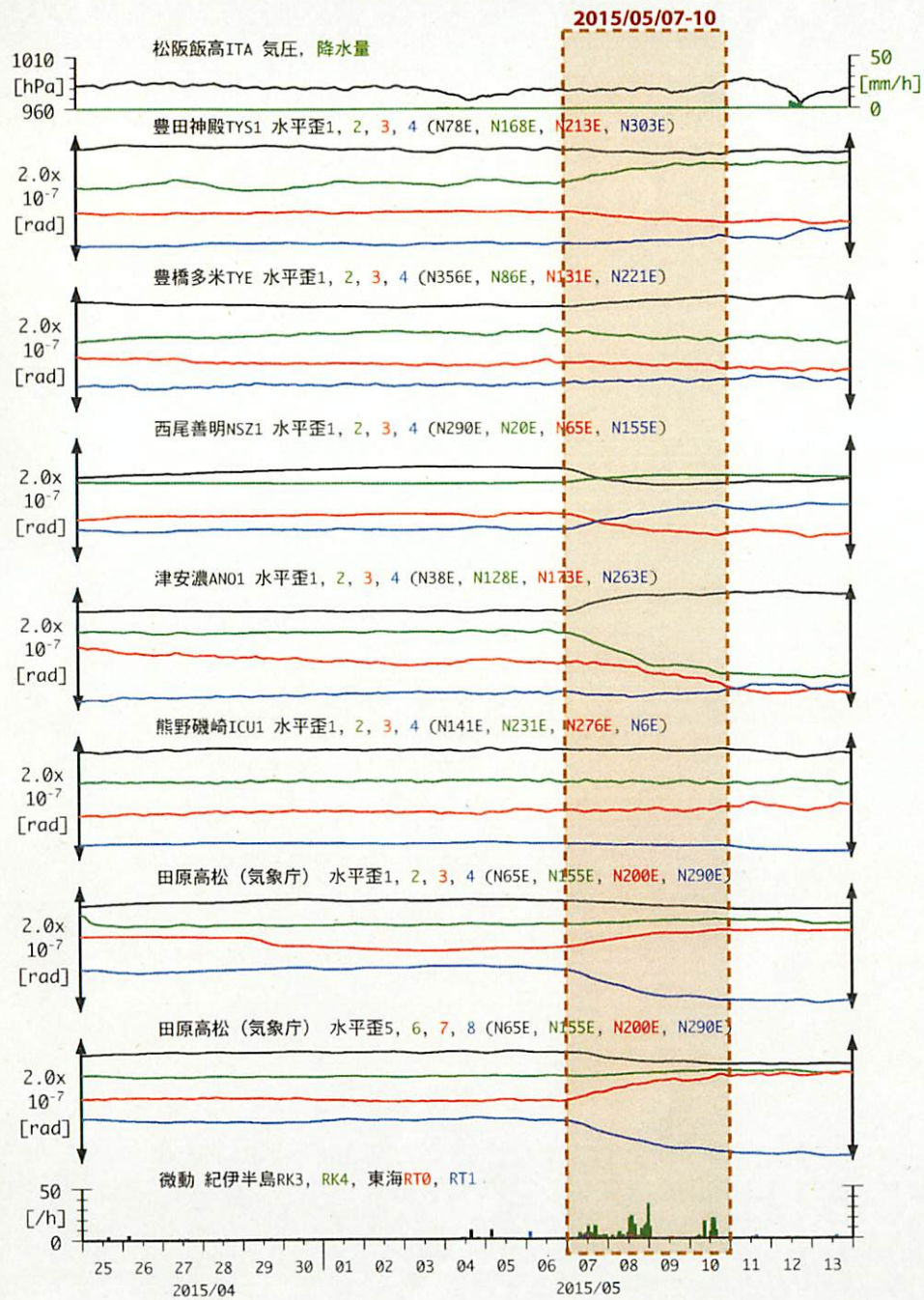
図 25：紀伊半島・東海地方における歪・傾斜観測結果 (2015/04/25 00:00 - 2015/05/14 00:00 (JST))
