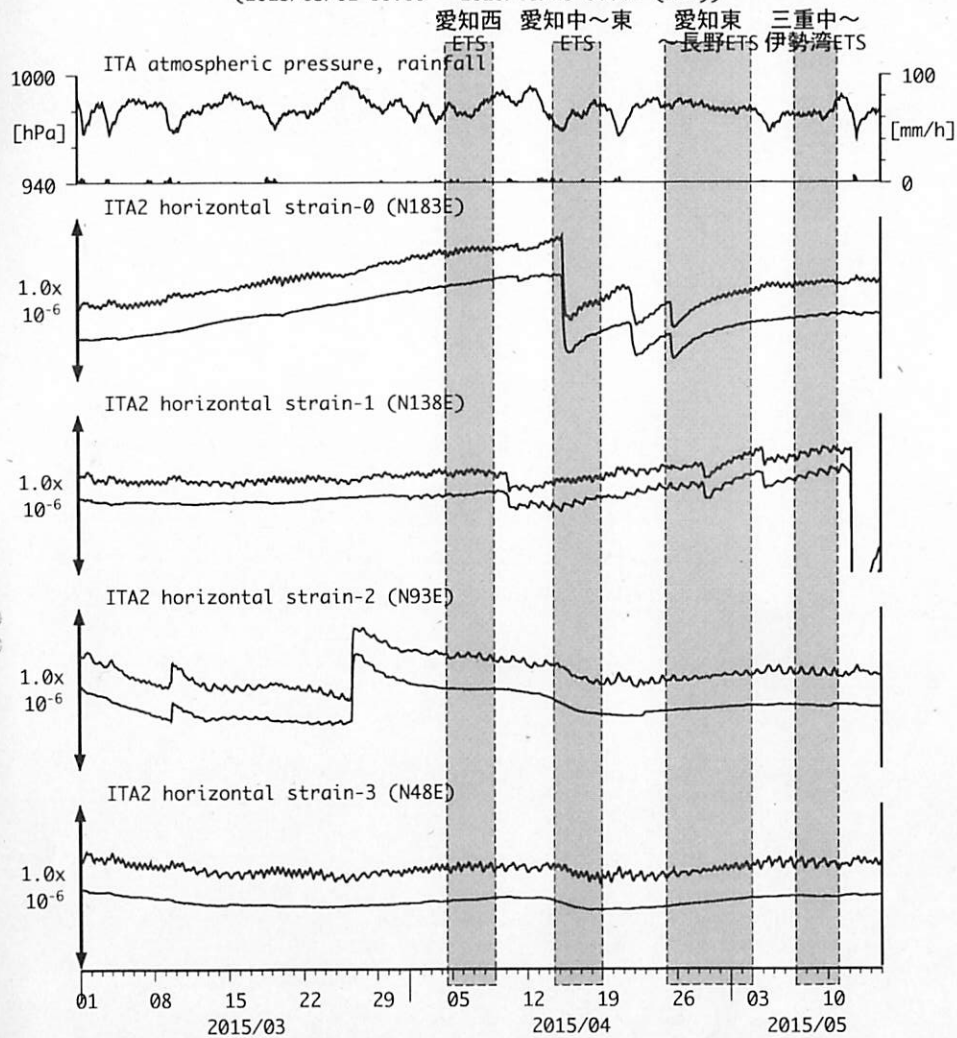
図11: Crustal strain changes at ITA 松阪飯高 (時間値) (2015/03/01 00:00 - 2015/05/15 00:00 (JST))
