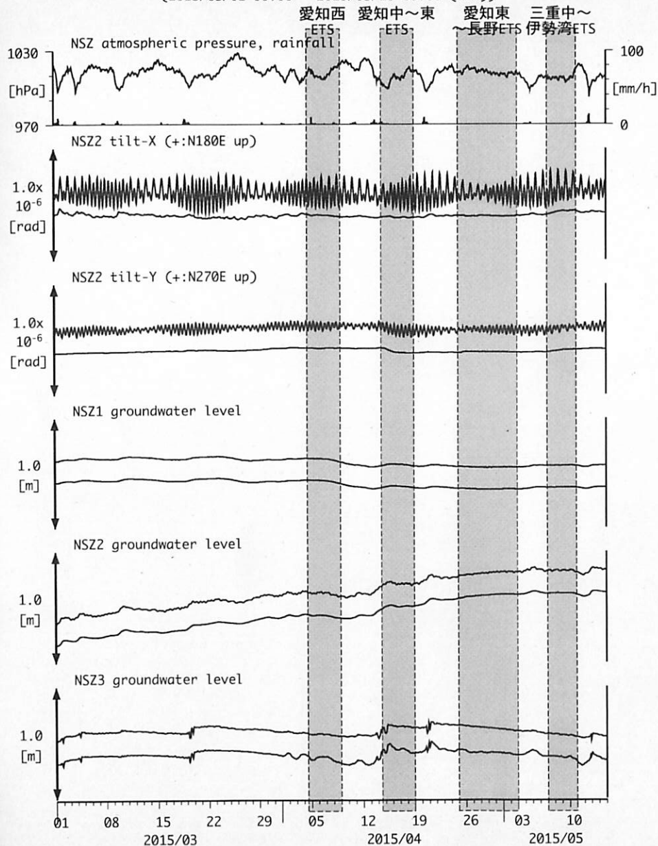
図5: Tilt and groundwater level changes at NSZ 西尾善明 (時間値) (2015/03/01 00:00 - 2015/05/15 00:00 (JST))
