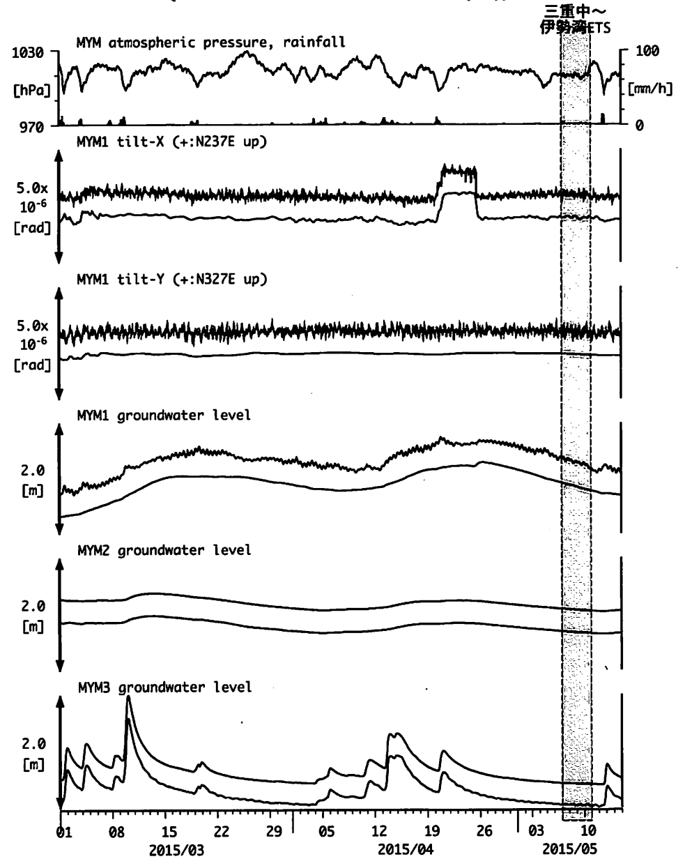
図14: Tilt and groundwater level changes at MYM 紀北海山 (時間値) (2015/03/01 00:00 - 2015/05/15 00:00 (JST))
