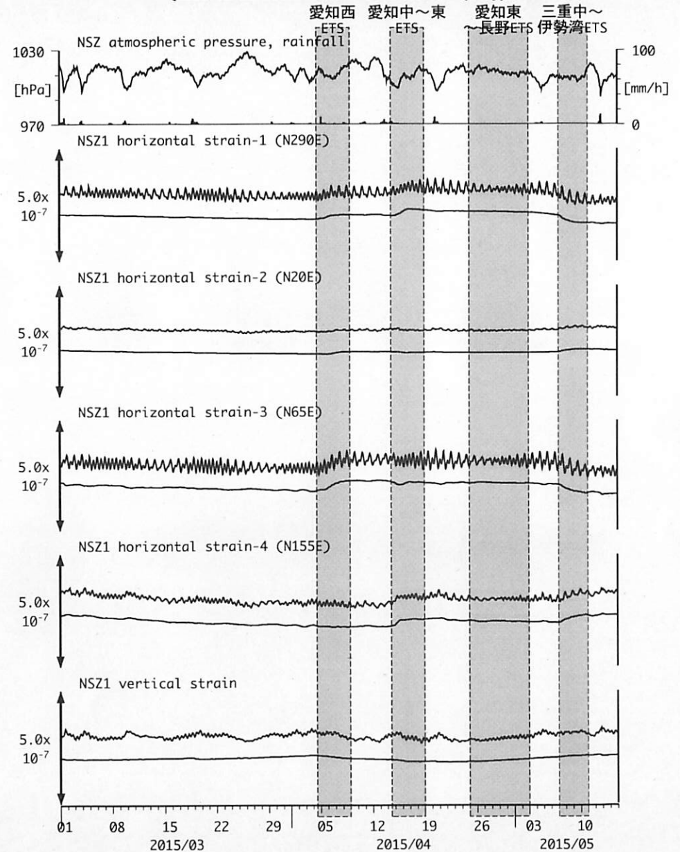
図4: Crustal strains changes at NSZ 西尾善明 (時間値) (2015/03/01 00:00 - 2015/05/15 00:00 (JST))
