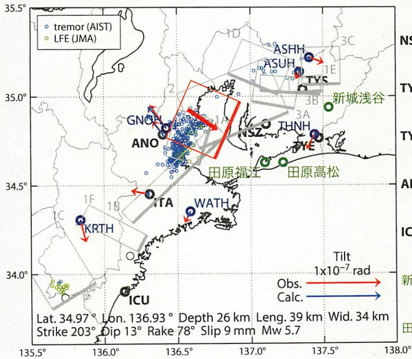
(b1) 推定された断層モデル, 傾斜の比較
