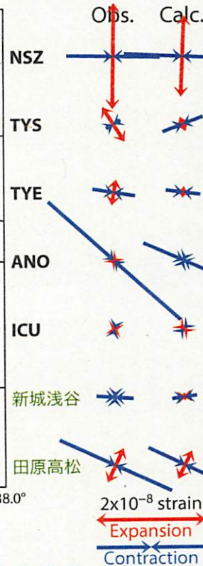
図 26 : 2015/05/07-10 の多成分歪計・傾斜計の変化 (図 25 網掛) を説明する断層モデル。
