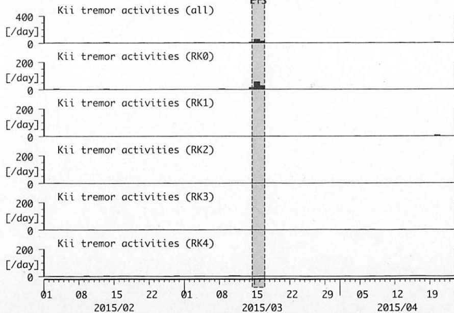
図 23 (上段) 紀伊半島における深部低周波微動の時空間分布、(下段) 各領域における発生頻度 (日値)。
