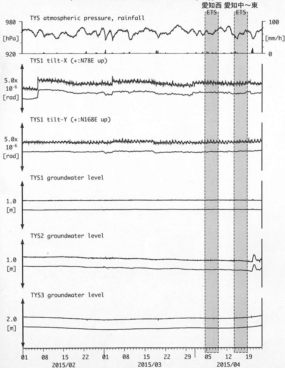
図3: Tilt and groundwater level changes at TYS 豊田神殿 (時間値) (2015/02/01 00:00 - 2015/04/24 00:00 (JST))
