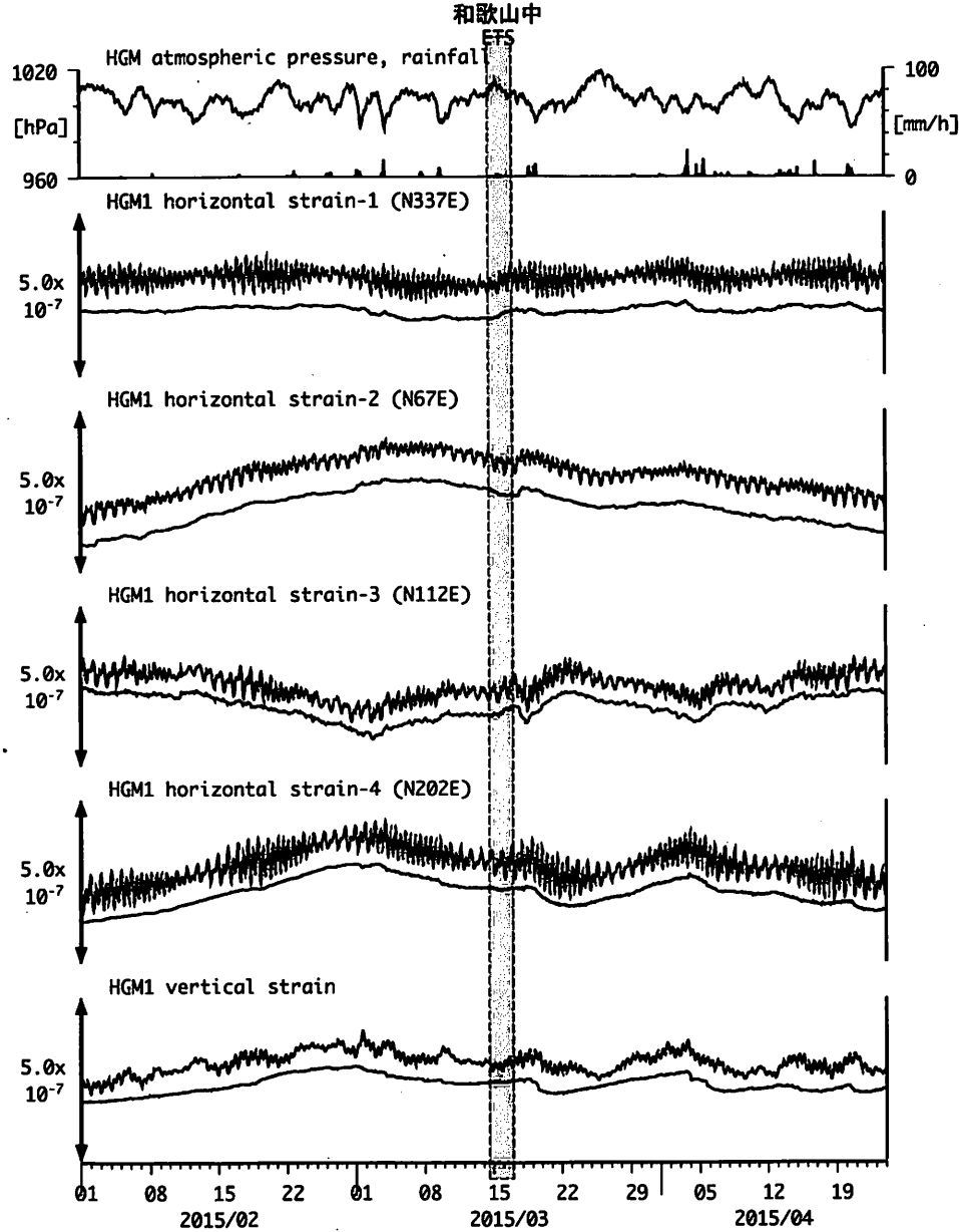
図17: Crustal strains changes at HGM 田辺本宮 (時間値) (2015/02/01 00:00 - 2015/04/24 00:00 (JST))
