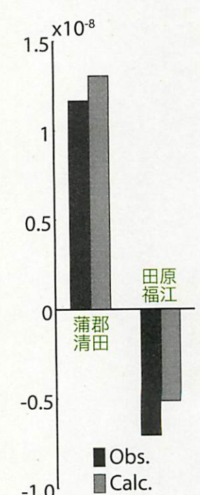
図 26 : 2015/4/4PM-4/8 の多成分歪計・傾斜計の変化 (図 25 網掛 [A]) を説明する断層モデル。
