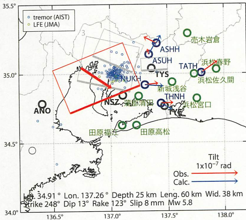
図 26 : 2015/4/4PM-4/8 の多成分歪計・傾斜計の変化 (図 25 網掛 [A]) を説明する断層モデル。
