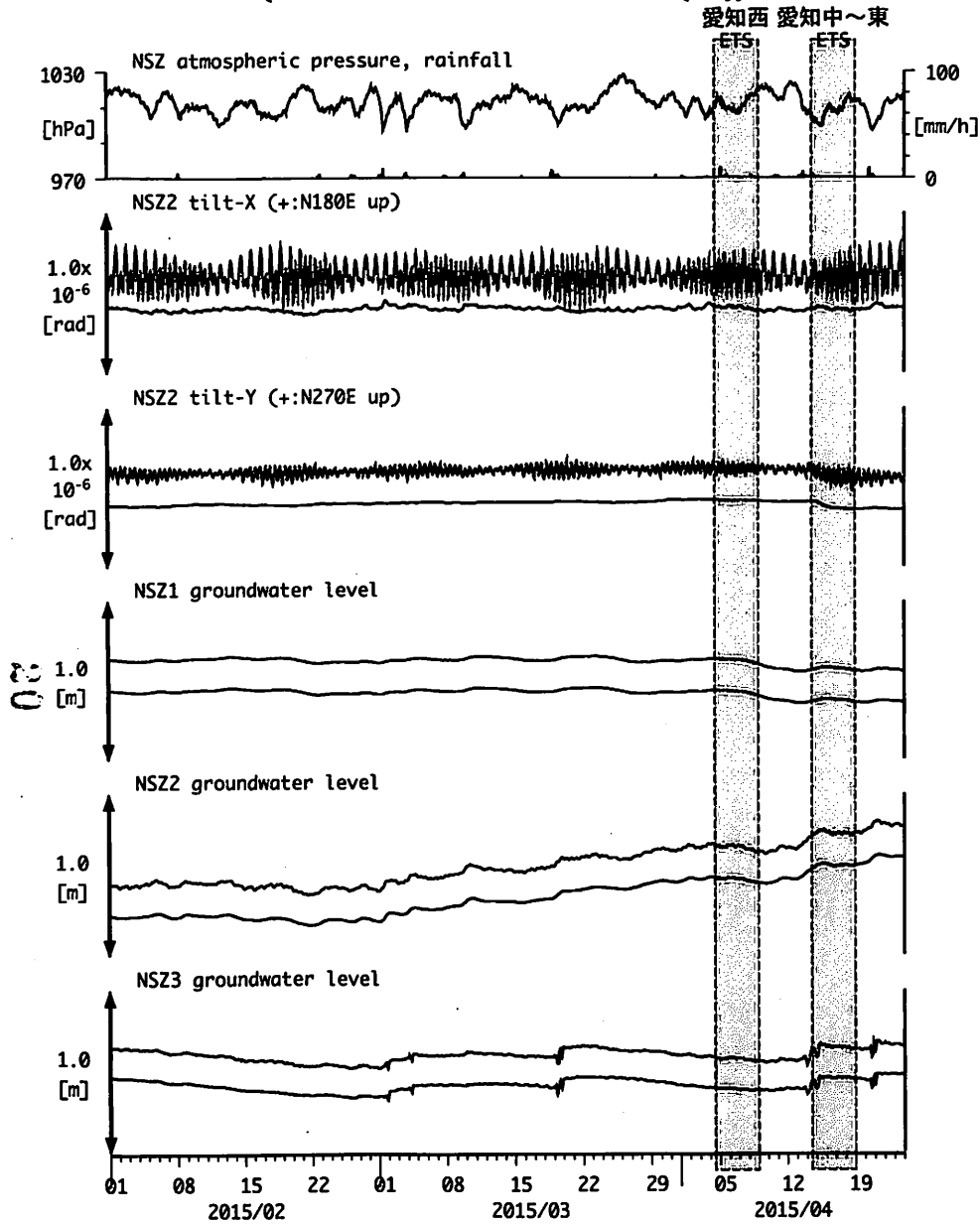
図5: Tilt and groundwater level changes at NSZ 西尾善明 (時間値) (2015/02/01 00:00 - 2015/04/24 00:00 (JST))
