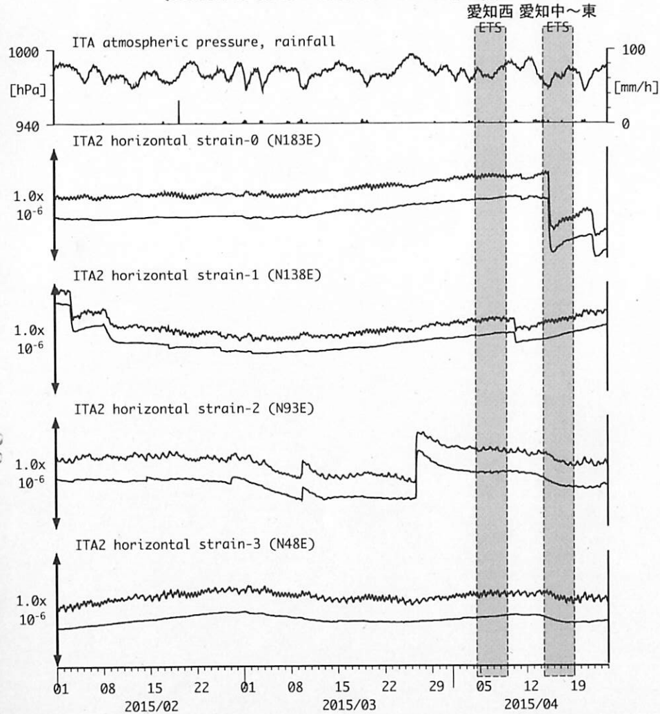
図11: Crustal strain changes at ITA 松阪飯高 (時間値) (2015/02/01 00:00 - 2015/04/24 00:00 (JST))
