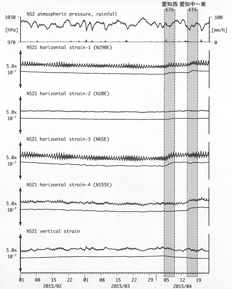
図4: Crustal strains changes at NSZ 西尾善明 (時間値) (2015/02/01 00:00 - 2015/04/24 00:00 (JST))
