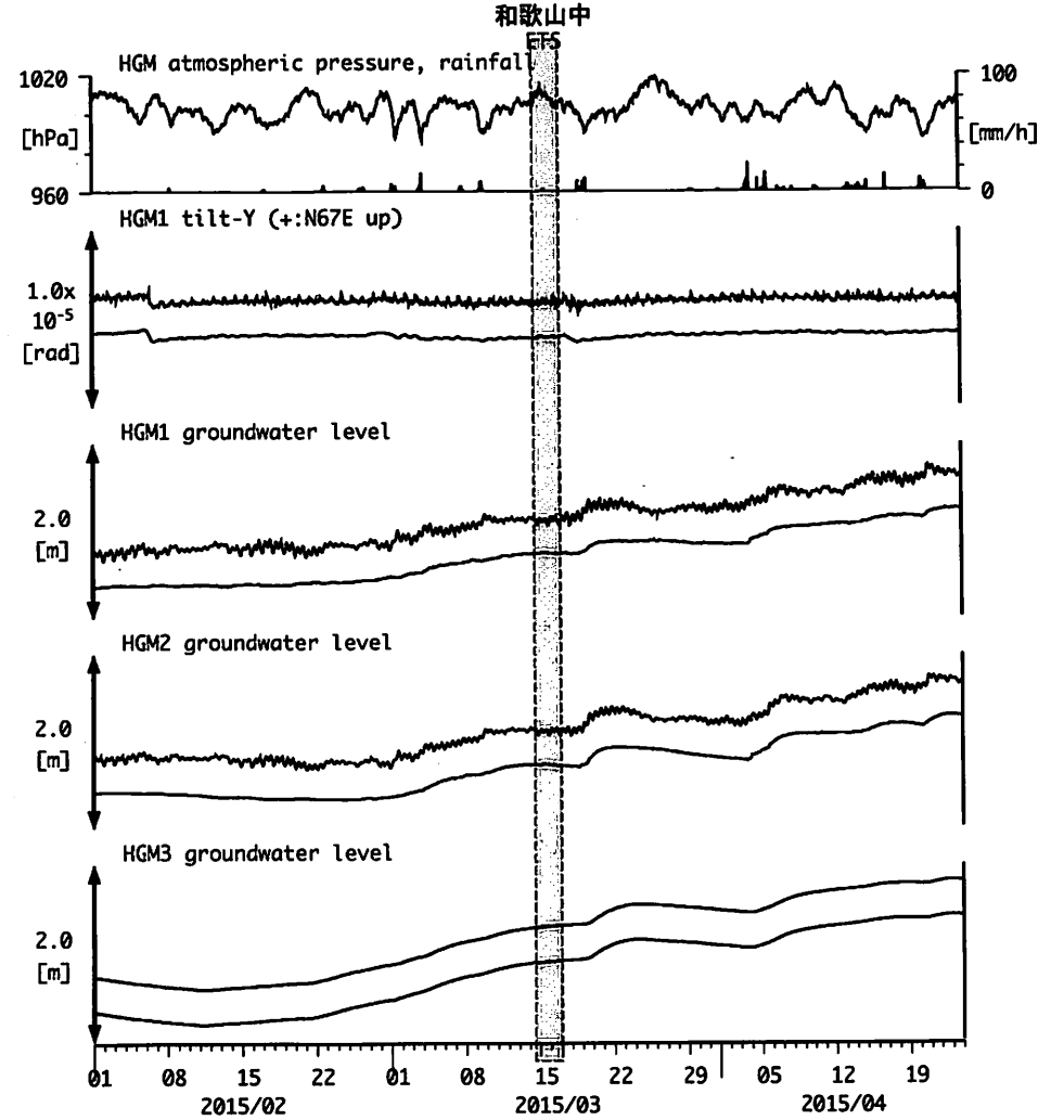
図18: Tilt and groundwater level changes at HGM 田辺本宮 (時間値) (2015/02/01 00:00 - 2015/04/24 00:00 (JST))
