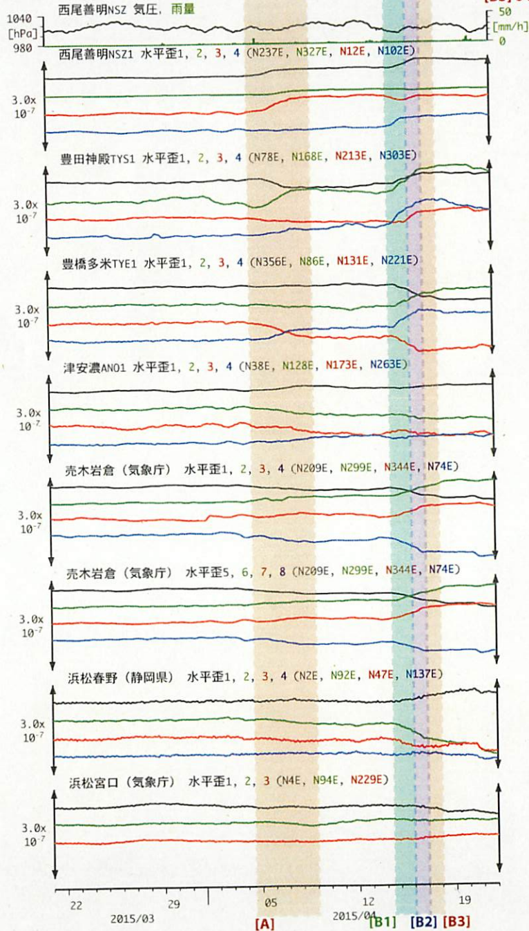
図25：東海地方における歪・地下水・傾斜観測結果 (2015/03/21 00:00 - 2015/04/22 00:00 (JST))
