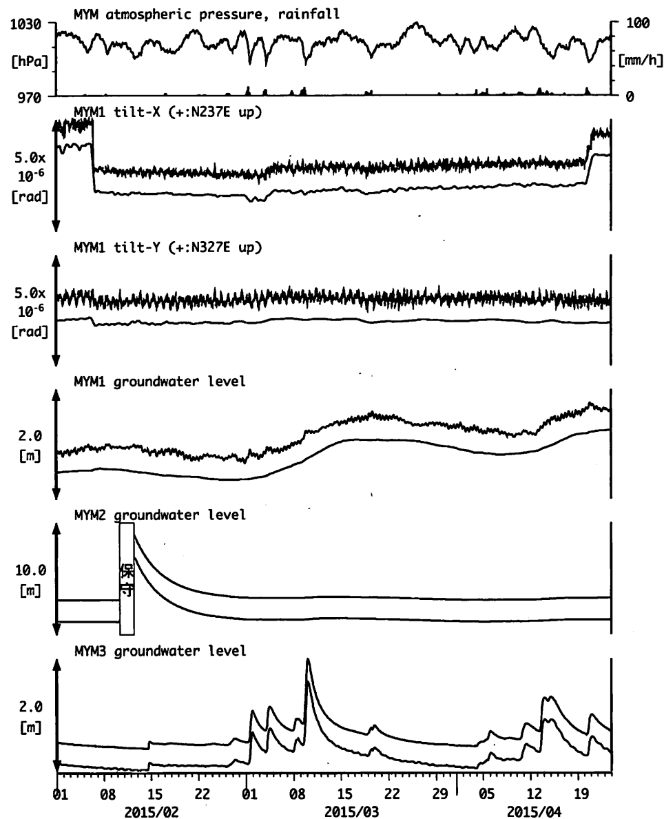
図14 : Tilt and groundwater level changes at MYM 紀北海山 (時間値) (2015/02/01 00:00 - 2015/04/24 00:00 (JST))
