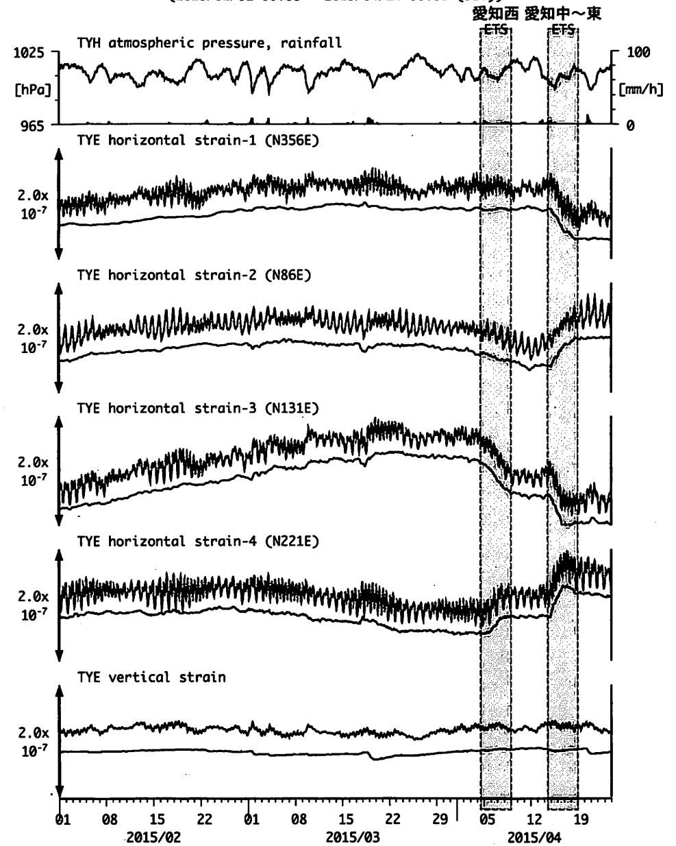
図6: Crustal strain changes at TYE 豊橋多米 (時間値) (2015/02/01 00:00 - 2015/04/24 00:00 (JST))
