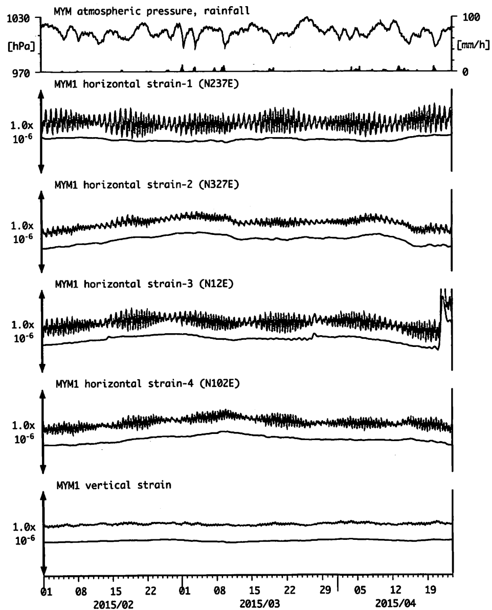
図13 : Crustal strain changes at MYM 紀北海山 (時間値) (2015/02/01 00:00 - 2015/04/24 00:00 (JST))
