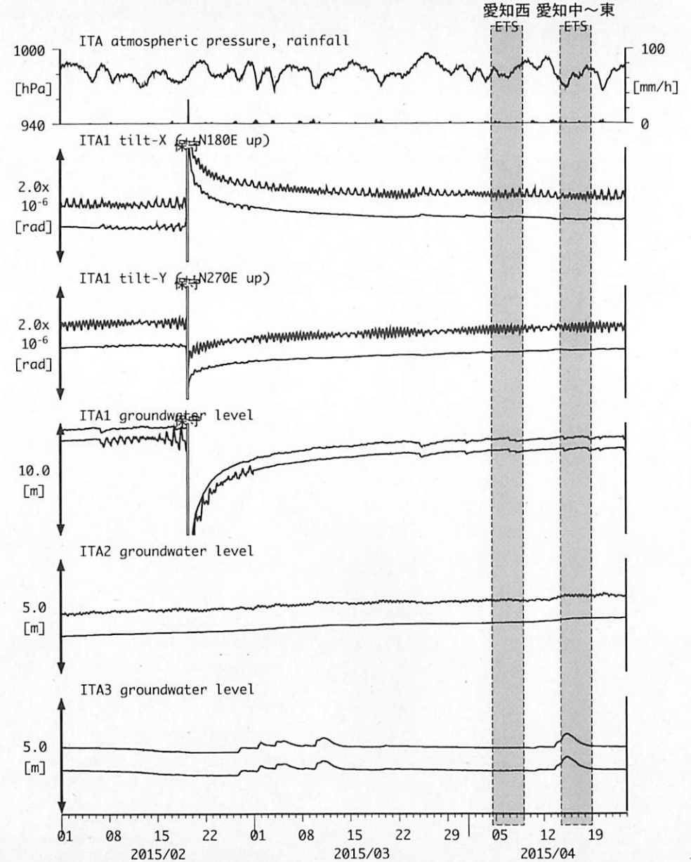
図12: Tilt and groundwater level changes at ITA 松阪飯高 (時間値) (2015/02/01 00:00 - 2015/04/24 00:00 (JST))
