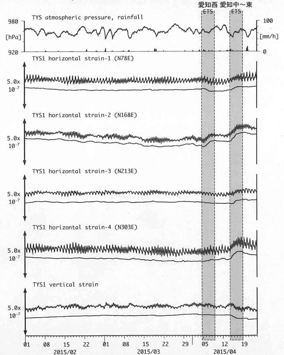
図2: Crustal strains changes at TYS 豊田神殿 (時間値) (2015/02/01 00:00 - 2015/04/24 00:00 (JST))
