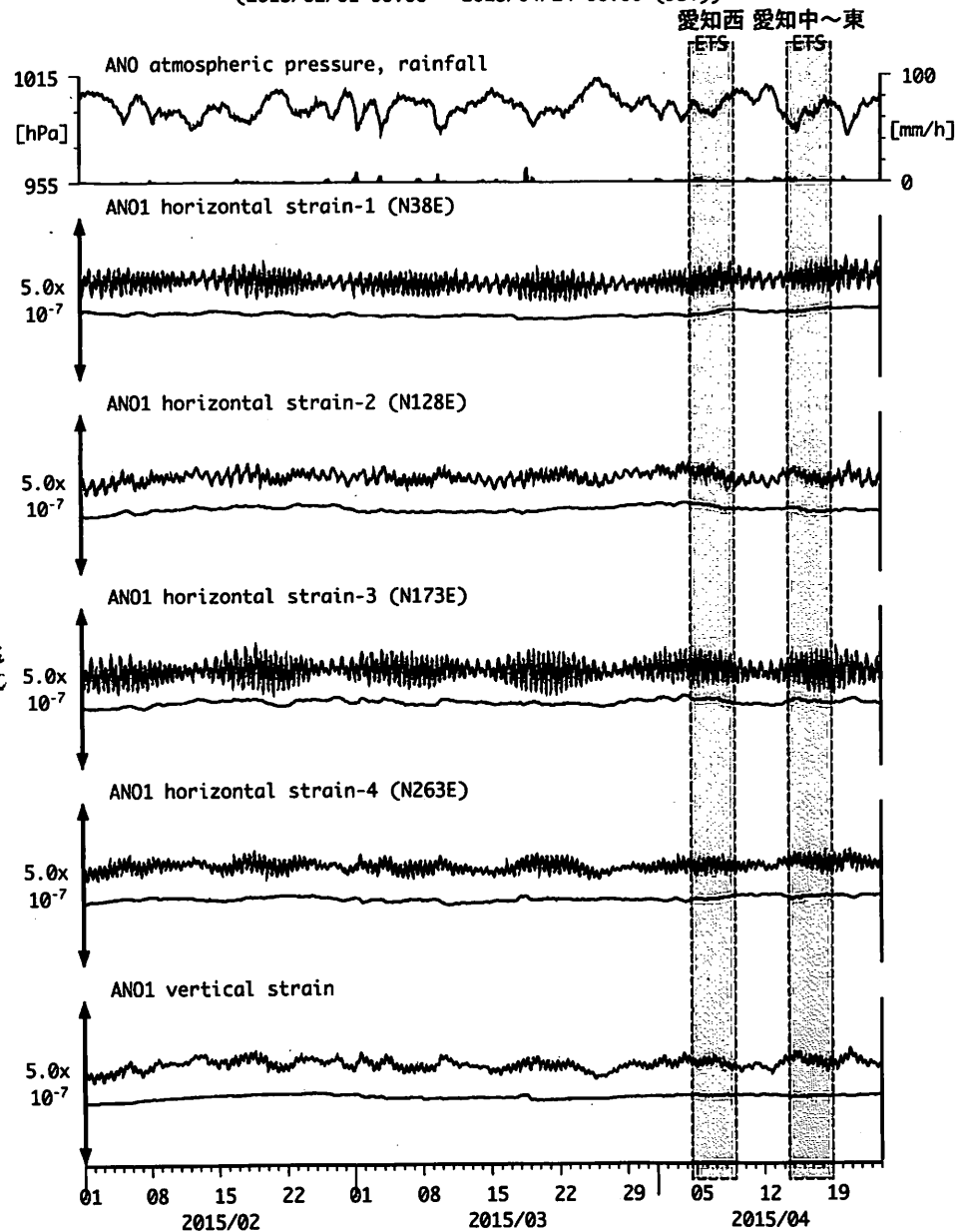
図9 : Crustal strains changes at ANO 津安濃 (時間値) (2015/02/01 00:00 - 2015/04/24 00:00 (JST))
