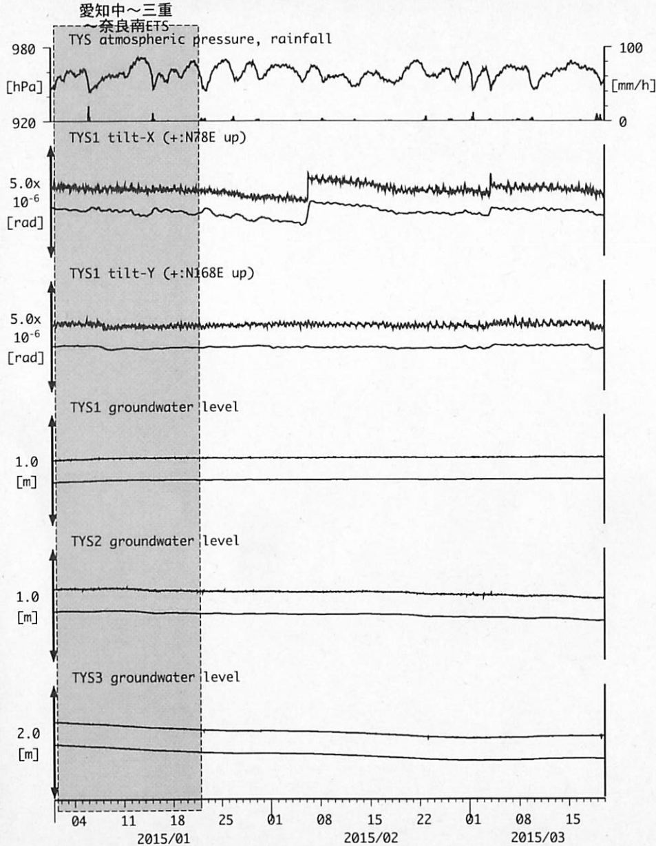
図3: Tilt and groundwater level changes at TYS 豊田神殿 (時間値) (2015/01/01 00:00 - 2015/03/20 00:00 (JST))
