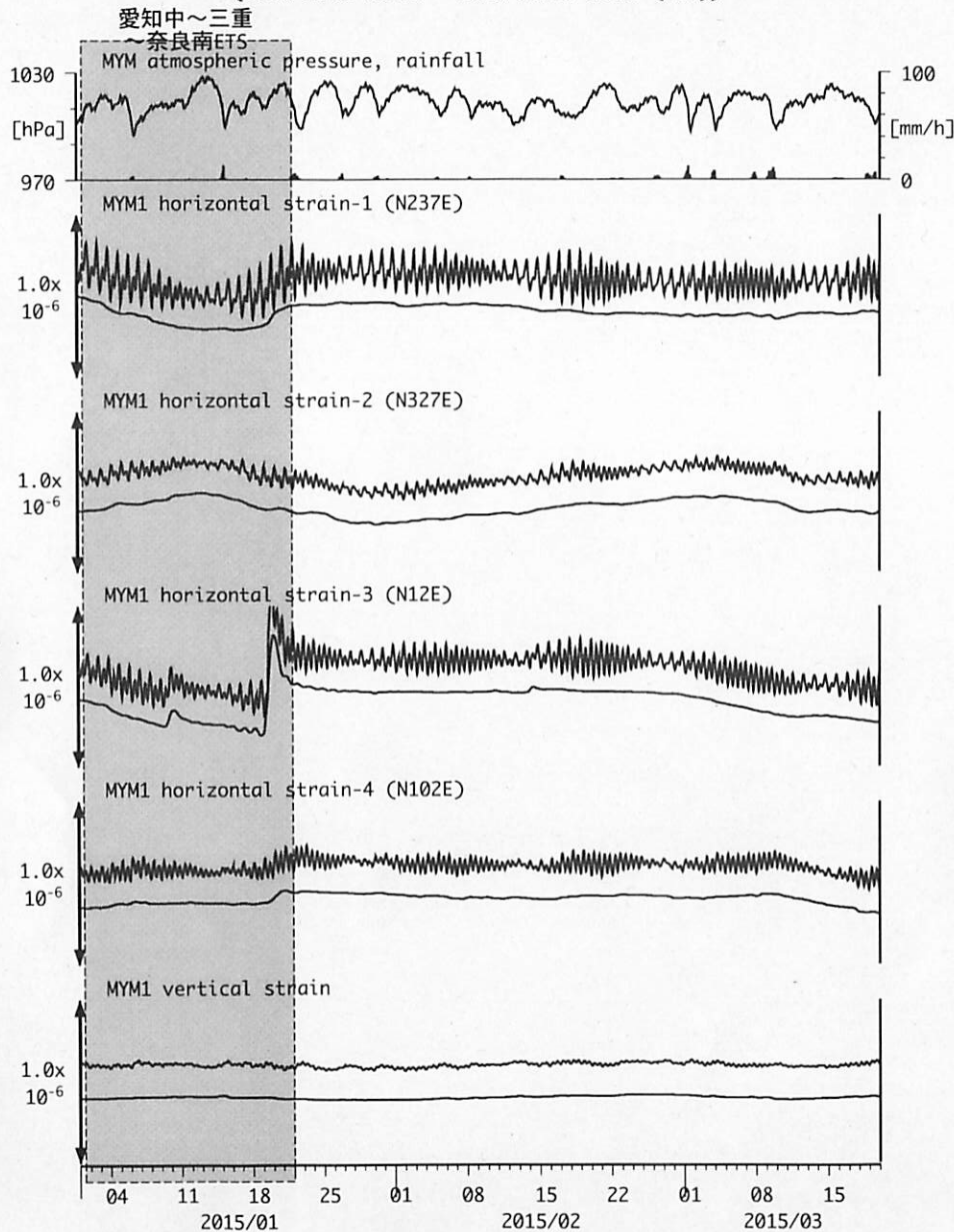
図13: Crustal strain changes at MYM 紀北海山 (時間値) (2015/01/01 00:00 - 2015/03/20 00:00 (JST))
