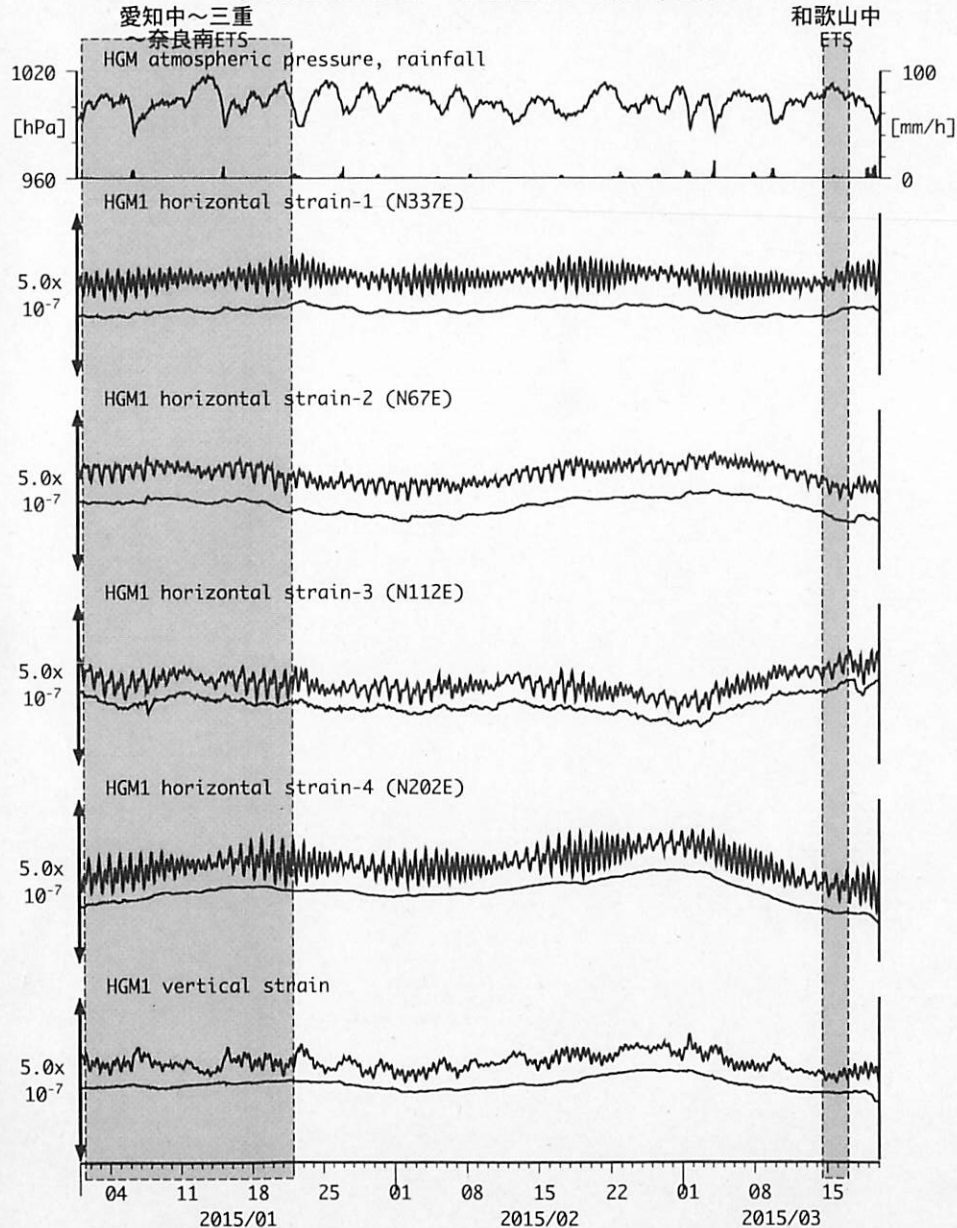
図17: Crustal strains changes at HGM 田辺本宮 (時間値) (2015/01/01 00:00 - 2015/03/20 00:00 (JST))
