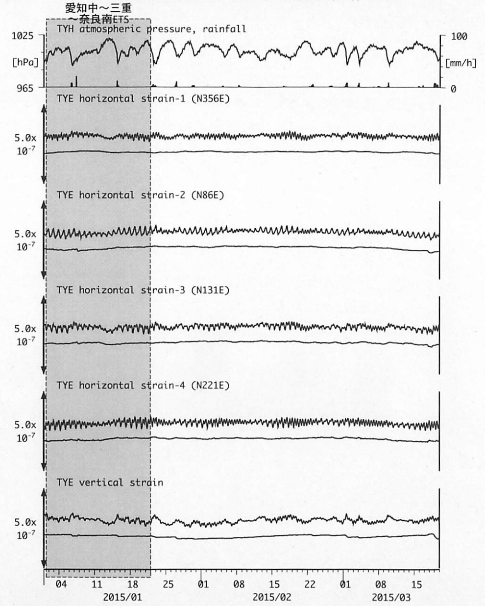
図6: Crustal strain changes at TYE 豊橋多米 (時間値) (2015/01/01 00:00 - 2015/03/20 00:00 (JST))
