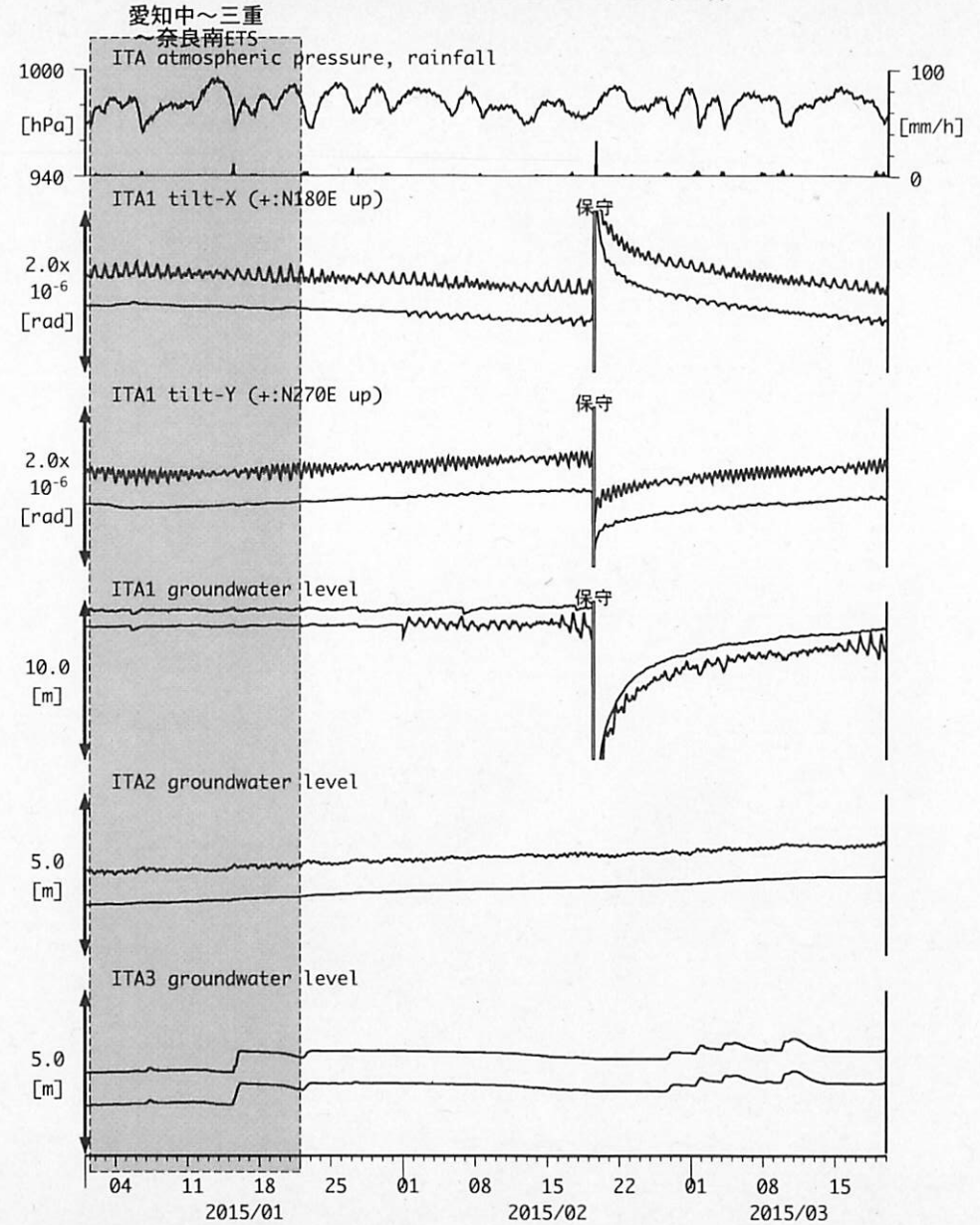
図12: Tilt and groundwater level changes at ITA 松阪飯高 (時間値) (2015/01/01 00:00 - 2015/03/20 00:00 (JST))
