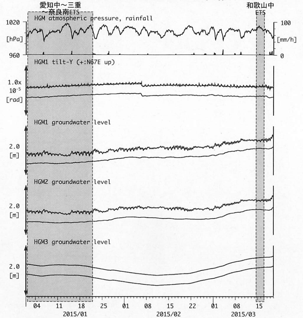
図18: Tilt and groundwater level changes at HGM 田辺本宮 (時間値) (2015/01/01 00:00 - 2015/03/20 00:00 (JST))
