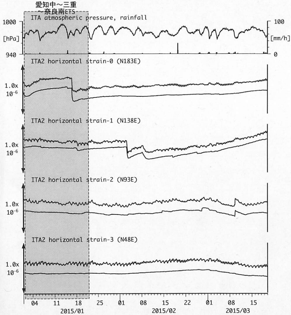
図11: Crustal strain changes at ITA 松阪飯高 (時間値) (2015/01/01 00:00 - 2015/03/20 00:00 (JST))
