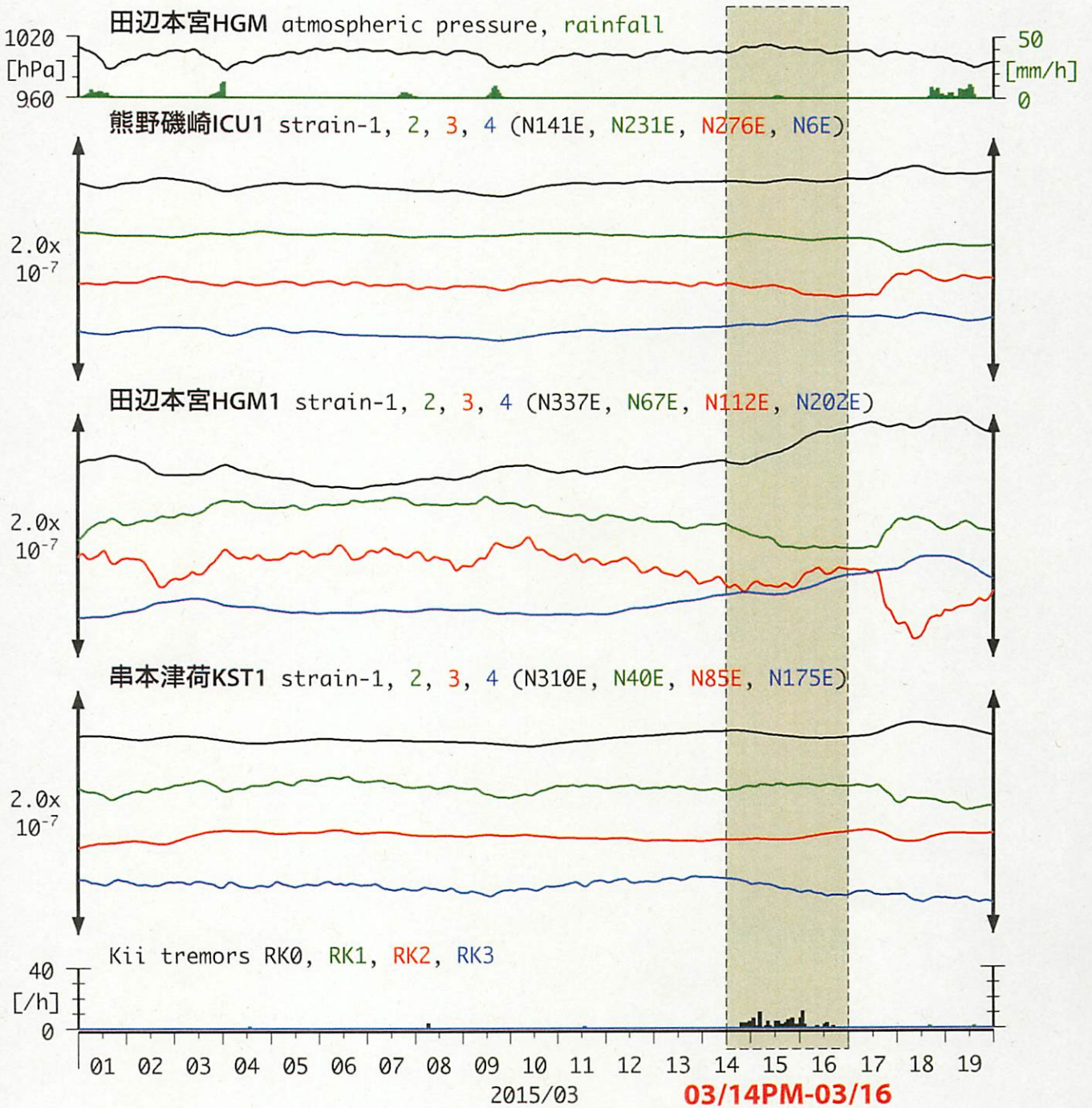
図 25 : 2015/03/01 0:00 - 03/20 0:00 の三重県・和歌山県の 3 観測点における水平歪の変化と、紀伊半島周辺の深部低周波微動の個数。水平歪は BAYTAP-G により潮汐・気圧応答・ノイズ成分除去後、さらに 03/01 0:00 - 03/14 0:00 の値を用いて 1 次トレンドを除去したものを示している。
