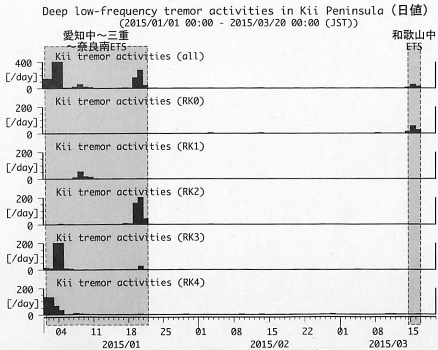
図 23 (上段) 紀伊半島における深部低周波微動の時空間分布、(下段) 各領域における発生頻度 (日値)。
