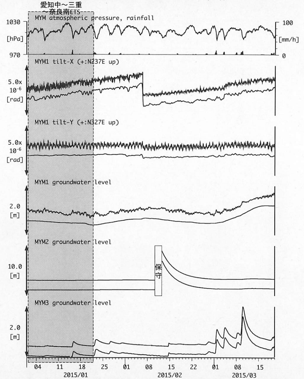
図14: Tilt and groundwater level changes at MYM 紀北海山 (時間値) (2015/01/01 00:00 - 2015/03/20 00:00 (JST))
