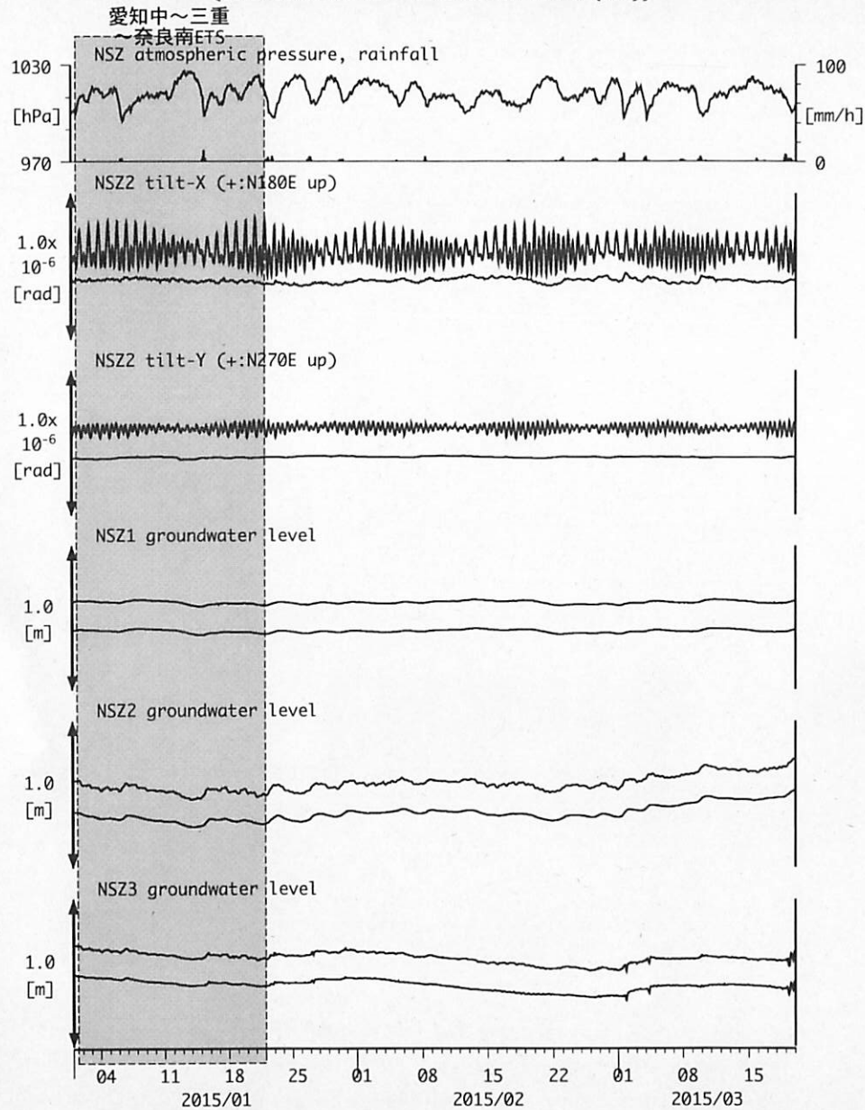
図5: Tilt and groundwater level changes at NSZ 西尾善明 (時間値) (2015/01/01 00:00 - 2015/03/20 00:00 (JST))
