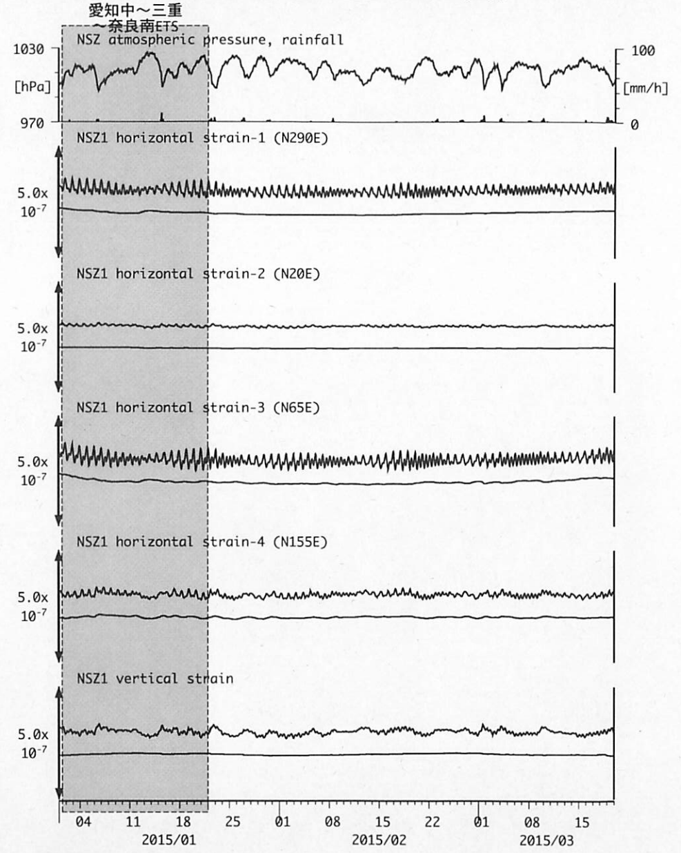
図4: Crustal strains changes at NSZ 西尾善明 (時間値) (2015/01/01 00:00 - 2015/03/20 00:00 (JST))
