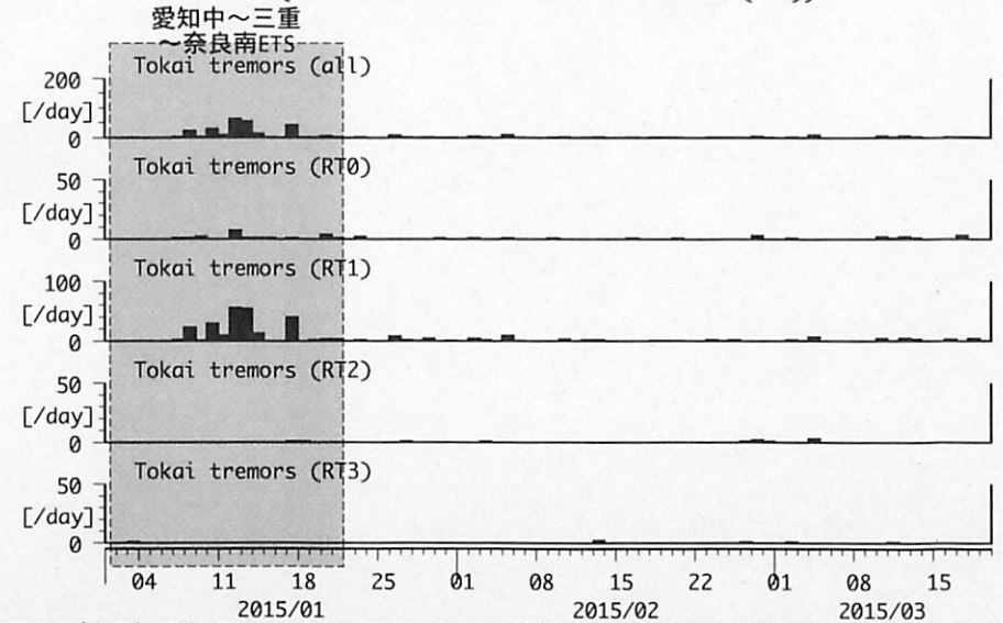
図22 (上段) 愛知県およびその周辺における深部低周波微動の時空間分布、(下段) 各領域における発生頻度 (日値)。
