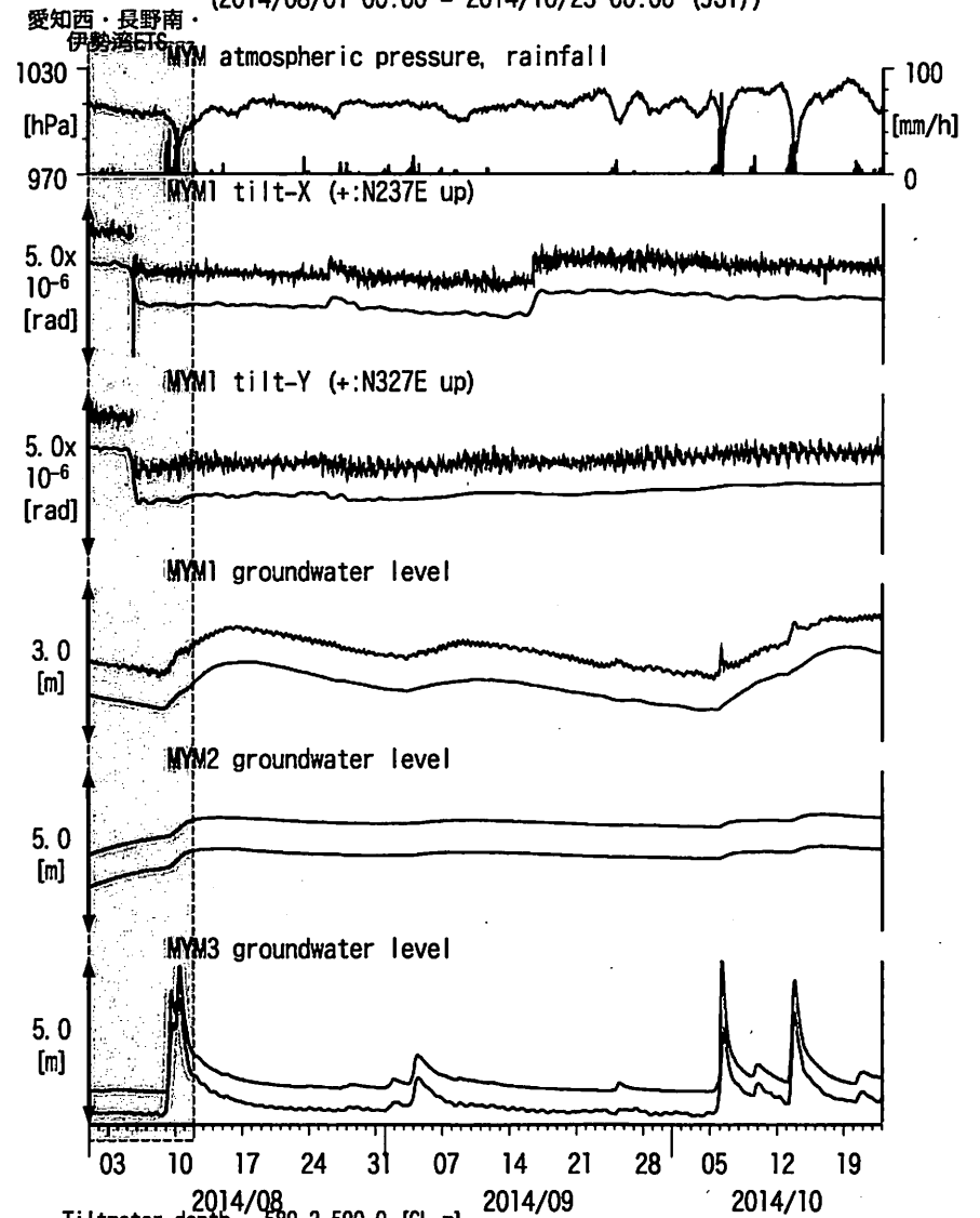
図14: Tilt and groundwater level changes at MYM 紀北海山 (時間値) (2014/08/01 00:00 - 2014/10/23 00:00 (JST))
