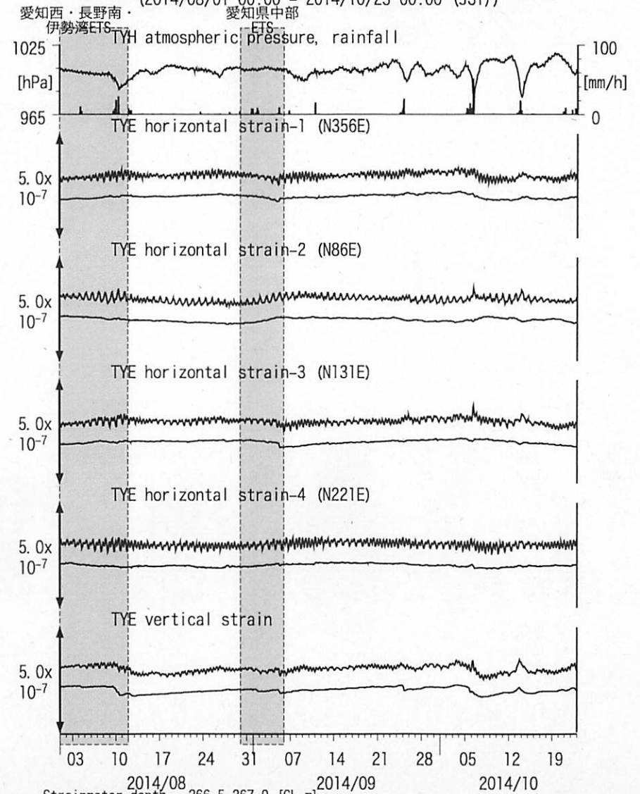
図6: Crustal strain changes at TYE 豊橋多米 (時間値) (2014/08/01 00:00 - 2014/10/23 00:00 (JST))
