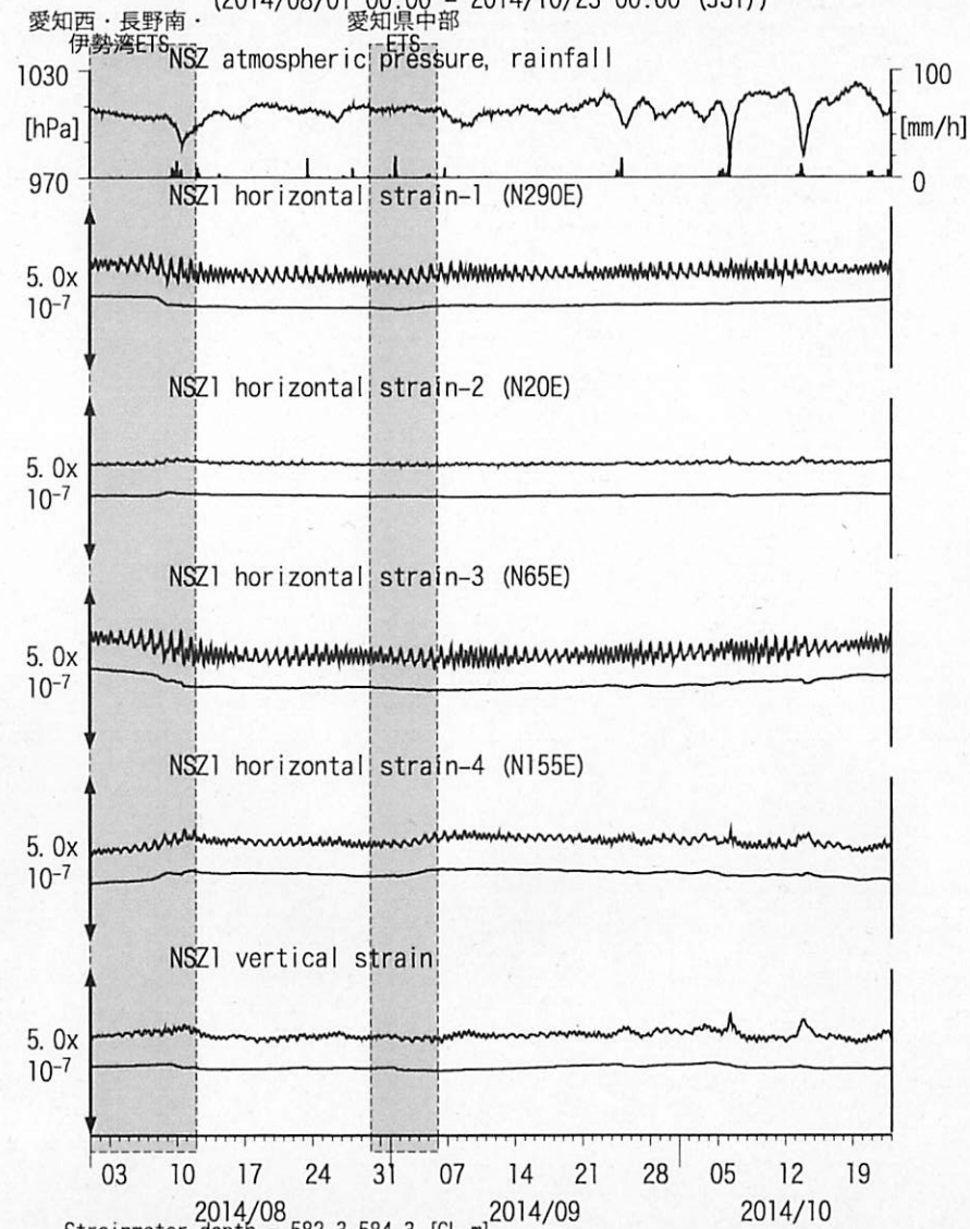
図4: Crustal strains changes at NSZ 西尾善明 (時間値) (2014/08/01 00:00 - 2014/10/23 00:00 (JST))
