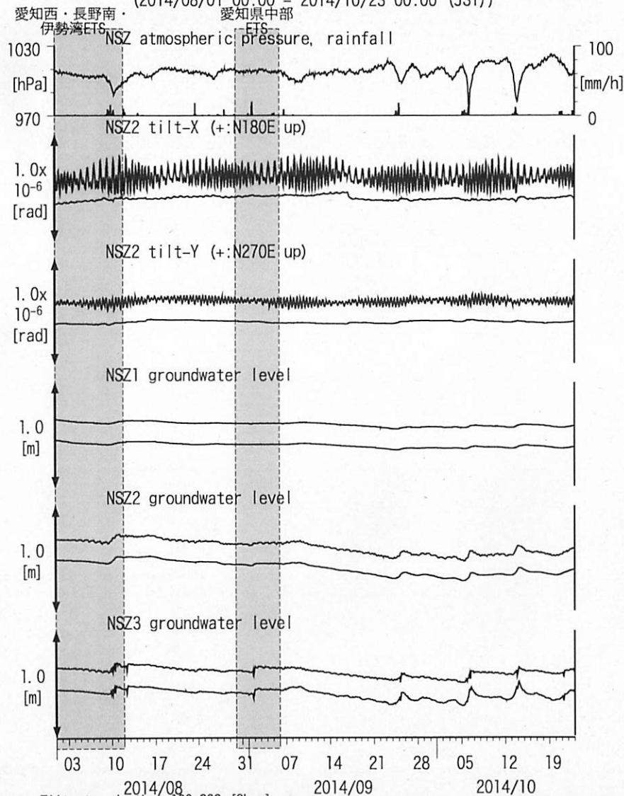
図5: Tilt and groundwater level changes at NSZ 西尾善明 (時間値) (2014/08/01 00:00 - 2014/10/23 00:00 (JST))
