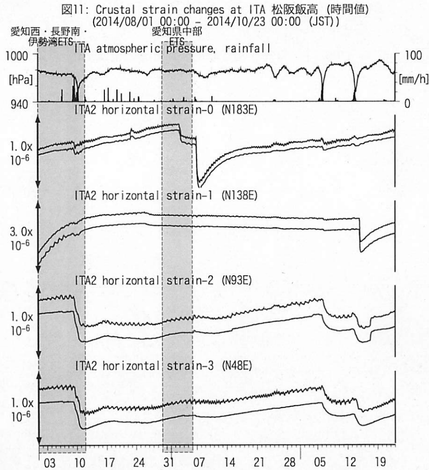
図11: Crustal strain changes at ITA 松阪飯高 (時間値) (2014/08/01 00:00 - 2014/10/23 00:00 (JST)) 愛知西・長野南・伊勢湾 ETS 愛知県中部 ETS ITA atmospheric pressure, rainfall Strainmeter depth = 181.3-183.6 [GL-m] 上: 1次トレンド除去 下: BAYTAP-Gにより潮汐・気圧応答・ノイズ成分除去後に1次トレンド除去
