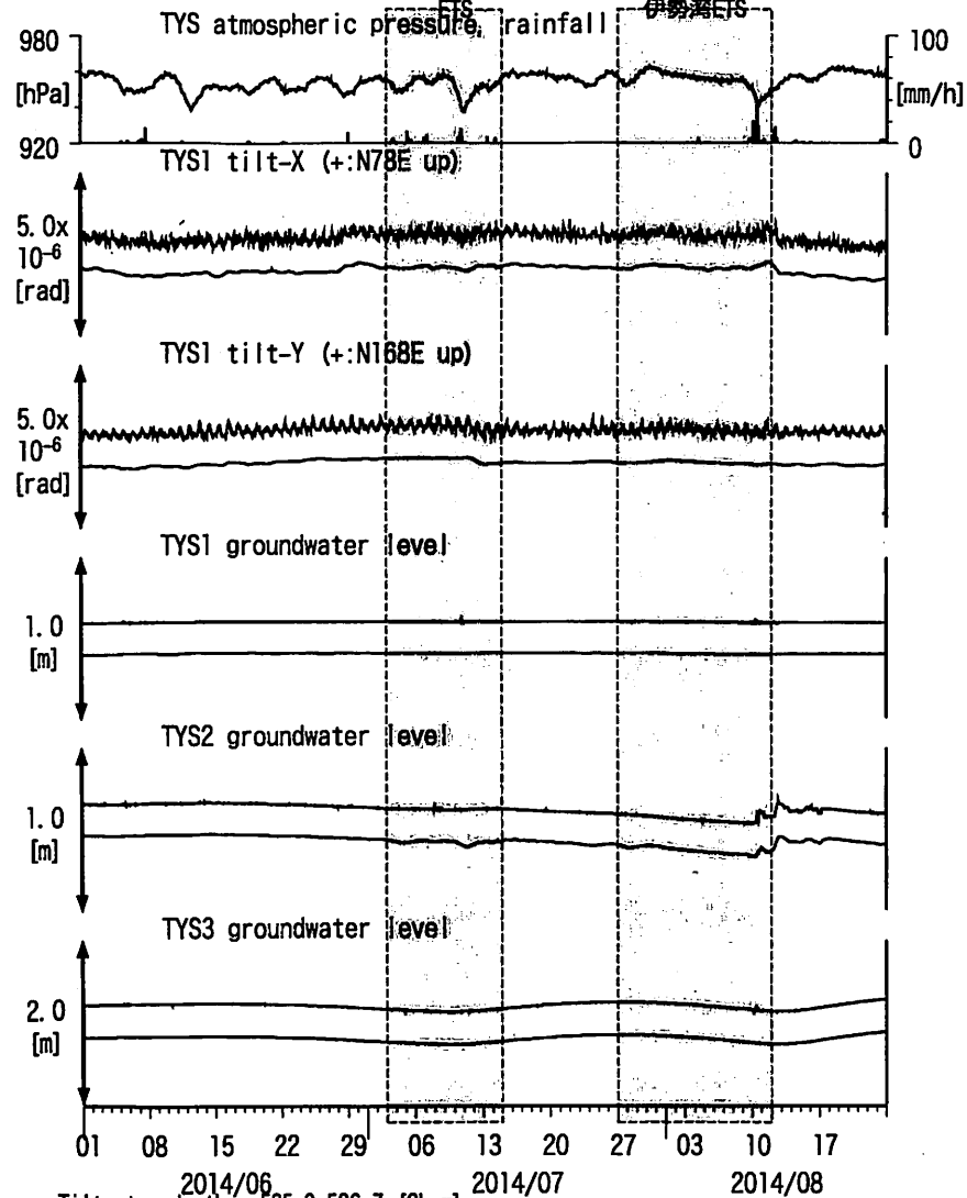
図3: Tilt and groundwater level changes at TYS 豊田神殿 (時間値) (2014/06/01 00:00 - 2014/08/24 00:00 (JST)) 伊勢湾~奈良南 愛知西・長野南 伊勢湾ETS
