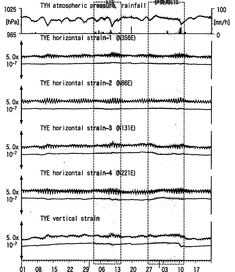
図6: Crustal strain changes at TYE 豊橋多米 (時間値) (2014/06/01 00:00 - 2014/08/24 00:00 (JST)) 伊勢湾~奈良南 愛知西・長野南・伊勢湾ETS
