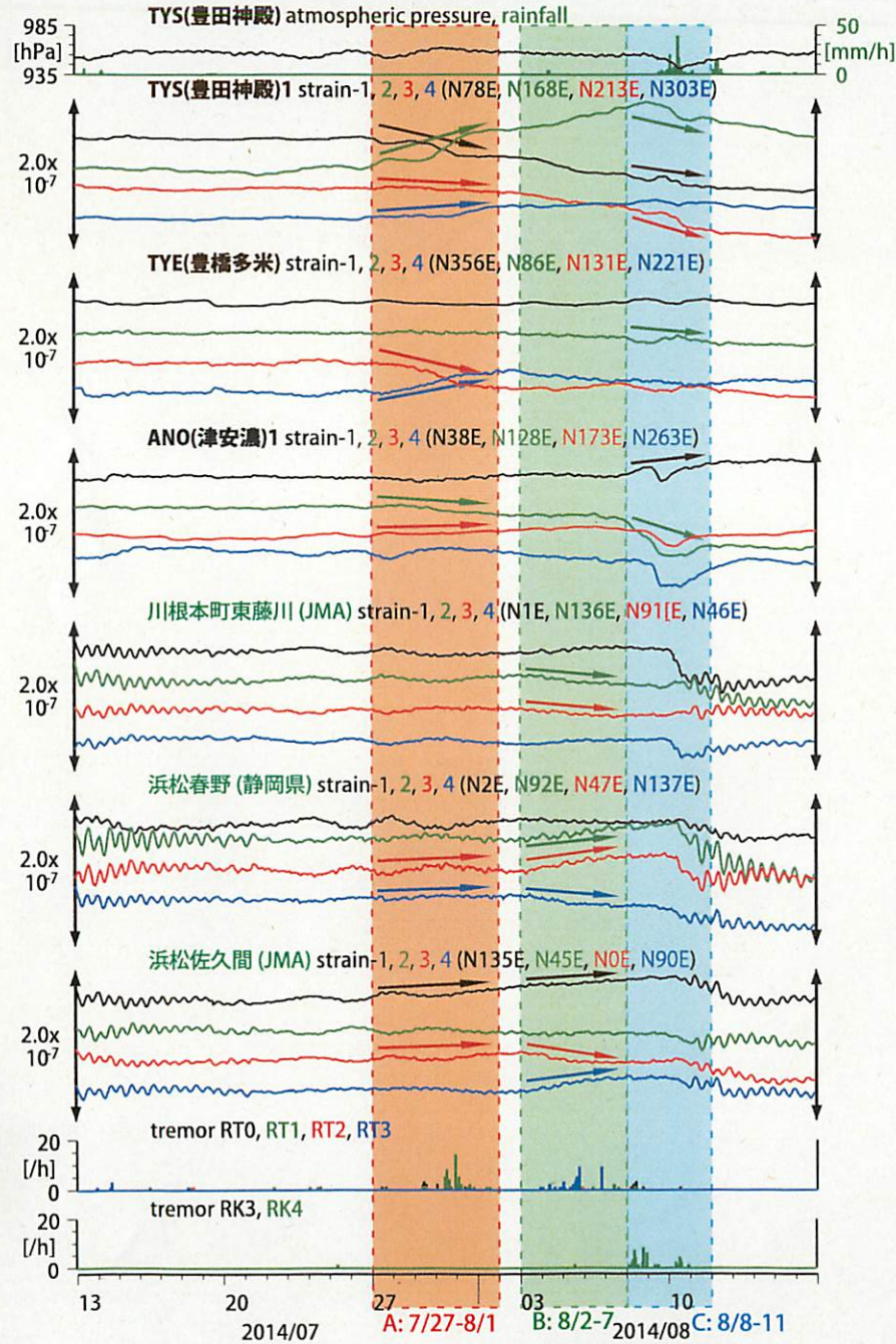
図25: 東海地方における歪・地下水・傾斜観測結果(時間値) (2014/07/13 00:00 - 2014/08/17 00:00 (JST))
