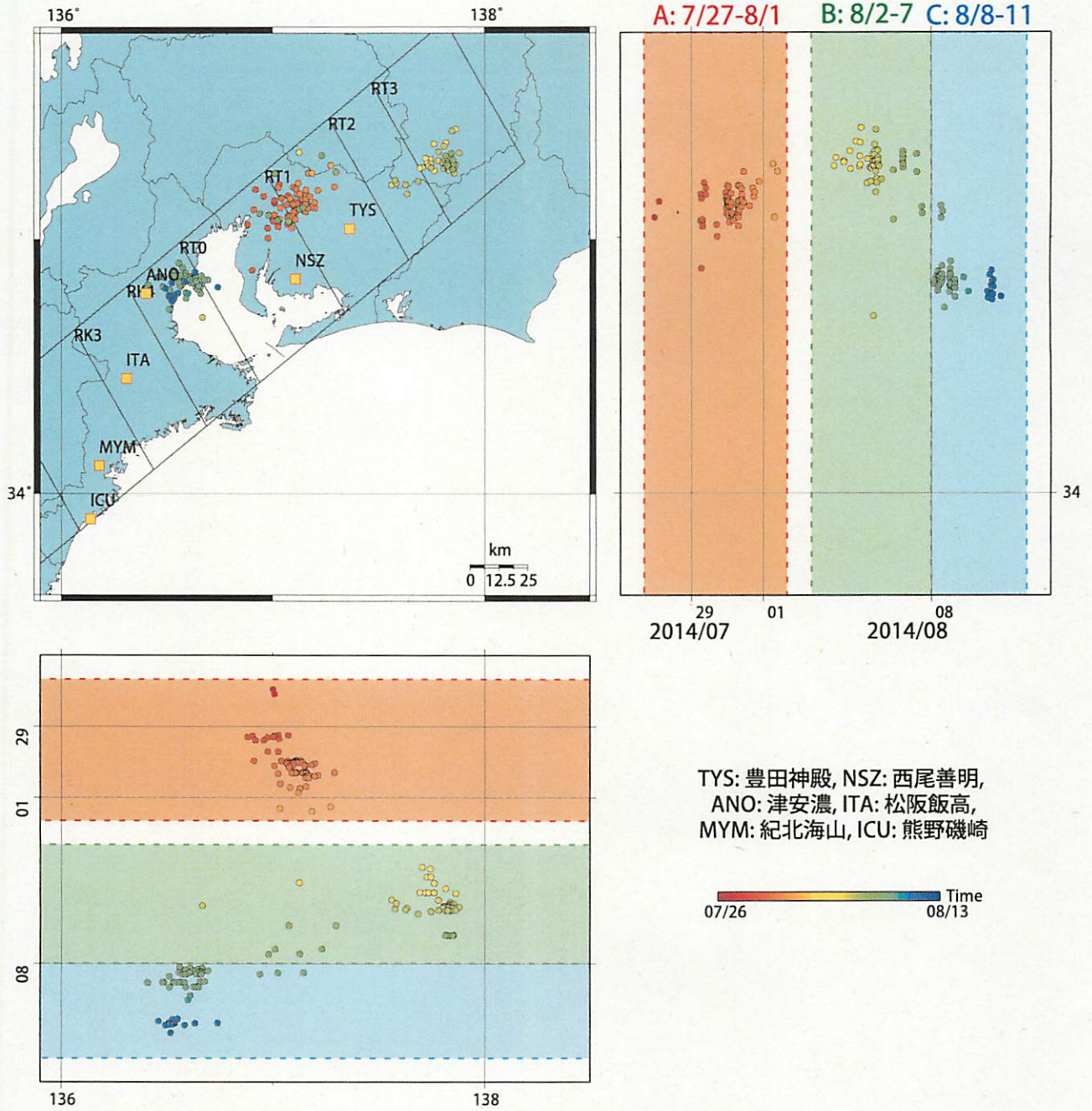
図24: 2014/7/26 0:00 - 8/13 0:00 における愛知県周辺の深部低周波微動の時空間分布図。エンベロープ相関法により決定。
