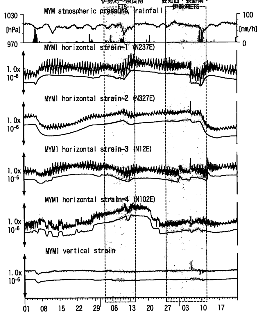
図13: Crustal strain changes at MYM 紀北海山 (時間値) (2014/06/01 00:00 - 2014/08/24 00:00 (JST))
