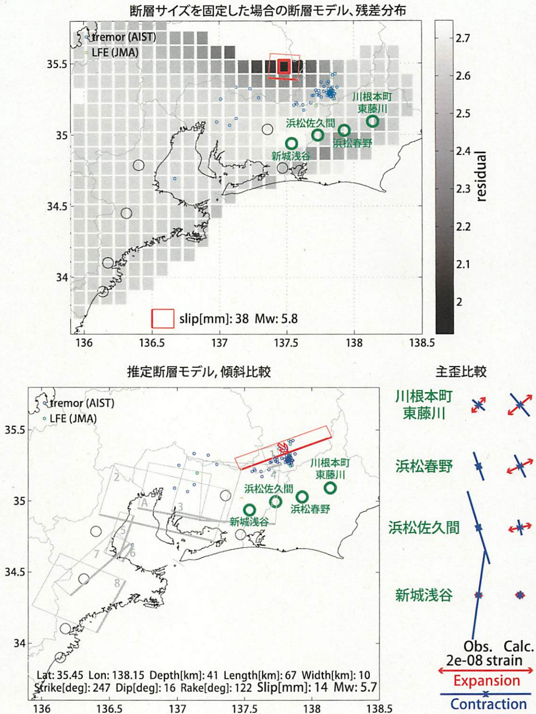
図27: (上段)プレート境界面上のパッチ(断層面)をすべらせた際の、歪の観測値と計算値の残差分布図。断層面サイズは固定(20x20km)。赤色矩形は最小残差の断層面を表す。このパッチのすべり量、Mwを下部に示している。
