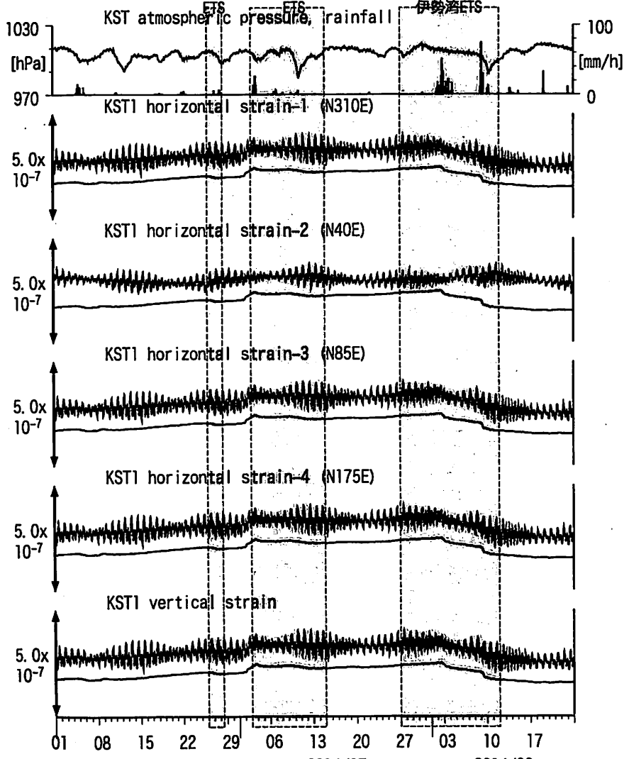
図19: Crustal strain changes at KST 串本津荷 (時間値) (2014/06/01 00:00 - 2014/08/24 00:00 (JST)) 和歌山中伊勢湾~奈良南 愛知西・長野南・伊勢湾ETS
