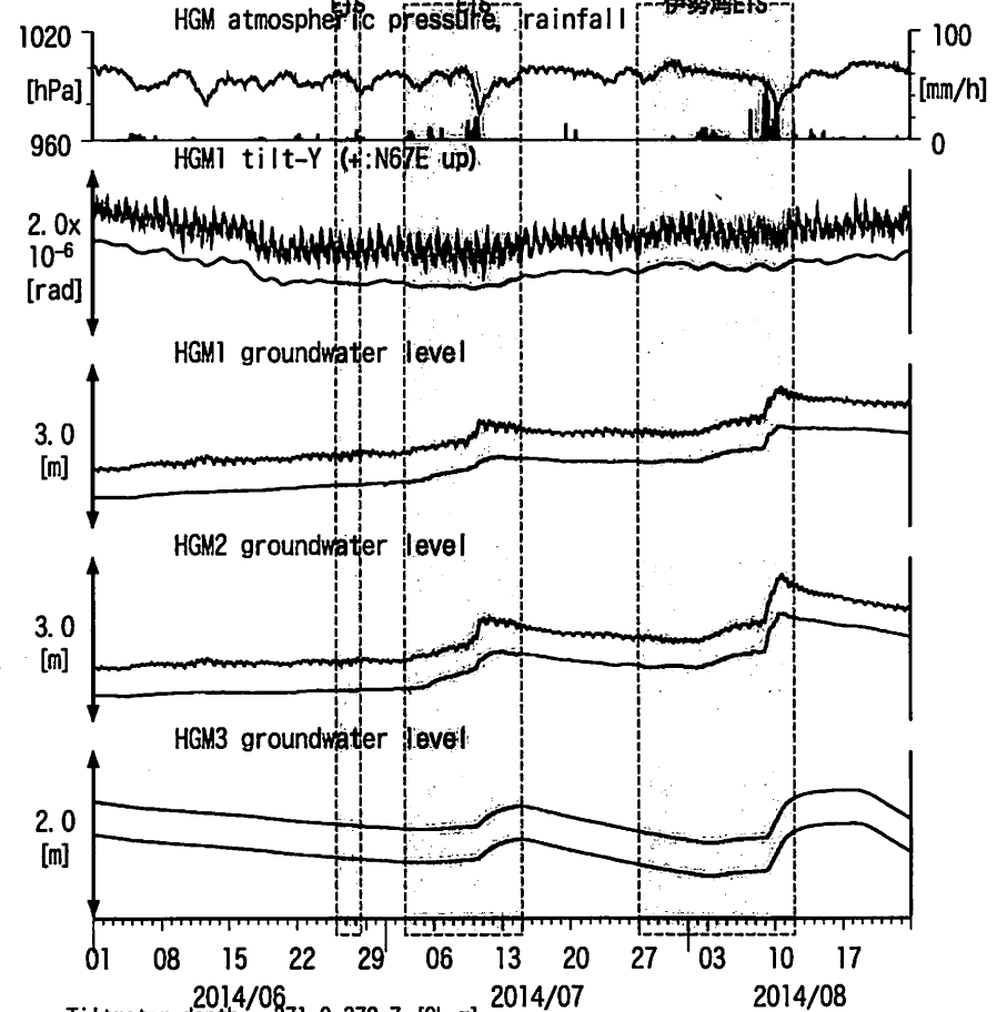
図18: Tilt and groundwater level changes at HGM 田辺本宮 (時間値) (2014/06/01 00:00 - 2014/08/24 00:00 (JST)) 和歌山中伊勢湾~奈良南 愛知西・長野南・伊勢湾ETS
