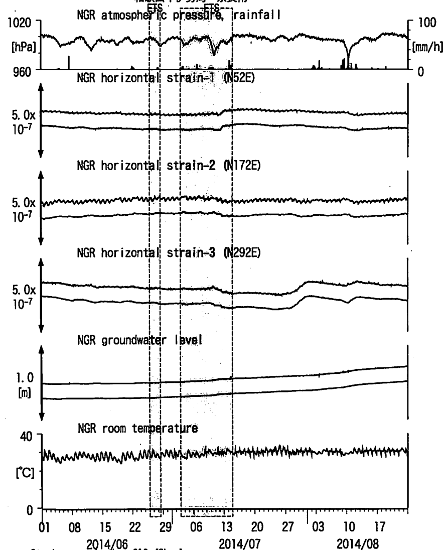
図21: Crustal strain and groundwater level changes at 岩出東坂本 (時間値) (2014/06/01 00:00 - 2014/08/24 00:00 (JST)) 和歌山中伊勢湾~奈良南
