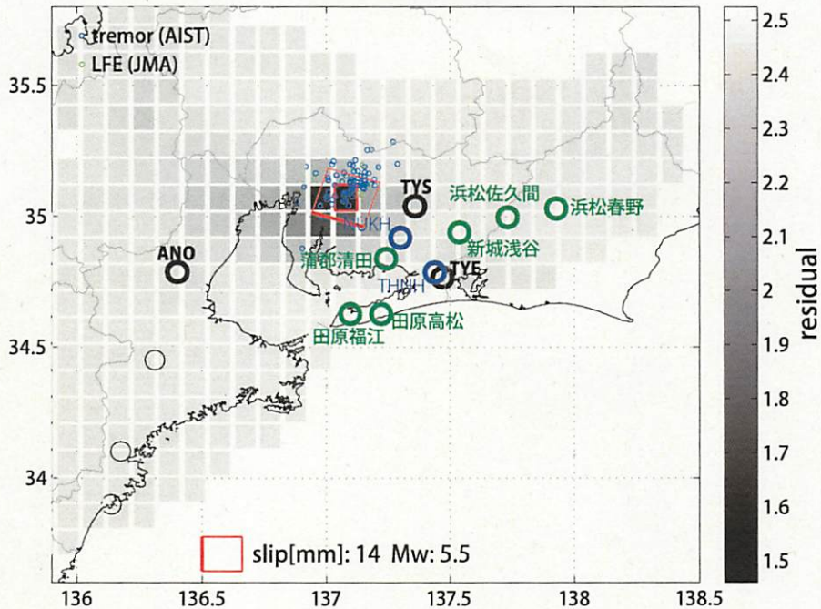
推定断層モデル、傾斜比較
