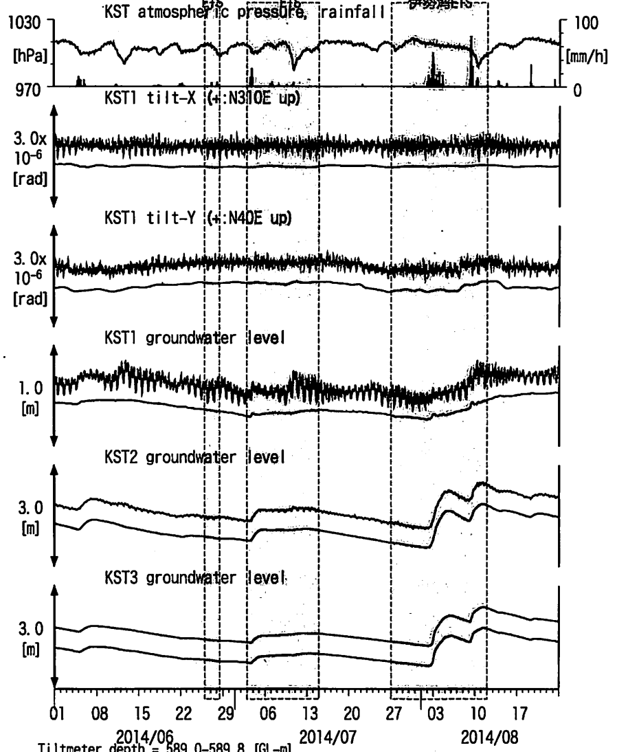
図20: Tilt and groundwater level changes at KST 串本津荷 (時間値) (2014/06/01 00:00 - 2014/08/24 00:00 (JST)) 和歌山中伊勢湾~奈良南 愛知西・長野南・伊勢湾ETS
