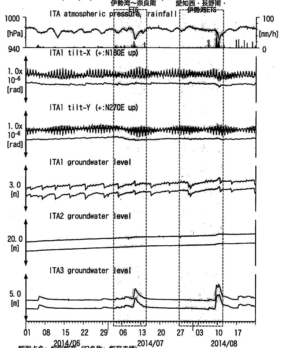
図12: Tilt and groundwater level changes at ITA 松阪飯高 (時間値) (2014/06/01 00:00 - 2014/08/24 00:00 (JST))
