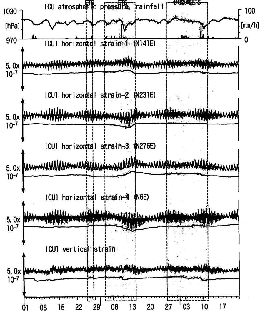
図15: Crustal strain changes at ICU 熊野磯崎 (時間値) (2014/06/01 00:00 - 2014/08/24 00:00 (JST)) 和歌山中伊勢湾~奈良南 愛知西・長野南・伊勢湾ETS
