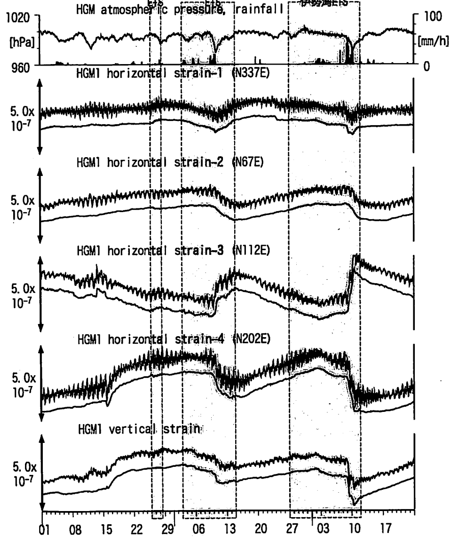
図17: Crustal strains changes at HGM 田辺本宮 (時間値) (2014/06/01 00:00 - 2014/08/24 00:00 (JST)) 和歌山中伊勢湾~奈良南 愛知西・長野南・伊勢湾ETS
