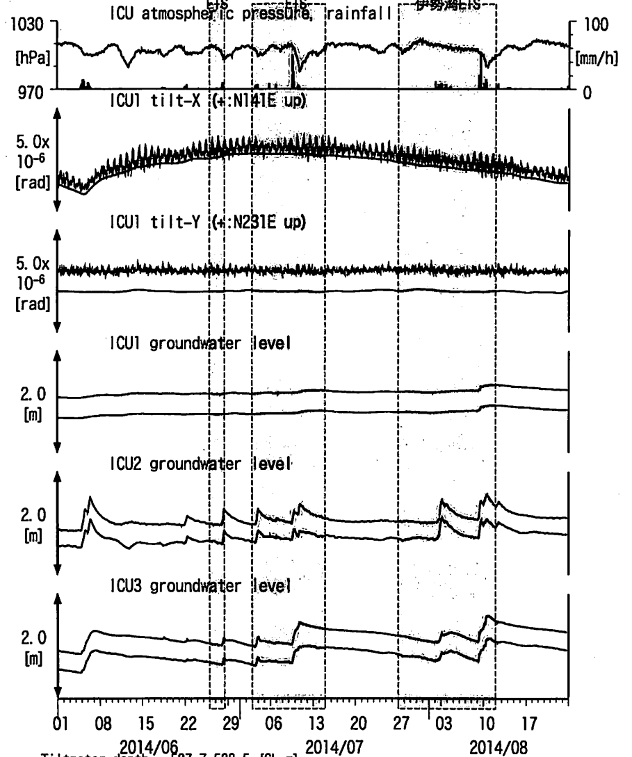
図16: Tilt and groundwater level changes at ICU 熊野磯崎 (時間値) (2014/06/01 00:00 - 2014/08/24 00:00 (JST)) 和歌山中伊勢湾~奈良南 愛知西・長野南・伊勢湾ETS
