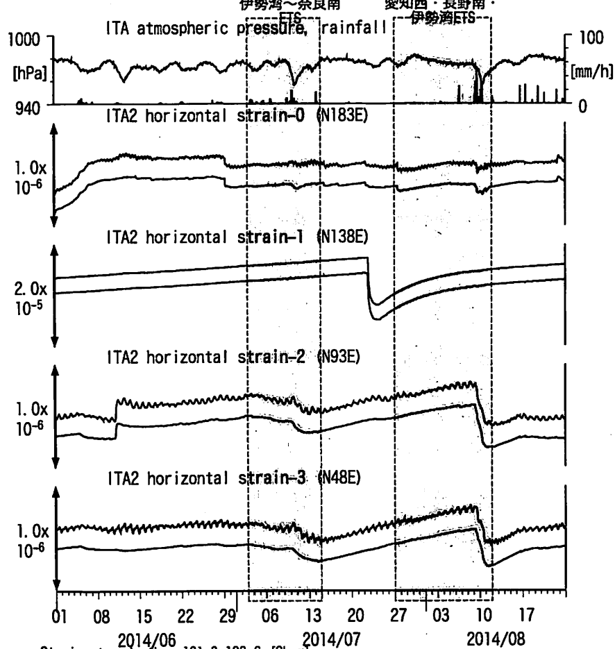
図11: Crustal strain changes at ITA 松阪飯高 (時間値) (2014/06/01 00:00 - 2014/08/24 00:00 (JST))
