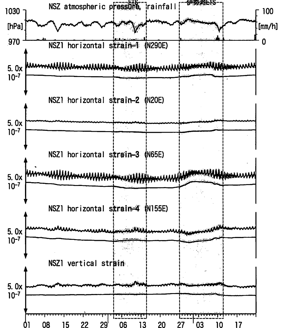
図4: Crustal strains changes at NSZ 西尾善明 (時間値) (2014/06/01 00:00 - 2014/08/24 00:00 (JST)) 伊勢湾~奈良南 愛知西・長野南 伊勢湾ETS
