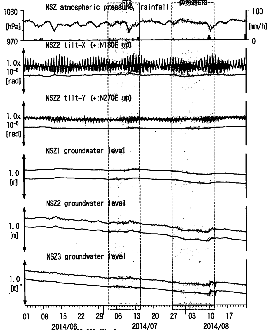
図5: Tilt and groundwater level changes at NSZ 西尾善明 (時間値) (2014/06/01 00:00 - 2014/08/24 00:00 (JST)) 伊勢湾~奈良南 愛知西・長野南・伊勢湾ETS
