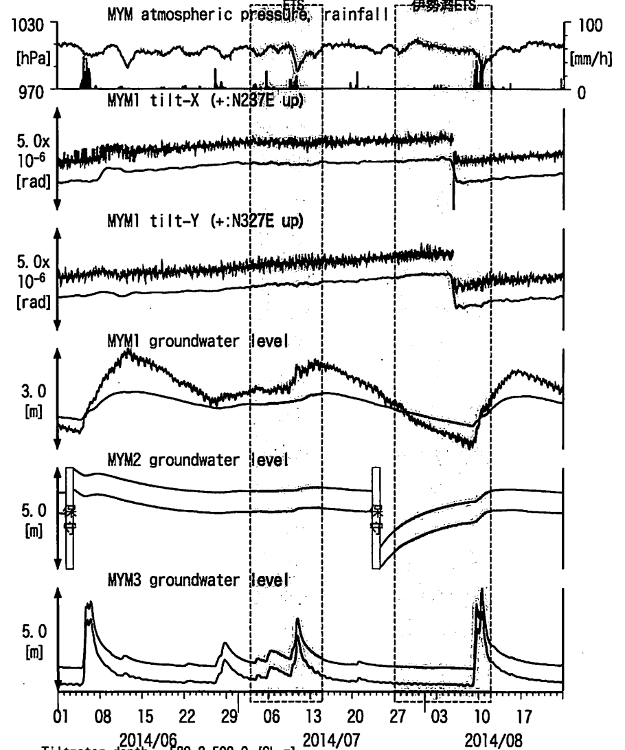
図14: Tilt and groundwater level changes at MYM 紀北海山 (時間値) (2014/06/01 00:00 - 2014/08/24 00:00 (JST))
