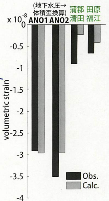
体積歪比較
