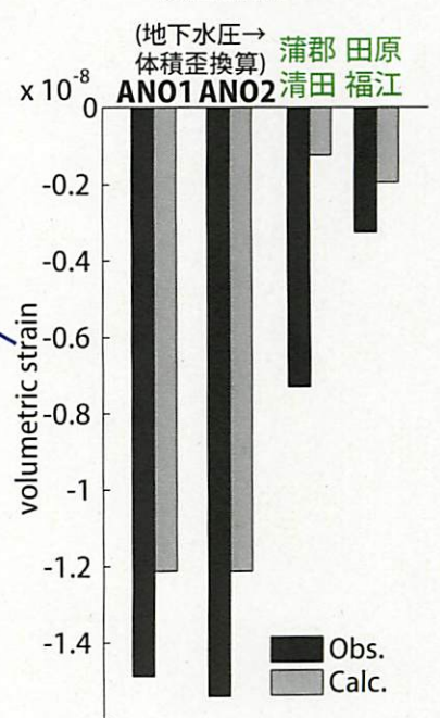
体積歪比較
