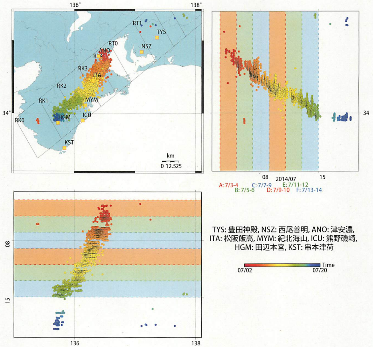
図24: 2014/7/2 0:00 - 7/20 0:00 における紀伊半島および愛知県周辺の深部低周波微動の時空間分布図。エンベロープ相関法により決定。
