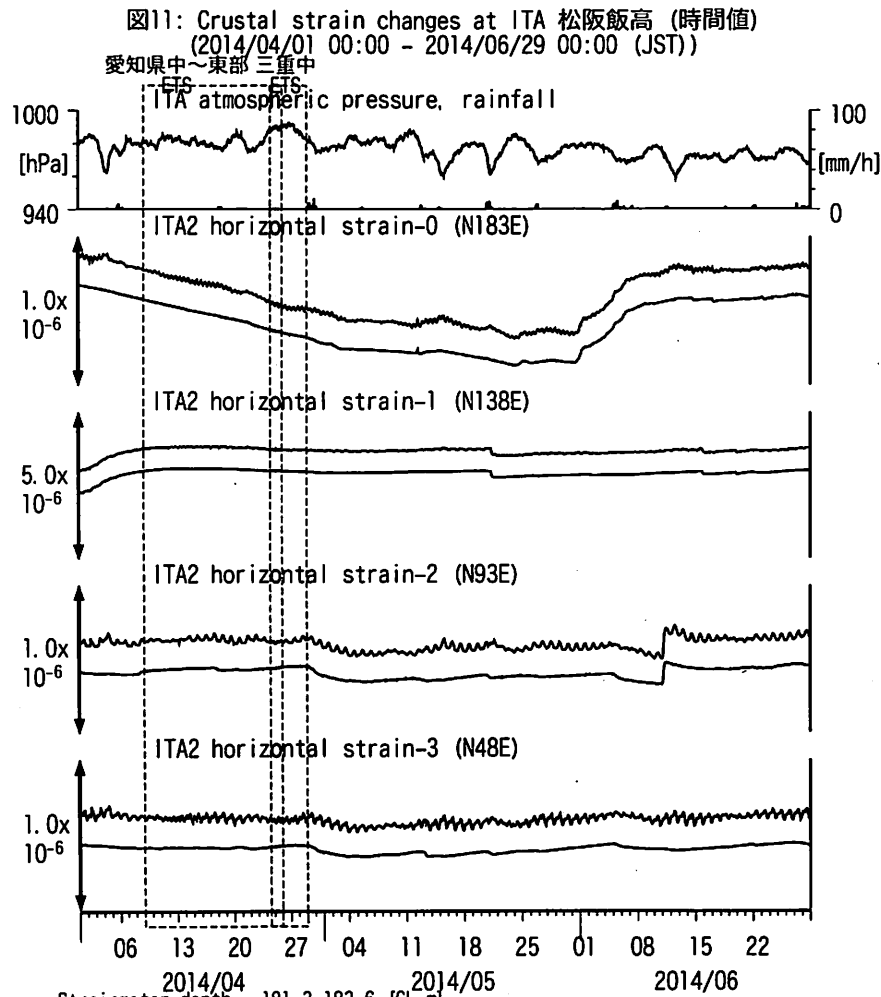
図11: Crustal strain changes at ITA 松阪飯高 (時間値) (2014/04/01 00:00 - 2014/06/29 00:00 (JST)) 愛知県中～東部 三重中 FTS FTS ITA atmospheric pressure, rainfall Strainmeter depth = 181.3-183.6 [GL-m] 上: 1次トレンド除去 下: BAYTAP-Gにより潮汐・気圧応答・ノイズ成分除去後に1次トレンド除去
