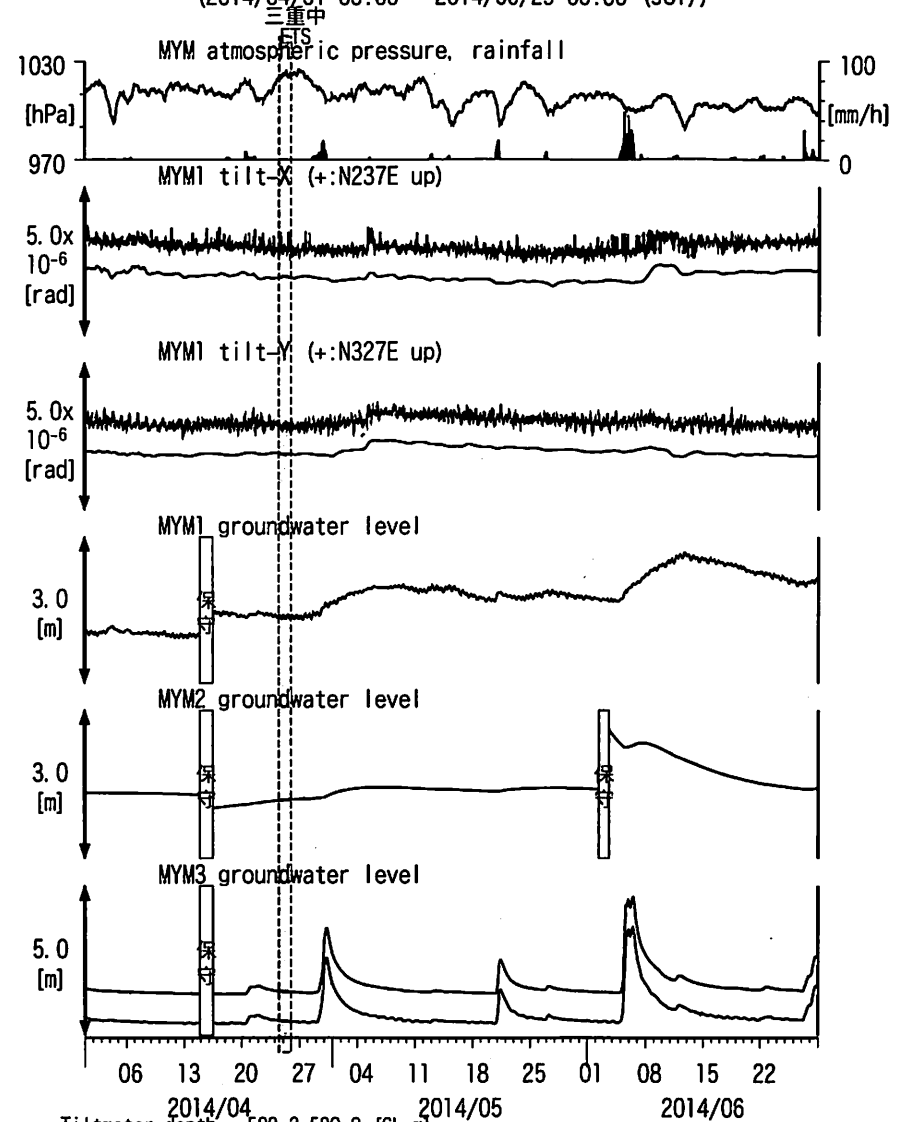
図14: Tilt and groundwater level changes at MYM 紀北海山 (時間値) (2014/04/01 00:00 - 2014/06/29 00:00 (JST))
