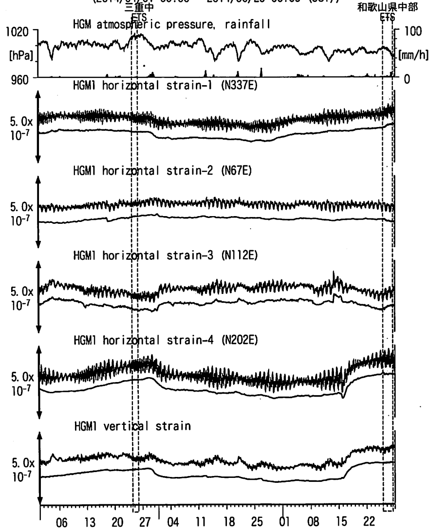
図17: Crustal strains changes at HGM 田辺本宮 (時間値) (2014/04/01 00:00 - 2014/06/29 00:00 (JST))
