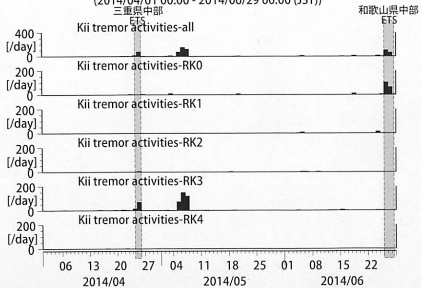
図 23: 紀伊半島における深部低周波微動の時空間分布 (上段)、各領域における発生頻度 (日値)。
