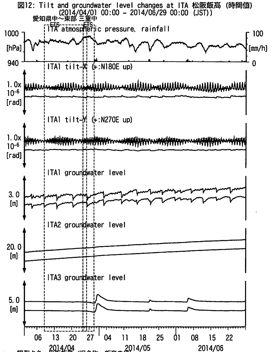
図12: Tilt and groundwater level changes at ITA 松阪飯高 (時間値) (2014/04/01 00:00 - 2014/06/29 00:00 (JST)) 愛知県中～東部 三重中 FTS FTS ITA atmospheric pressure, rainfall 観測点名: 松阪飯高 (旧名称: 飯高赤桶) Tiltmeter depth = 596.7-597.3 [GL-m] ITA1: Screen depth = 547.6-558.5 [GL-m] ITA2: Screen depth = 145.5-156.4 [GL-m] ITA3: Screen depth = 10.8-16.3 [GL-m] 上: tiltは1次トレンド除去 下: BAYTAP-Gにより潮汐・気圧応答・ノイズ成分除去、tiltは1次トレンドも除去 ITA2は2013/11/26に孔口を密閉した
