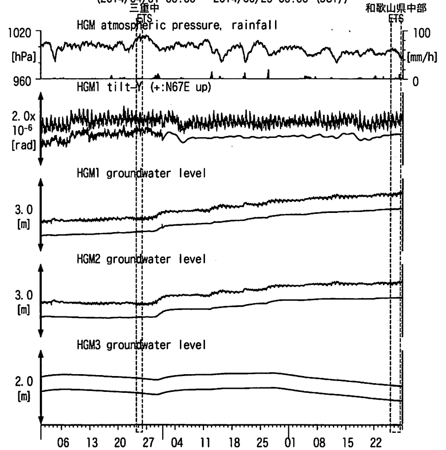
図18: Tilt and groundwater level changes at HGM 田辺本宮 (時間値) (2014/04/01 00:00 - 2014/06/29 00:00 (JST))
