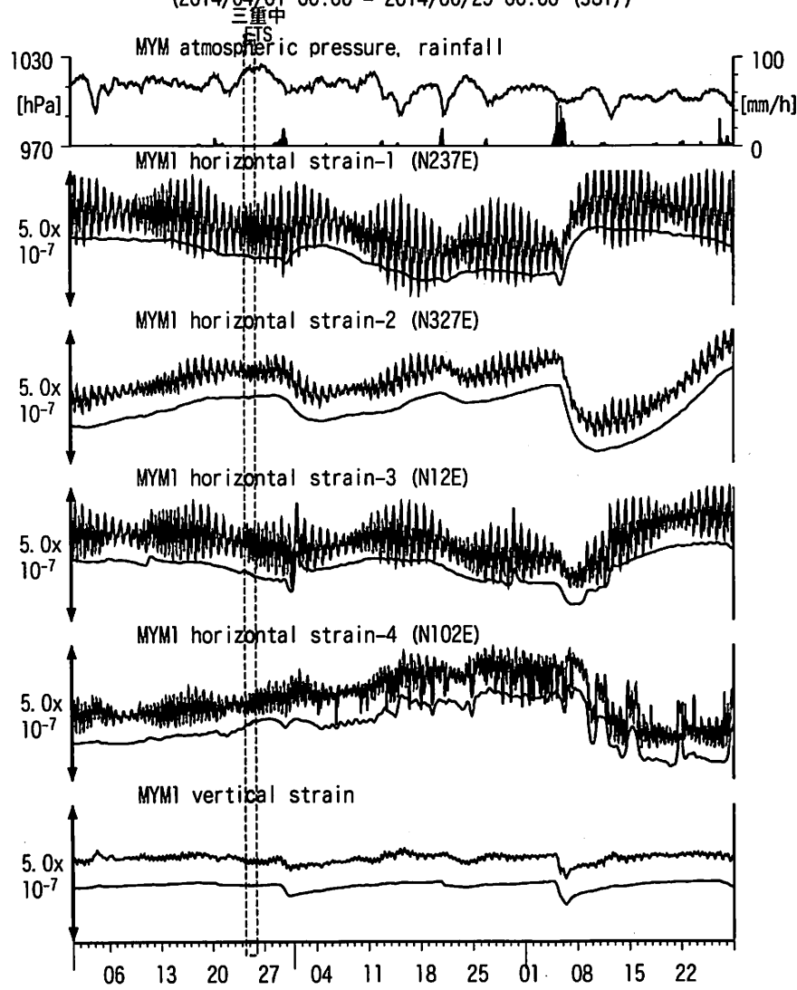
図13: Crustal strain changes at MYM 紀北海山 (時間値) (2014/04/01 00:00 - 2014/06/29 00:00 (JST))
