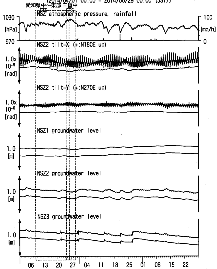
図5: Tilt and groundwater level changes at NSZ 西尾善明 (時間値) (2014/04/01 00:00 - 2014/06/29 00:00 (JST))
