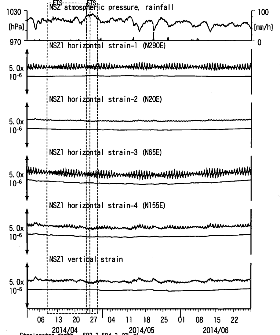
図4: Crustal strains changes at NSZ 西尾善明 (時間値)
