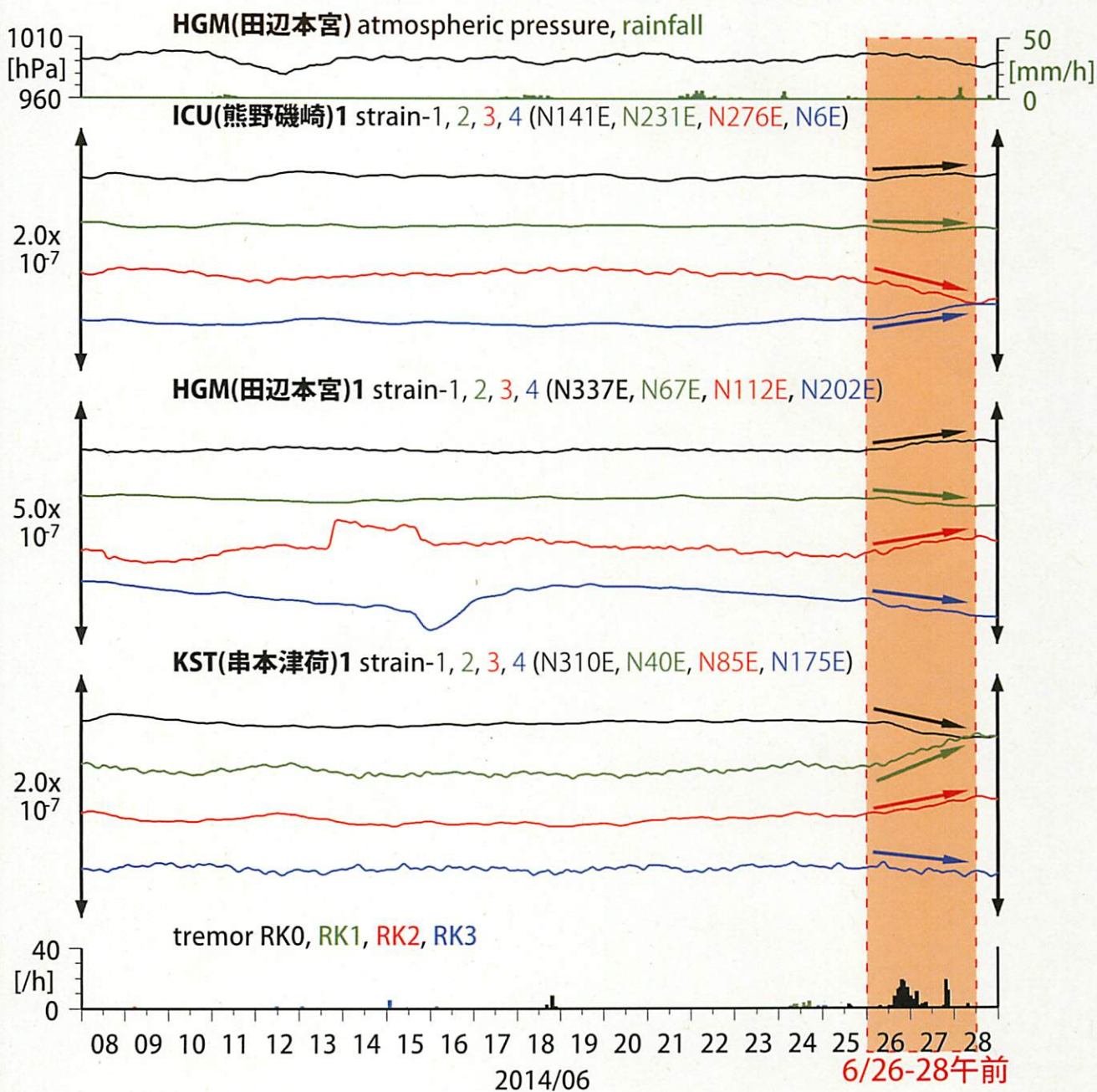
図25: 紀伊半島における歪観測結果 (2014/06/08 00:00 - 2014/06/29 00:00 (JST))
