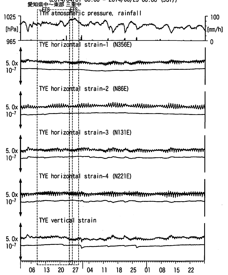
図6: Crustal strain changes at TYE 豊橋多米 (時間値) (2014/04/01 00:00 - 2014/06/29 00:00 (JST))
