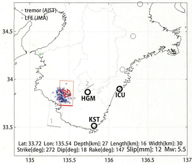
推定断層モデル、傾斜比較
