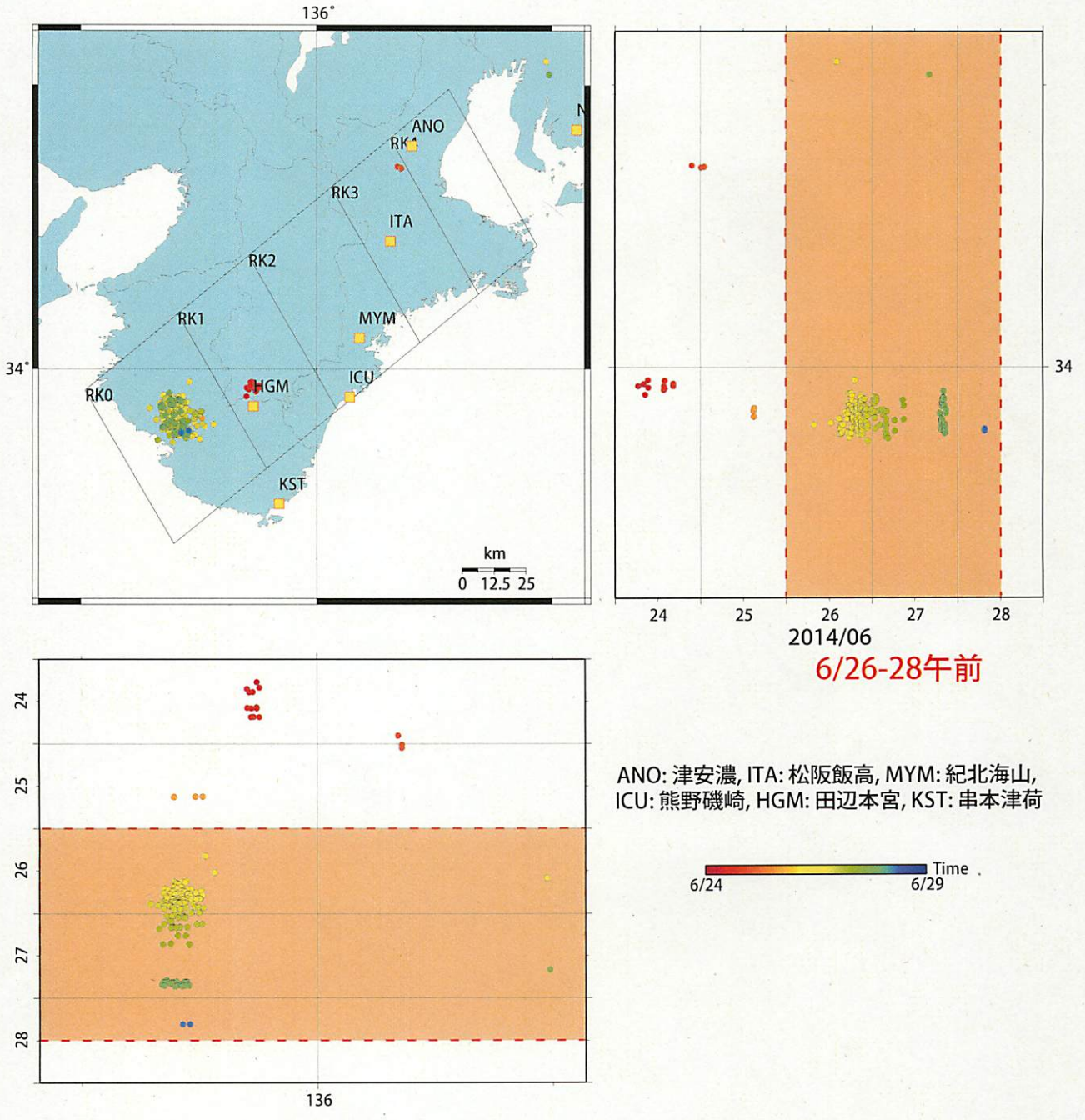
図24: 2014/6/24 0:00 - 6/29 0:00 における紀伊半島周辺の深部低周波微動の時空間分布図。エンベロープ相関法により決定。
