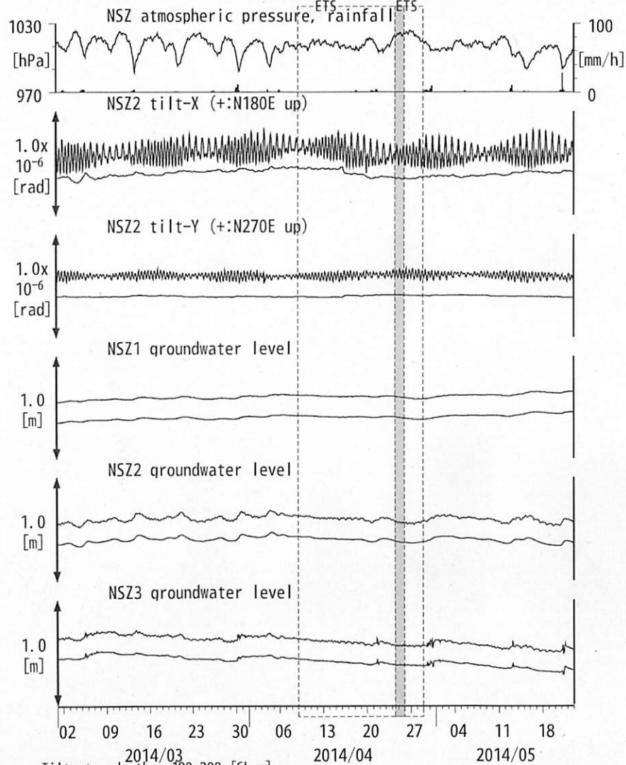
図5: Tilt and groundwater level changes at NSZ 西尾善明 (時間値) (2014/03/01 00:00 - 2014/05/23 00:00 (JST)) 愛知県中～東部 三重中
