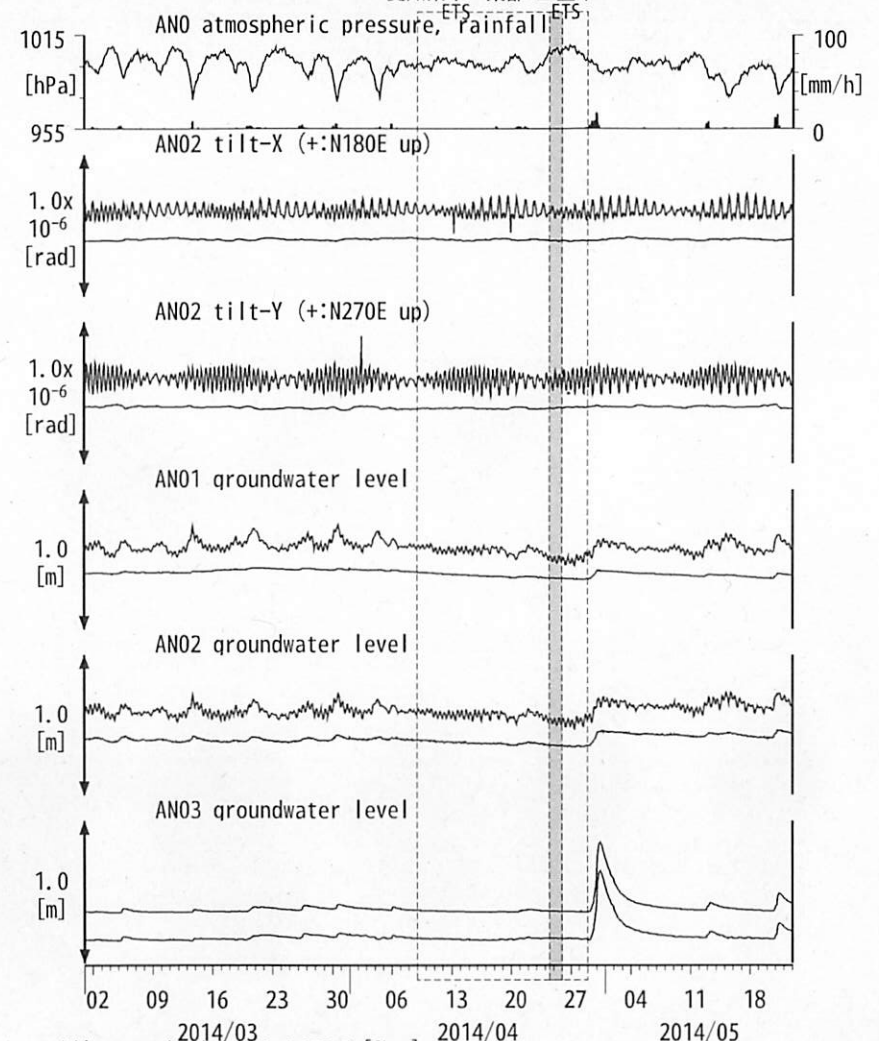
図10: Tilt and groundwater level changes at ANO 津安濃 (時間値) (2014/03/01 00:00 - 2014/05/23 00:00 (JST)) 愛知県中~東部 三重中
