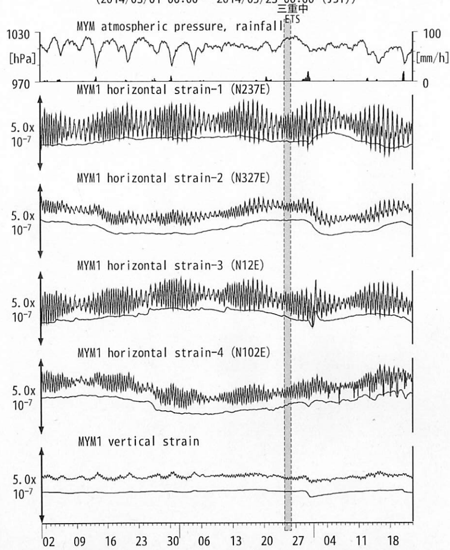
図13: Crustal strain changes at MYM 紀北海山 (時間値) (2014/03/01 00:00 - 2014/05/23 00:00 (JST))
