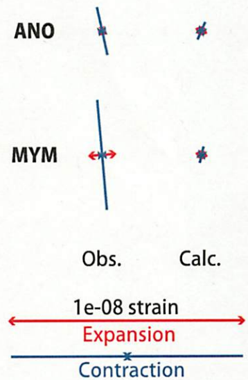
図32: (上段)プレート境界面上のパッチ(断層面)をすべらせた際の、歪・傾斜の観測値と計算値の残差分布図。断層面サイズは固定(20x20km)。赤色矩形は最小残差の断層面を表す。このパッチのすべり量、Mwを下部に示している。
