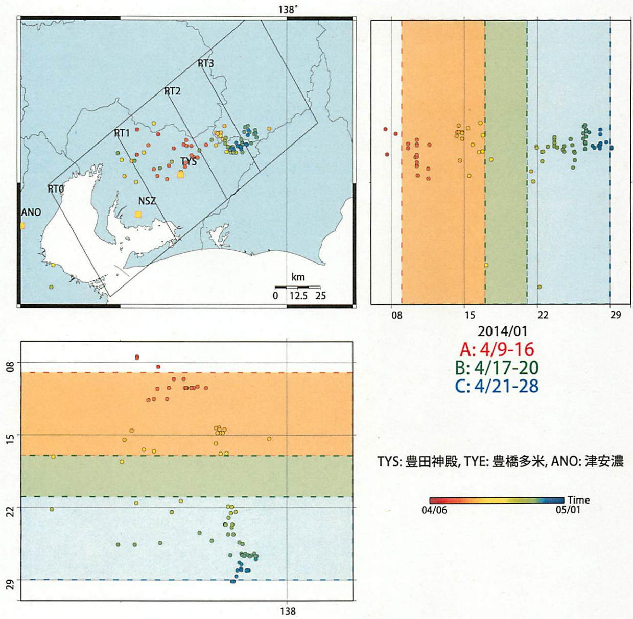
図24: 2014/4/9 0:00 - 5/1 0:00 における愛知県周辺の深部低周波微動の時空間分布図。エンベロープ相関法により決定。
