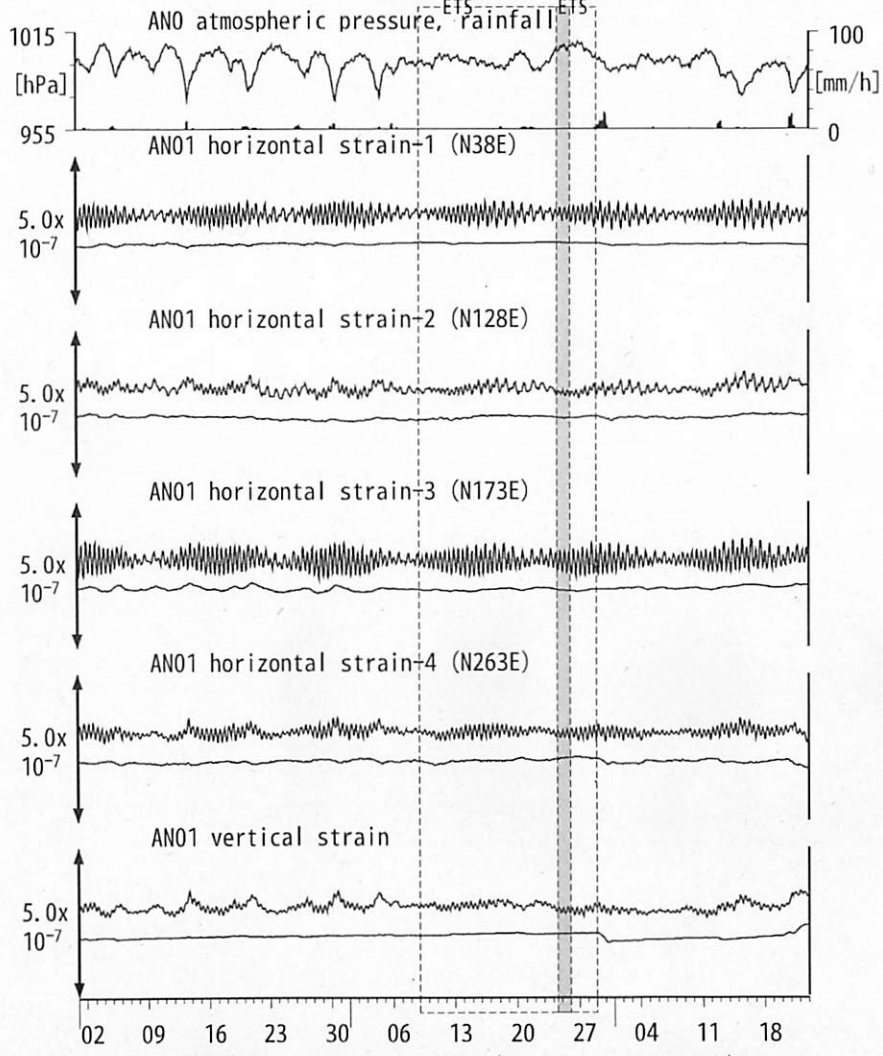
図9: Crustal strains changes at ANO 津安濃 (時間値) (2014/03/01 00:00 - 2014/05/23 00:00 (JST)) 愛知県中~東部 三重中
