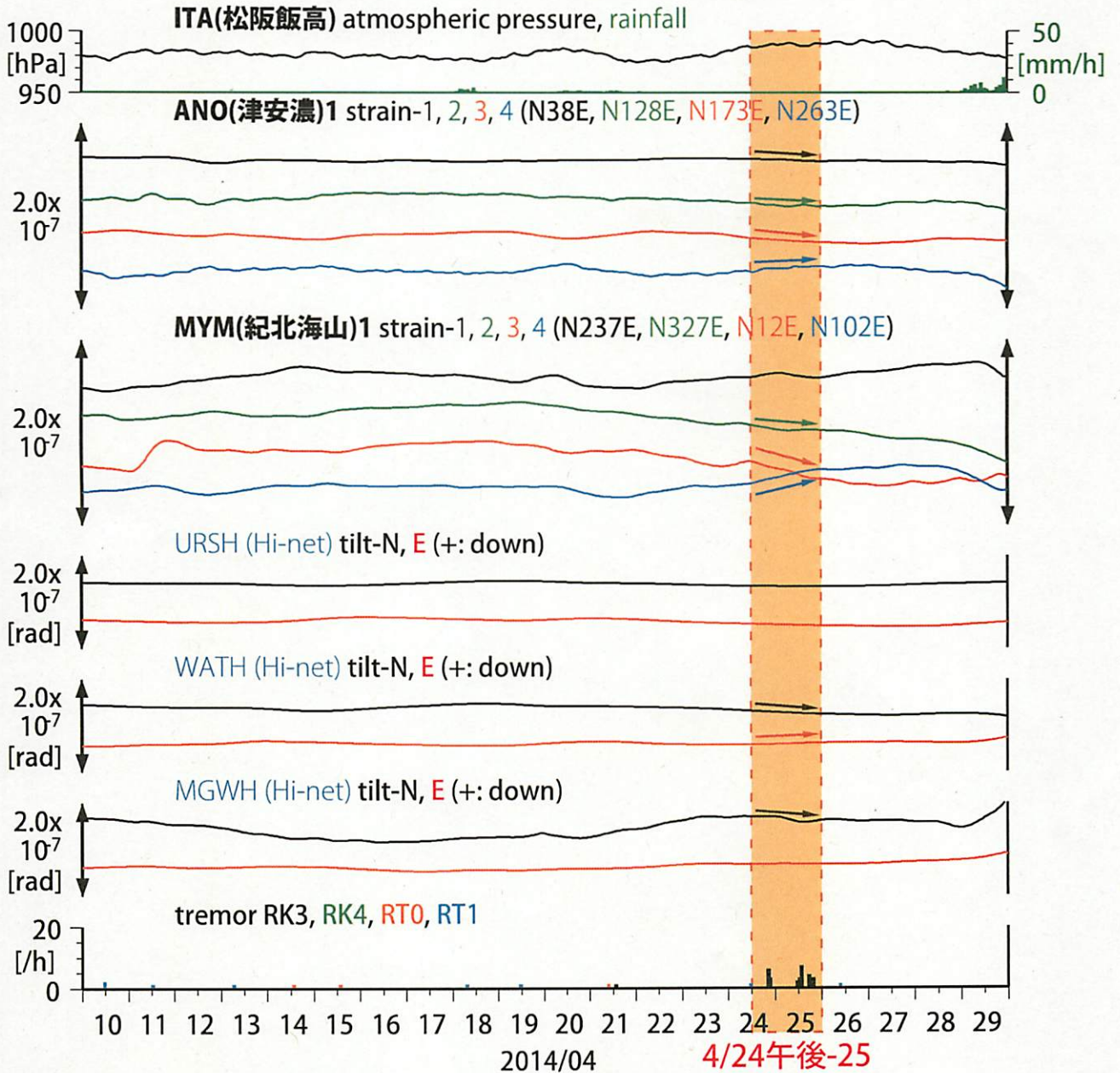
図31: 愛知県～三重県における歪観測結果 (時間値) (2014/04/10 00:00 - 2014/04/30 00:00 (JST))
