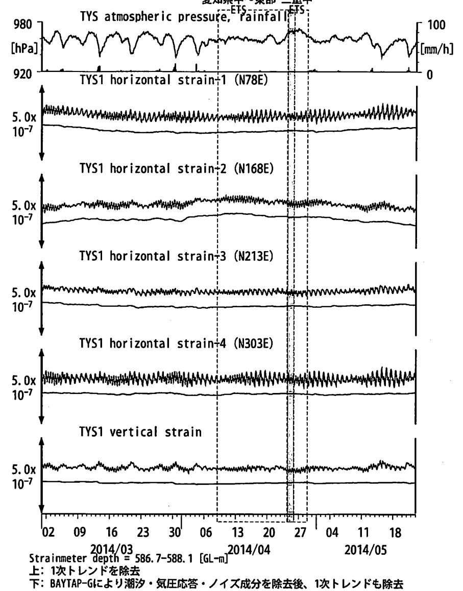
図2: Crustal strains changes at TYS 豊田神殿 (時間値) (2014/03/01 00:00 - 2014/05/23 00:00 (JST)) 愛知県中～東部 三重中
