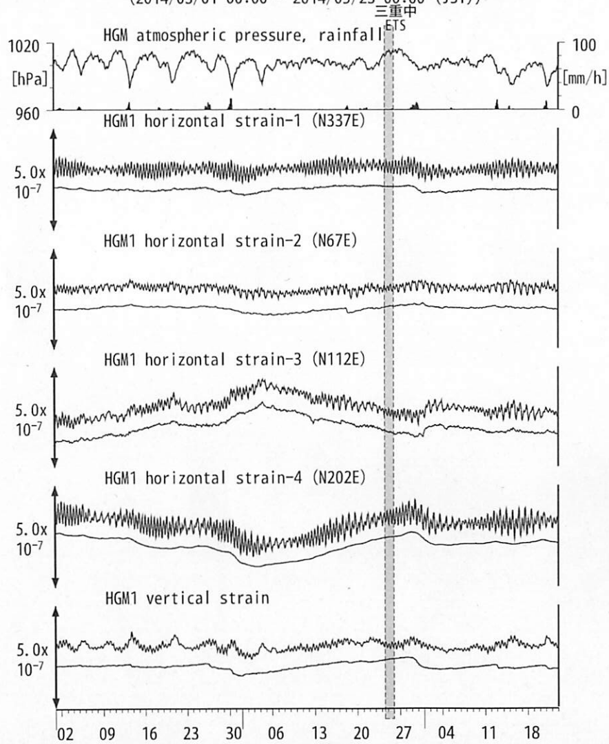
図17: Crustal strains changes at HGM 田辺本宮 (時間値) (2014/03/01 00:00 - 2014/05/23 00:00 (JST))
