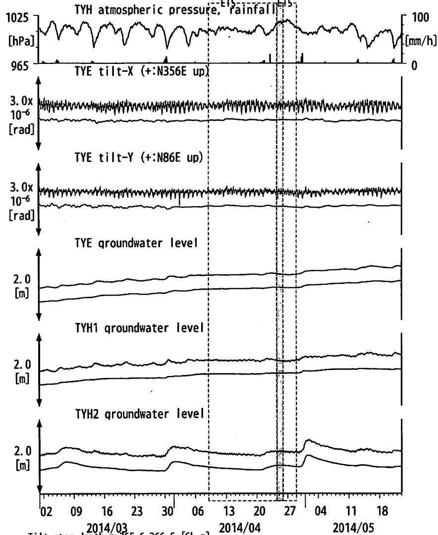
図7: Tilt and groundwater level changes at TYE and TYH 豊橋多米・豊橋 (2014/03/01 00:00 - 2014/05/23 00:00 (JST)) 愛知県中～東部 三重中
