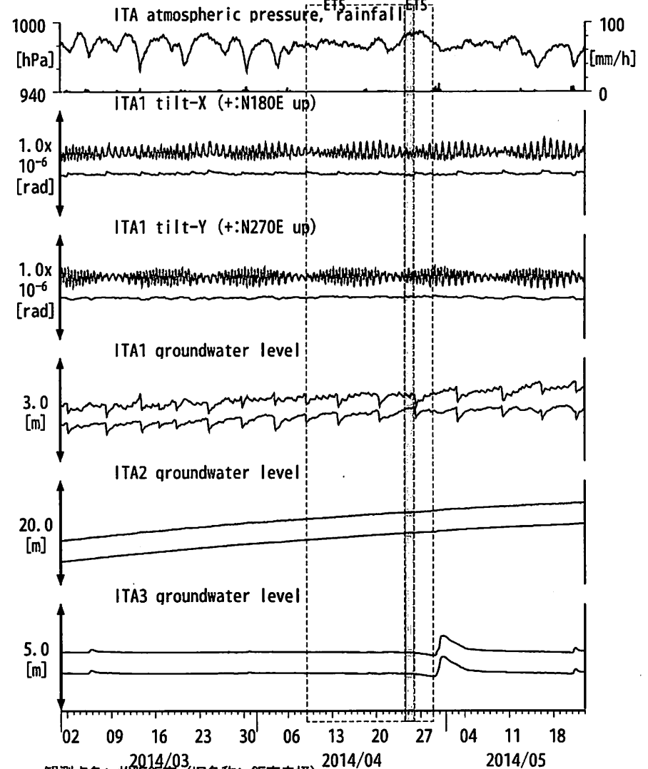
図12: Tilt and groundwater level changes at ITA 松阪飯高 (時間値) (2014/03/01 00:00 - 2014/05/23 00:00 (JST)) 愛知県中～東部 三重中
