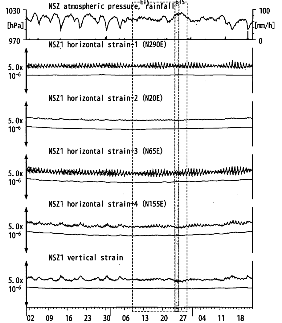
図4: Crustal strains changes at NSZ 西尾善明 (時間値) (2014/03/01 00:00 - 2014/05/23 00:00 (JST)) 愛知県中~東部 三重中
