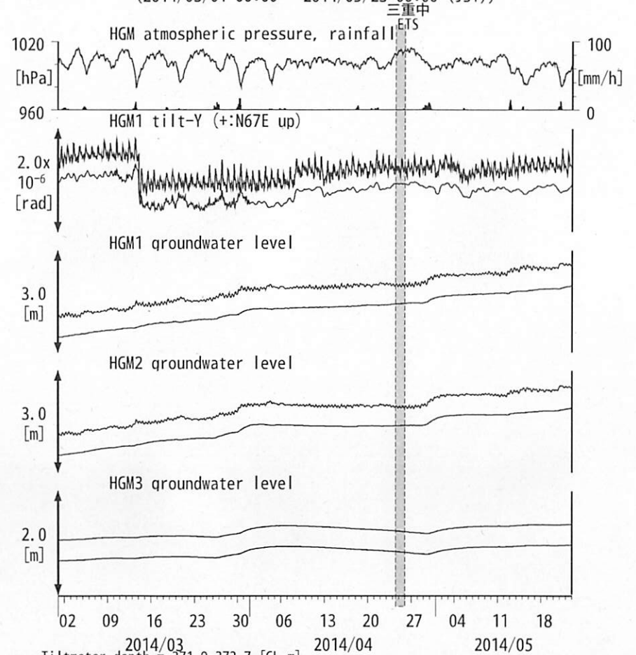
図18: Tilt and groundwater level changes at HGM 田辺本宮 (時間値) (2014/03/01 00:00 - 2014/05/23 00:00 (JST))
