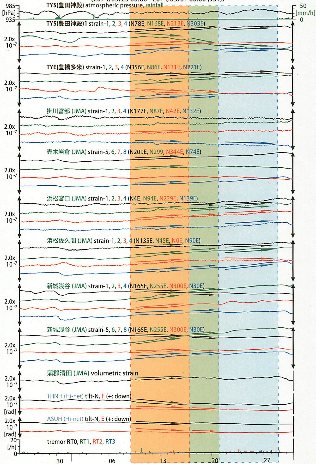
図25: 東海地方における歪・傾斜観測結果 (時間値) (2014/03/25 00:00 - 2014/05/01 00:00 (JST))
