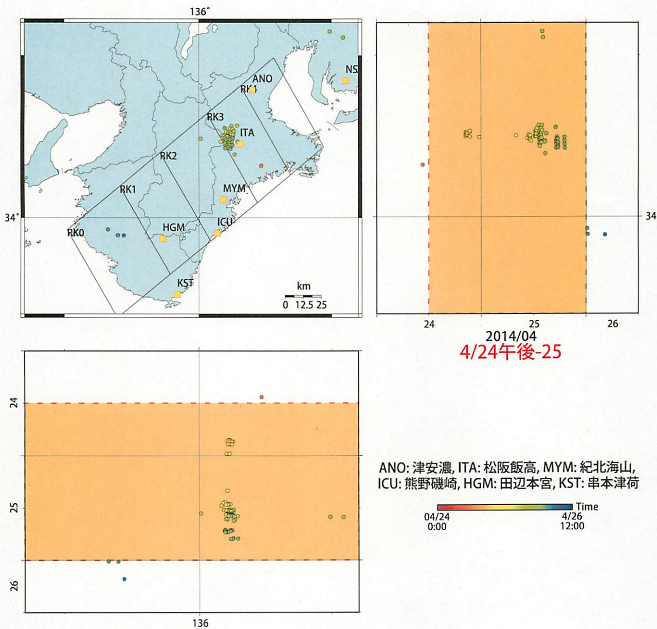
図30: 2014/4/24 0:00 - 4/26 12:00 における紀伊半島周辺の深部低周波微動の時空間分布図。エンベロープ相関法により決定。
