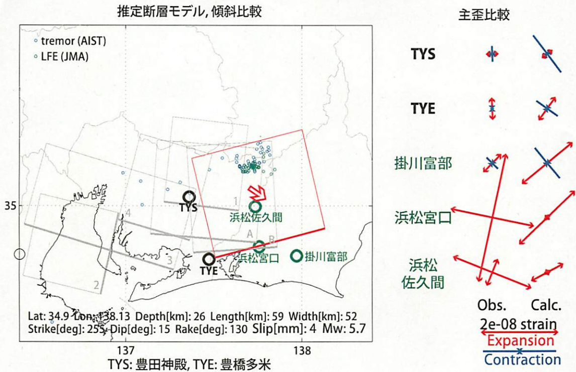
図29: 主な微動発生領域を含むように断層面を推定した結果(赤色矩形)。位置を微動域に限定して推定した。主歪の観測値とモデルからの計算値との比較を右側に示す。灰色の矩形は、最近周辺で発生した短期的SSEの推定断層面を示す。
