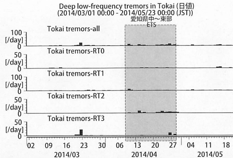
図 23: 愛知県およびその周辺における深部低周波微動の時空間分布 (上段)、各領域における発生頻度 (日値)。
