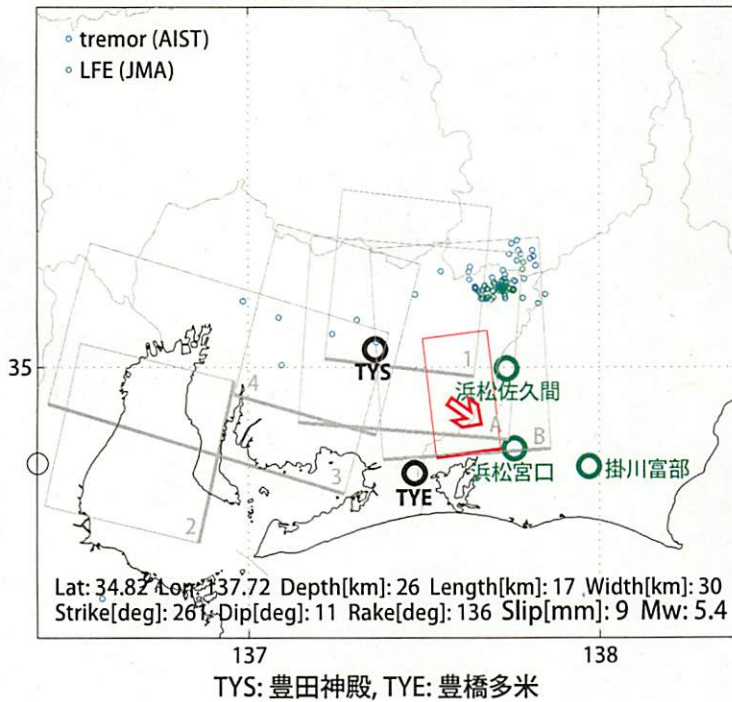
推定断層モデル、傾斜比較
