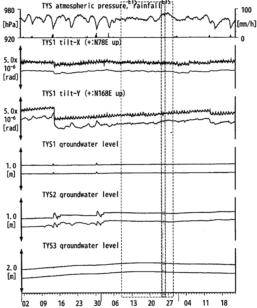
図3: Tilt and groundwater level changes at TYS 豊田神殿 (時間値) (2014/03/01 00:00 - 2014/05/23 00:00 (JST)) 愛知県中~東部 三重中
