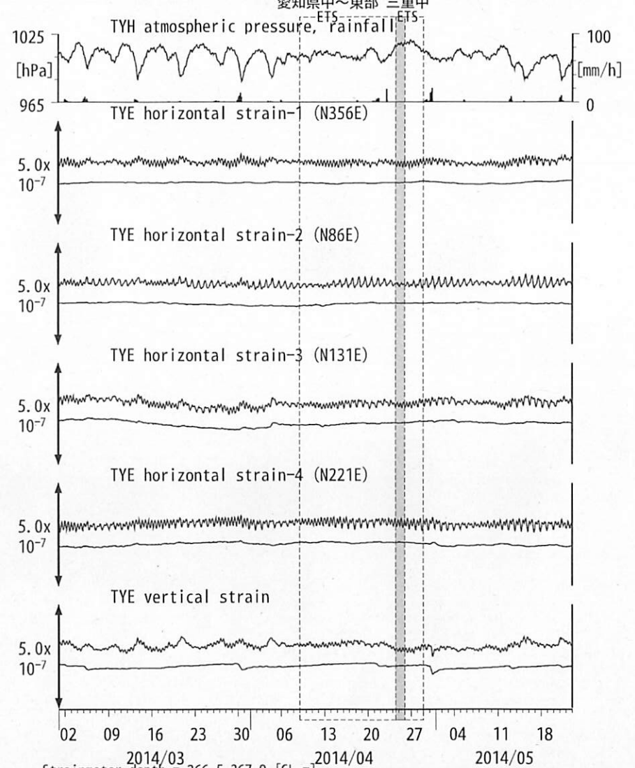
図6: Crustal strain changes at TYE 豊橋多米 (時間値) (2014/03/01 00:00 - 2014/05/23 00:00 (JST)) 愛知県中～東部 三重中
