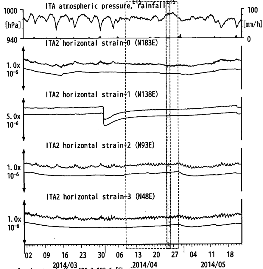
図11: Crustal strain changes at ITA 松阪飯高 (時間値) (2014/03/01 00:00 - 2014/05/23 00:00 (JST)) 愛知県中～東部 三重中
