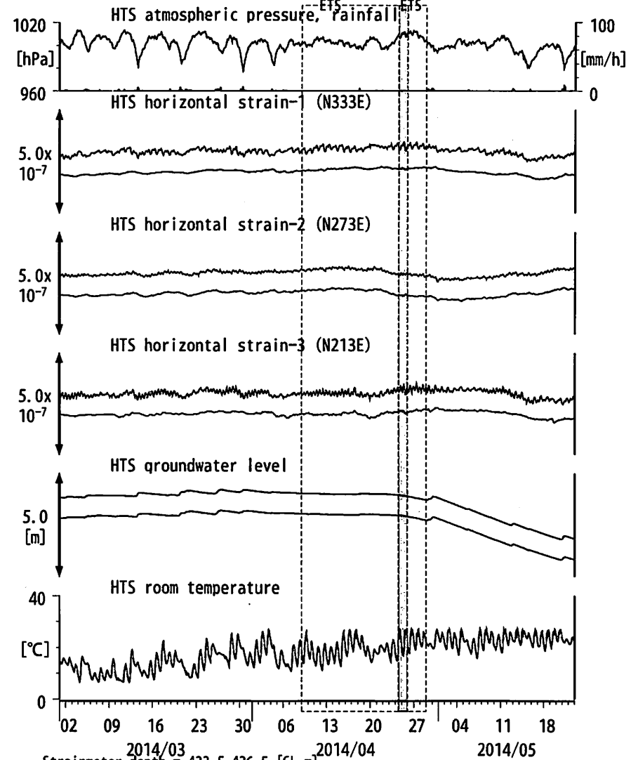
図8: Crustal strain and groundwater level changes at HTS 愛荘香之庄 (2014/03/01 00:00 - 2014/05/23 00:00 (JST)) 愛知県中～東部 三重中
