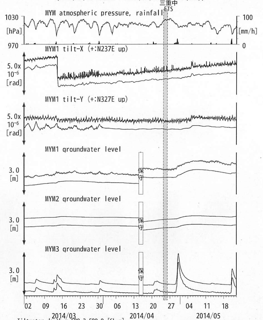
図14: Tilt and groundwater level changes at MYM 紀北海山 (時間値) (2014/03/01 00:00 - 2014/05/23 00:00 (JST))
