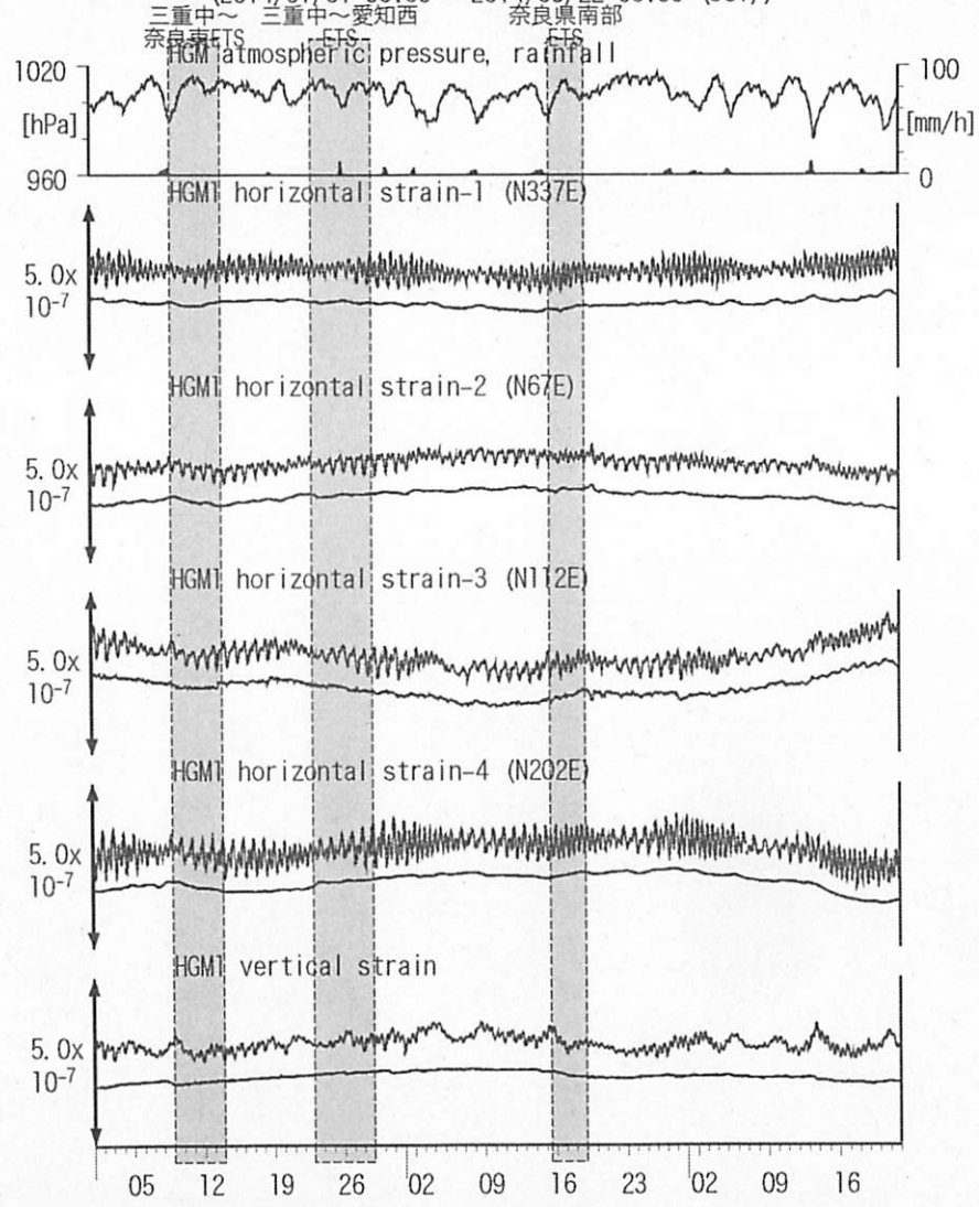
図17: Crustal strains changes at HGM 田辺本宮 (時間値) (2014/01/01 00:00 - 2014/03/22 00:00 (JST))
