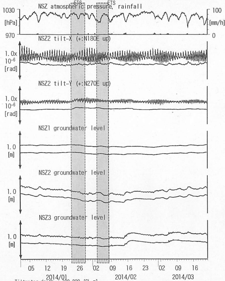
図5: Tilt and groundwater level changes at NSZ 西尾善明 (時間値) (2014/01/01 00:00 - 2014/03/22 00:00 (JST)) 三重中～愛知西 愛知県中部
