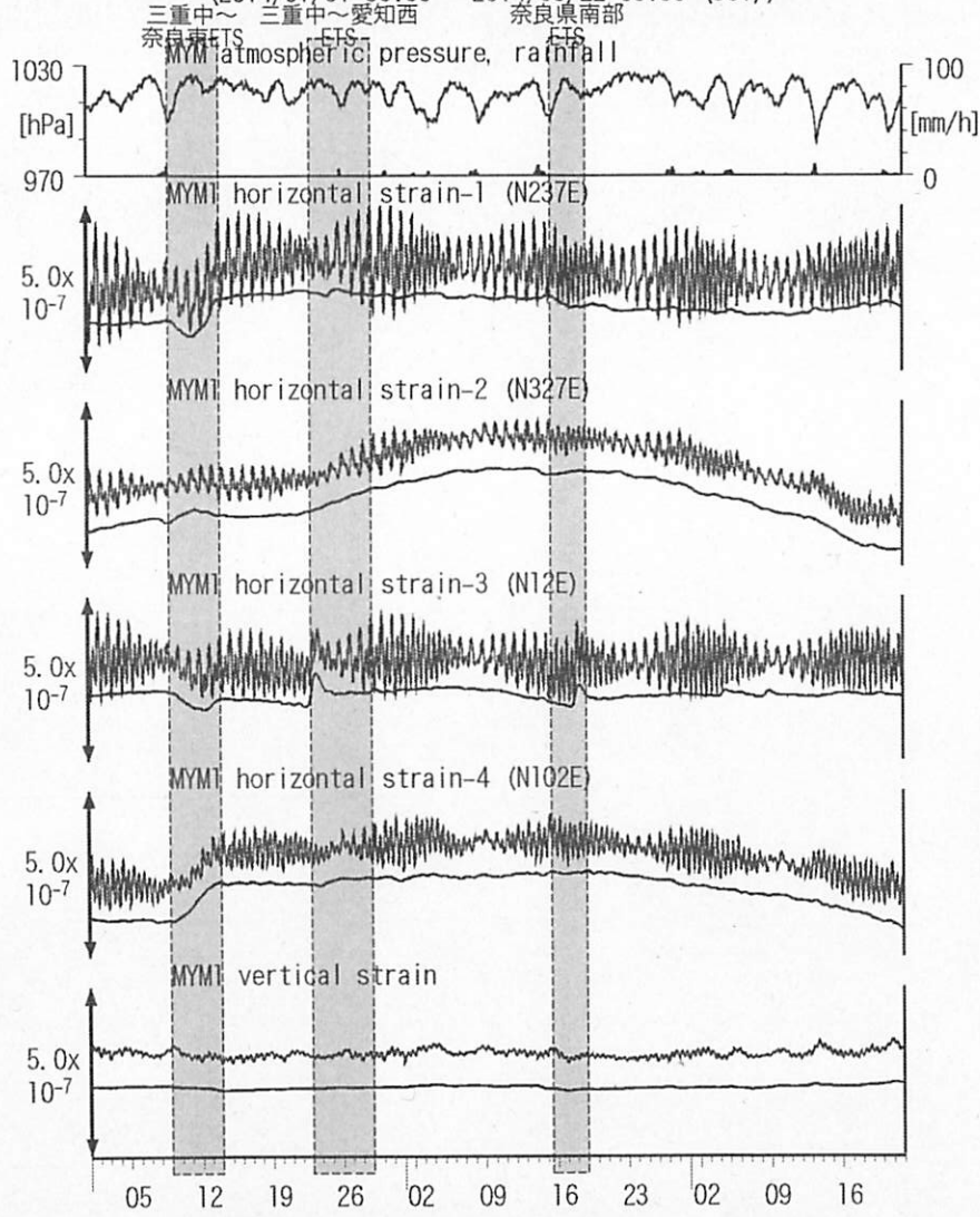
図13: Crustal strain changes at MYM 紀北海山 (時間値) (2014/01/01 00:00 - 2014/03/22 00:00 (JST))
