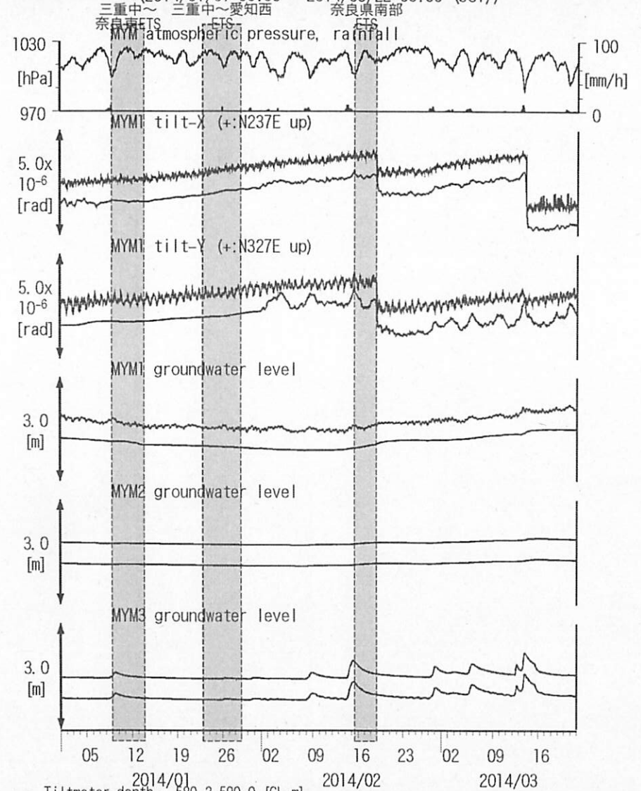
図14: Tilt and groundwater level changes at MYM 紀北海山 (時間値) (2014/01/01 00:00 - 2014/03/22 00:00 (JST))
