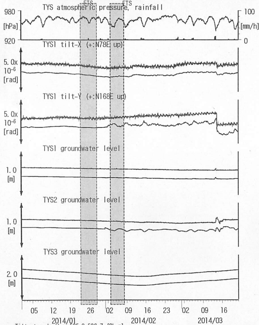
図3: Tilt and groundwater level changes at TYS 豊田神殿 (時間値) (2014/01/01 00:00 - 2014/03/22 00:00 (JST)) 三重中~愛知西 愛知県中部
