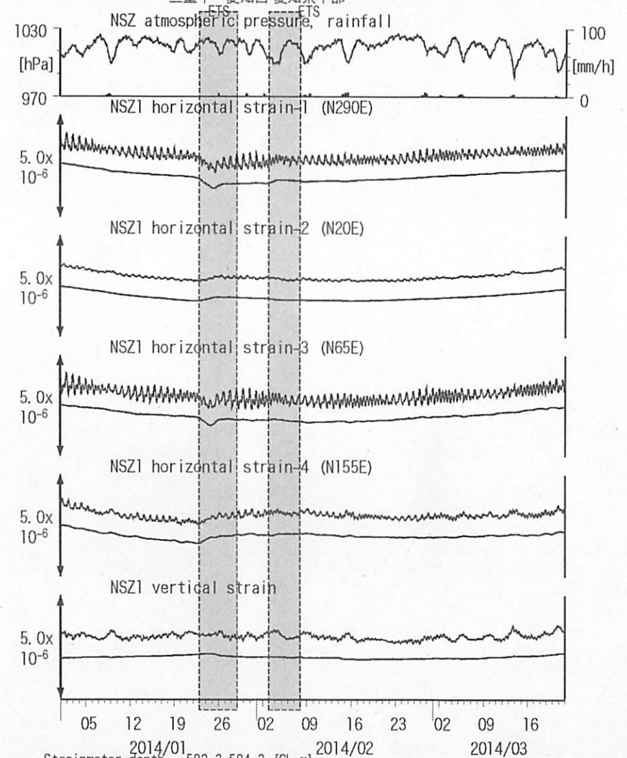
図4: Crustal strains changes at NSZ 西尾善明 (時間値) (2014/01/01 00:00 - 2014/03/22 00:00 (JST)) 三重中~愛知西 愛知県中部
