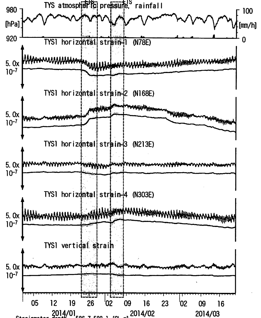
図2: Crustal strains changes at TYS 豊田神殿 (時間値) (2014/01/01 00:00 - 2014/03/22 00:00 (JST)) 三重中～愛知西 愛知県中部
