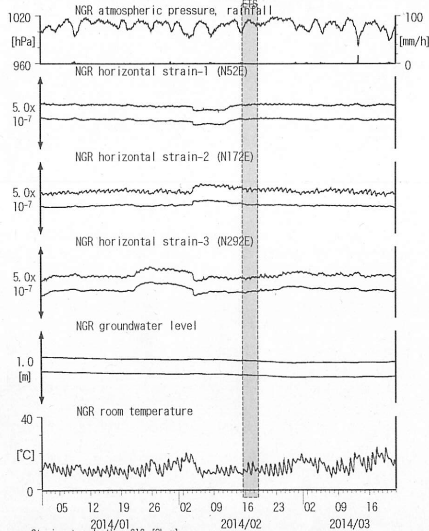
図21: Crustal strain and groundwater level changes at 岩出東坂本 (時間値) (2014/01/01 00:00 - 2014/03/22 00:00 (JST)) 奈良県南部
