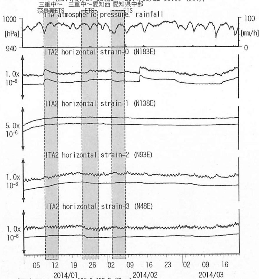
図11: Crustal strain changes at ITA 松阪飯高 (時間値) (2014/01/01 00:00 - 2014/03/22 00:00 (JST))
