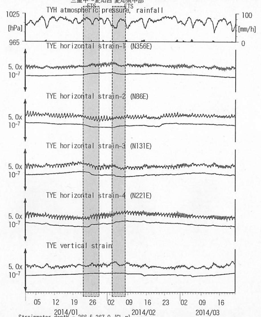
図6: Crustal strain changes at TYE 豊橋多米 (時間値) (2014/01/01 00:00 - 2014/03/22 00:00 (JST)) 三重中～愛知西 愛知県中部
