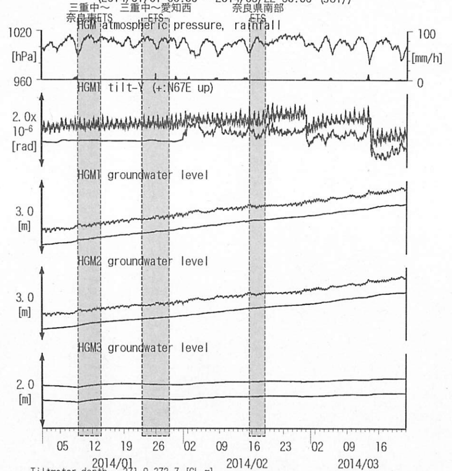
図18: Tilt and groundwater level changes at HGM 田辺本宮 (時間値) (2014/01/01 00:00 - 2014/03/22 00:00 (JST))
