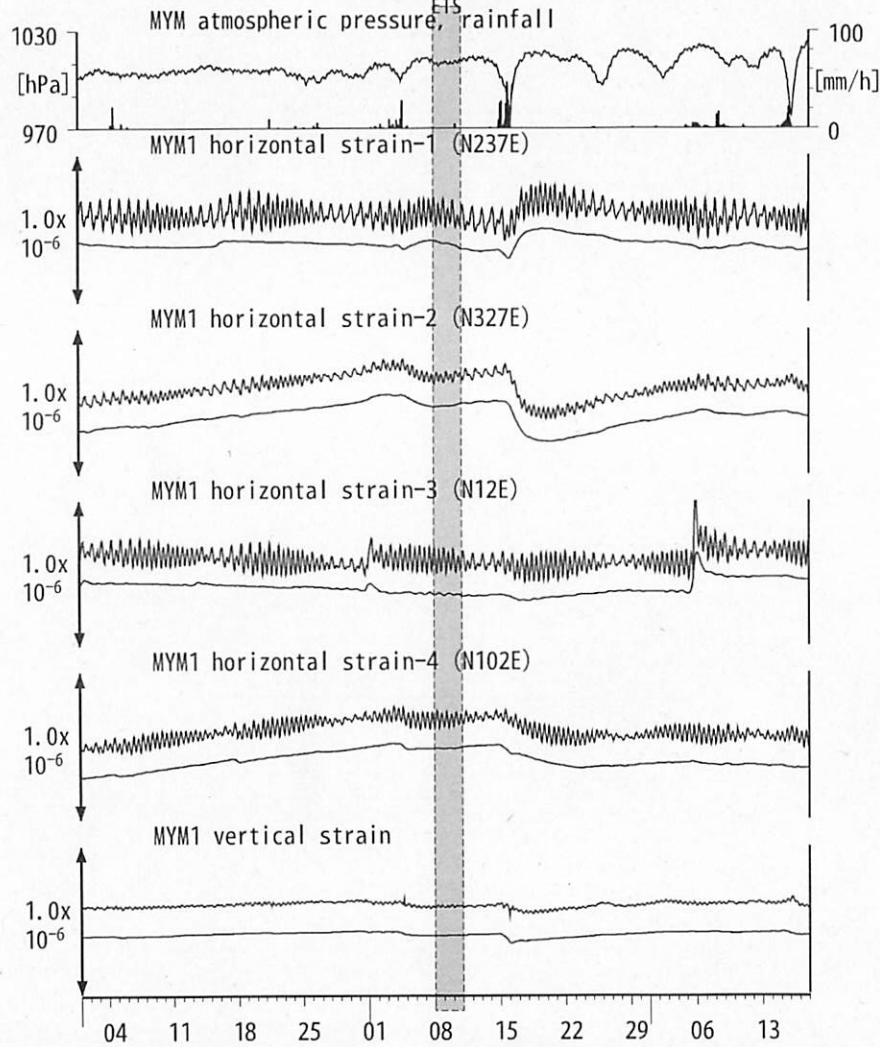
図11: Crustal strain changes at MYM 紀北海山 (時間値) (2013/08/01 00:00 - 2013/10/18 00:00 (JST)) 三重中~伊勢湾
