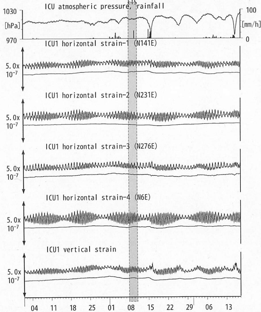
図13: Crustal strain changes at ICU 熊野磯崎 (時間値) (2013/08/01 00:00 - 2013/10/18 00:00 (JST)) 三重中~伊勢湾
