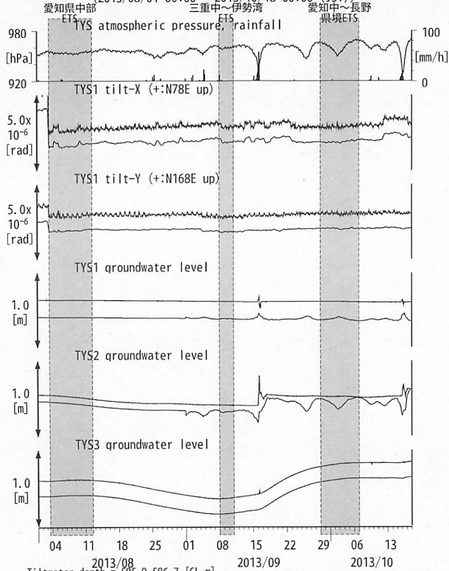
図3: Tilt and groundwater level changes at TYS 豊田神殿 (時間値) (2013/08/01 00:00 - 2013/10/18 00:00 (JST))
