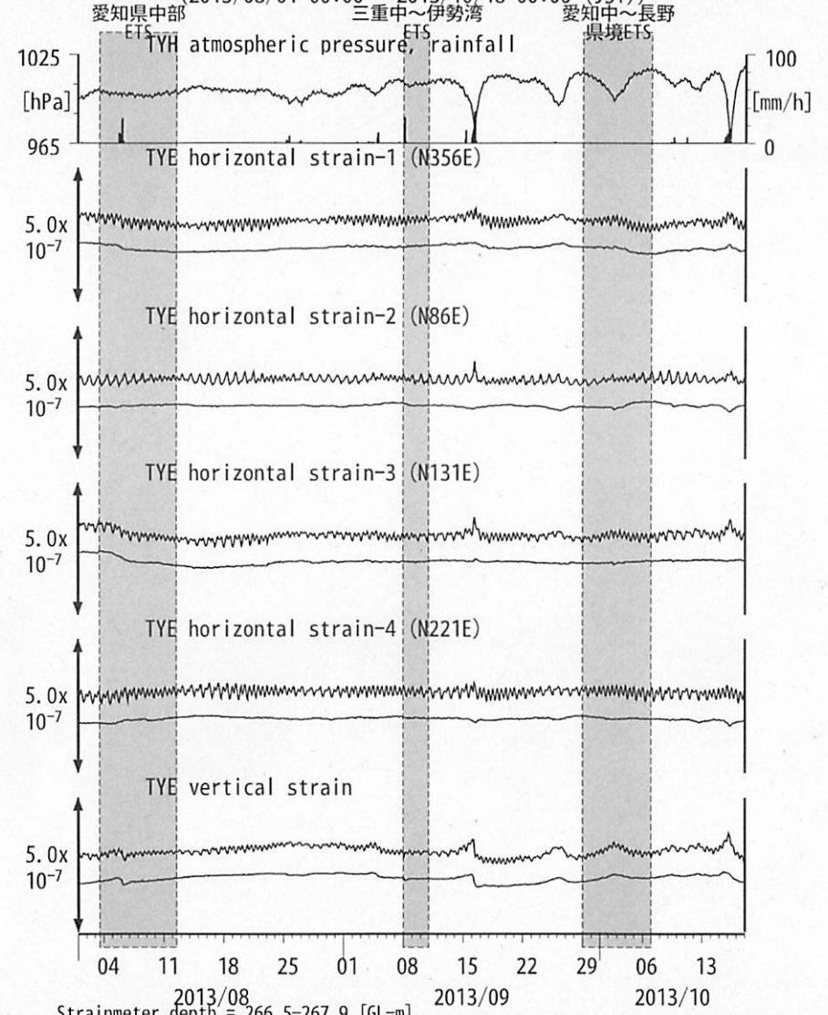
図4: Crustal strain changes at TYE 豊橋多米 (時間値) (2013/08/01 00:00 - 2013/10/18 00:00 (JST))
