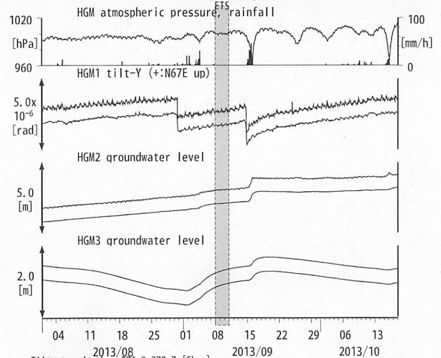
図16: Tilt and groundwater level changes at HGM 田辺本宮 (時間値) (2013/08/01 00:00 - 2013/10/18 00:00 (JST)) 三重中~伊勢湾
