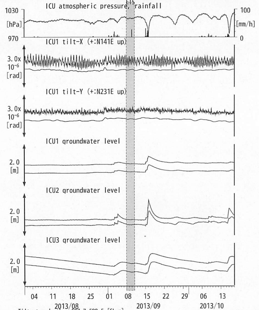
図14: Tilt and groundwater level changes at ICU 熊野磯崎 (時間値) (2013/08/01 00:00 - 2013/10/18 00:00 (JST)) 三重中~伊勢湾
