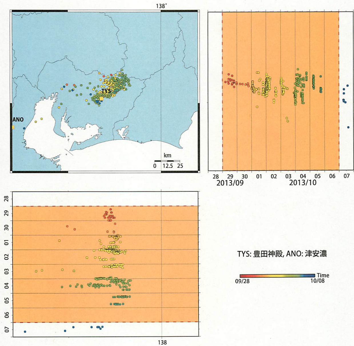
図22: 2013/9/28 0:00 - 10/8 0:00 における愛知県周辺の深部低周波微動の時空間分布図。エンベロープ相関法により決定。
