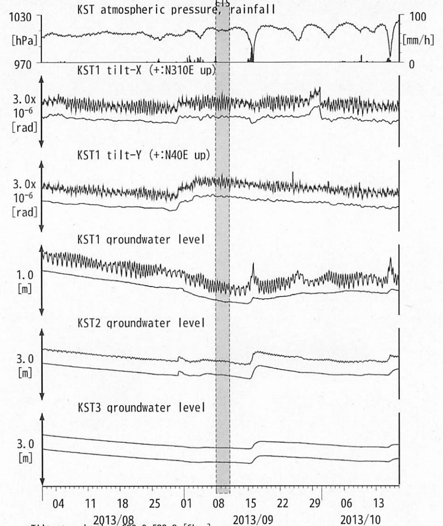
図18: Tilt and groundwater level changes at KST 串本津荷 (時間値) (2013/08/01 00:00 - 2013/10/18 00:00 (JST)) 三重中~伊勢湾
