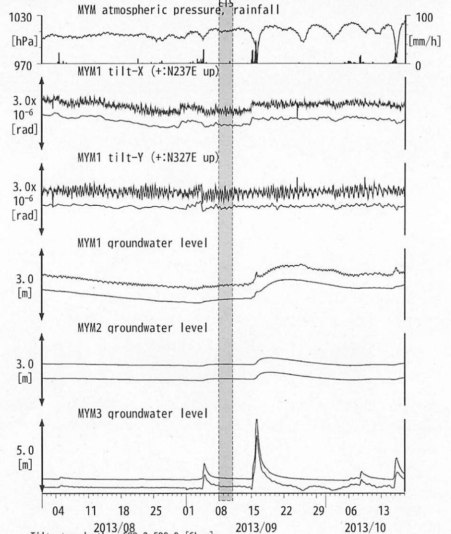
図12: Tilt and groundwater level changes at MYM 紀北海山 (時間値) (2013/08/01 00:00 - 2013/10/18 00:00 (JST)) 三重中~伊勢湾
