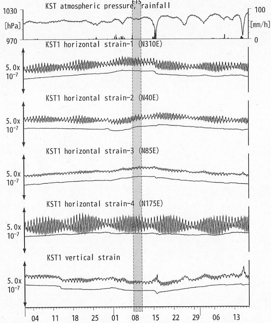
図17: Crustal strain changes at KST 串本津荷 (時間値) (2013/08/01 00:00 - 2013/10/18 00:00 (JST)) 三重中~伊勢湾
