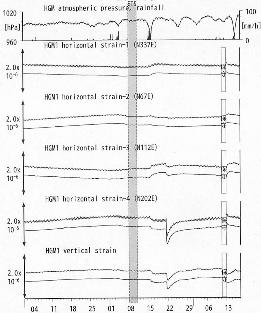
図15: Crustal strains changes at HGM 田辺本宮 (時間値) (2013/08/01 00:00 - 2013/10/18 00:00 (JST)) 三重中~伊勢湾
