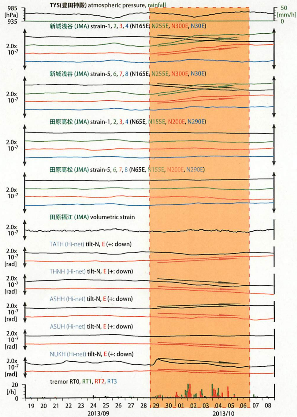
歪・傾斜は直線トレンド、潮汐・気圧応答・ノイズ成分除去 (BAYTAP-G)
