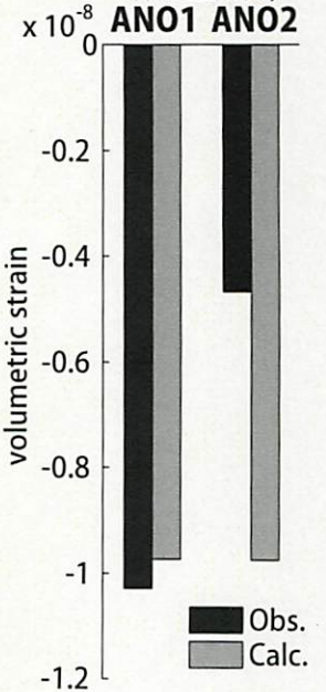
体積歪比較 (地下水圧→体積歪換算)
