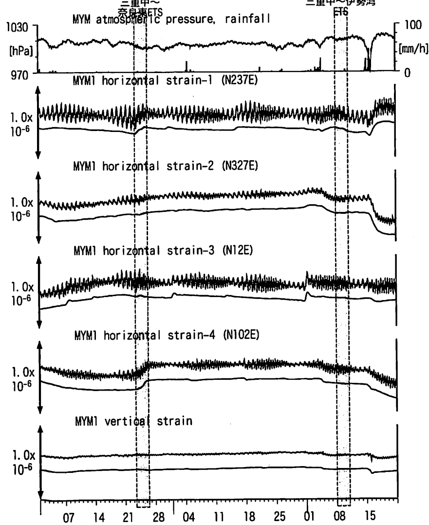
図11: Crustal strain changes at MYM 紀北海山 (時間値) (2013/07/01 00:00 - 2013/09/22 00:00 (JST))
