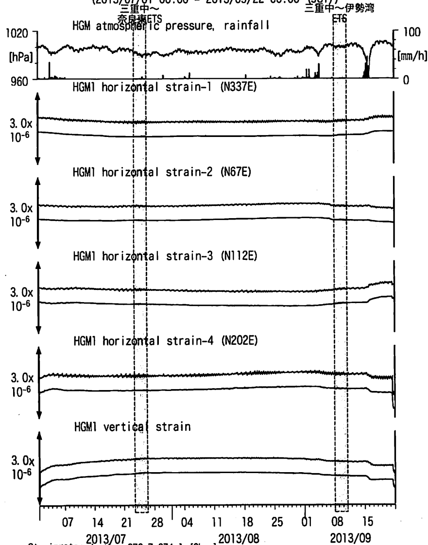
図15: Crustal strains changes at HGM 田辺本宮 (時間値) (2013/07/01 00:00 - 2013/09/22 00:00 (JST))
