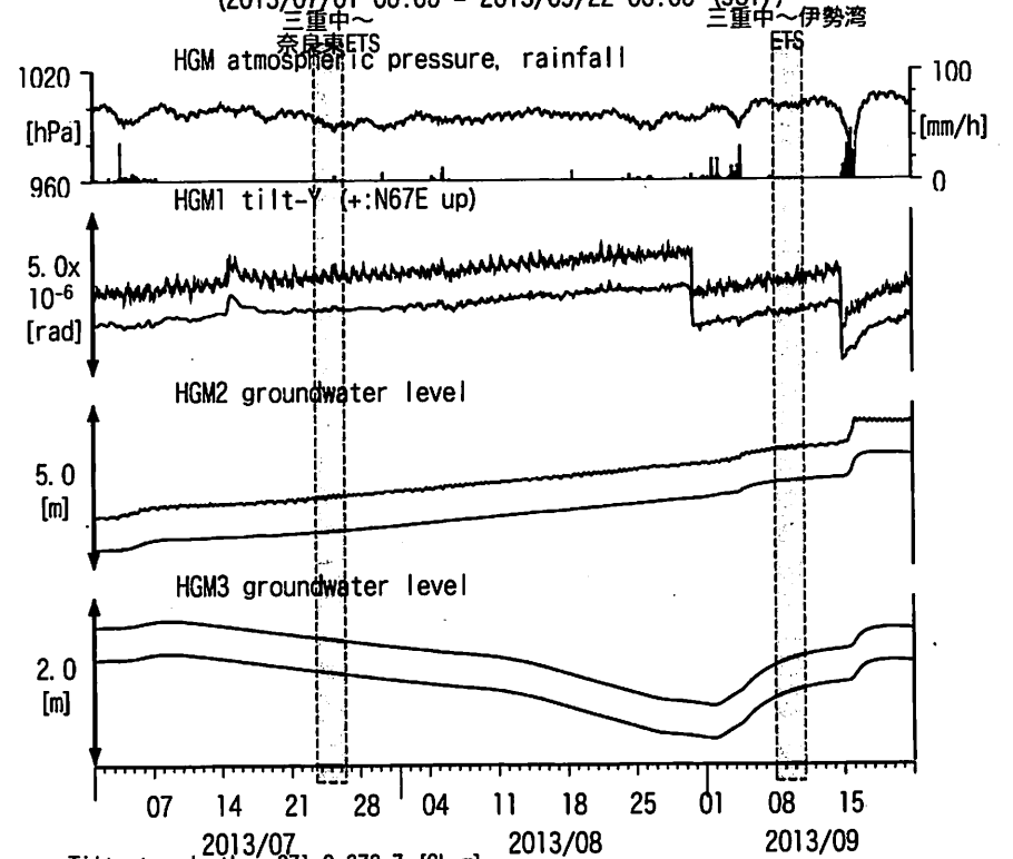
図16: Tilt and groundwater level changes at HGM 田辺本宮 (時間値) (2013/07/01 00:00 - 2013/09/22 00:00 (JST))
