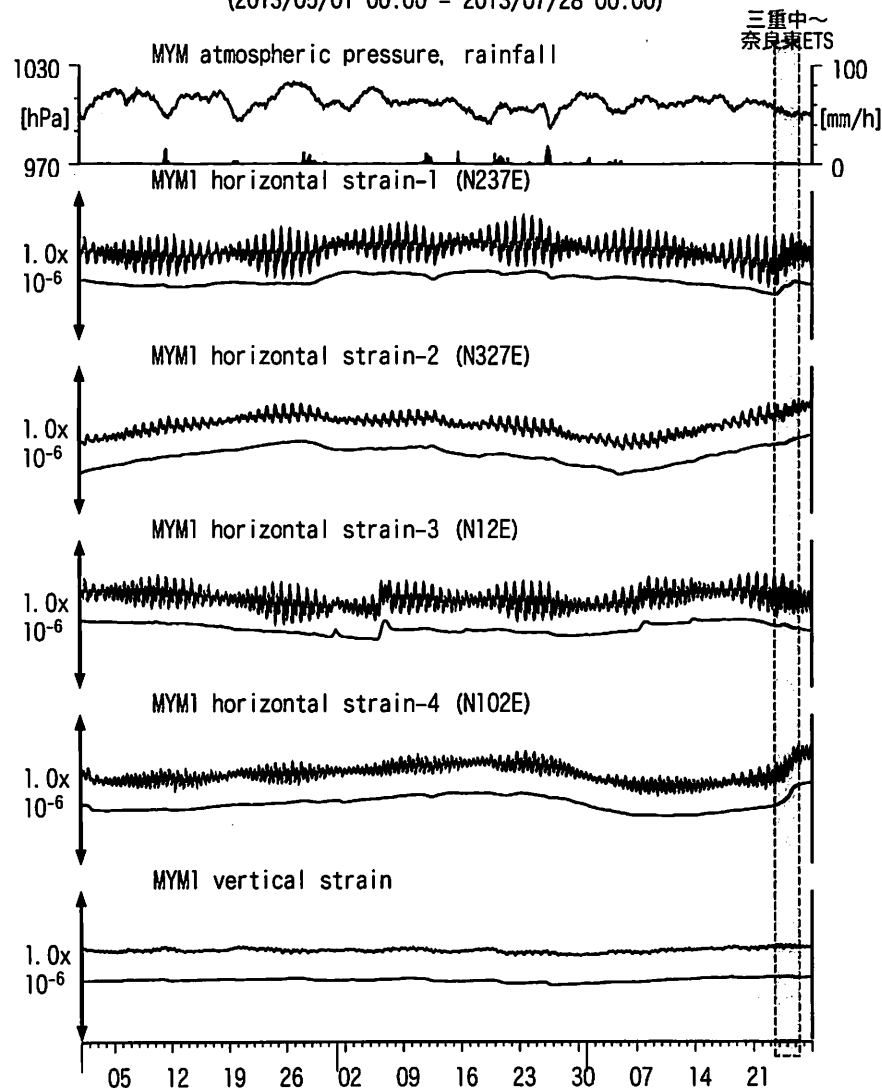
図11: Crustal strain changes at MYM 紀北海山 (時間値) (2013/05/01 00:00 - 2013/07/28 00:00)
