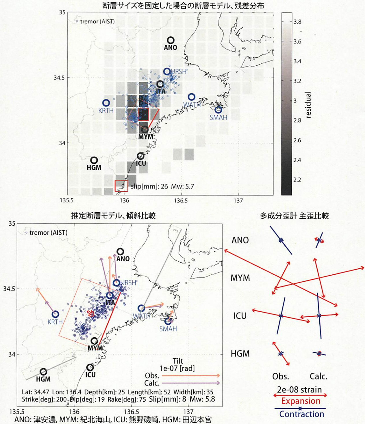
図29: (上段)プレート境界面上のパッチ(断層面)をすべらせた際の、歪・傾斜の観測値と計算値の残差分布図。断層面サイズは固定(20x20km)。赤色矩形は最小残差の断層面を表す。このパッチのすべり量、Mwを下部に示している。
