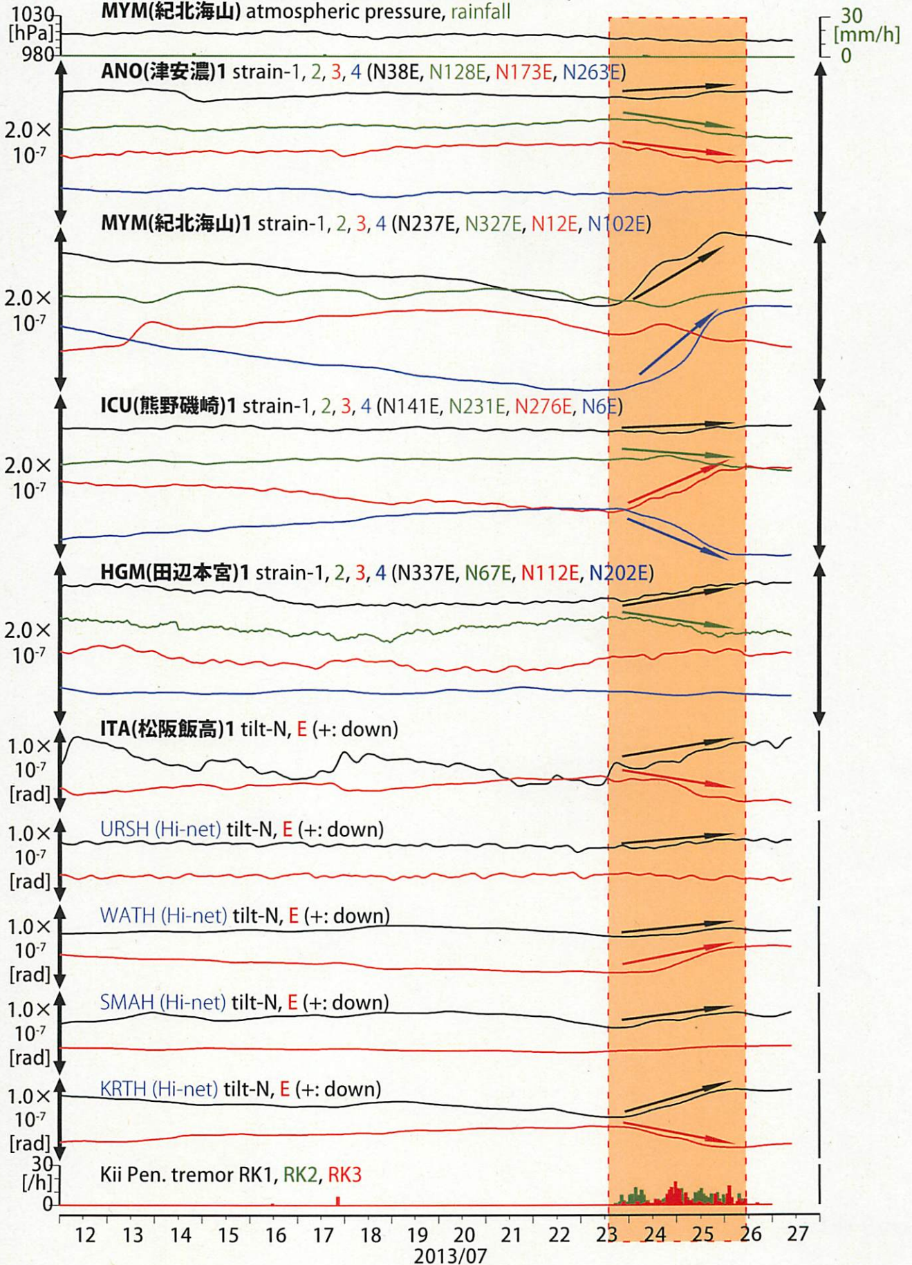
図28: 紀伊半島における歪・傾斜観測結果 (2013/07/12 00:00 - 2013/07/27 10:00)
