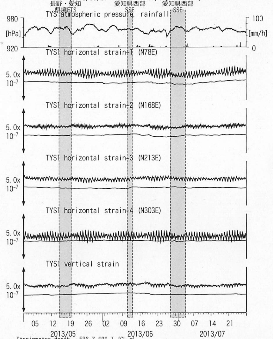
図2: Crustal strains changes at TYS 豊田神殿 (時間値) (2013/05/01 00:00 - 2013/07/28 00:00)
