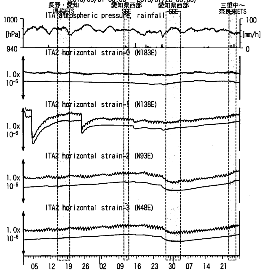
図9: Crustal strain changes at ITA 松阪飯高 (時間値) (2013/05/01 00:00 - 2013/07/28 00:00)
