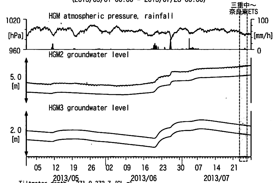
図16: Groundwater level changes at HGM 田辺本宮 (時間値) (2013/05/01 00:00 - 2013/07/28 00:00)
