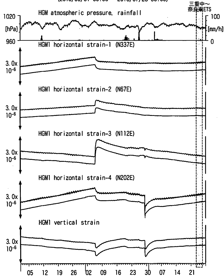
図15: Crustal strains changes at HGM 田辺本宮 (時間値) (2013/05/01 00:00 - 2013/07/28 00:00)
