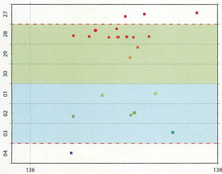
図22: 2013/6/27 0:00 - 7/5 0:00 における愛知県～三重県の深部低周波微動の時空間分布図。エンベロープ相関法により決定。
