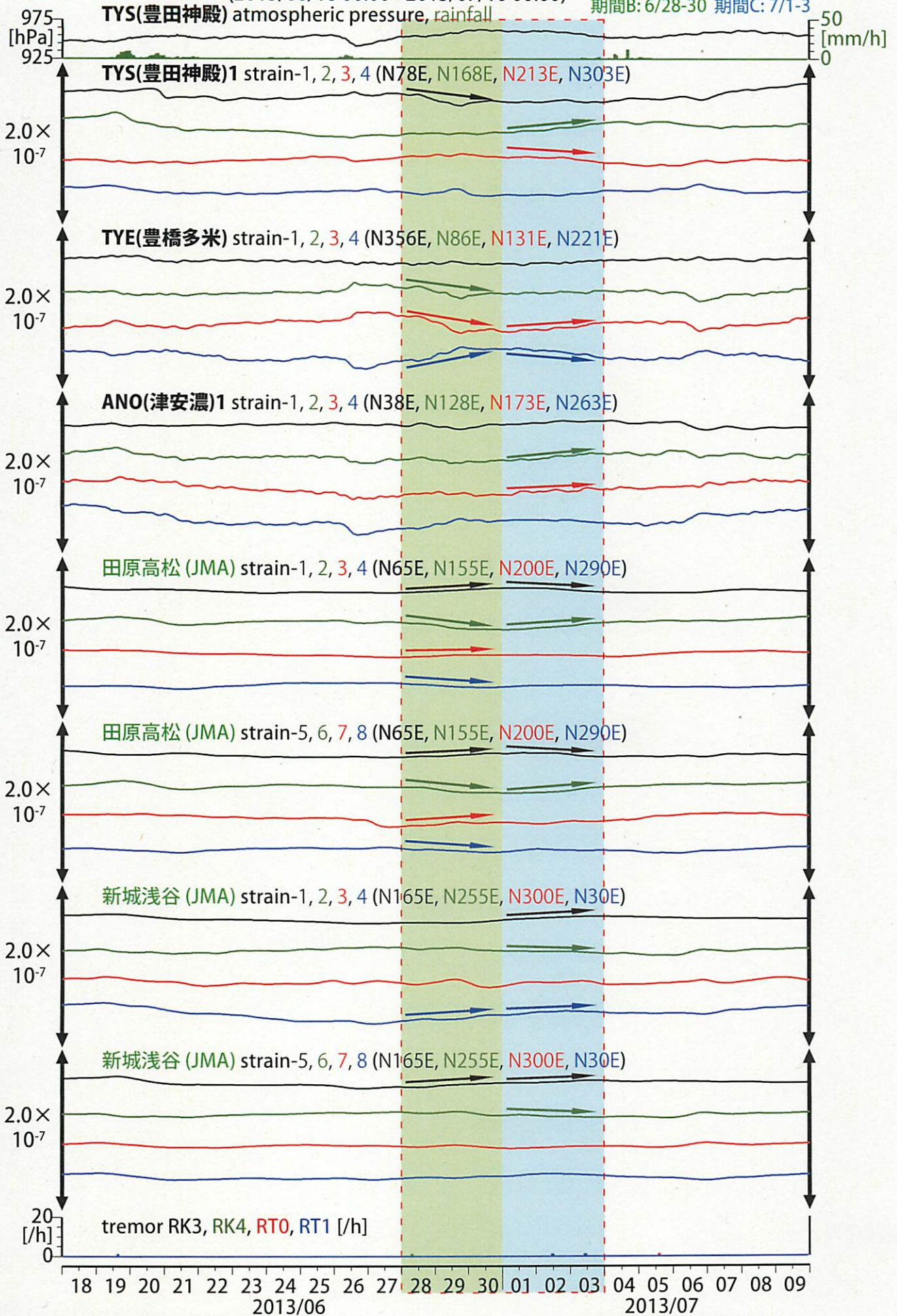
図23: 愛知県～三重県における歪観測結果 (時間値)
