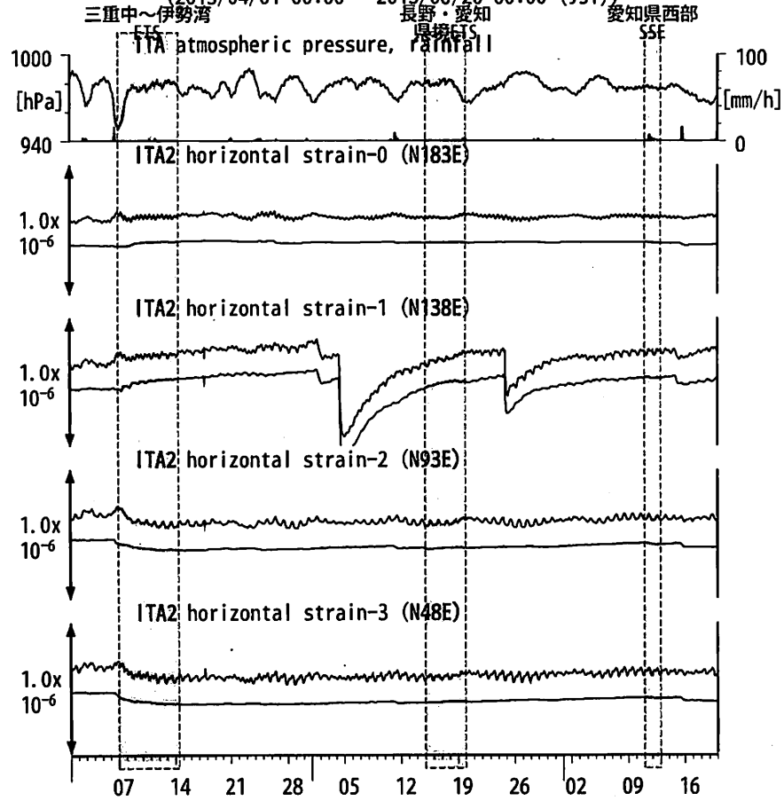
図9: Crustal strain changes at ITA 松阪飯高 (時間値) (2013/04/01 00:00 - 2013/06/20 00:00 (JST))
