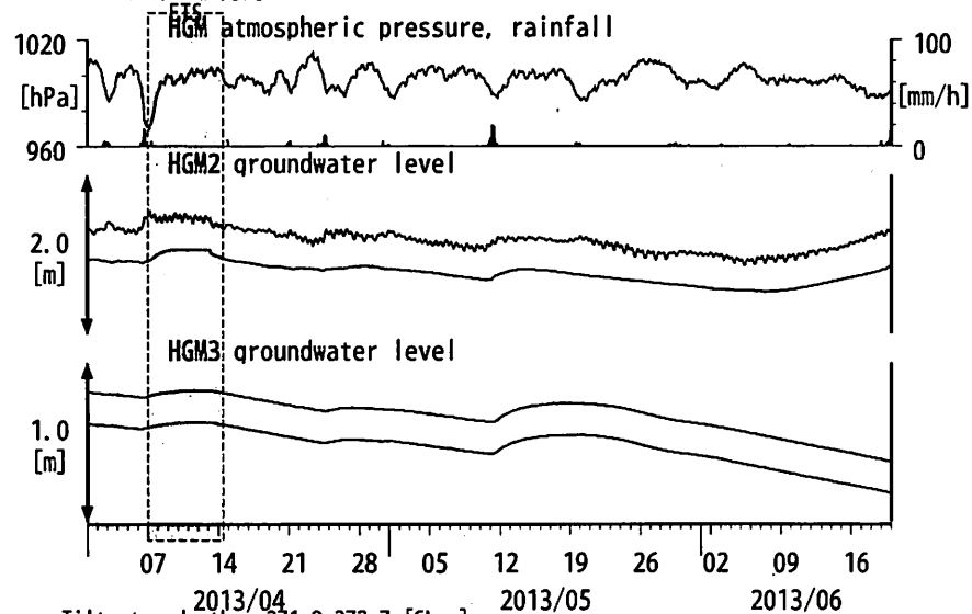
図16: Tilt and groundwater level changes at HGM 田辺本宮 (時間値) (2013/04/01 00:00 - 2013/06/20 00:00 (JST))
