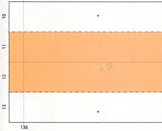
図22: 2013/6/10 0:00 - 6/14 0:00 における愛知県～三重県の深部低周波微動の時空間分布図。 エンベロープ相関法により決定。
