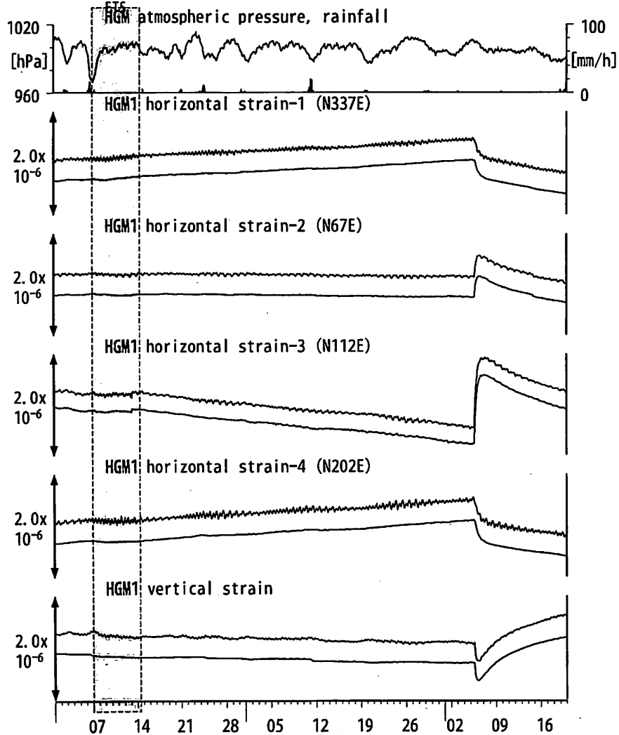
図15: Crustal strains changes at HGM 田辺本宮 (時間値) (2013/04/01 00:00 - 2013/06/20 00:00 (JST))
