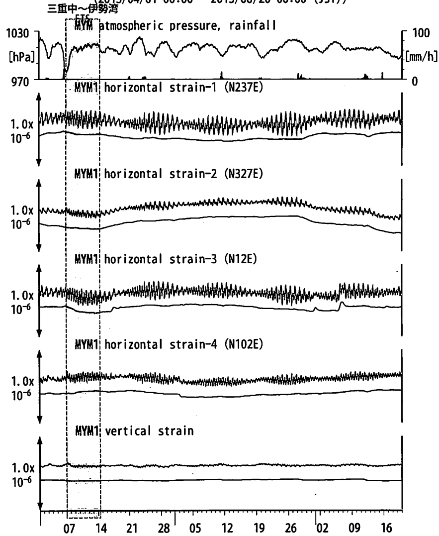
図11: Crustal strain changes at MYM 紀北海山 (時間値) (2013/04/01 00:00 - 2013/06/20 00:00 (JST))
