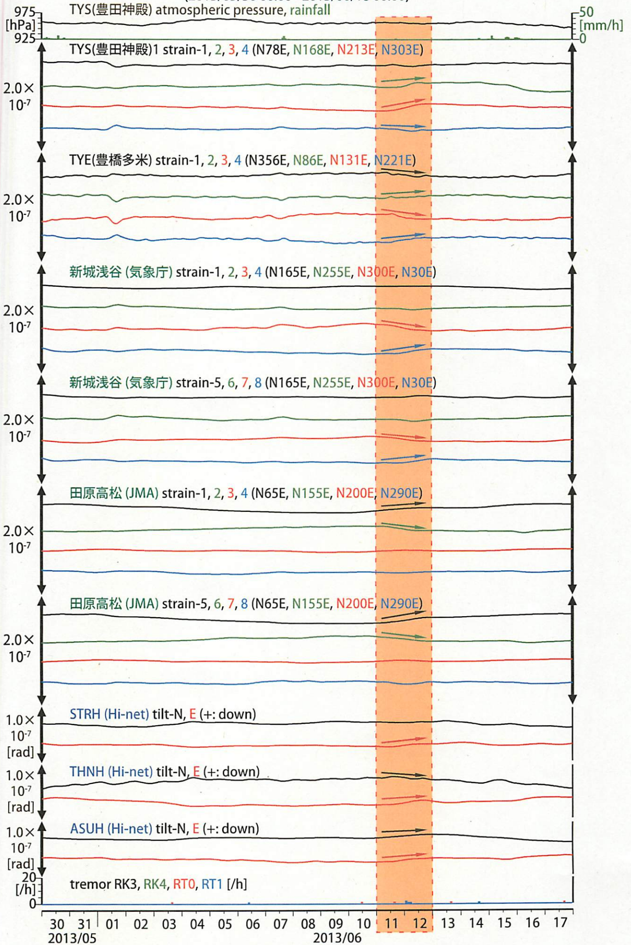
図23: 愛知県～三重県における歪観測結果 (時間値) (2013/05/30 00:00 - 2013/06/18 00:00)
