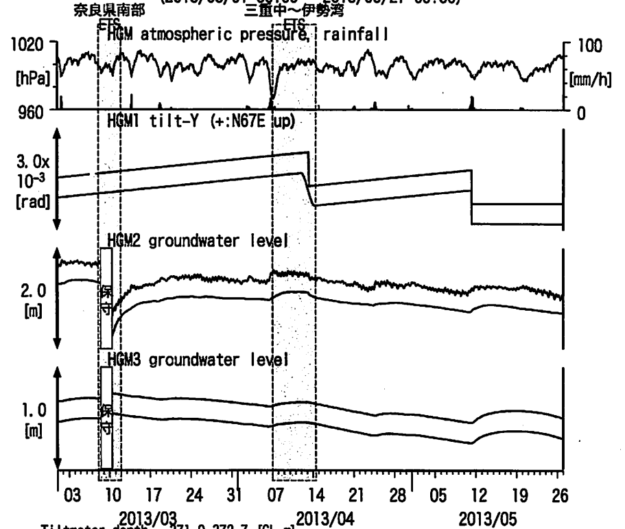
図16: Tilt and groundwater level changes at HGM 田辺本宮 (時間値) (2013/03/01 00:00 - 2013/05/27 00:00)
