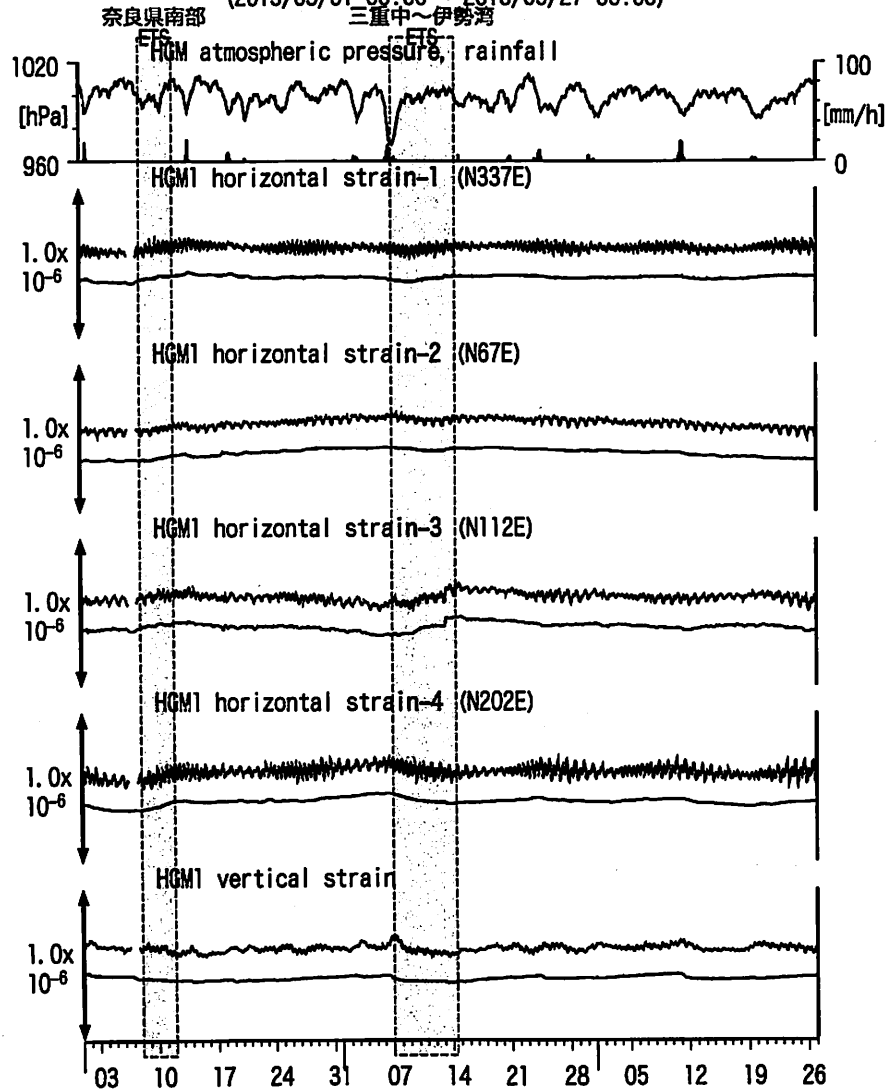
図15: Crustal strains changes at HGM 田辺本宮 (時間値) (2013/03/01 00:00 - 2013/05/27 00:00)
