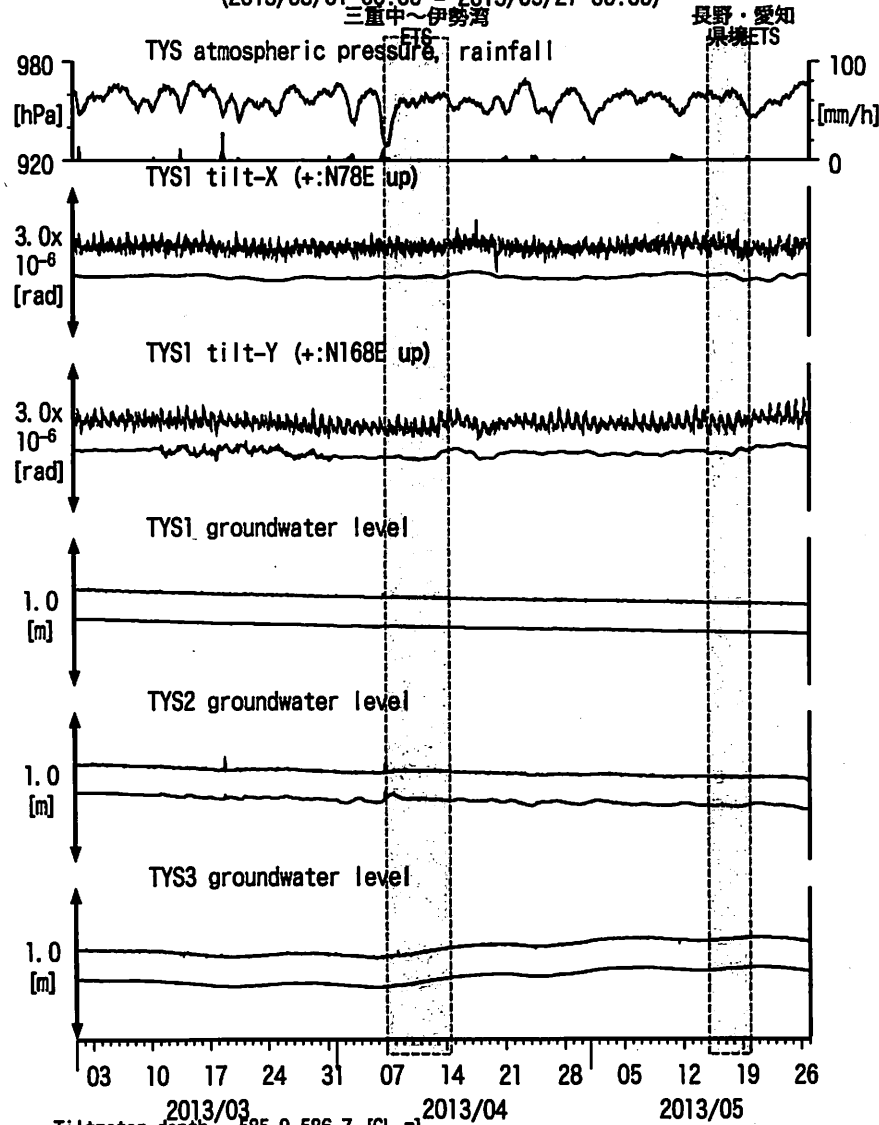
図3: Tilt and groundwater level changes at TYS 豊田神殿 (時間値) (2013/03/01 00:00 - 2013/05/27 00:00)
