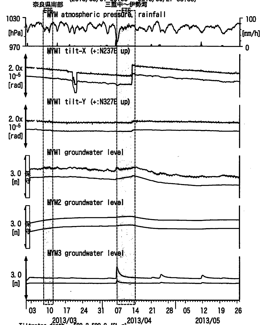
図12: Tilt and groundwater level changes at MYM 紀北海山 (時間値) (2013/03/01 00:00 - 2013/05/27 00:00)
