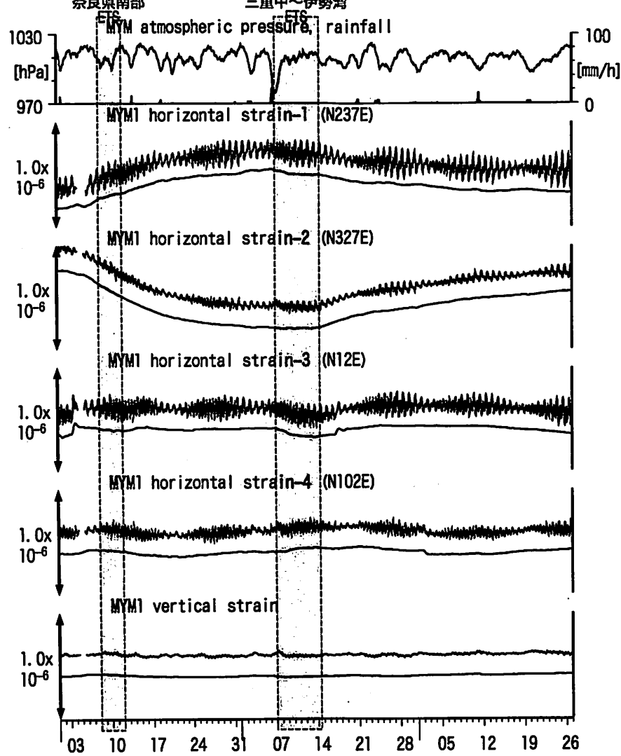
図11: Crustal strain changes at MYM 紀北海山 (時間値) (2013/03/01 00:00 - 2013/05/27 00:00)
