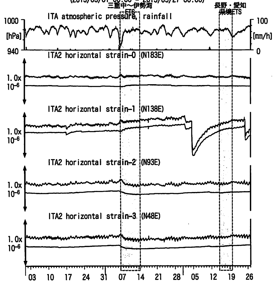
図9: Crustal strain changes at ITA 松阪飯高 (時間値) (2013/03/01 00:00 - 2013/05/27 00:00)
