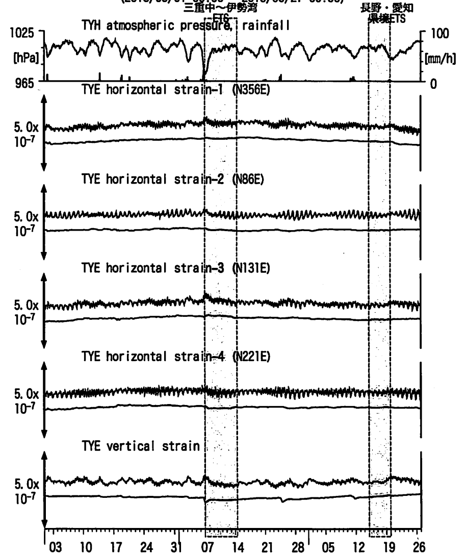
図4: Crustal strain changes at TYE 豊橋多米 (時間値) (2013/03/01 00:00 - 2013/05/27 00:00)
