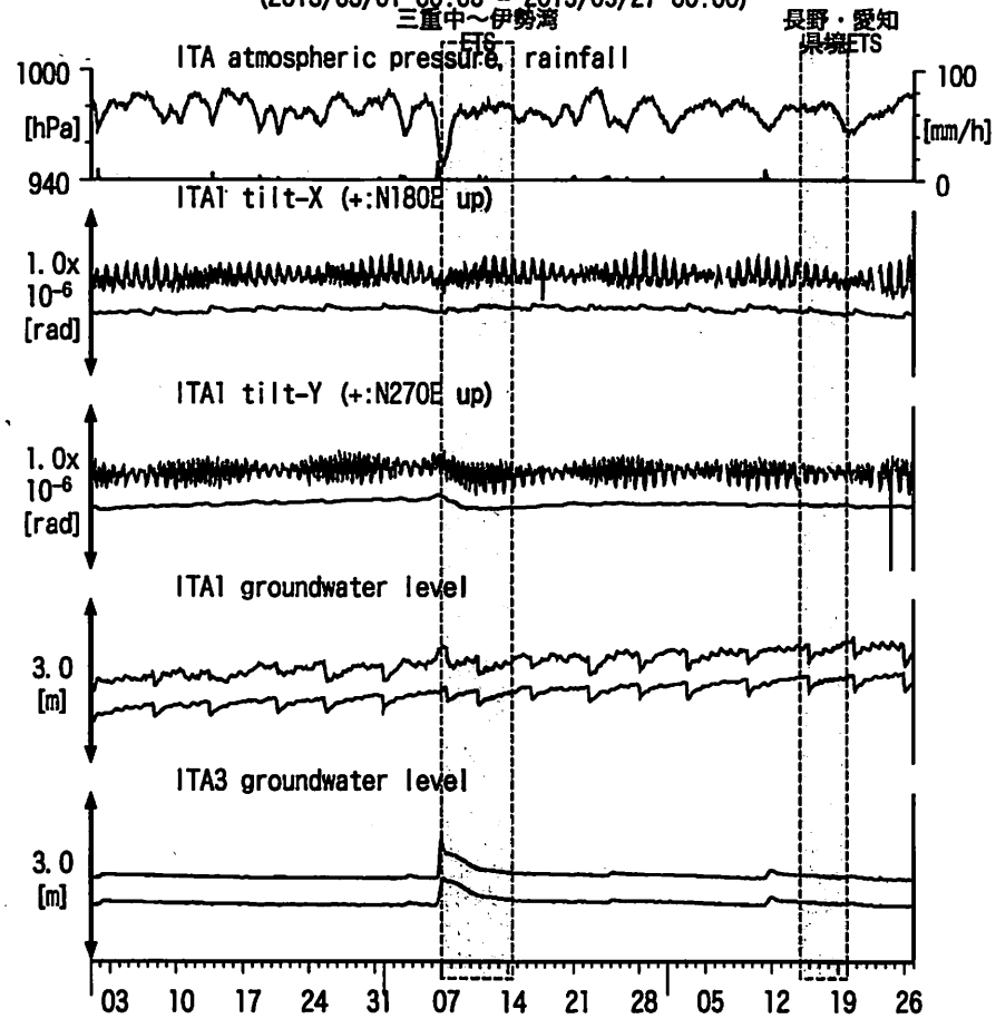
図10: Tilt and groundwater level changes at ITA 松阪飯高 (時間値) (2013/03/01 00:00 - 2013/05/27 00:00)
