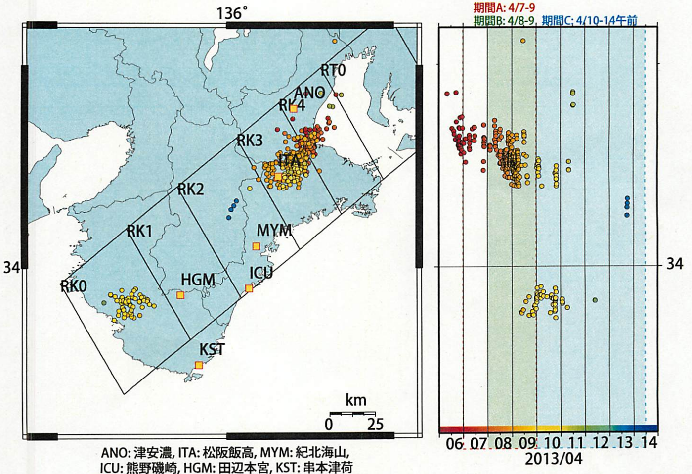
図22: 2013/4/6 0:00 - 4/13 0:00 における紀伊半島の深部低周波微動の時空間分布図。 エンベロープ相関法により決定。
