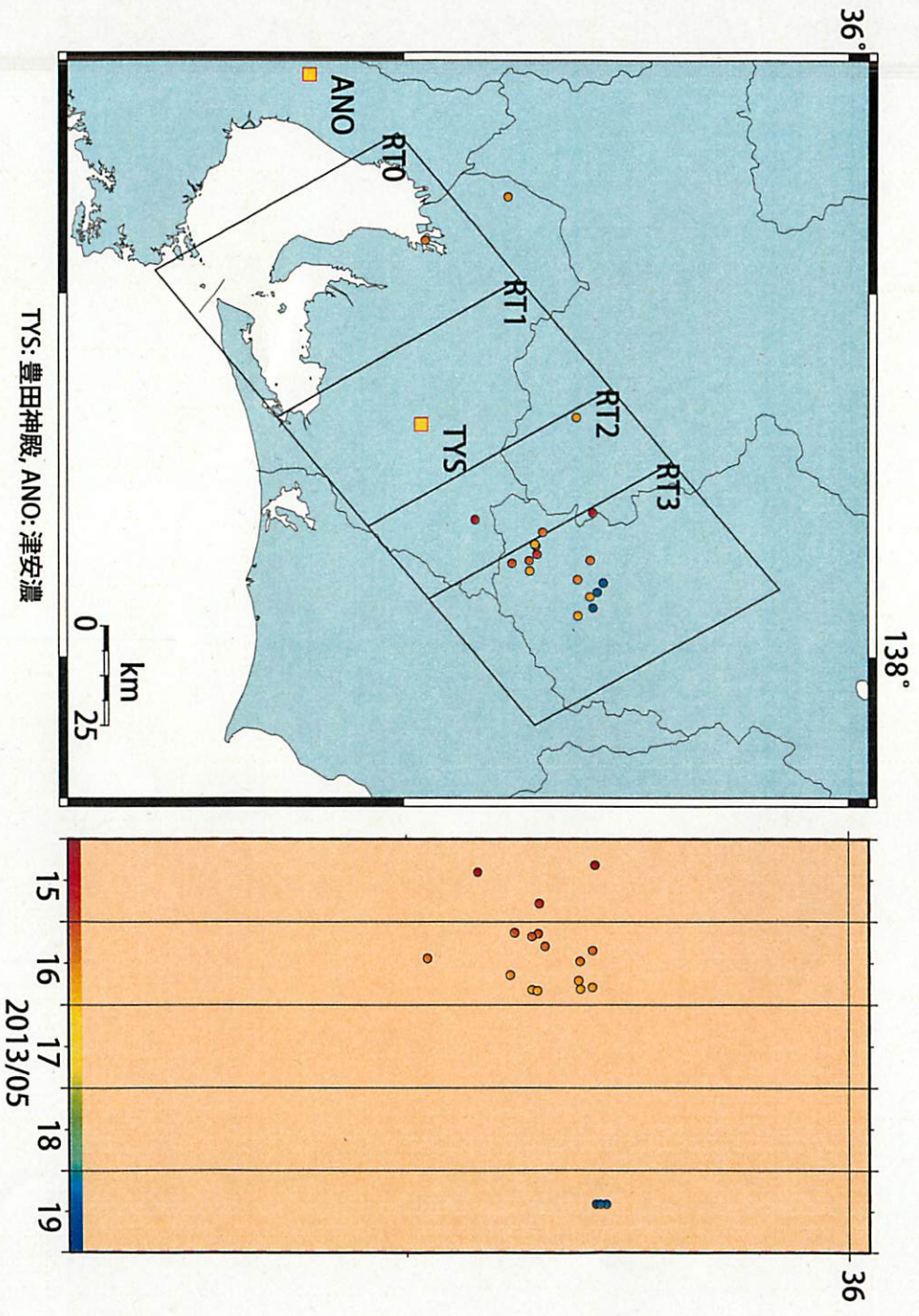
図22: 2013/5/15 0:00 - 5/20 0:00 における東海地方の深部低周波微動の時空間分布図。 エンベロープ相関法により決定。
