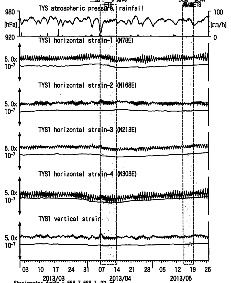
図2: Crustal strains changes at TYS 豊田神殿 (時間値) (2013/03/01 00:00 - 2013/05/27 00:00) 三重中～伊勢湾 長野・愛知 泉境ETS
