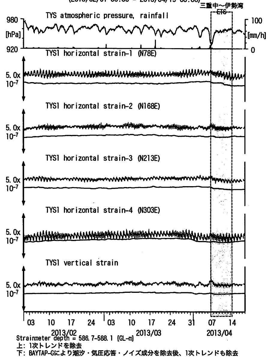
図2: Crustal strains changes at TYS 豊田神殿 (時間値) (2013/02/01 00:00 - 2013/04/19 00:00)
