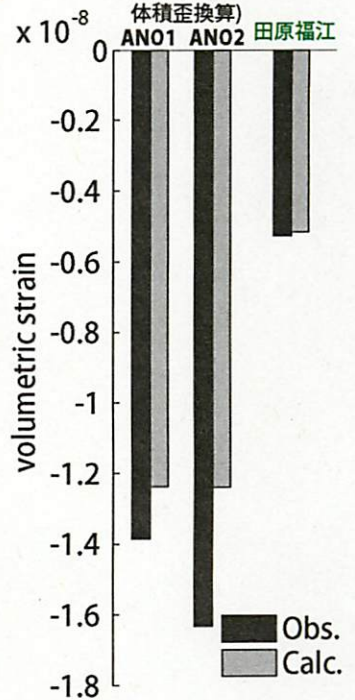
体積歪比較 (地下水圧→ 体積歪換算)
