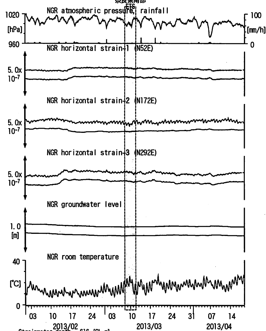
図19: Crustal strain and groundwater level changes at 岩出東坂本 (時間値) (2013/02/01 00:00 - 2013/04/19 00:00) 奈良県南部
