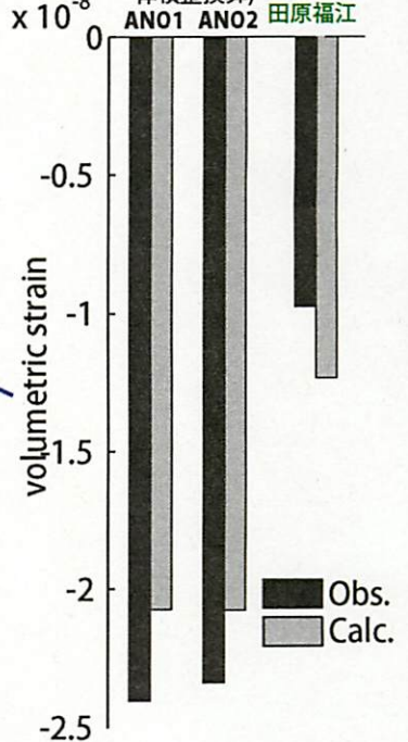
体積歪比較 (地下水圧→ 体積歪換算)
