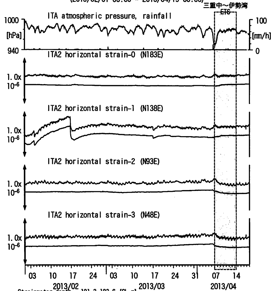
図9: Crustal strain changes at ITA 松阪飯高 (時間値) (2013/02/01 00:00 - 2013/04/19 00:00)
