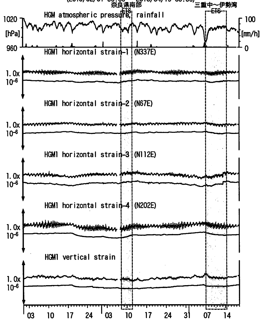
図15: Crustal strains changes at HGM 田辺本宮 (時間値) (2013/02/01 00:00 - 2013/04/19 00:00)
