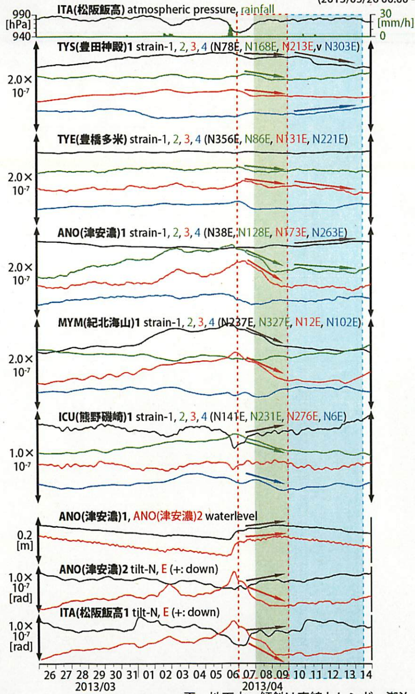
図23: 愛知県~三重県における歪・地下水・傾斜・微動観測結果(時間値) (2013/03/26 00:00 - 2013/04/15 00:00)
