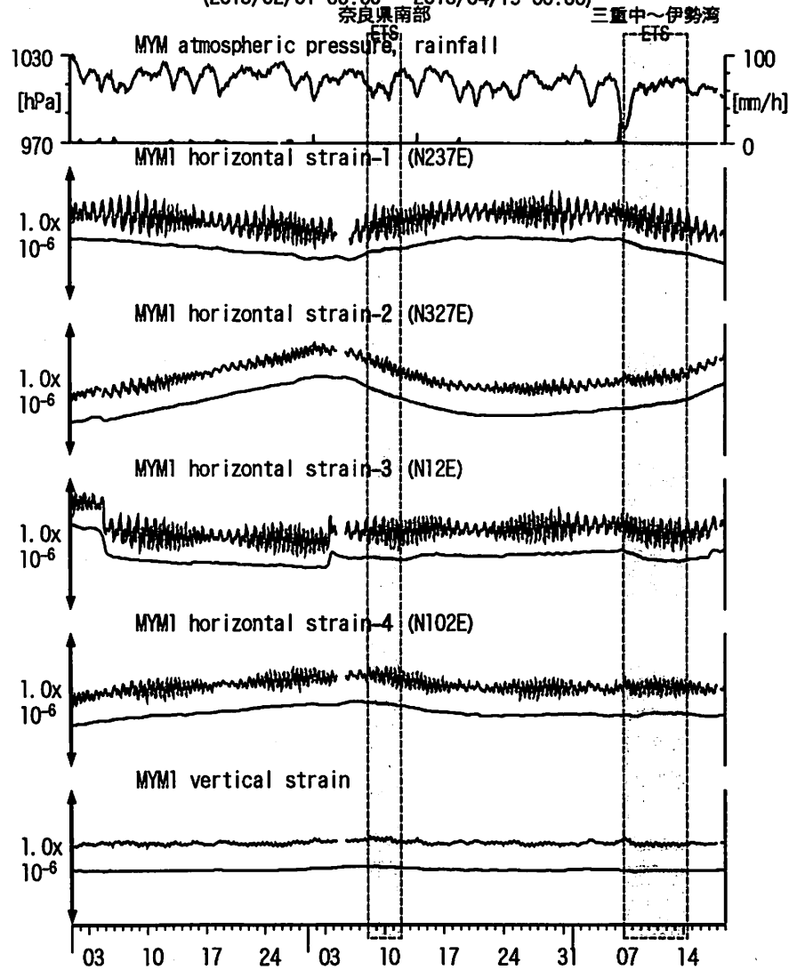
図11: Crustal strain changes at MYM 紀北海山 (時間値) (2013/02/01 00:00 - 2013/04/19 00:00)
