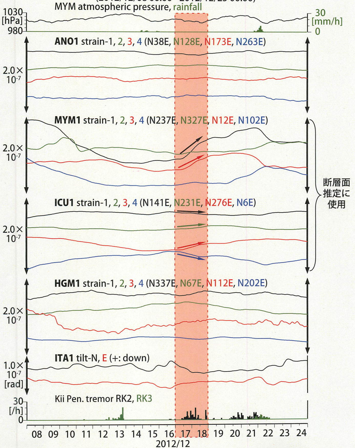
図23: 紀伊半島における歪・傾斜観測結果 (2012/12/08 00:00 - 2012/12/25 00:00)
