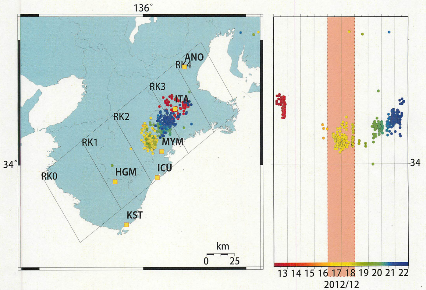
図22: 2012/12/13 0:00 - 12/23 0:00 における紀伊半島の深部低周波微動の時空間分布図。 エンベロープ相関法により決定。
