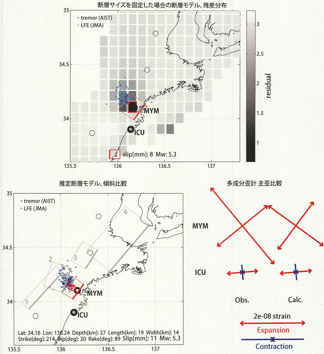
図24: (上段)プレート境界面上のパッチ(断層面)をすべらせた際の、歪・傾斜の観測値と計算値の残差分布図。断層面サイズは固定(20x20km)。赤色矩形は最小残差の断層面を表す。このパッチのすべり量、Mwを下部に示している。残差の小さい領域(色の濃い領域)が広くコントラストが低く、任意性が高いと考えられる。
