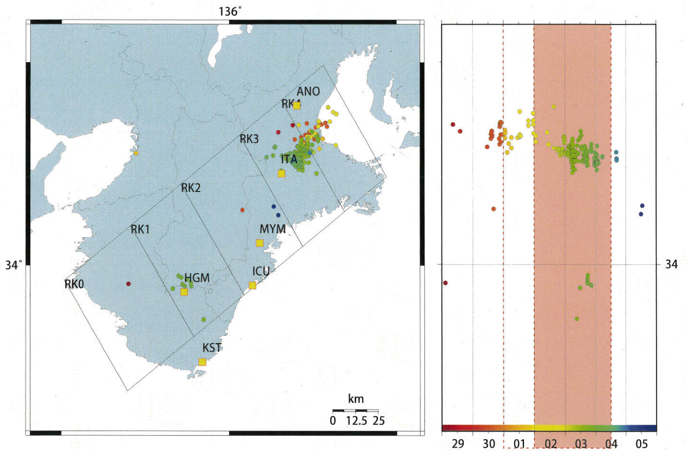
図22: 2012/9/29 0:00 - 10/6 0:00 における紀伊半島の深部低周波微動の時空間分布図。 エンベロープ相関法により決定。
