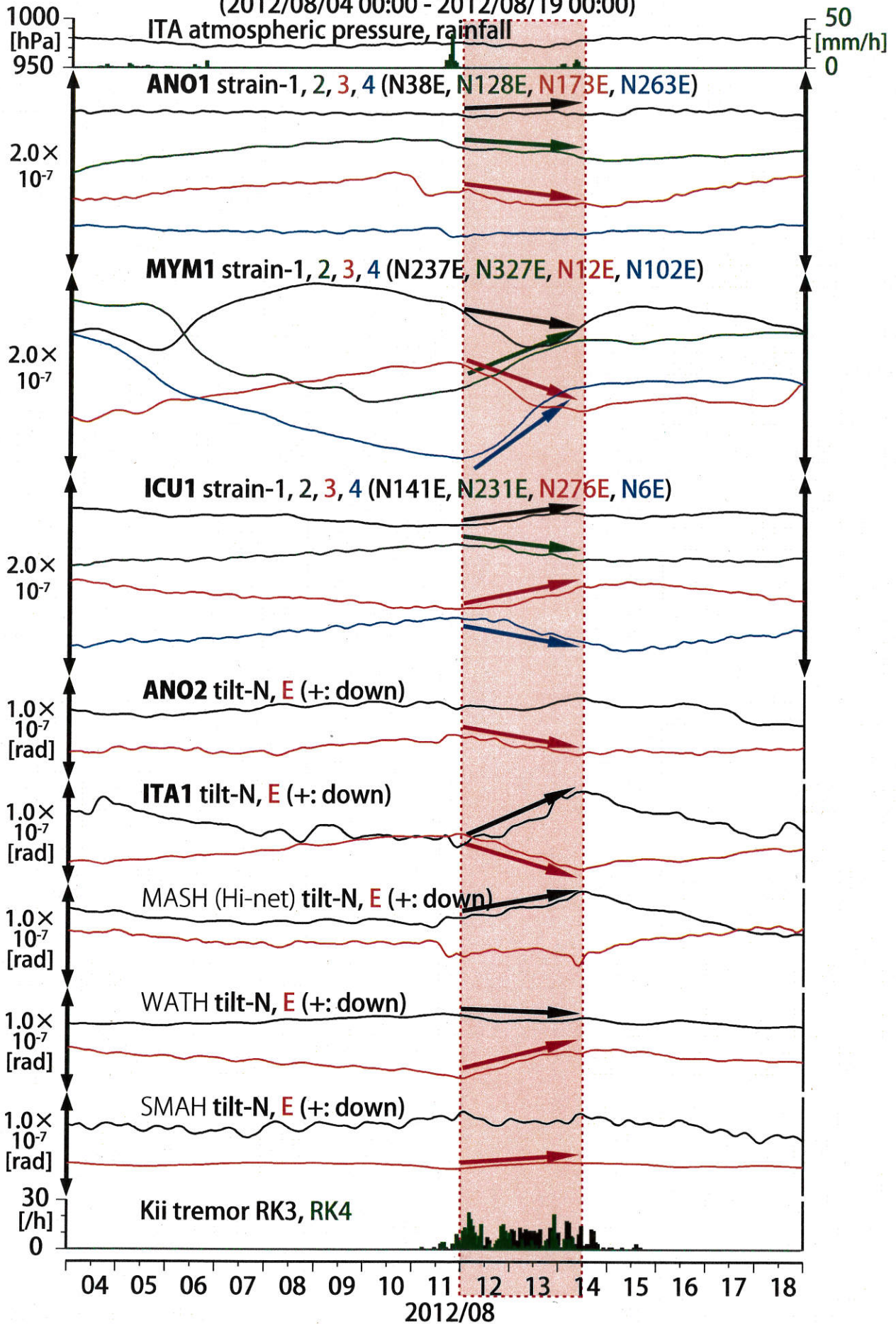
図23: 紀伊半島における歪・傾斜観測結果 (2012/08/04 00:00 - 2012/08/19 00:00)
