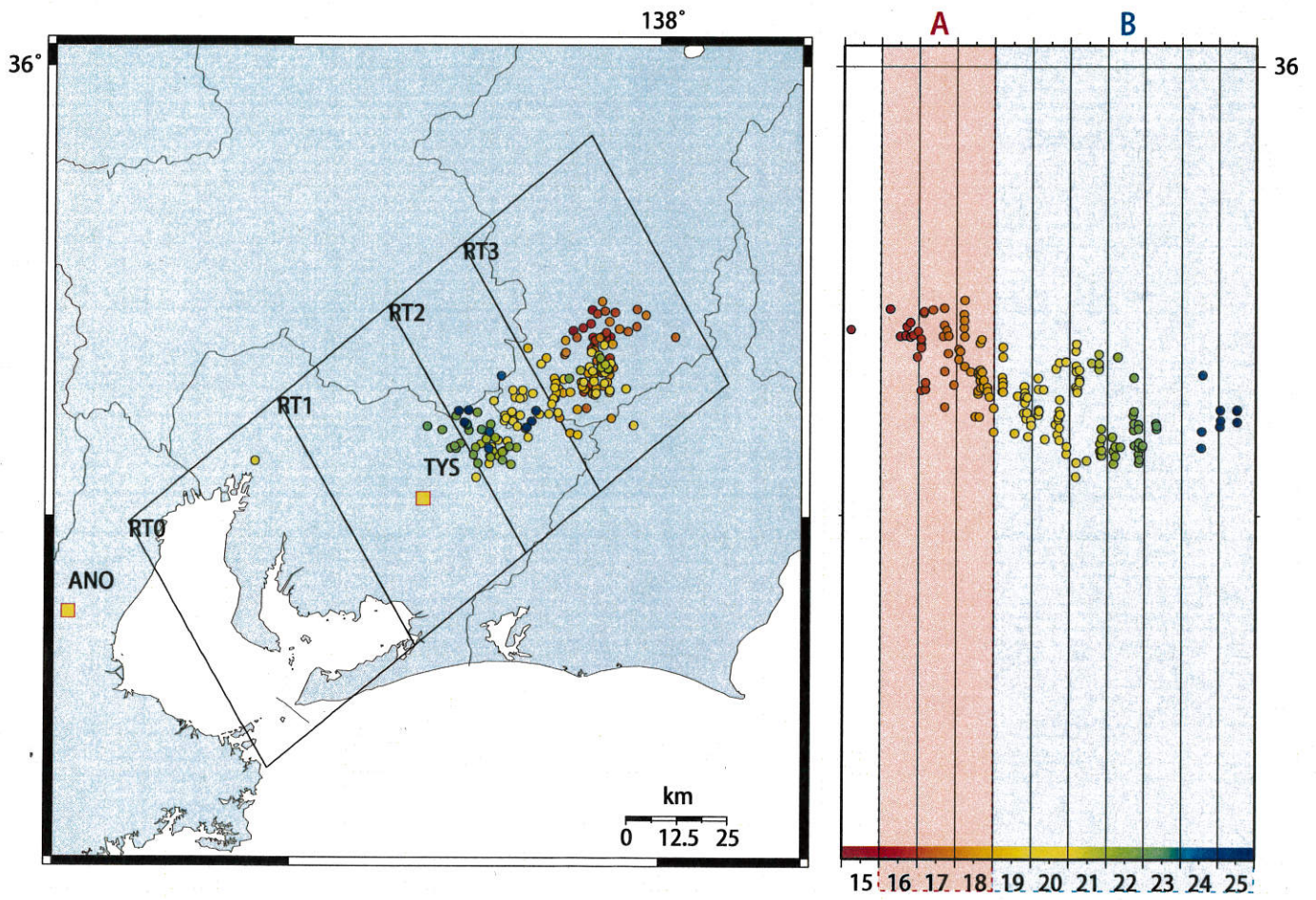
図25: 2012/8/15 0:00 - 8/26 0:00 における東海地方の深部低周波微動の時空間分布図。 エンベロップ相関法により決定。
