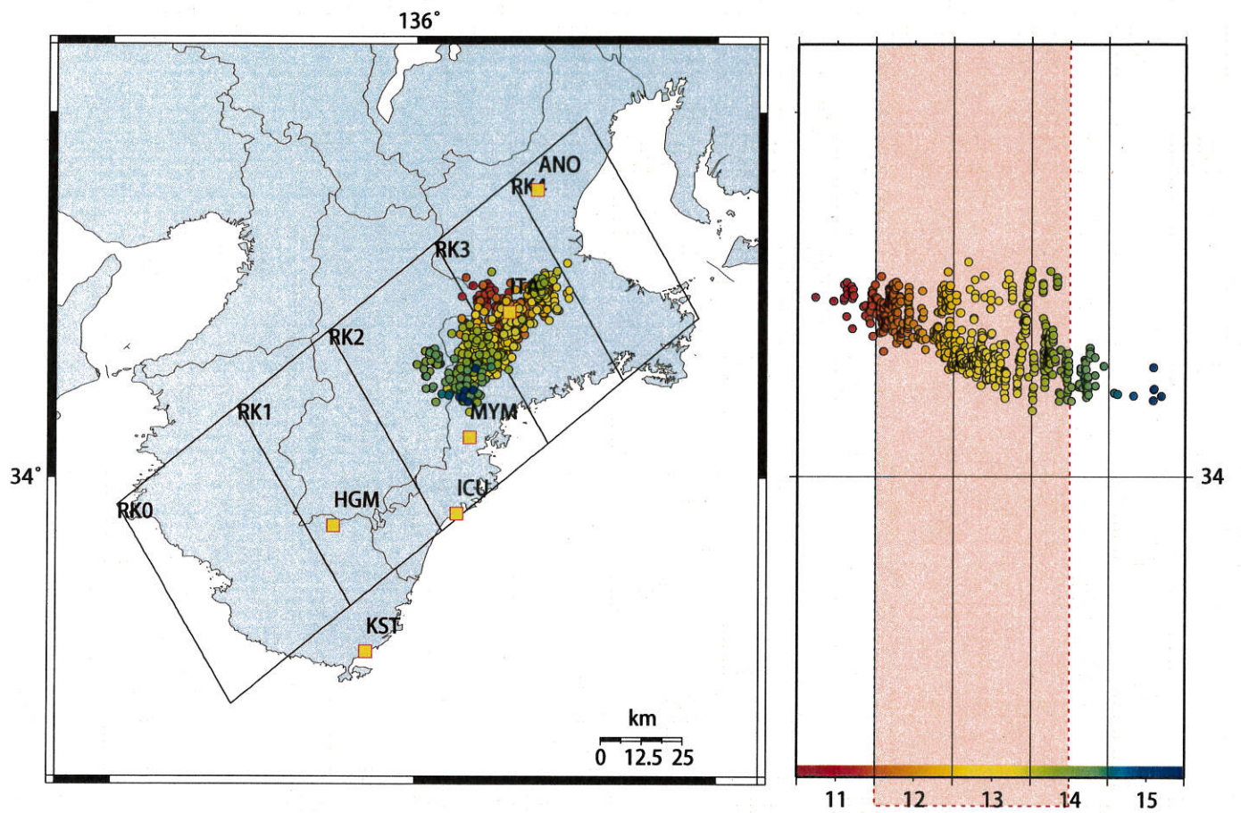
図22: 2012/8/11 0:00 - 8/16 0:00 における紀伊半島の深部低周波微動の時空間分布図。 エンベロープ相関法により決定。
