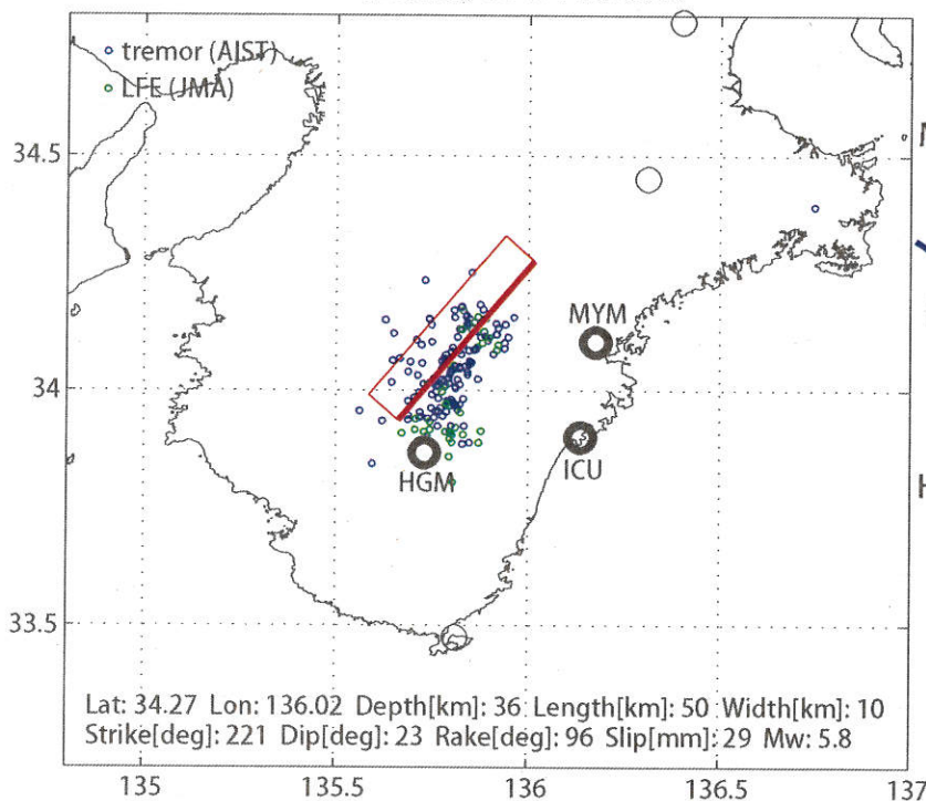
推定断層モデル、傾斜比較
