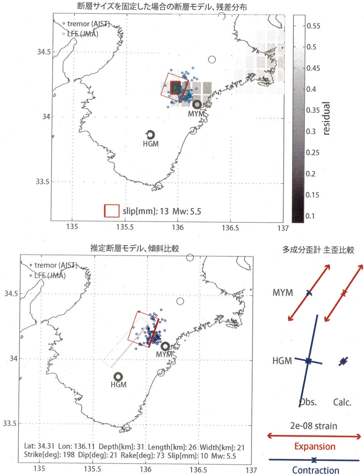
図25: (上段)プレート境界面上のパッチ(断層面)をすべらせた際の、歪・傾斜の観測値と計算値の残差分布図。断層面サイズは固定(20x20km)。赤色矩形は最小残差の断層面を表す。このパッチのすべり量、Mwを下部に示している。
