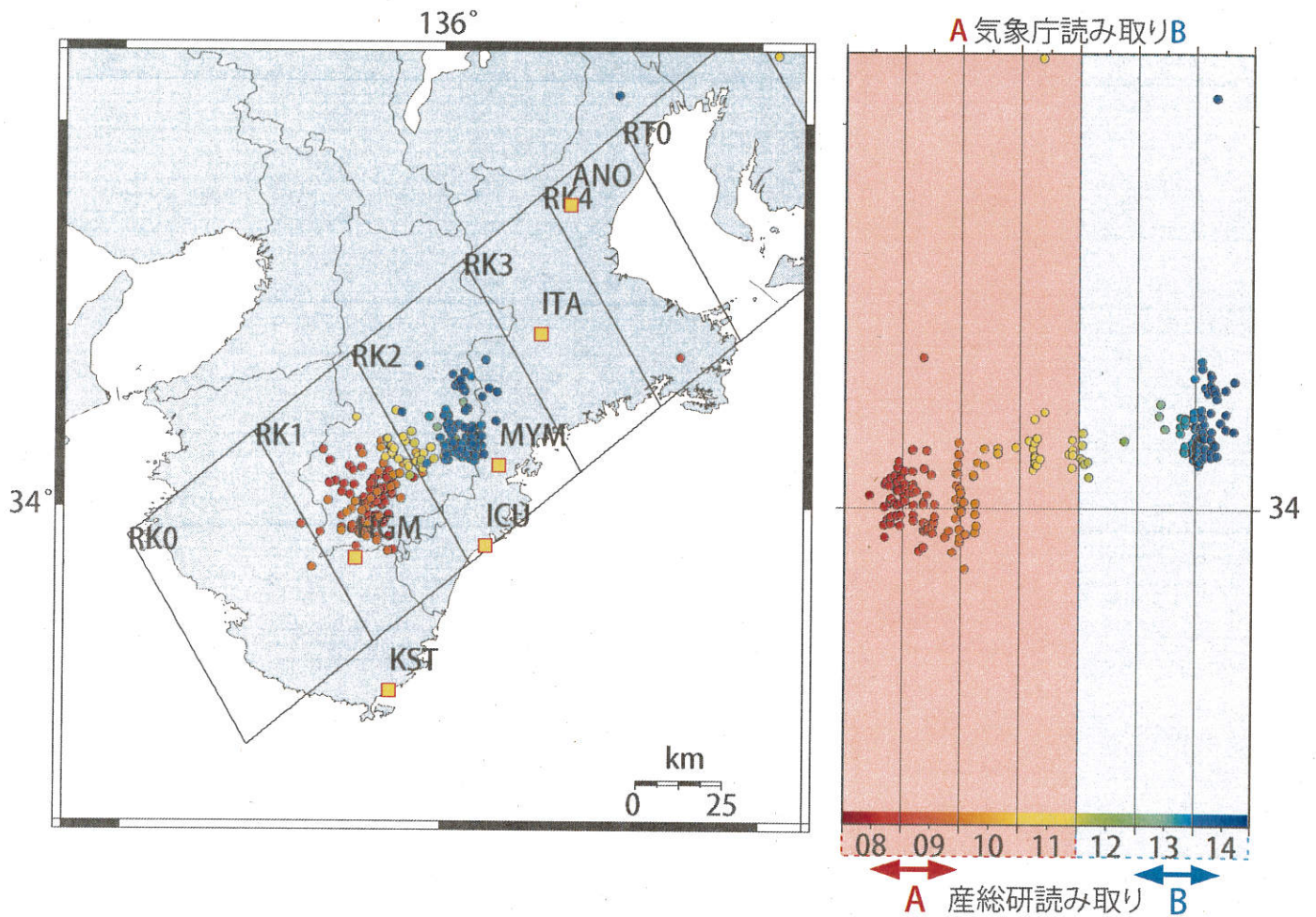
図22: 2012/6/8 0:00 - 6/15 0:00 における紀伊半島の深部低周波微動の時空間分布図。 エンベロープ相関法により決定。
