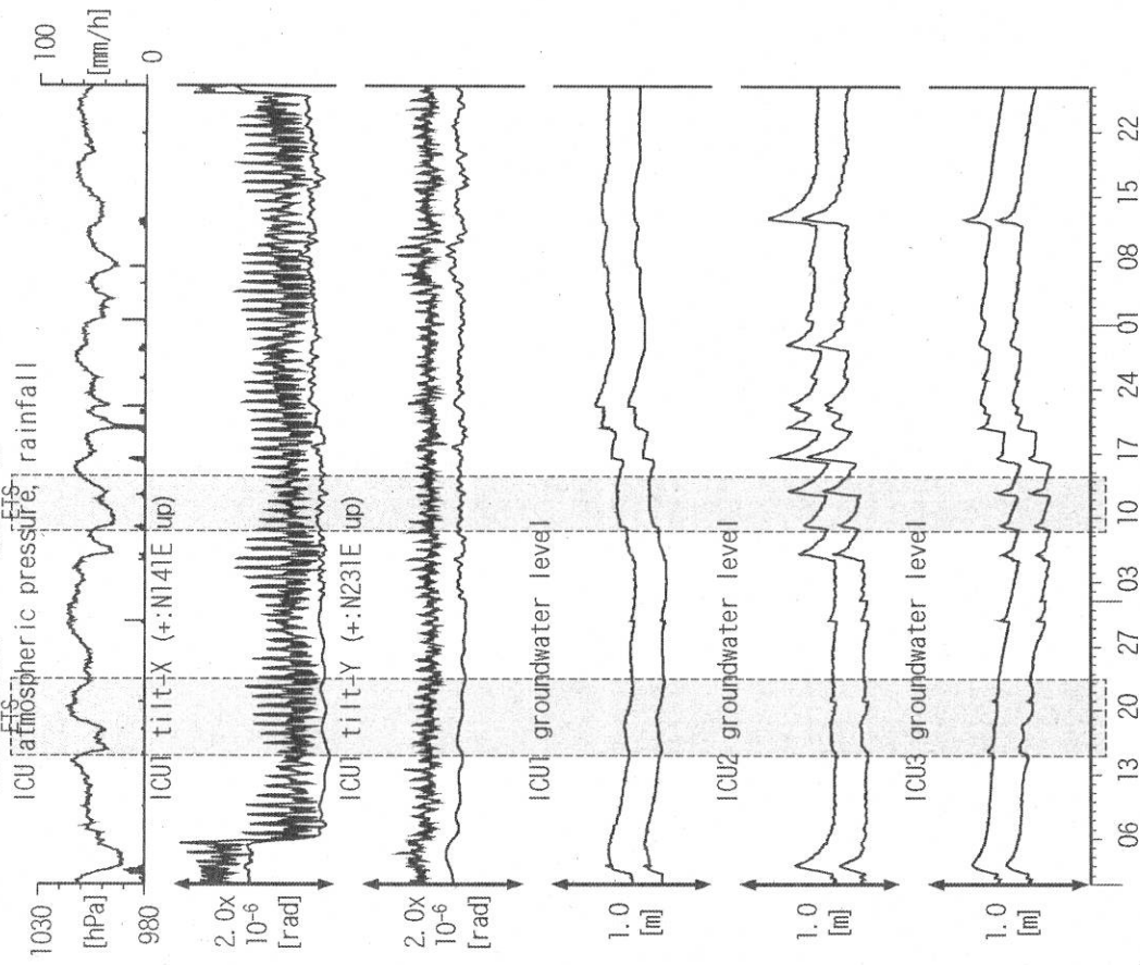
図14: Tilt and groundwater level changes at ICU (時間値) (2012/05/01 00:00 - 2012/07/27 00:00) 三重中～伊勢湾 奈良南～東
