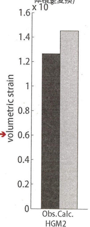
体積歪比較 (地下水圧→体積歪変換)
