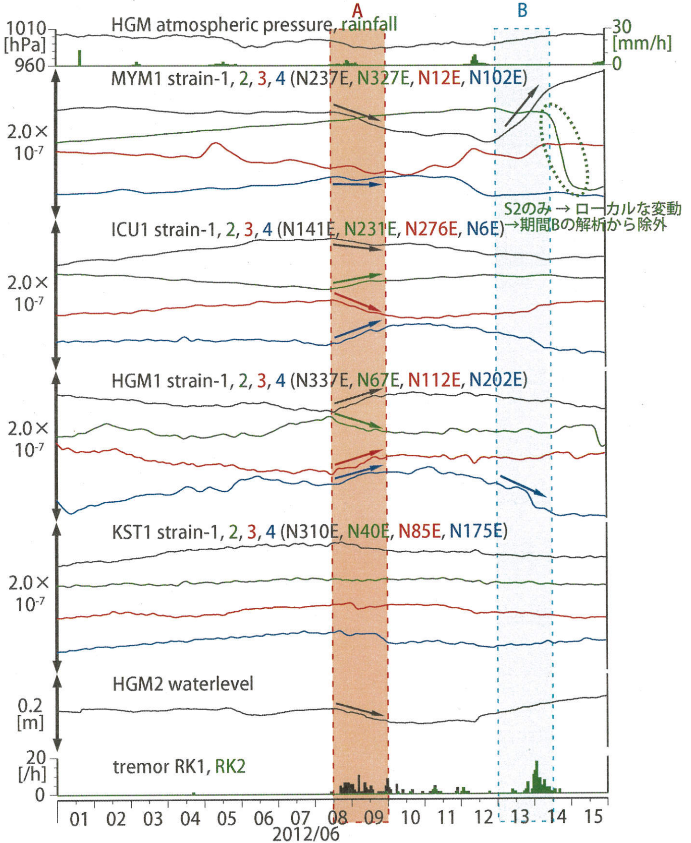
図23: 紀伊半島における歪・地下水・傾斜観測結果 (2012/06/01 00:00 - 2012/06/16 00:00)
