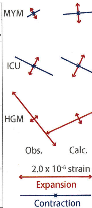
多成分歪計 主歪比較
