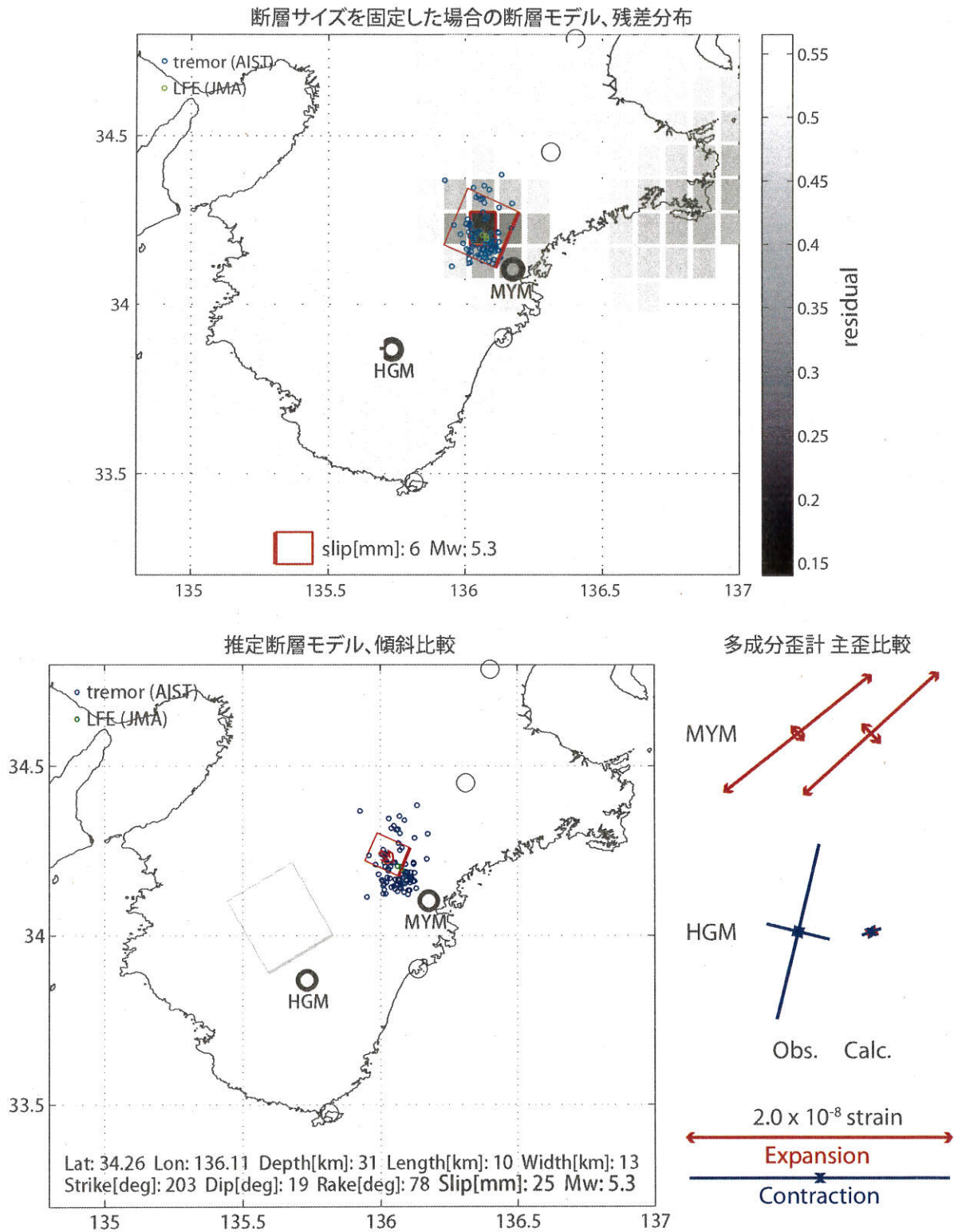
図25: (上段)プレート境界面上のパッチ(断層面)をすべらせた際の、歪・傾斜の観測値と計算値の残差分布図。断層面サイズは固定(20x20km)。赤色矩形は最小残差の断層面を表す。このパッチのすべり量、Mwを下部に示している。残差の小さい領域(色の濃い領域)が広くコントラストが低いため、任意性が高いと考えられる。
