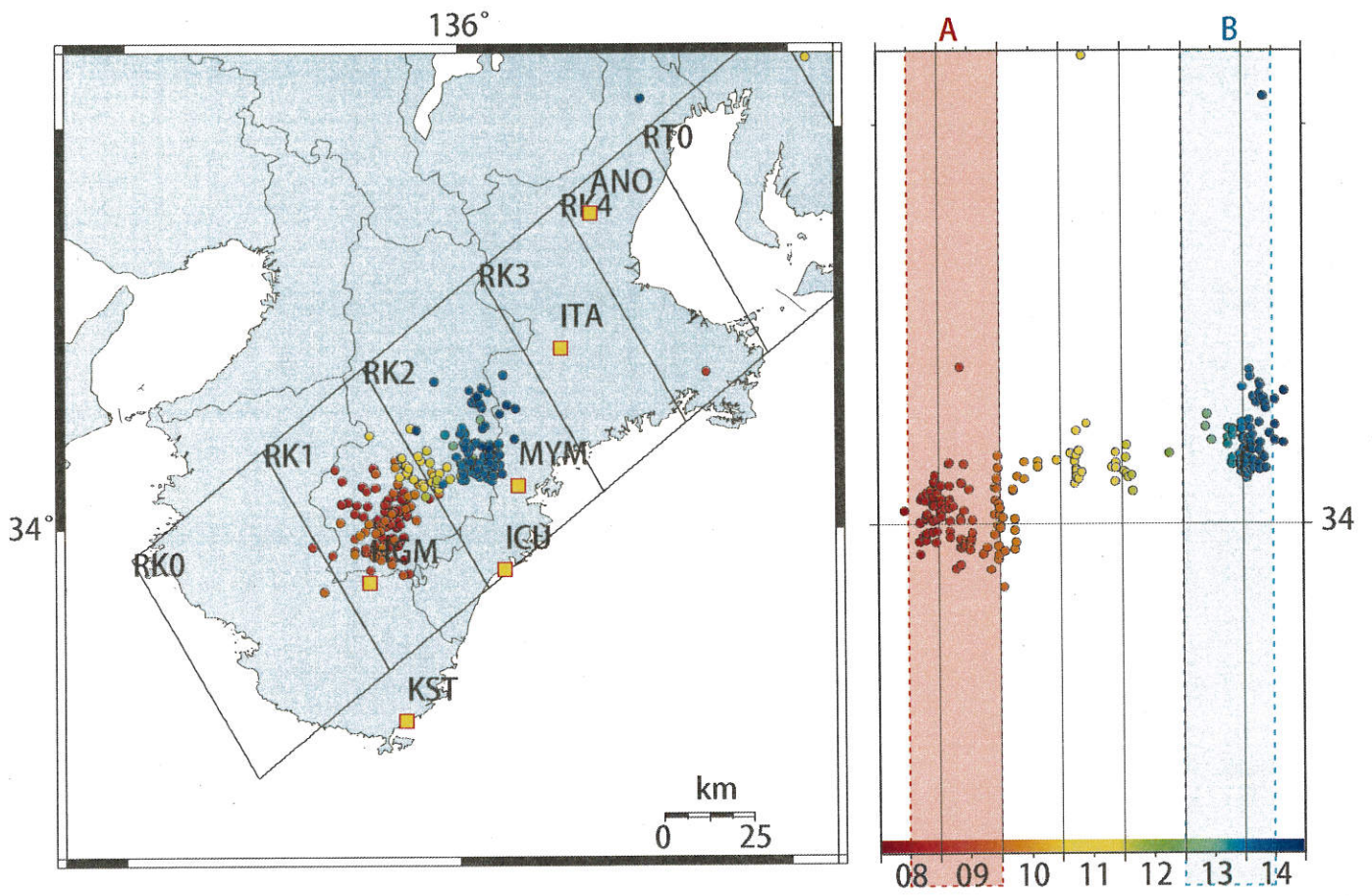
図22: 2012/6/8 0:00 - 6/15 0:00 における紀伊半島の深部低周波微動の時空間分布図。 エンベロープ相関法により決定。
