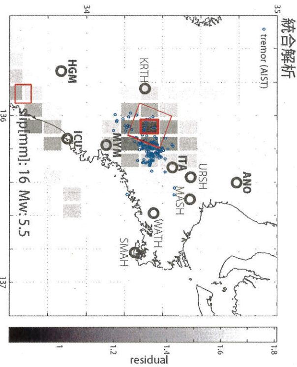
図24: プレート境界面上のバッチ(断面)をすべらせた際の、歪・傾斜の観測値と計算値の残差分布図。 小さな青色丸印は産総研による深部低周波微動、緑色丸印は気象庁一元化カタログによる低周波イベントの震央位置を示す。太字は産総研の、細字は防災科研Hi-netの観測点名を示す。バッチサイズは20×20km、すべり量は1-100mmで可変(1mm間隔)。表示しているグリッドは断面下端中央の位置を示す。黒色矩形は最小残差の断面面を表す。このバッチのすべり量、Mwを下部に示している。太黒丸は計算に使用した観測点を示す。統合解析では、残差の小さい領域(色の濃い領域)が、歪のみ・傾斜のみの場合より狭まっており、一意性が高まっていると考えられる。
