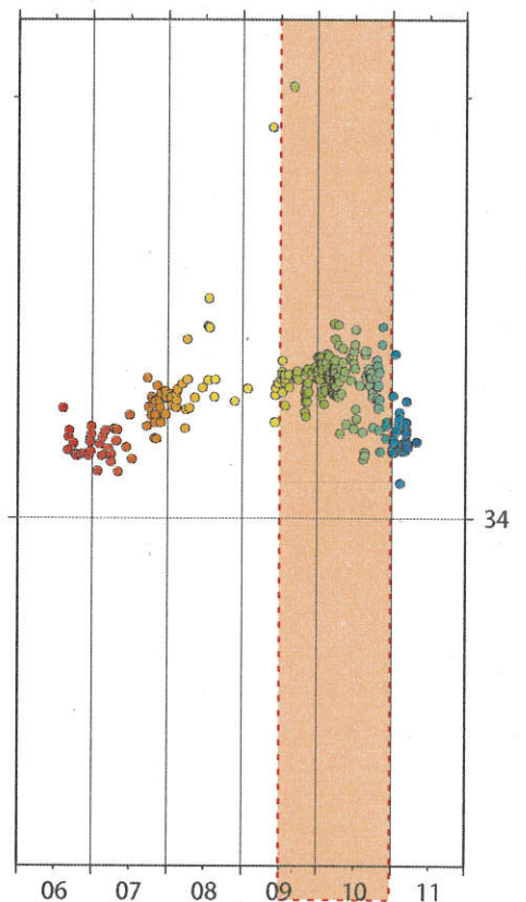
図 22: 2012/2/6 0:00 - 2/12 0:00 における紀伊半島の深部低周波微動の時空間分布図。エンベロップ相関法により決定。
