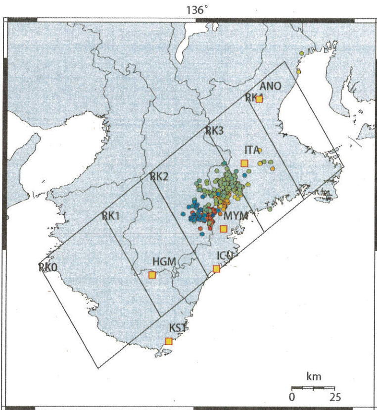
図 22: 2012/2/6 0:00 - 2/12 0:00 における紀伊半島の深部低周波微動の時空間分布図。エンベロップ相関法により決定。
