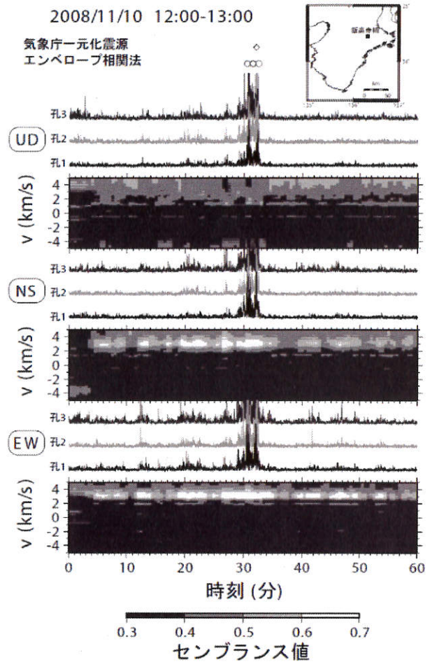
センブランス解析結果例. (今西他 2009 より引用.)
