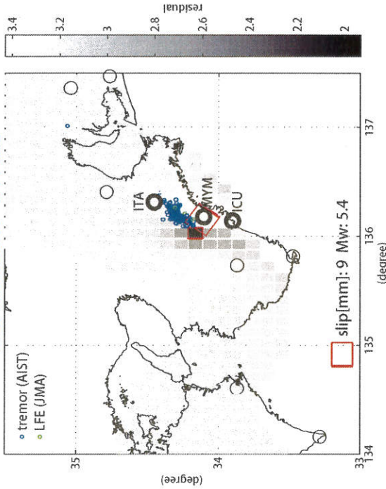
図24: プレート境界面上のハッチ(断層面)をすべらせた際の、歪3成分の観測値と計算値の残差分布図。青丸は産総研による深部低周波微動震央、ハッチサイズは20×20km、すべり量は1-100mmで可変(1mm間隔)。赤線は最小残差のハッチおよび断層面を表す。このハッチのすべり量、Mwを下部に示している。太黒丸は計算に使用した観測点を示す。
