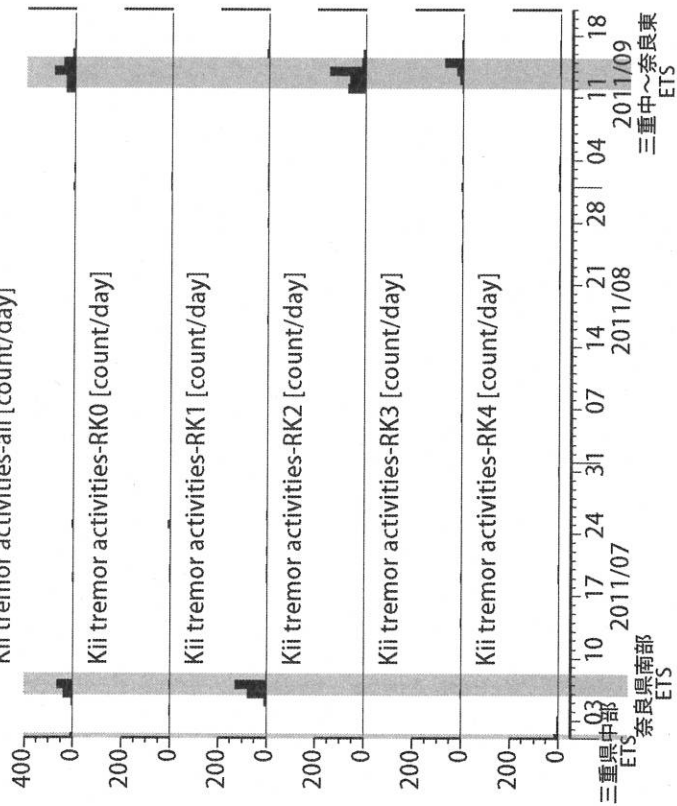
図 21: 紀伊半島～愛知県における深部低周波微動の時空間分布(上段)、各領域における発生頻度(日値)。エンベロープ相関法により決定した。防災科研 Hi-net、気象庁、東京大学、京都大学、名古屋大学、高知大学、九州大学の地震波形記録を用いました。
