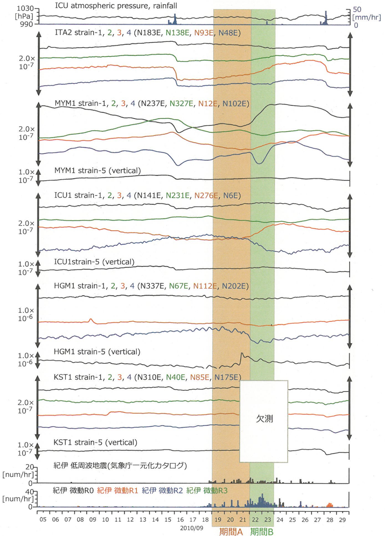
図20: 紀伊半島における歪観測結果 (時間値) (2010/09/05 00:00 - 2010/09/30 00:00)
