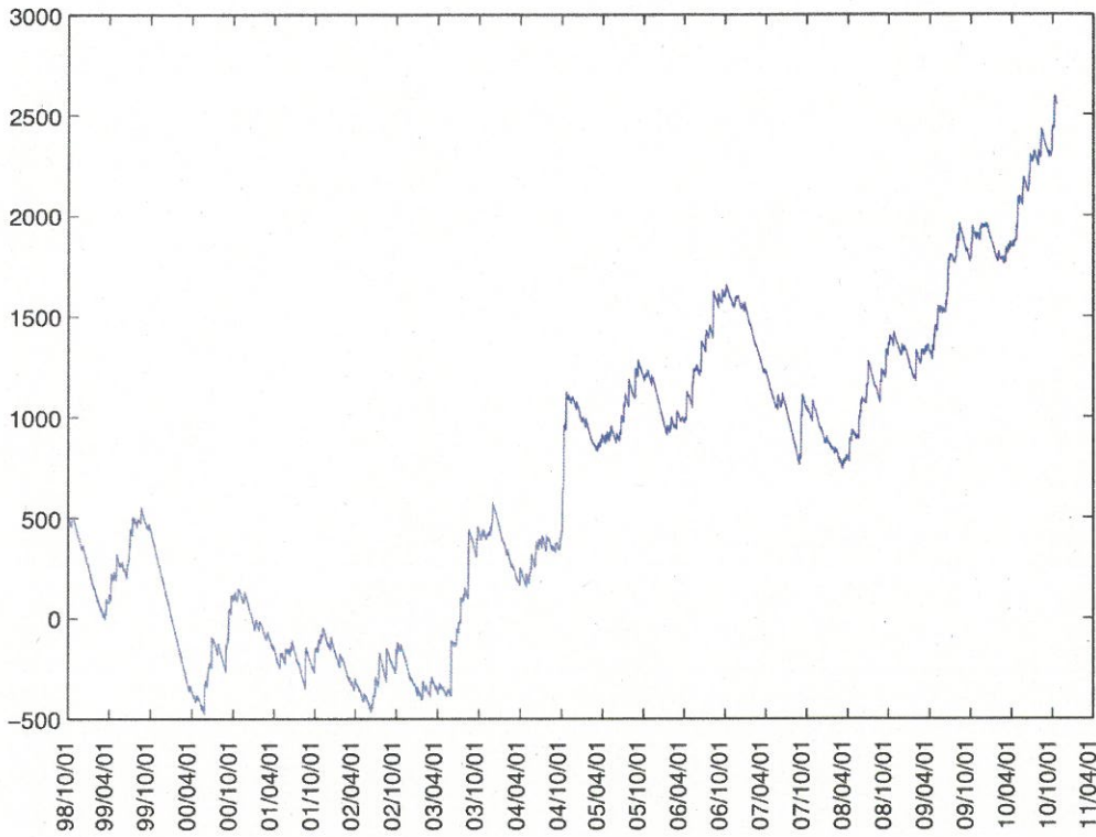
榛原観測井 降雨量の積算からトレンド除去後のグラフ (mm) (1998. 10. 1-2010. 10. 22)
