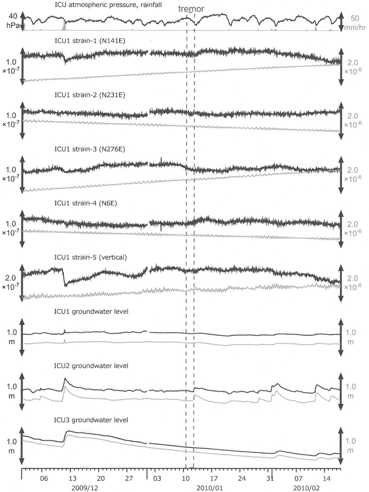
図3: 紀伊半島南部の地下水・歪観測結果: ICU (時間値) (2009/12/01 00:00 - 2010/02/18 00:00)
