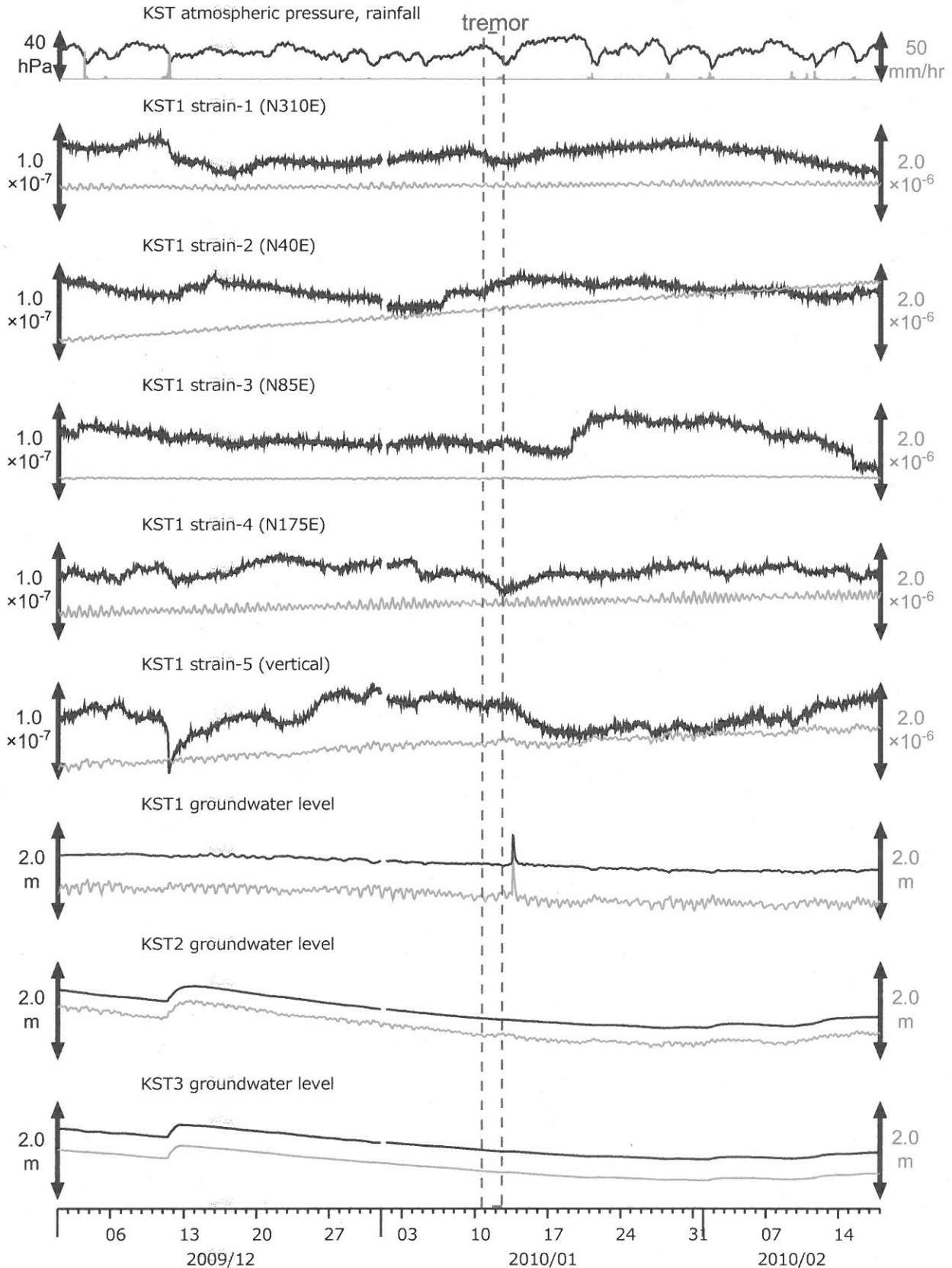
図5: 紀伊半島南部の地下水・歪観測結果: KST (時間値) (2009/12/01 00:00 - 2010/02/18 00:00)
