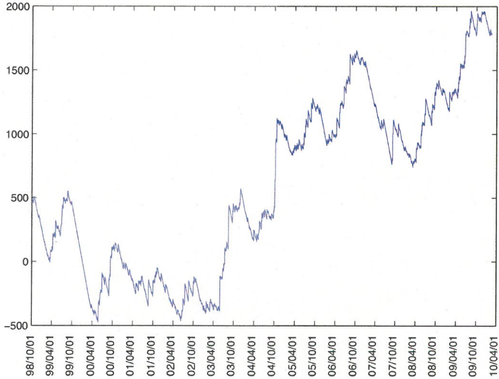
榛原観測井 降雨量の積算からトレンド除去後のグラフ (mm) (1998. 10. 1-2010. 02. 15)
