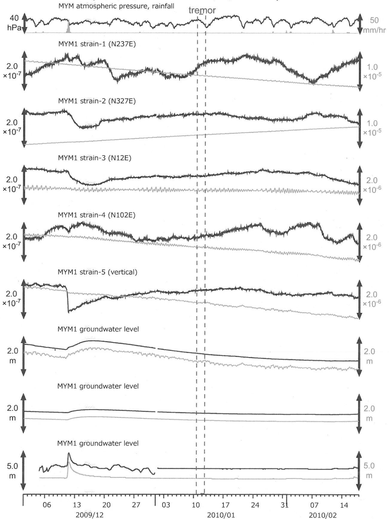
図2: 紀伊半島南部の地下水・歪観測結果: MYM (時間値) (2009/12/01 00:00 - 2010/02/18 00:00)
