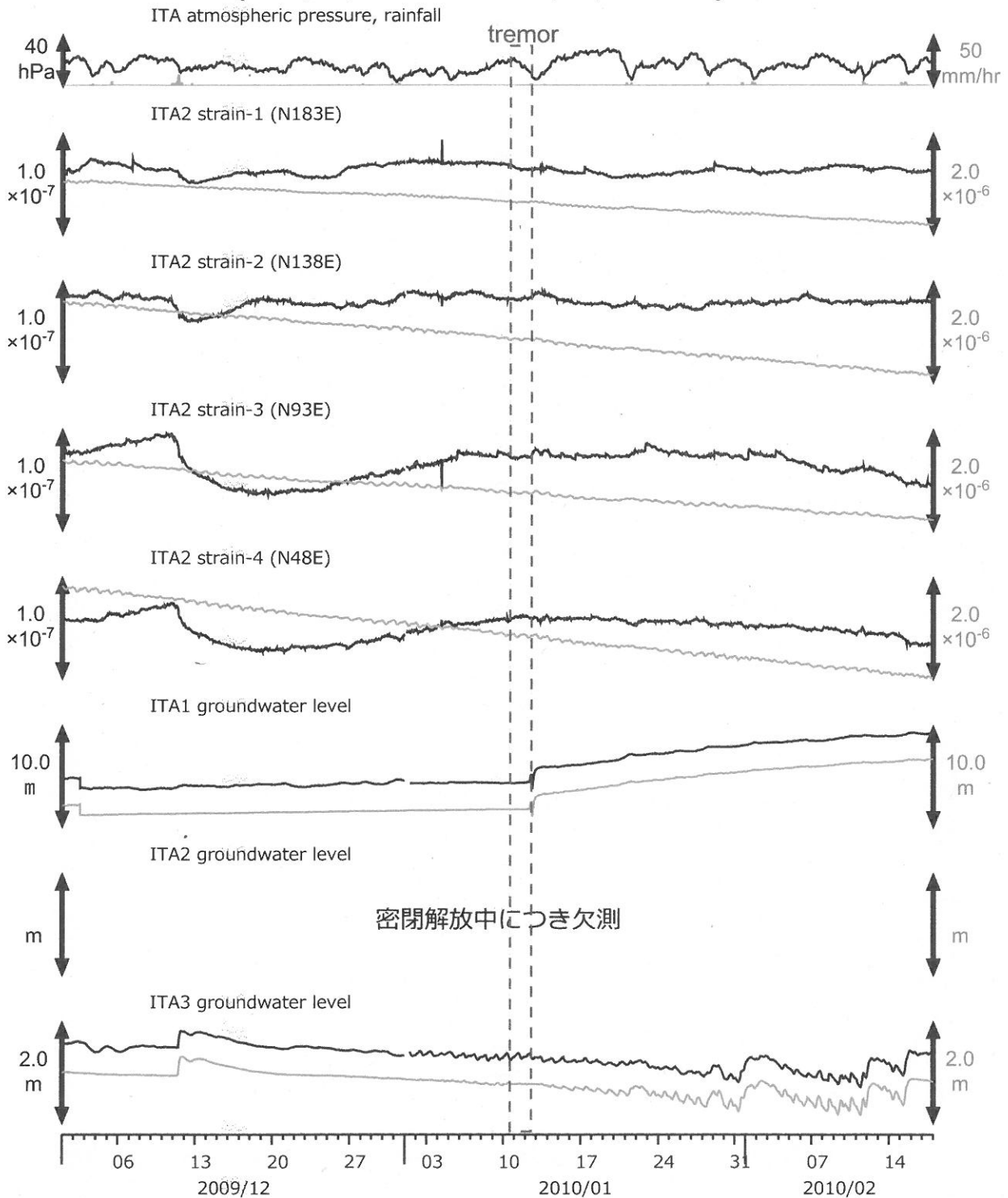
図1: 紀伊半島南部の地下水・歪観測結果: ITA (時間値) (2009/12/01 00:00 - 2010/02/18 00:00)
