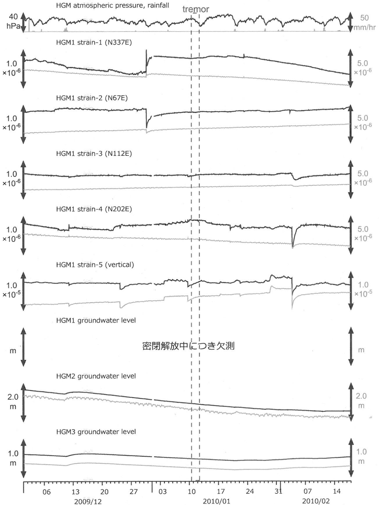
図4: 紀伊半島南部の地下水・歪観測結果: HGM (時間値) (2009/12/01 00:00 - 2010/02/18 00:00)
