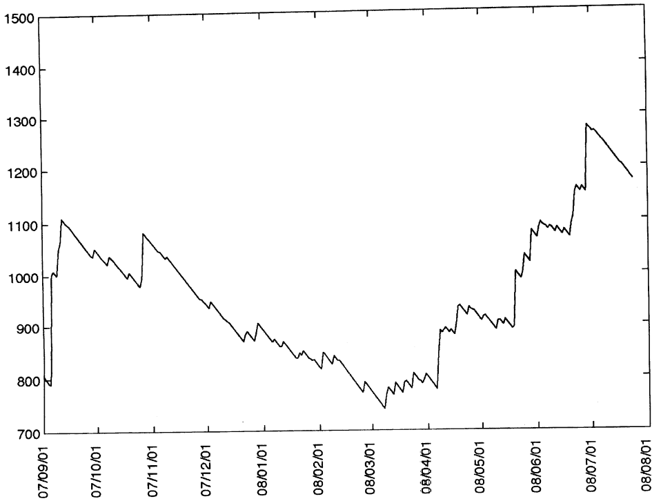
榛原観測井 降雨量の積算からトレンド除去後のグラフ (mm) (2007. 9. 1-2008. 7. 24)
