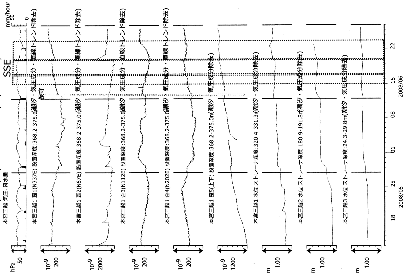
図6: 紀伊半島南部の地下水・歪観測結果: 本宮三越(B., TAP) (時間値) (2008/05/13 00:00 - 2008/06/27 00:00)
