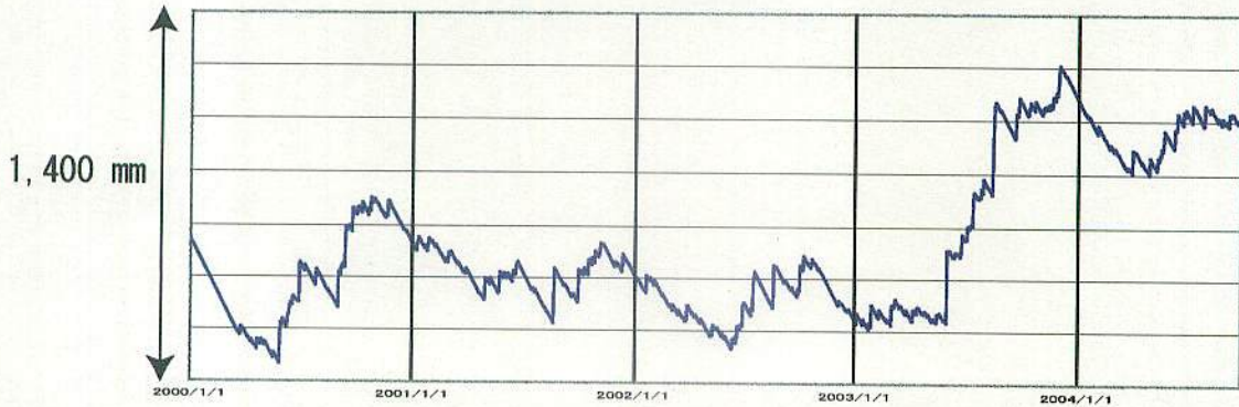
浜岡雨量 (トレンド除去後)
