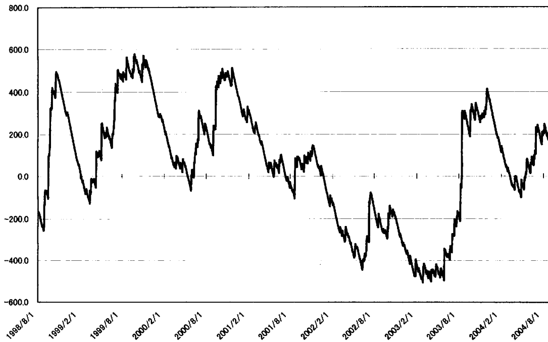
榛原観測井 降雨量の積算からトレンド除去後のグラフ (mm) (1998. 8. 1-2004. 8. 29)
