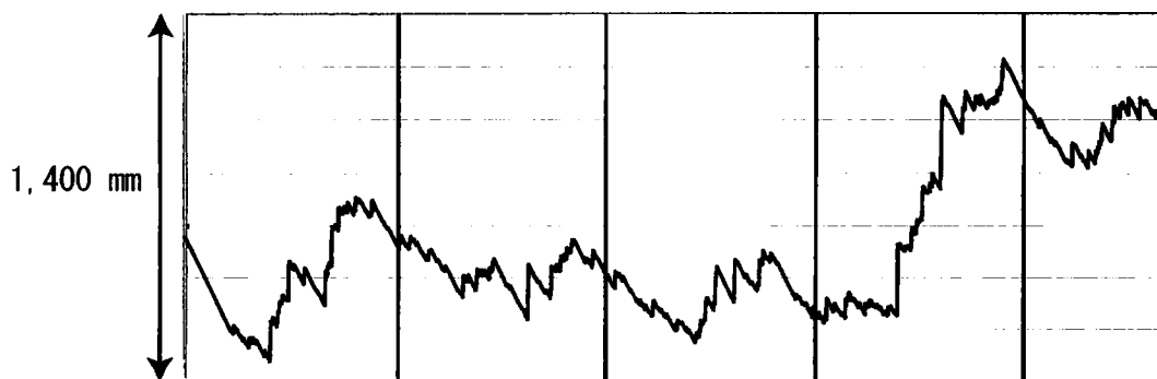
浜岡雨量 (トレンド除去後)
