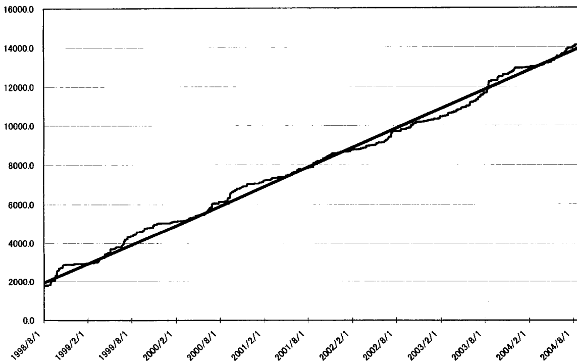
榛原の降雨量の積算グラフ (1998. 8. 1-2004. 8. 29) (mm)
