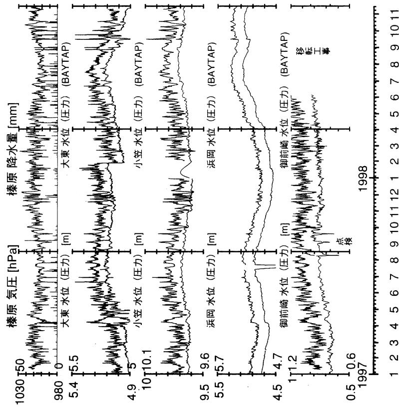
東海地域南部 地下水観測結果 (時間値) (1997/01/01 00:00 - 1998/11/16 00:00)
