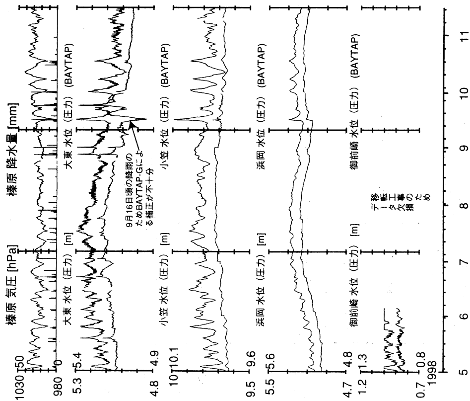
東海地域南部 地下水観測結果 (時間値) (1998/05/01 00:00 - 1998/11/16 00:00)
