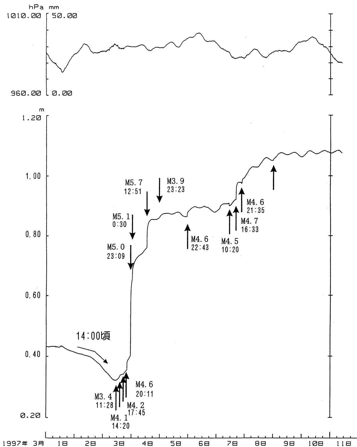
第5図 1997年3月1日～3月10日の大室山北における地下水位観測結果。矢印は、主な地震の発生時を示す。
