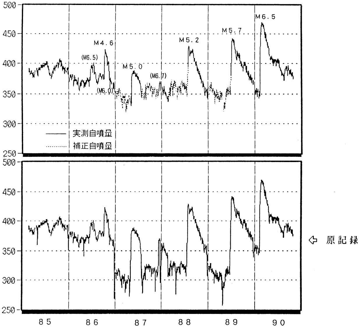
赤沢6号温泉の自噴量変動（揚水補正後） 1985-1990
