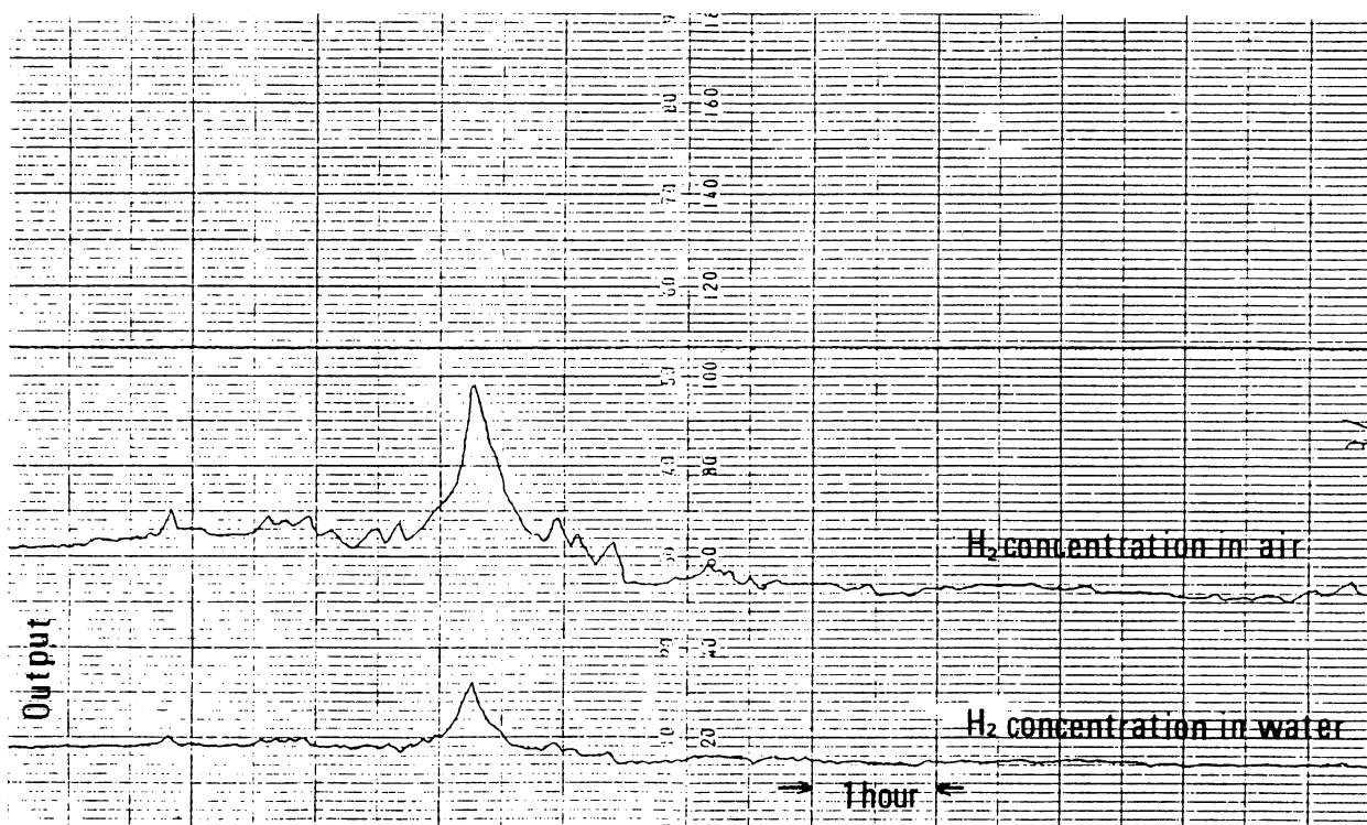
第 5 図 伊東市赤沢 6 号泉における溶存水素濃度の経時変化図
