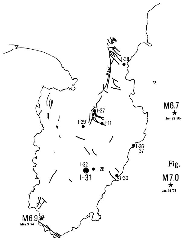
第1図 観測井の位置（～確実な活断層）
