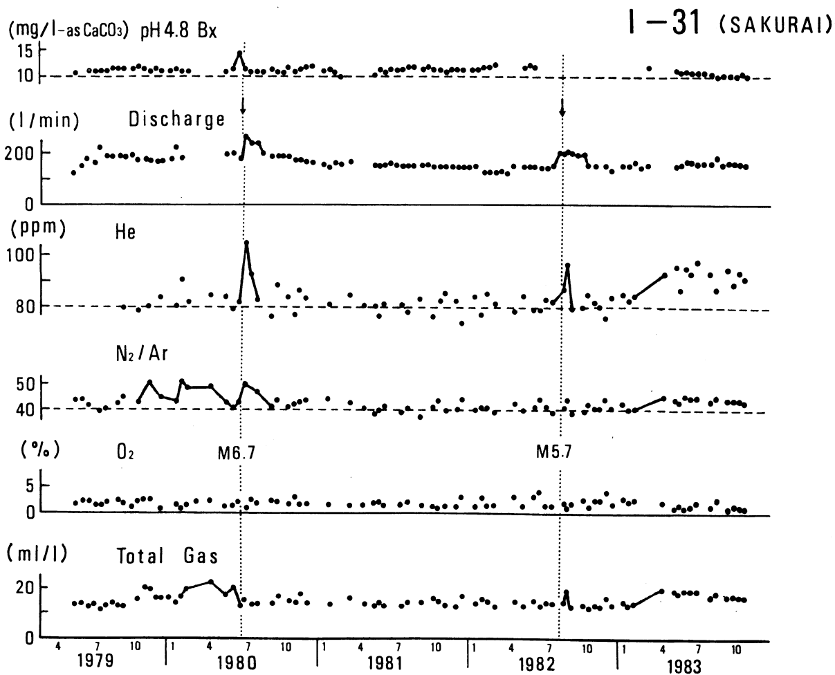
第2図 桜井温泉の溶存ガス組成変動
