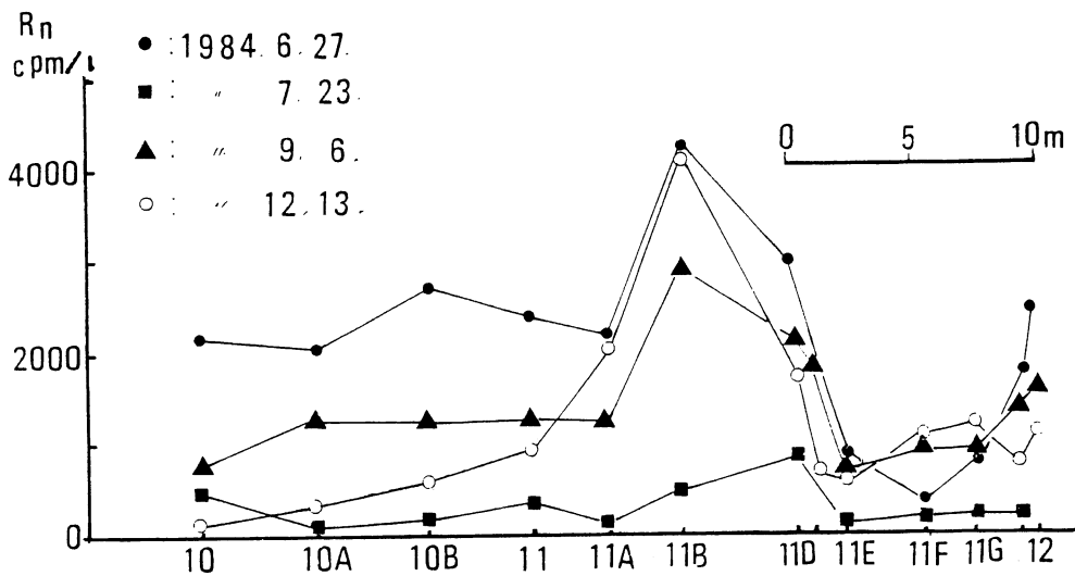
第2図 観測線上におけるラドン濃度の分布と変化
