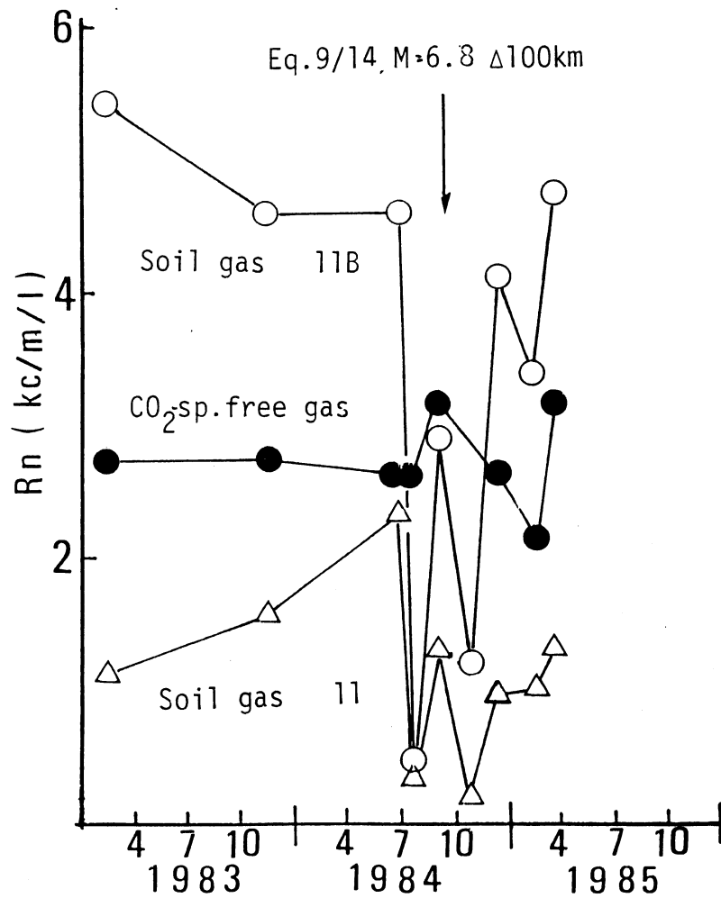
第3図 土中およびCO 2 泉遊離ガス中のラドン濃度の経時変化
