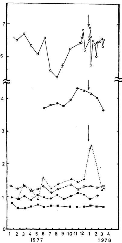
第4図 伊豆半島におけるラドン濃度観測結果 (1回/月)
