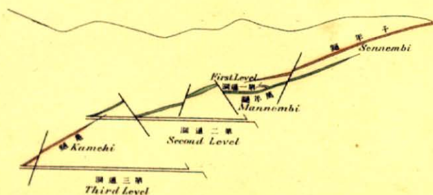
圖面斷縱 VERTICAL SECTION
