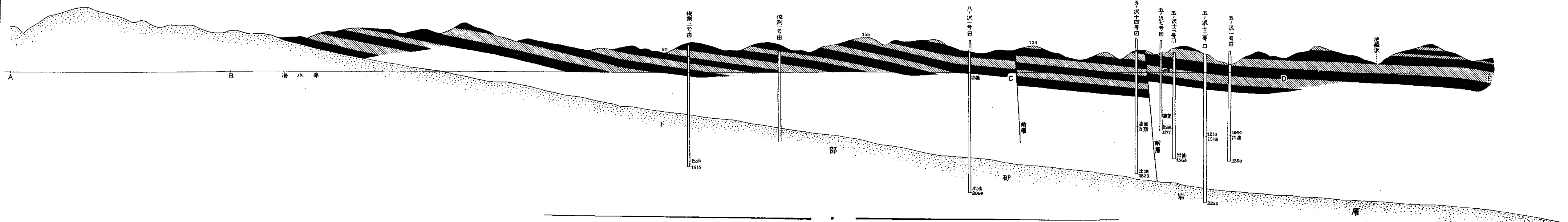
俊別背斜主要部線 F G H I J K L M 断面圖
