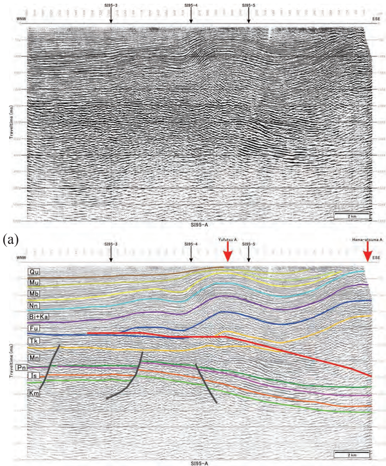
第3図 SI95-A 測線の解釈図 (a)通常処理マイグレーション後時間断面. (b)MDRS 処理マイグレーション後時間断面. 上段:元の断面. 下段:解釈断面. 地層名の略号は以下の各解釈図ですべて共通であり, 以下の通りとなっている. Qu: 第四系, Mu: 鶴川層, Mb: 萌別層, Nn: 荷菜層, Bi: 平取層, Ka: 軽舞層, Fu: 振迫層, Kb: 川端層, Tk: 滝の上層, Mn: 南長沼層, Pn: 幌内層, Is: 石狩層群, Km: 隈根尻層群. 赤太線: 活断層. 黒太線: 滝の上層堆積時以前に活動した正断層. 赤矢印: 背斜軸.
