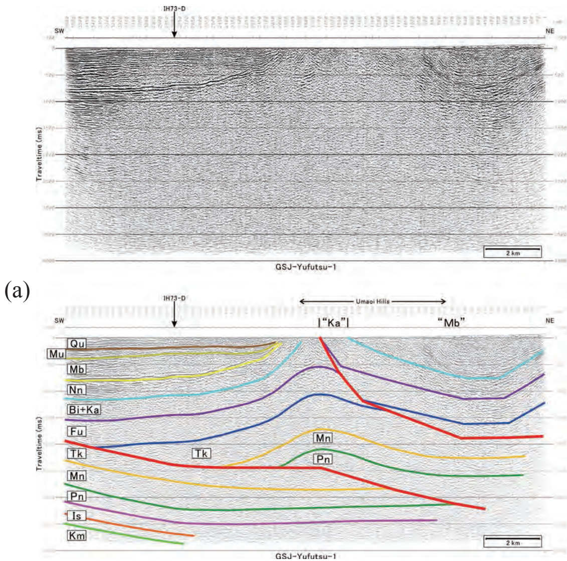
第 16 図 GSJ 勇払測線 1 の解釈図 (a) 通常処理マイグレーション後時間断面. (b) MDRS 処理マイグレーション後時間断面. (c) MDRS 処理深度断面. 上段: 元の断面. 下段: 解釈断面. 地層名の略号については第 3 図参照. Fig.16 Interpreted seismic sections of GSJ-Yufutsu-1. (a) Conventional migrated time section. (b) MDRS migrated time section. (c) MDRS depth section. Top : original section. Bottom: interpreted section. For abbreviations, see Fig.3.
