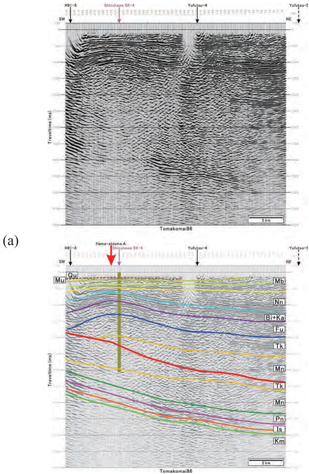
第 15 図 苫小牧 86 測線の解釈図 (a) 通常処理マイグレーション後時間断面. (b)MDRS 処理マイグレーション後時間断面. (c)通常処理深度断面. (d)MDRS 処理深度断面. 上段:元の断面. 下段:解釈断面. 地層名の略号については第 3 図参照.
