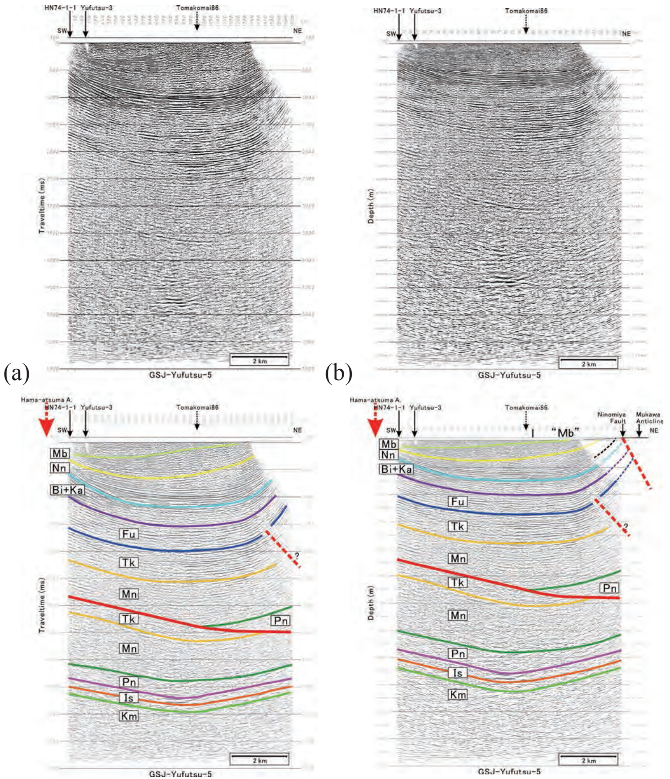
第 20 図 GSJ 勇払測線 5 の解釈図 (a) 通常処理マイグレーション後時間断面. (b) 通常処理深度断面. 上段：元の断面. 下段：解釈断面. 地層名の略号については第 3 図参照. Fig.20 Interpreted seismic section of GSJ-Yufutsu-5. (a) Conventional migrated time section. (b) Conventional depth section. Top : original section. Bottom: interpreted section. For abbreviations, see Fig.3.
