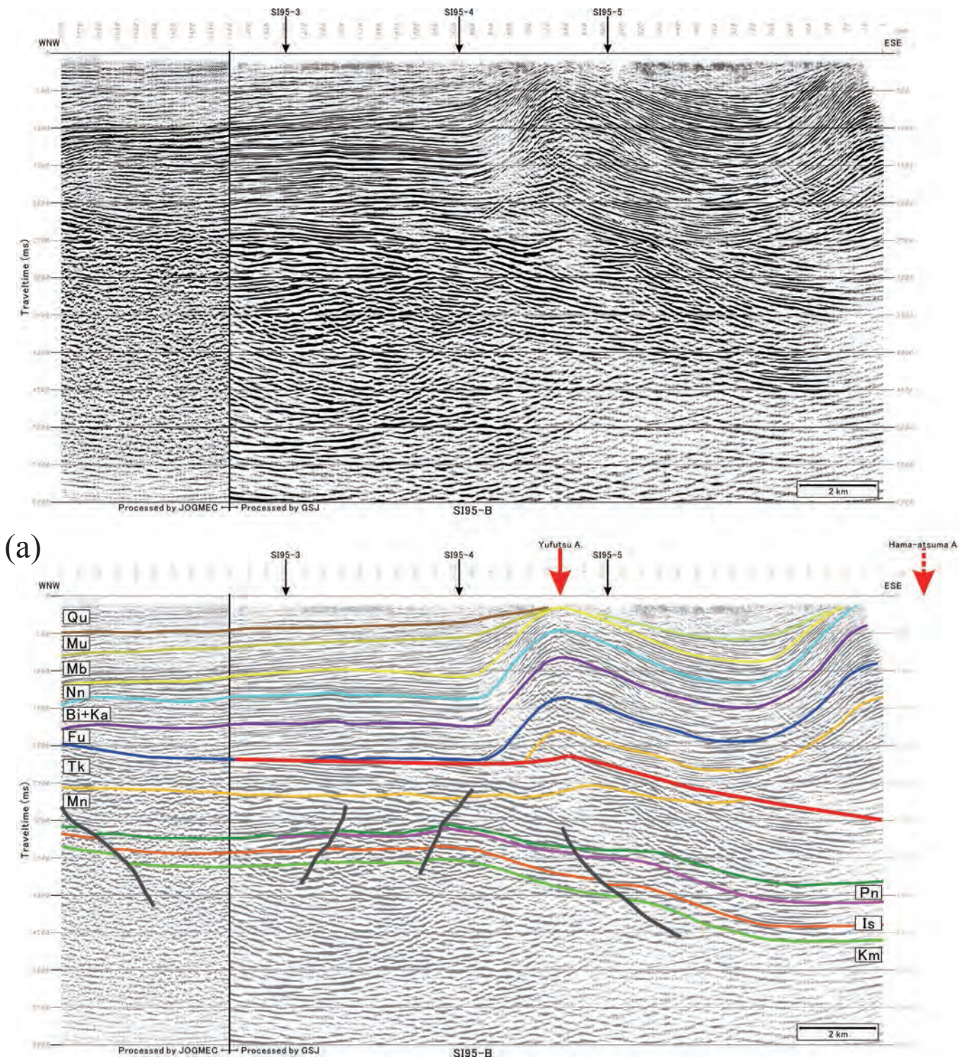
第4図 SI95-B 測線の解釈図 (a) 通常処理マイグレーション後時間断面. (b)MDRS 処理マイグレーション後時間断面. 上段: 元の断面. 下段: 解釈断面. 地層名の略号については第3図参照.
