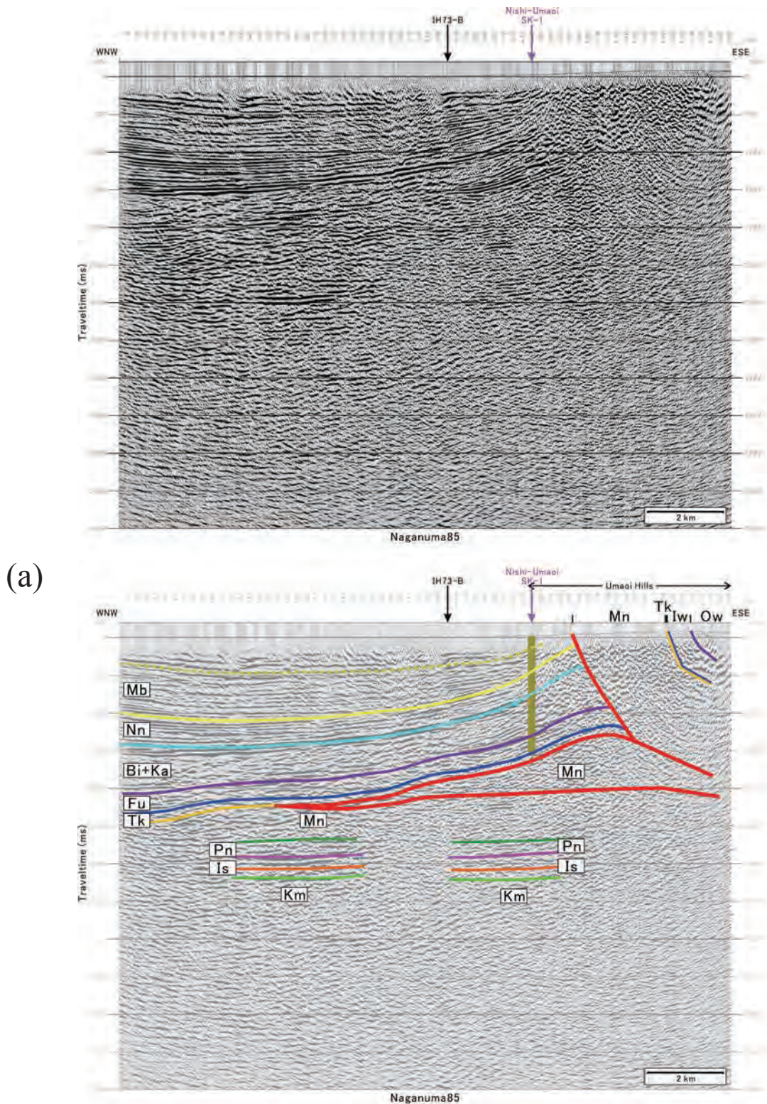
第14図 長沼85測線の解釈図 (a)通常処理マイグレーション後時間断面。(b)MDRS処理マイグレーション後時間断面。(c)通常処理深度断面。(d)MDRS処理深度断面。上段：元の断面。下段：解釈断面。地層名の略号については第3図参照。
