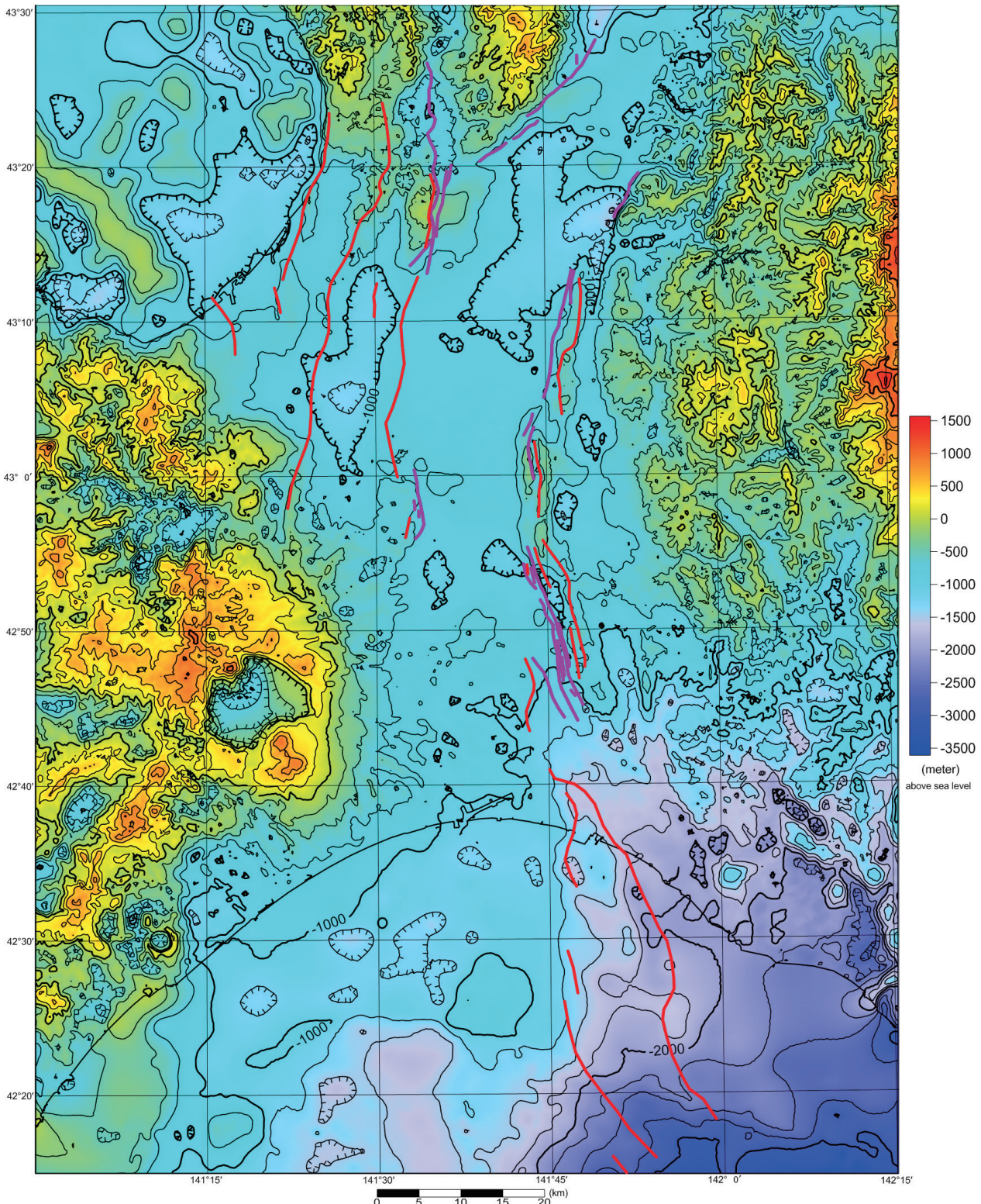
第 3 図 石狩低地帯及び周辺地域の重力基盤。密度差を 0.5\text{g}/\text{cm}^3 とし、コンター間隔は 250m で表示した。コンターの数値は海拔。紫色と赤色の太い実線は第 1 図と同じ。
