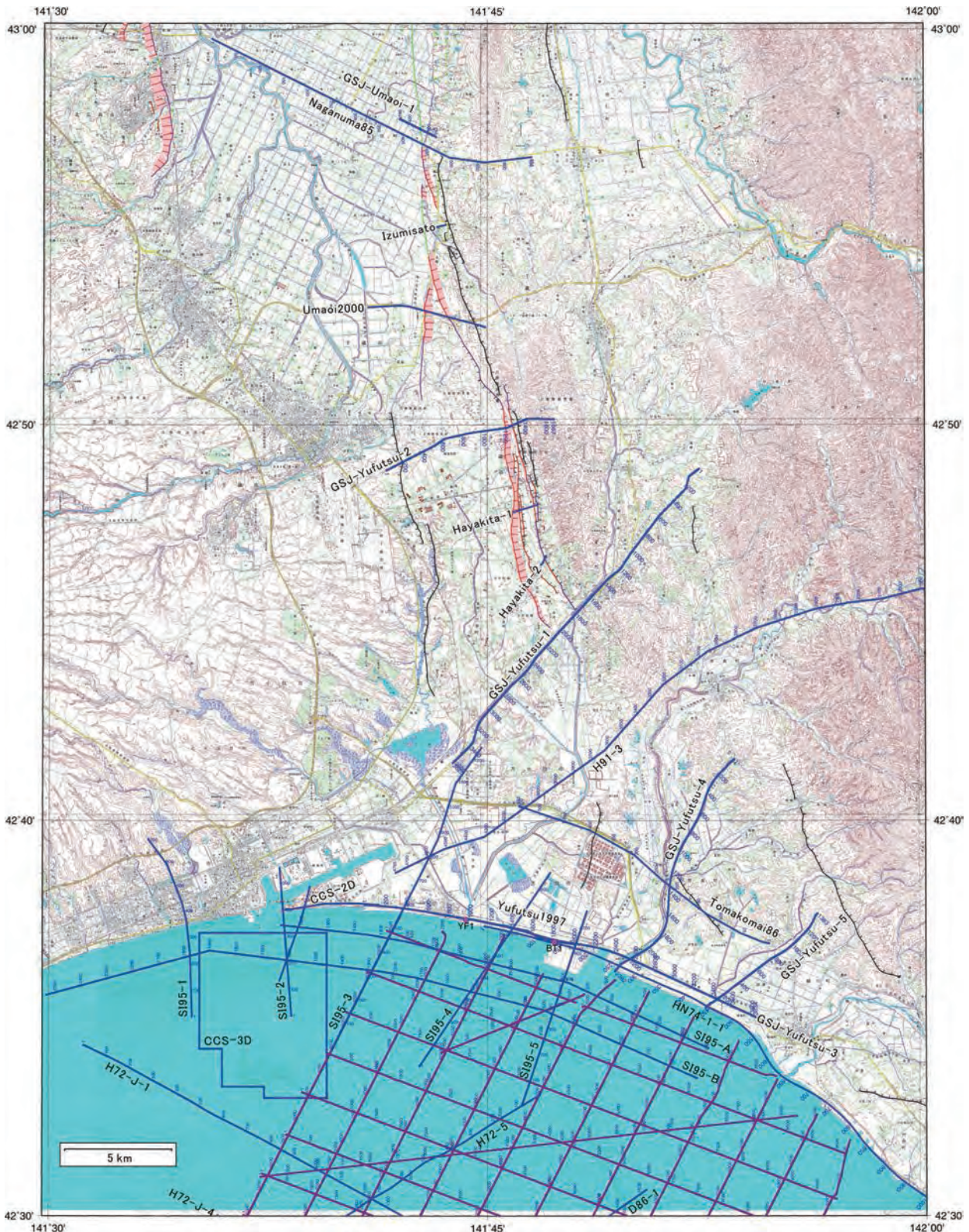
第2図 石狩低地南部周辺の反射法地震探査測線。青線：反射法地震探査測線。紫線：佐藤(2013; 2014)の高分解能音波探査測線。海底地形：日本水路協会発行海底地形デジタルデータ M7006「津軽海峡東部」。活断層データ：中田・今泉編(2002)による。基図：国土地理院数値地図 50,000「苫小牧」、「鶴川」、「千歳」、「早来」、「恵庭」、「追分」。
