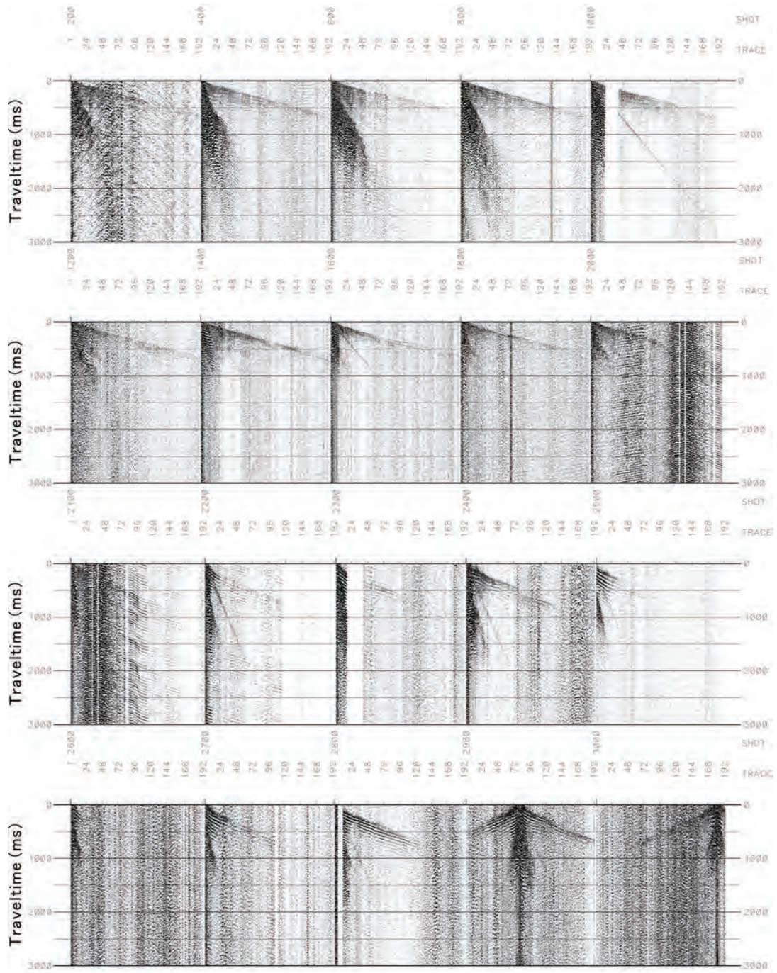
第9図 GSJ 勇払測線3の発震記録例. Fig.9 Examples of shot gathers of the GSJ-Yufutsu-3.
