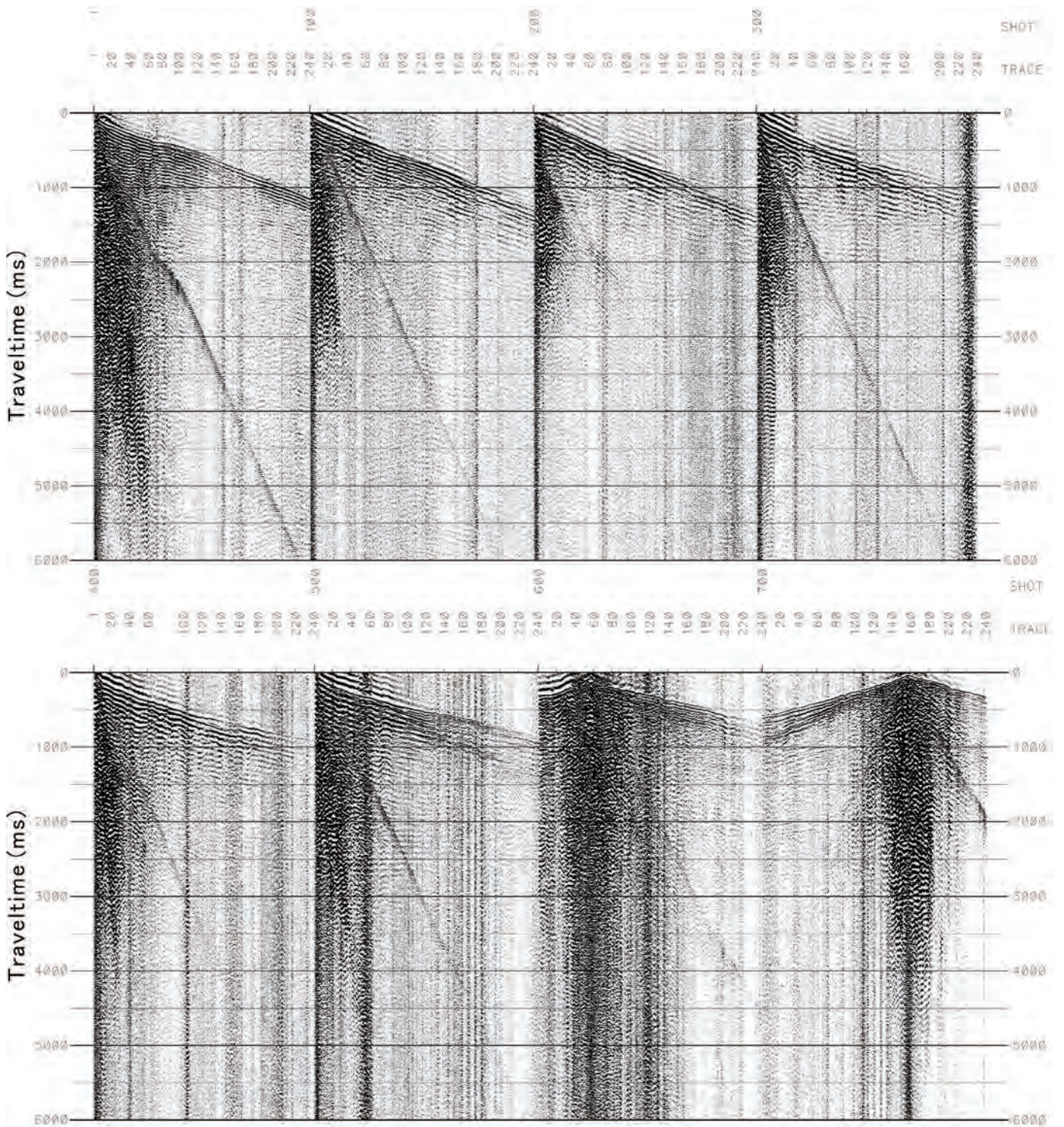
第 11 図 GSI 勇払測線 5 の発震記録例. Fig.11 Examples of shot gathers of the GSI-Yufutsu-5.
