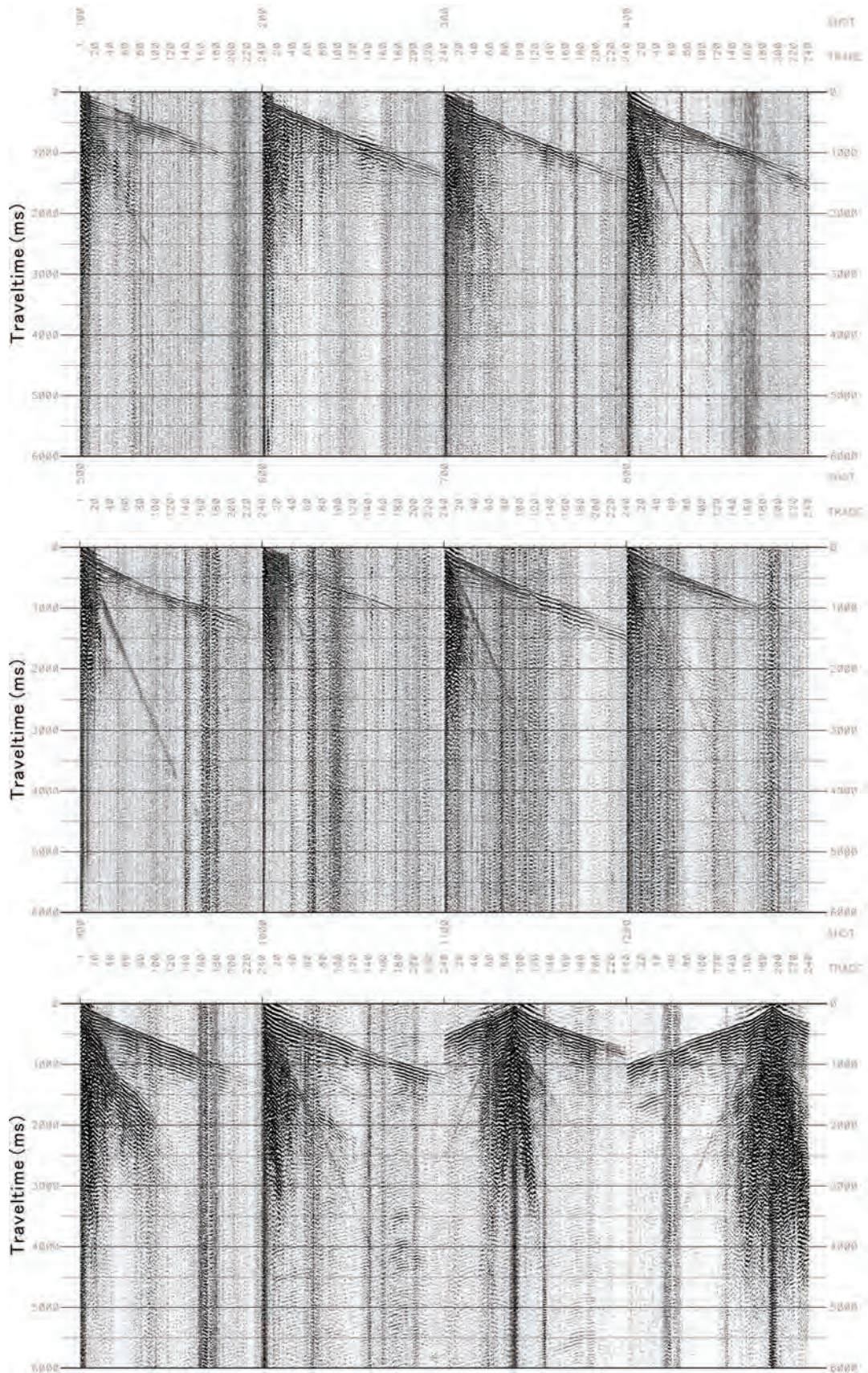
第 10 図 GSI 勇払測線 4 の発震記録例。 Fig.10 Examples of shot gathers of the GSI-Yufutsu-4.
