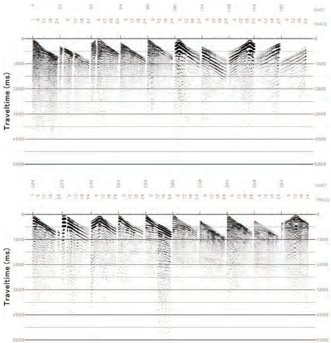
第 12 図 HN74-1-1 測線の発震記録例. Fig.12 Examples of shot gathers of the HN74-1-1.
