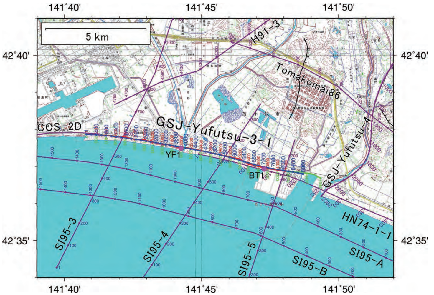
第5図 GSJ 勇払測線 3-1 の詳細測線図 説明は第4図参照。
