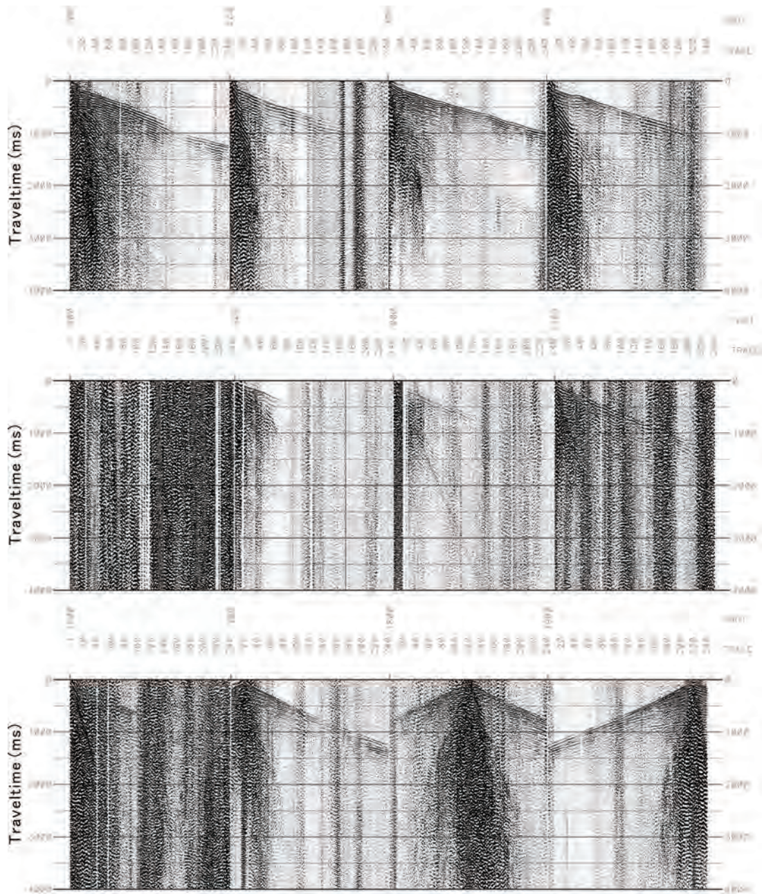
第7図 GSJ 勇払測線 1 の発震記録例. Fig.7 Examples of shot gathers of the GSJ-Yufutsu-1.
