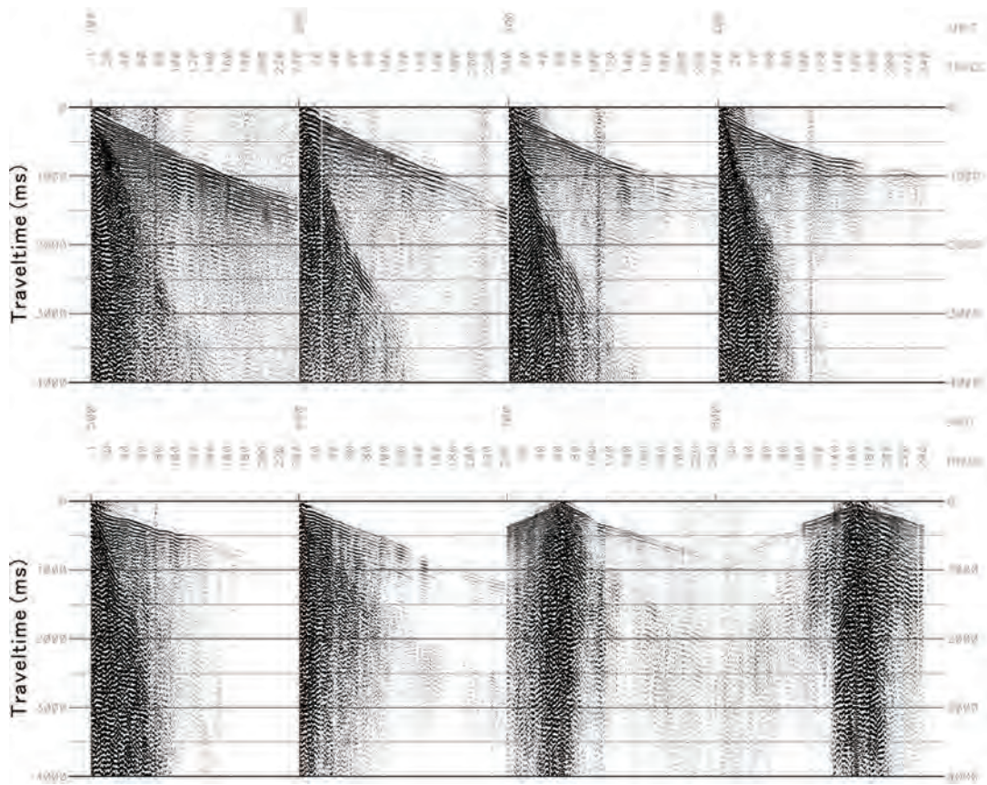
第 8 図 GSI 勇払測線 2 の発震記録例. Fig.8 Examples of shot gathers of the GSI-Yufutsu-2.
