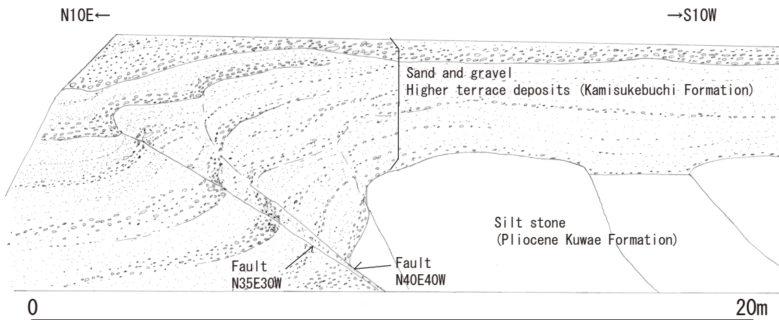
第9図 葡萄山地南方延長・臥牛山断層の第四紀後期の活動を示す露頭。A：中部更新統・坪根層と鮮新統・鉾江層を境する正断層，およびそれらを不整合に覆う高位段丘堆積物（上助淵層）。位置は第7図のLoc.1。B：高位段丘堆積物を変位させる低角西傾斜逆断層。位置は第7図のLoc.2。
