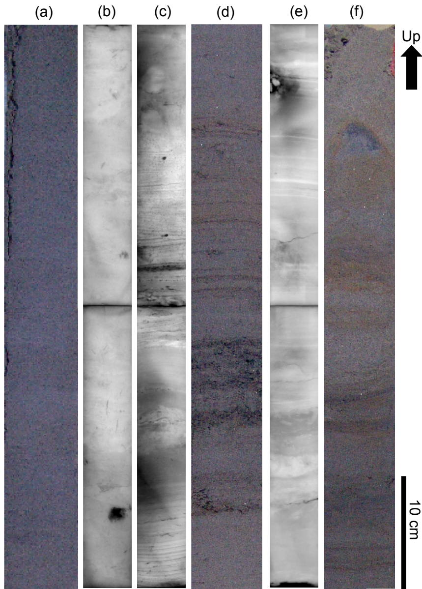
第7図 Ni09-AG ボーリング試料写真. (a) 31.0~31.5 m ; AG3 の均質なシルト (b) 28.25~28.75 m ; AG3 の均質なシルト層. 軟X線写真(陰影) (c) 22.25~22.75 m ; AG2 の斜交層理が確認される極細粒砂. 軟X線写真(陰影) (d) 21.7~21.2 m ; AG2 の斜交層理が確認される極細粒砂層 (g) 2.5~3.0 m ; AG1 の斜交層理が確認される細粒砂. 軟X線写真(陰影) (h) 1.0~1.5 m ; AG1 の斜交層理が確認される細粒砂.
