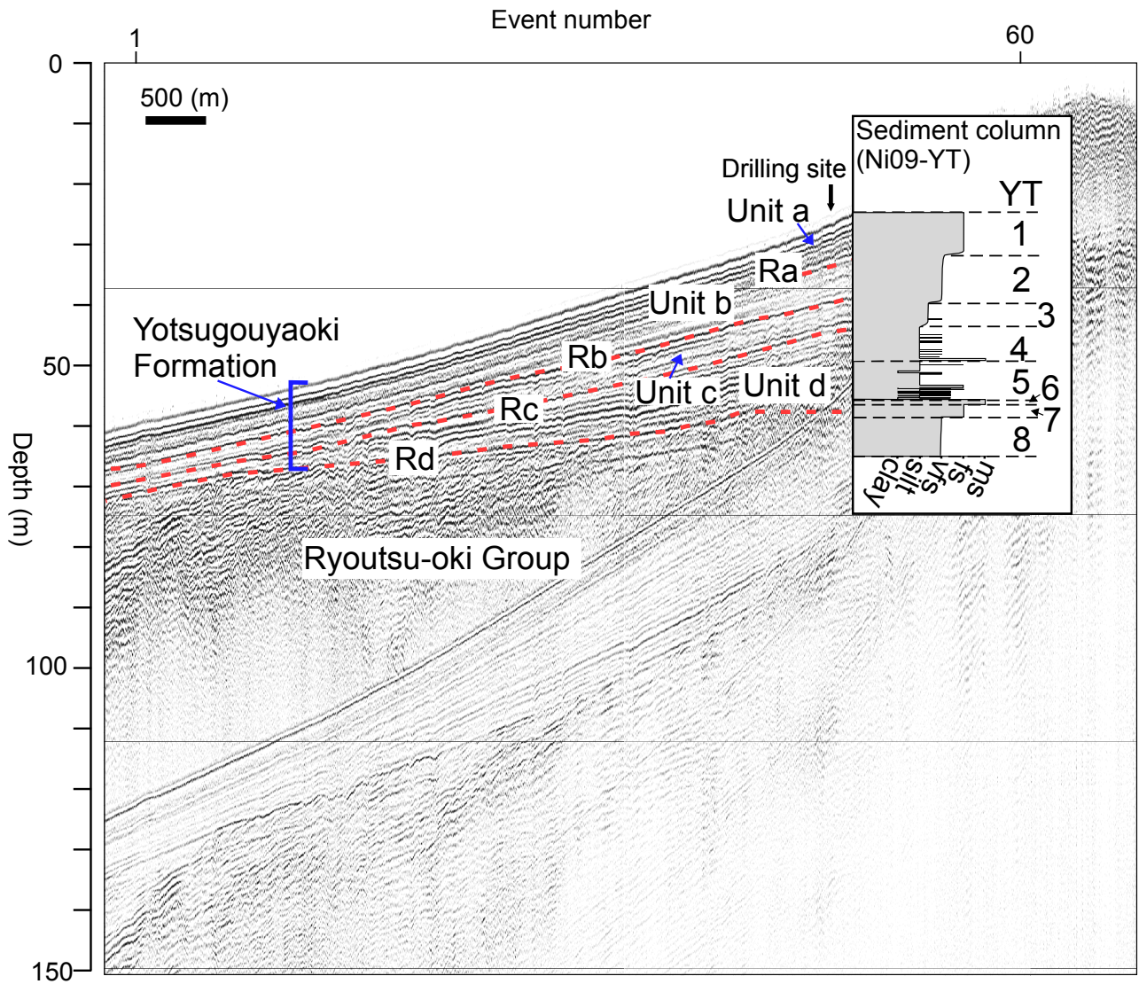
第5図 測線 E202 音波探査記録と Ni09-YT との対比図。
