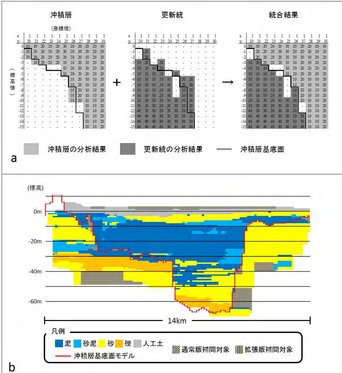
第 15 図 三次元グリッドモデルの統合処理過程の概念図 Fig.15 Schematic image displaying the method used to integrate the 3D grid models
