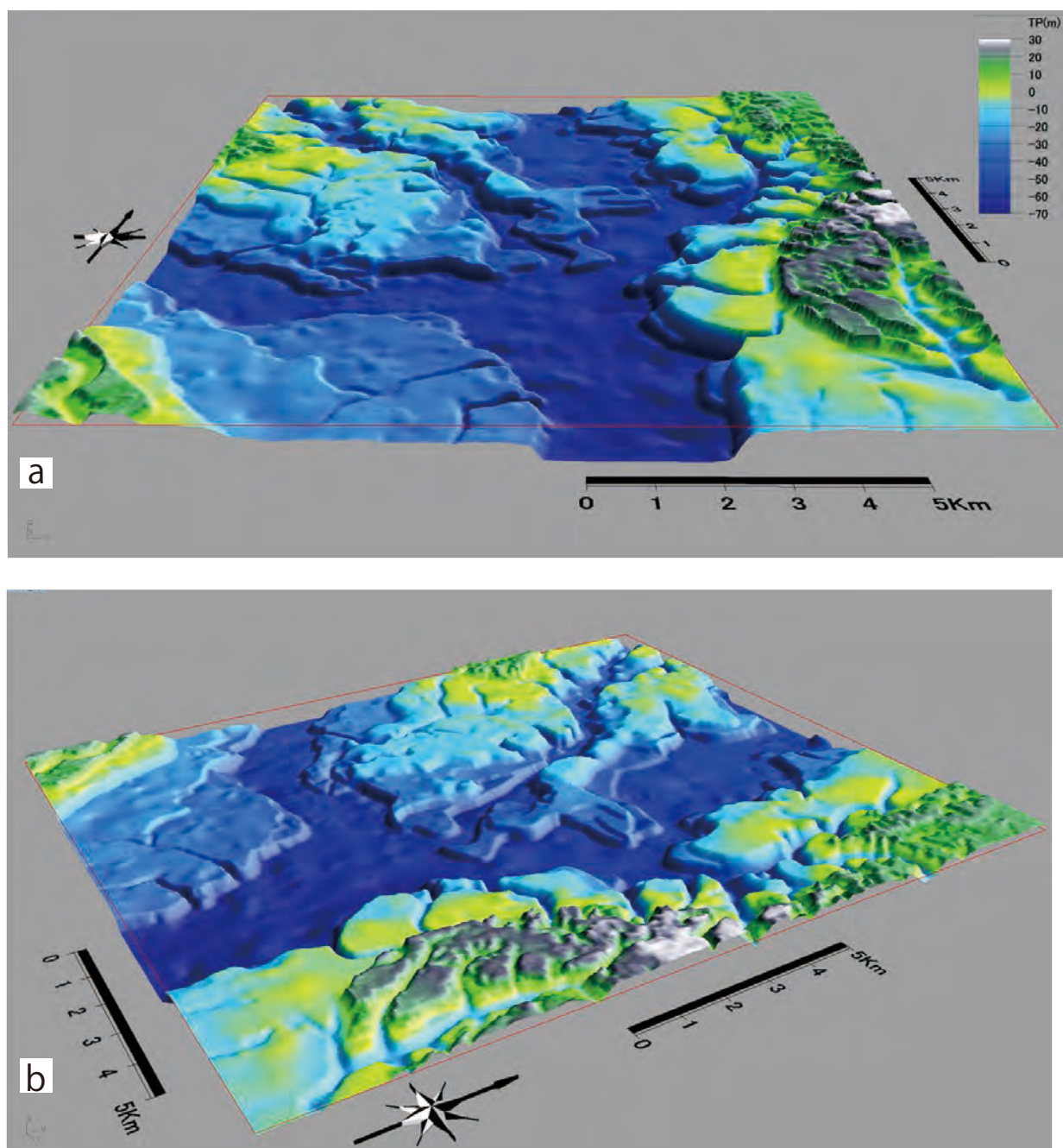
第 11 図 第 10 図の沖積層基底面モデルの鳥瞰図 (木村ほか, 2013)
